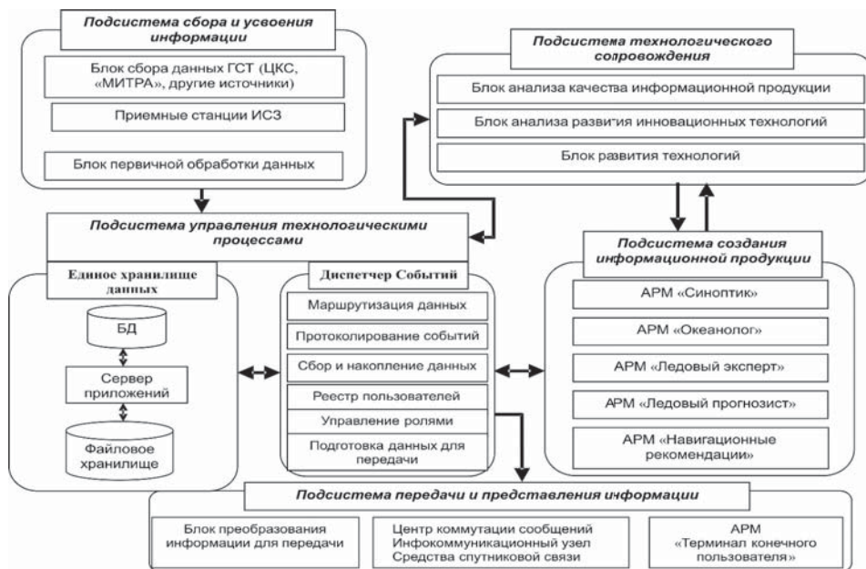
Рис. 1. Структурная схема комплекса АКМОН
