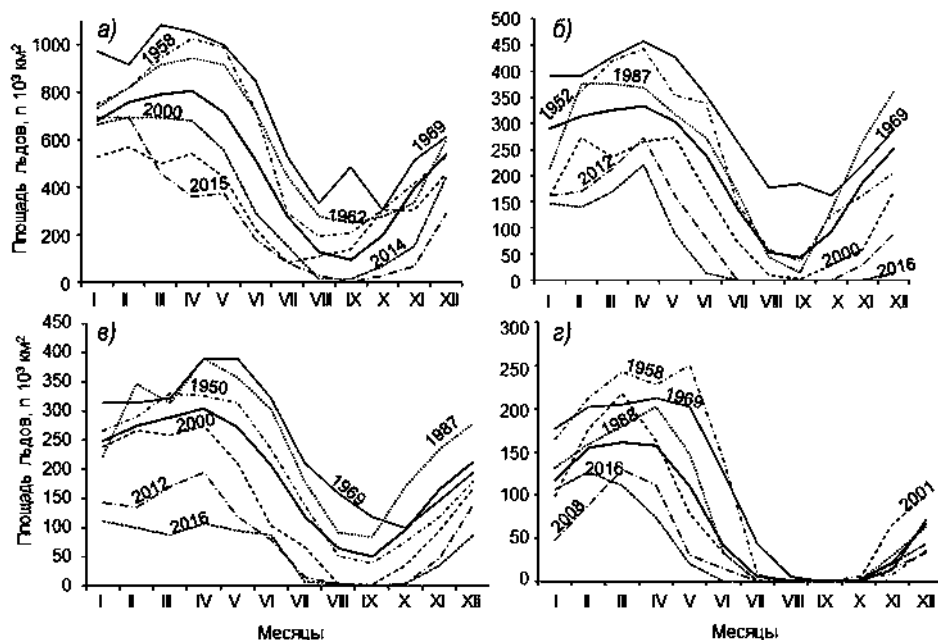
Рис. 2. Изменения площади ледяного покрова на всей акватории Баренцева моря ( a ), в западном ( б ), северо-восточном ( в ) и юго-восточном ( г ) районах в характерные годы (тонкие линии) и среднеегодовое значение за период 1928–2021 гг. (жирная линия)
