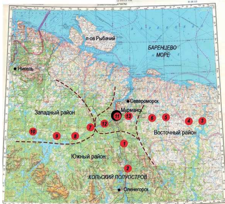
Рис. 1. Схема района работ. Кружками показаны станции отбора проб свежеснегавшего снега, нумерация соответствует таблице 1
