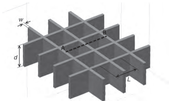
Рис. 3. Общий вид объемной модели полигонально-жильной структуры: серым цветом обозначены ледяные жилы, прозрачное заполнение между ними — мерзлый грунт; w — ширина жил, d — высота жил, L — расстояние между центрами полигонов; AB — линия профиля, на которой приводятся результаты расчета на рис. 5–8.
