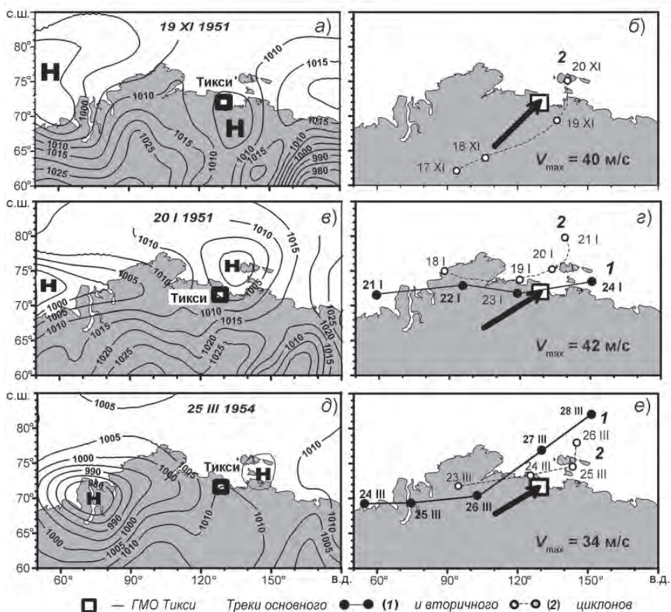
Рис. 8. Синоптические условия штормов 19 ноября, 20 января 1951 г. и 25 марта 1954 г. в районе Тикси: а, в, д — давление на уровне моря (гПа); б, з, е — векторы максимальной скорости ветра и датированные (число и месяц) траектории центров основного (1) и вторичного (2) циклонов.
