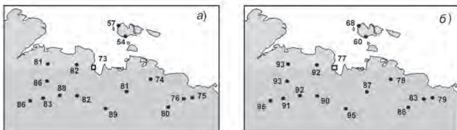
Рис. 6. Повторяемость (а, %) и годовой максимум (б) числа дней с температурой T \leq -30 °С с ноября по март за 1978–2010 гг.
