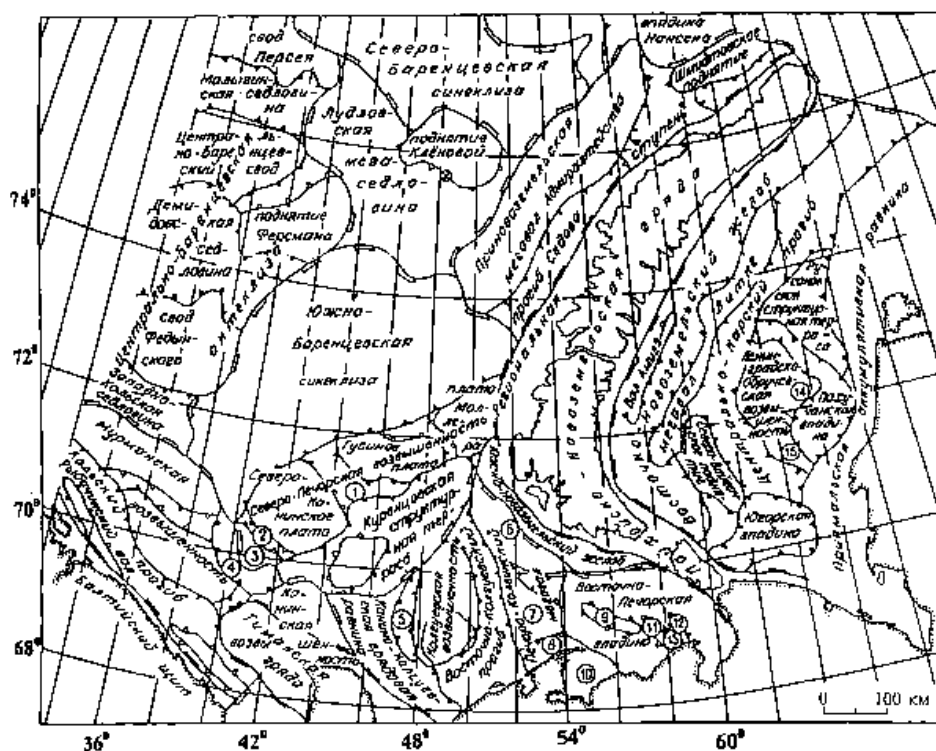
Рис. 2. Морфоструктурная схема Западно-Арктического шельфа России по В.В. Назимову.
