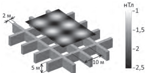
Рис. 9. Пример синтетического распределения аномального модуля вектора магнитной индукции ( F ) над полигонально-жильной структурой на высоте 3 м; ширина жил — w = 2 , высота жил — d = 5 м, расстояние между центрами полигонов — L = 10 м, магнитная восприимчивость мерзлого грунта — K = 10^{-3} СИ.
