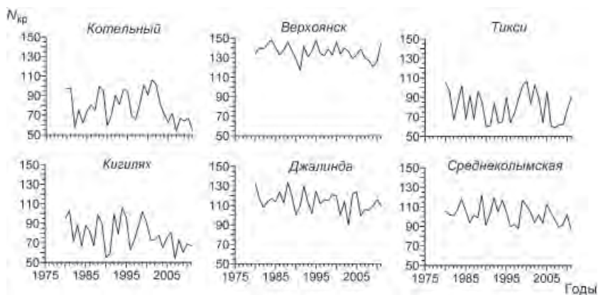
Рис. 5. Пространственно-временная изменчивость числа дней с температурой ниже -30\text{ }^{\circ}\text{C} за 1978–2010 гг. в холодный сезон с ноября по март.
