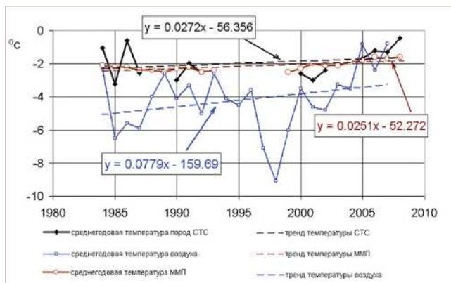
Рис. 2. Изменение среднегодовой температуры воздуха, пород деятельного слоя и многолетнемерзлых пород в скв. 59 на стационаре Болванский. Линии тренда и уравнения регрессии
