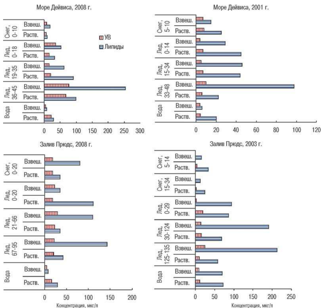
Рис. 4. Перераспределение липидов и УВ между растворенной и взвешенной формами в припайных льдах
