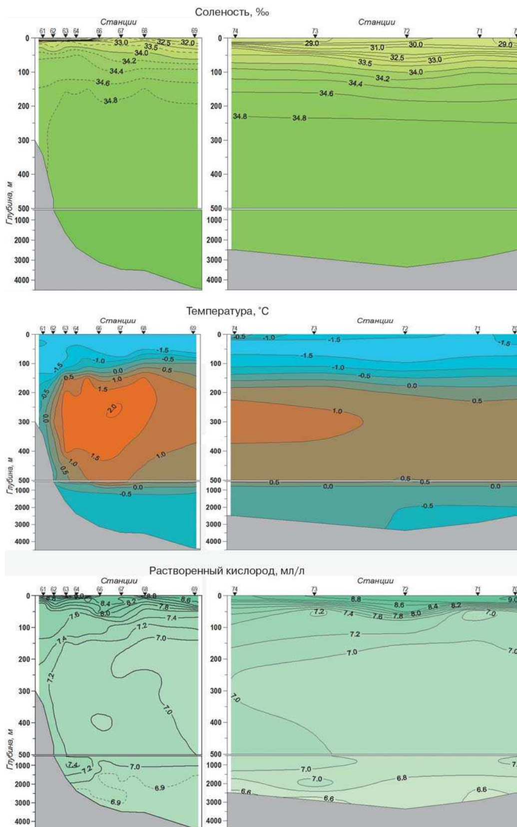
Вертикальное распределение температуры, солености и растворенного кислорода на разрезах
