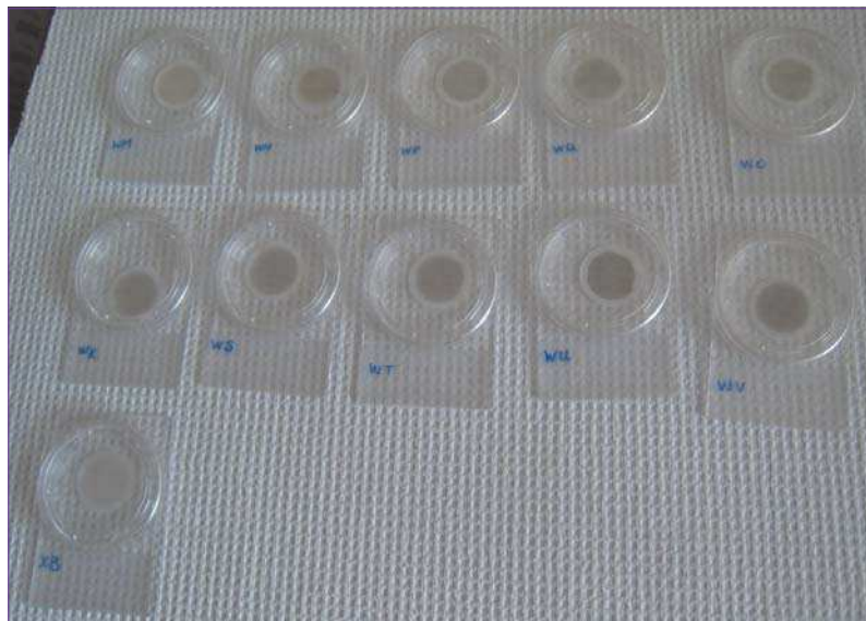
Образцы осевших на фильтры аэрозольных загрязнений проб снега в окрестностях Тикси. Большая степень почернения означает более высокий уровень загрязнения
