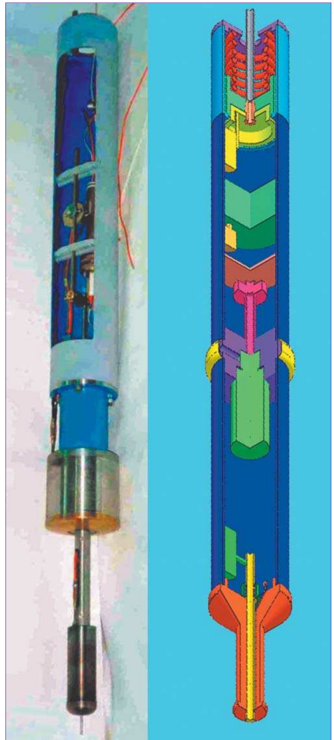
Внешний вид и схематический разрез рабочего макета теплового прибора ТБПО-132, разработанного для проникновения в подледниковое озеро Восток
