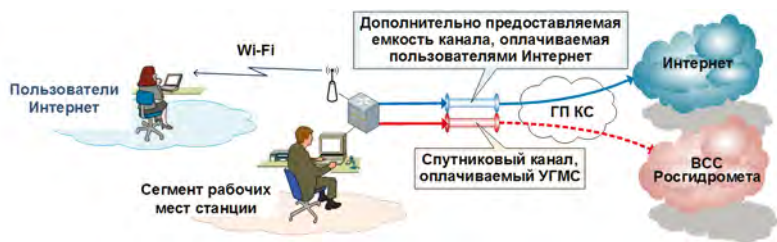
Рис. 6. Организация доступа в Интернет персонала ТДС (НЭС).
