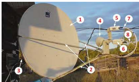
Рис. 8. Внешнее оборудование станции VSAT.
