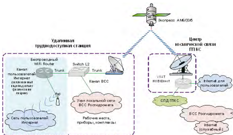
Рис. 7. Структурная схема подключения удаленных станций к БСС Росгидромета и Интернет по спутниковому каналу VSAT.
