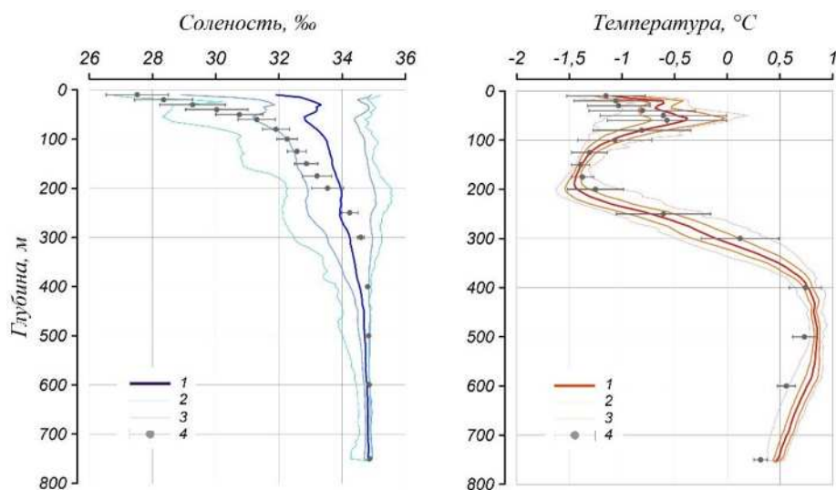
Рис. 3.1.4. Вертикальное распределение солёности и температуры воды в Канадской глубоководной котловине в сентябре 2024 г. по результатам измерений профилографа ИТР 143. Условные обозначения см. рис. 3.1.2.
