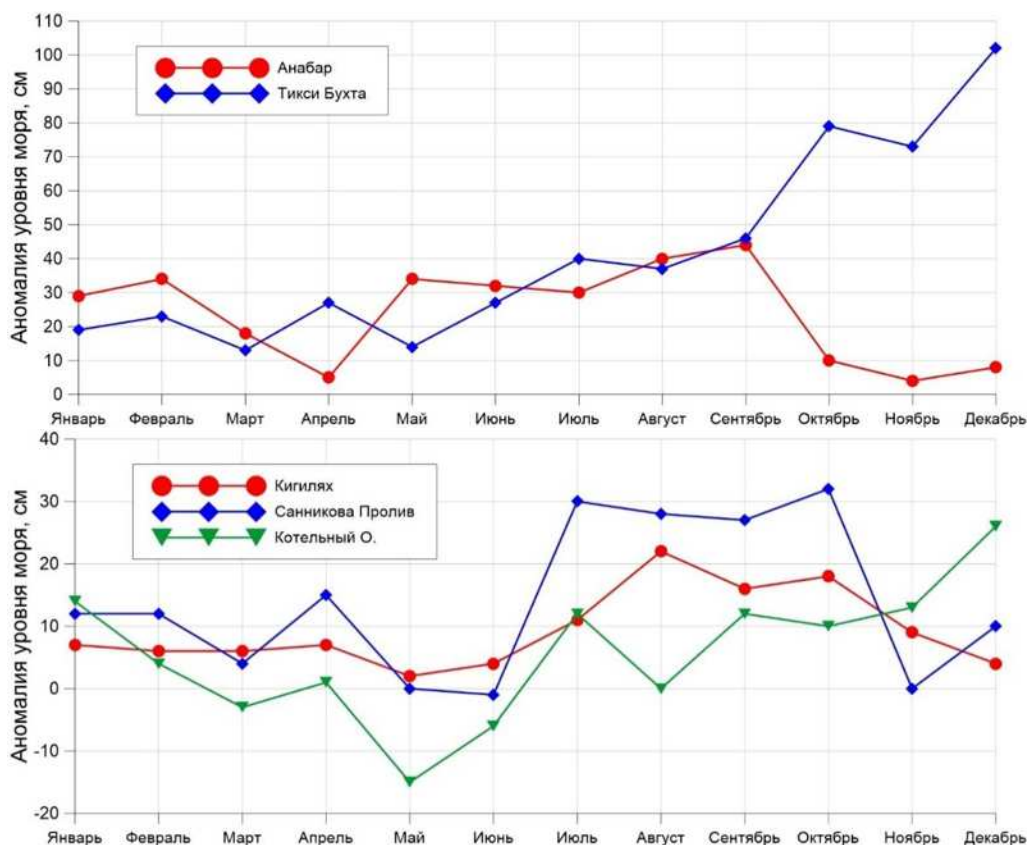
Рис. 3.2.2. Изменения среднemesячного значения уровня на станциях моря Лаптевых в 2024 г.
