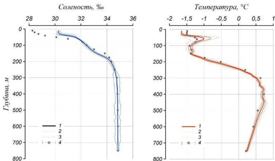
Рис. 3.1.3. Вертикальное распределение солености и температуры воды в Канадской глубоководной котловине в апреле — мае 2024 г. по результатам измерений профилографа ИТР 139.
