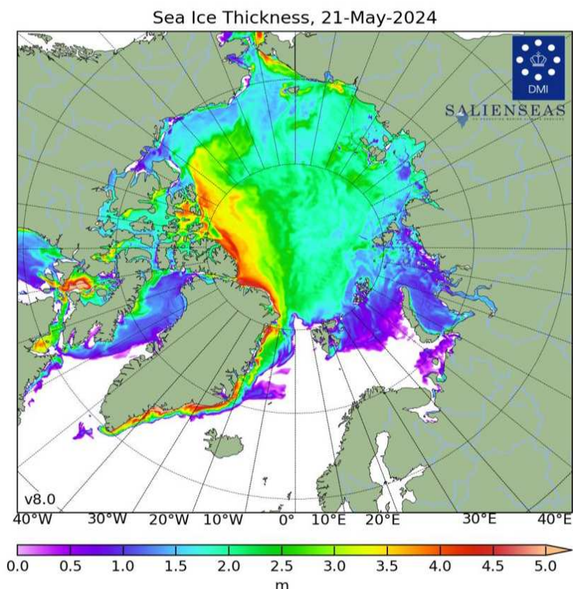
Рис. 2.2.7. Поля распределения средневзвешенной толщины льда совместной модели морской лед–океан HYCOM/CICE Датского метеорологического института 21.05.2024 г.
