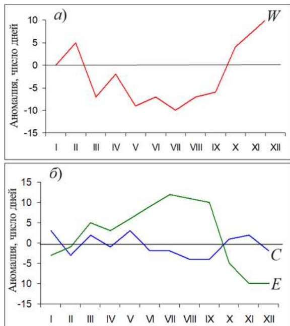
Рис. 1.1. Годовой ход среднемесячных значений аномалии числа дней с зональной (а) и меридиональными (б) формами циркуляции в атлантико-евразийском секторе в 2024 г. W — западная (зональная) форма, C — меридиональная форма, E — восточная (меридиональная) форма.
