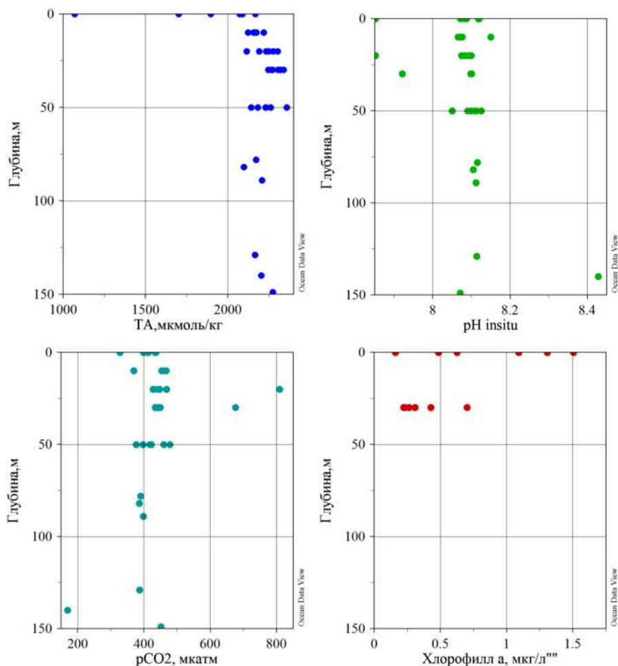
Рис. 3.4.1. Вертикальное распределение карбонатных параметров (общей щелочности, pH, pCO 2 ) и концентраций хлорофилла «а» в заливе Грёнфьорд, 07.09.2024 г.
