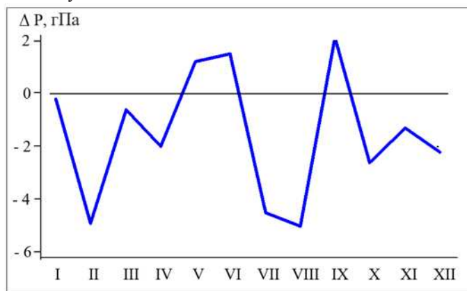
Рис. 1.9. Среднемесячные значения аномалии давления в январе — декабре 2024 г. в центральном полярном районе Арктики
