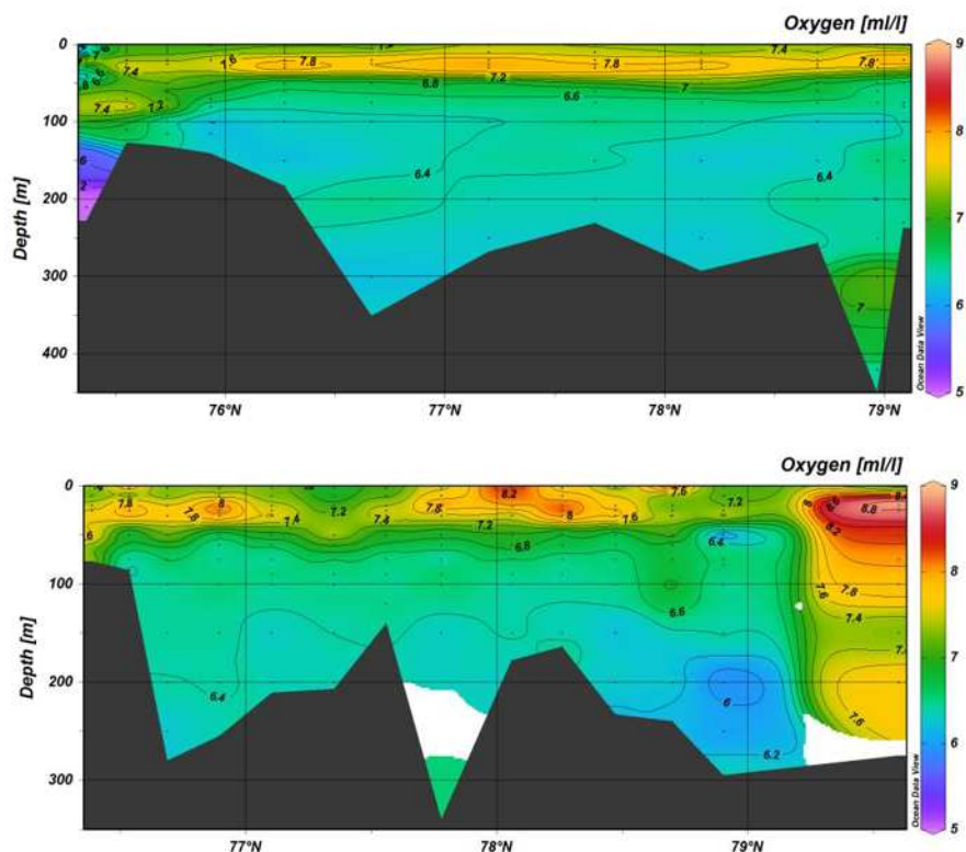
Рис. 3.4.6. Распределение растворенного кислорода (мл/л) в северо-восточной части Баренцева моря. Разрез 1, п-ов Адмиралтейство – о-в Виктория (сверху), Разрез 2, о-в Нортбрук – бухта Русская гавань (снизу) по данным рейса НИС «Профессор Молчанов» 2024 г.
