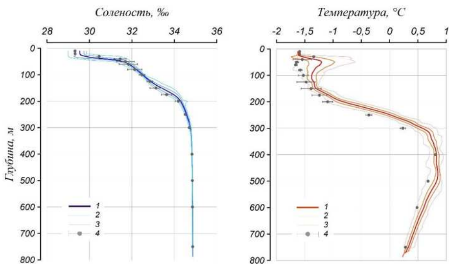
Рис. 3.1.2. Вертикальное распределение солености и температуры воды в Канадской глубоководной котловине в январе — марте 2024 г. по результатам измерений профилографа ИТР 139.
