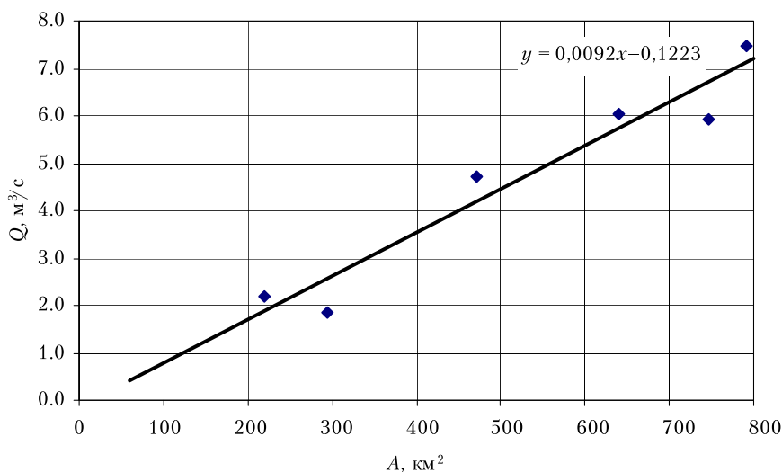
Рис. А.35. Зависимость среднегодового расхода воды ( \text{m}^3/\text{s} ) от площади водосбора ( \text{km}^2 )
