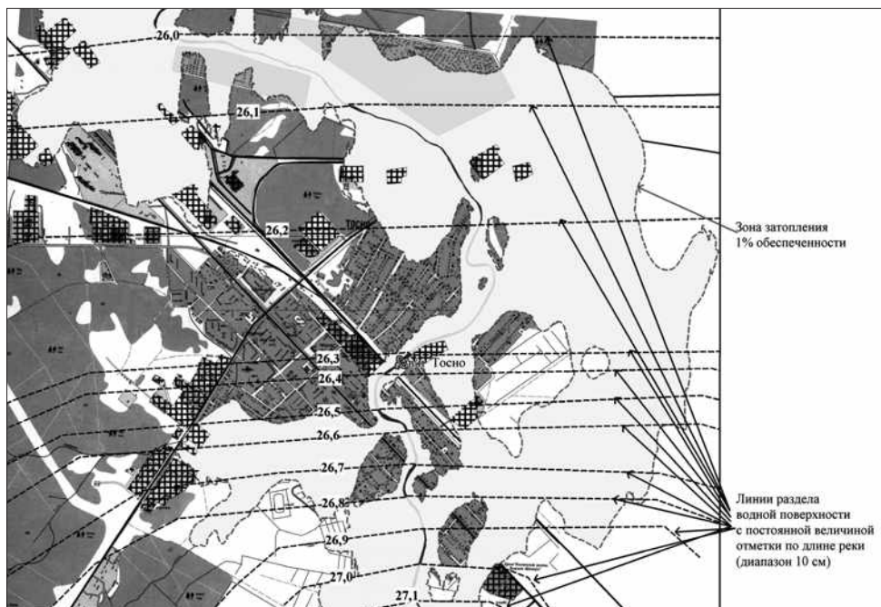
Рис. А.45. Схема наведения линий раздела водной поверхности с постоянной величиной отметки по длине реки
