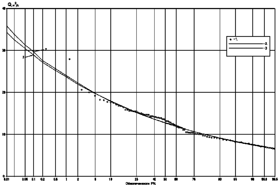
Рис. А. 18. Кривая обеспеченности минимального зимнего стока р. Обь — д. Медведево 1 — эмпирические точки, 2 — кривая обеспеченности по параметрам, рассчитанным по ряду, 3 — кривая обеспеченности по параметрам, обобщенным по району
