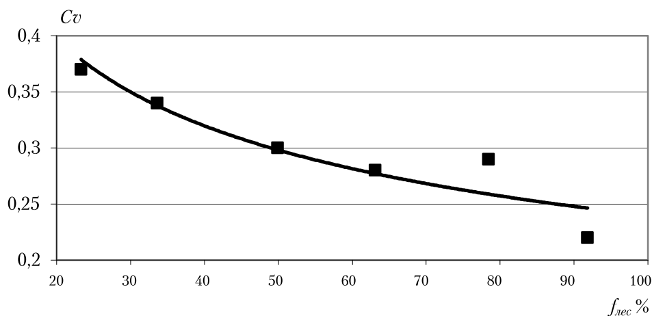
Рис. А.9. Зависимость коэффициентов вариации годового стока от залесенности водосборов рек Северо-запада и Севера ЕТР
