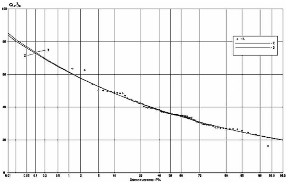
Рис. А. 19. Кривая обеспеченности минимального летнего стока р. Обь — д. Медведево 1 — эмпирические точки, 2 — кривая обеспеченности по параметрам, рассчитанным по ряду, 3 — кривая обеспеченности по параметрам, обобщенным по району
