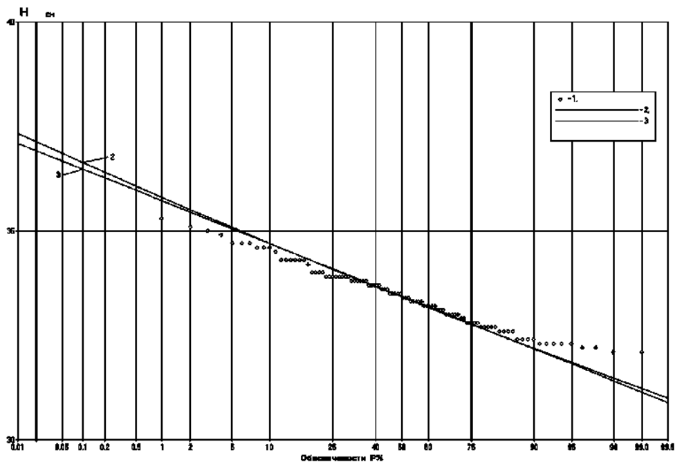
Рис. А.24. Кривая обеспеченности минимальных зимних уровней воды р. Обь — д. Медведево 1 — эмпирические точки, 2 — кривая обеспеченности, рассчитанная по параметрам ряда, 3 — кривая обеспеченности при C_s/C_v=0,01
