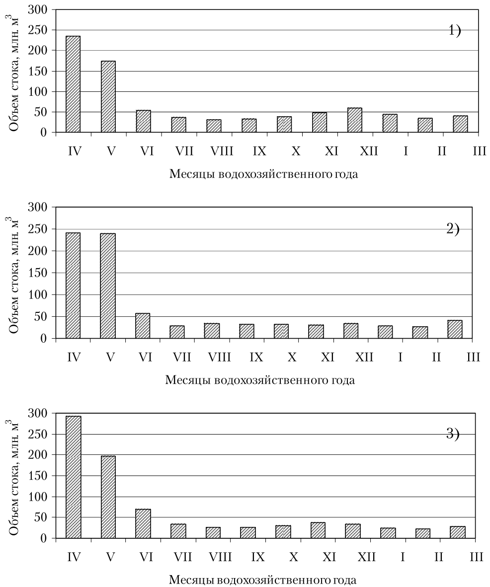
Рис. А.26. Расчетное внутригодовое распределение стока реки Луга — ст. Толмачево для года обеспеченностью P = 90\% ; 1 — метод среднего распределения стока за годы характерной градации водности, 2 — метод реального года, 3 — метод компоновки
