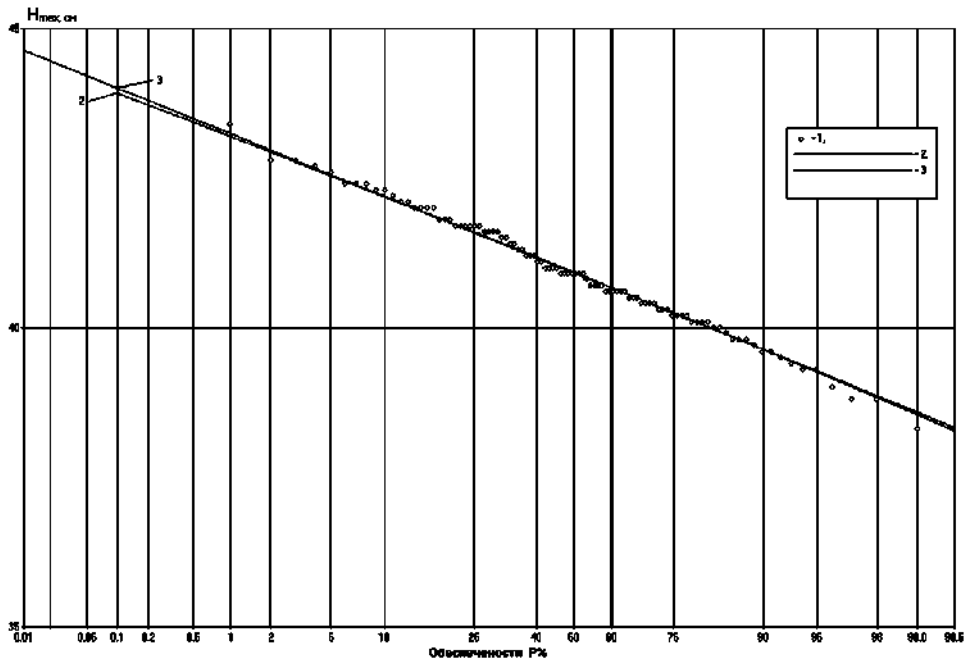
Рис. А.21. Кривая обеспеченности максимальных уровней воды р. Обь — д. Медведево 1 — эмпирические точки, 2 — кривая обеспеченности, рассчитанная по параметрам ряда, 3 — кривая обеспеченности при C_s/C_v=0,01
