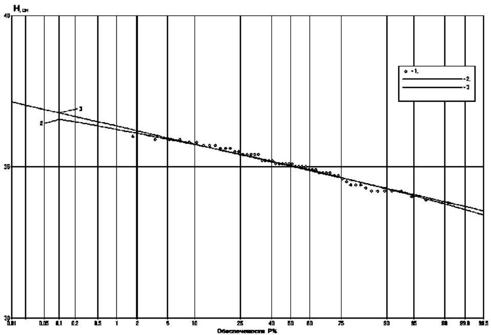
Рис. А.22. Кривая обеспеченности среднегодовых уровней р. Обь — д.Медведево 1 — эмпирические точки, 2 — кривая обеспеченности по параметрам, рассчитанным по ряду, 3 — кривая обеспеченности при C_s/C_v=0,01
