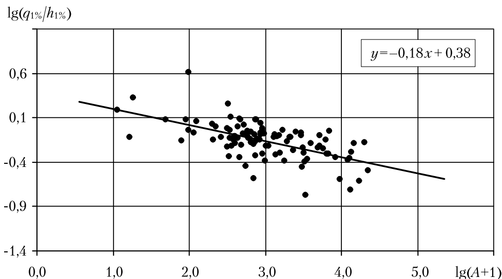
Рис. А.27. Районная редукционная зависимость максимального весеннего стока для рек Северо-Запада РФ.
