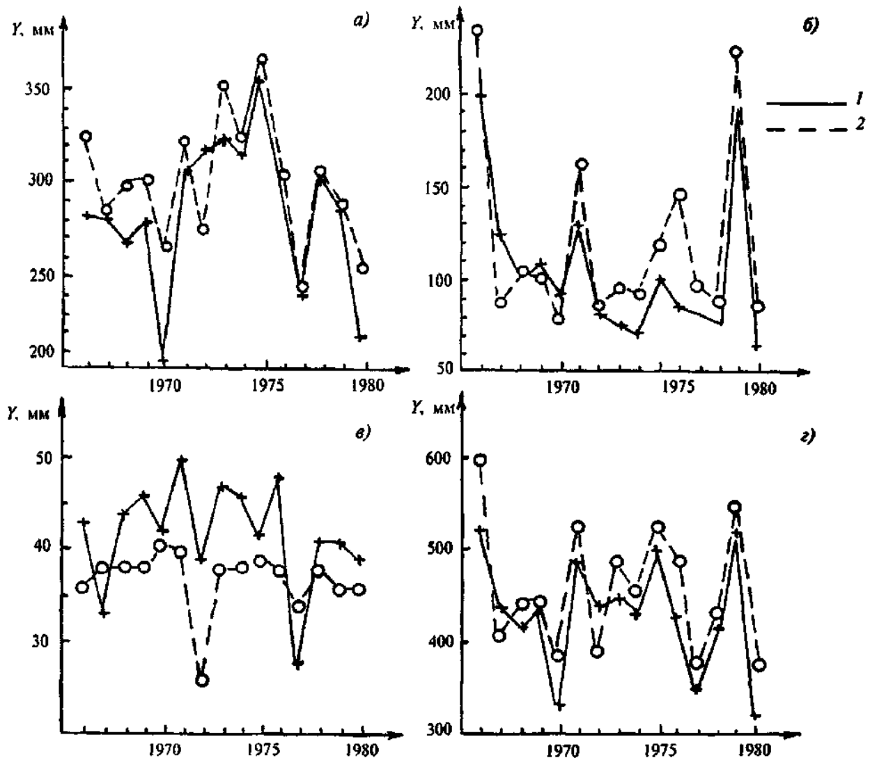
а) — весеннее половодье; б) — летне-осенний сезон; в) — сезон зимней межени; г) — годово́й сток Рисунок А.5 — Сравнение фактических (1) и рассчитанных (2) слоев стока р. Вага — с. Усть-Сюма
