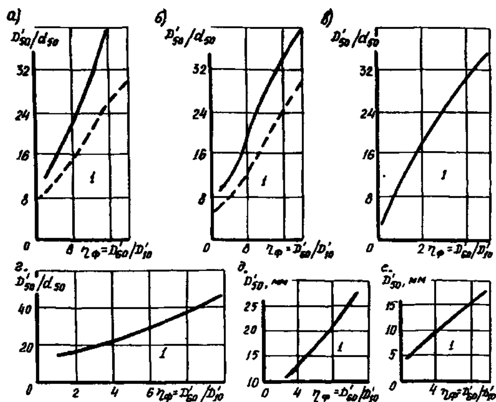
Рис. П 7 11 Графики для подбора первого слоя фильтра (сплошная кривая характеризует усредненный состав грунтов, пунктирная—граничный).
