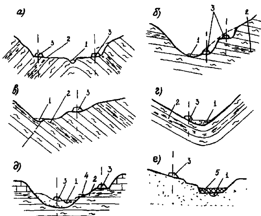
Рис П31 Рекомендуемые варианты трассирования дороги (долинным ходом) в наледных районах полувыемкой на разной высоте склона (а, б, в) и насыпью в прирусловой части поймы (г, д, е).
