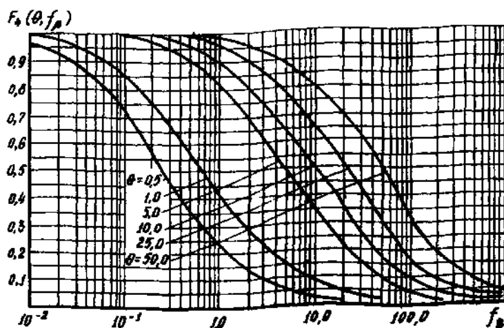
Рис П 78 Графики функции F_4(Q, f_3)
