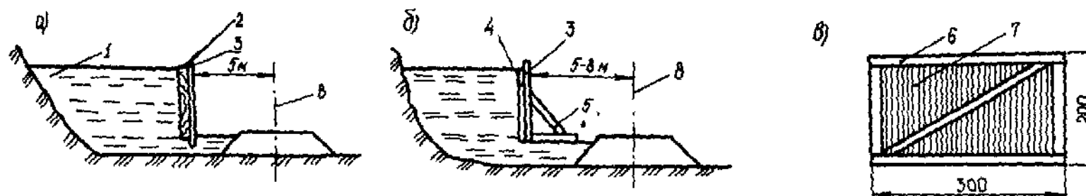
Рис 2.10 Схема расположения противоналедных заборов и щитов а—щпальный забор, б—забор из щитов с подкосами, в—схема щита, 1—наледь, 2—шпалы, 3—стойки, 4—щит, 5—подкос, 6—каркас из досок, 7—рубероид 2 слоя, 8—ось дороги
