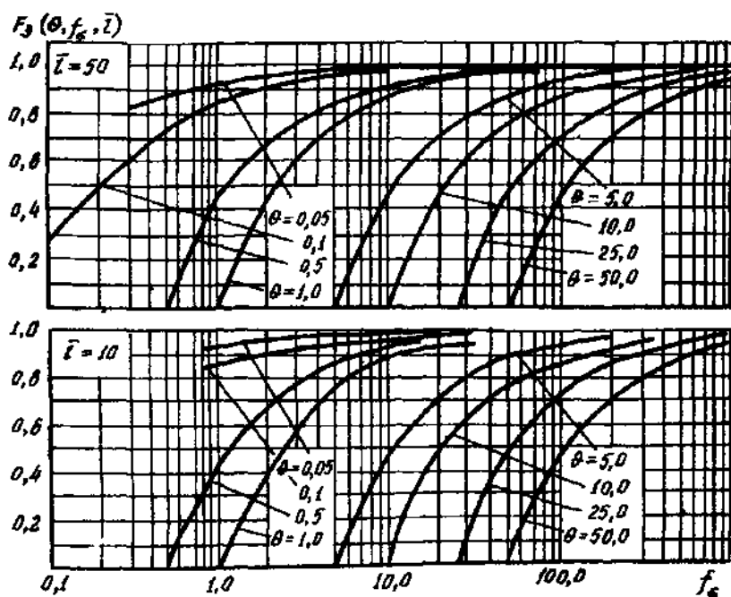
Рис П77 Графики функции F_3(Q, f_a, \bar{l})
