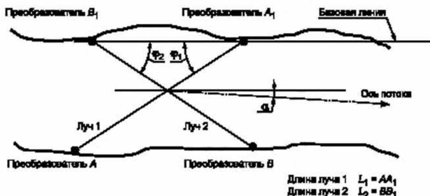
Рисунок 1 — Схема расположения преобразователей с пересекающимися лучами
