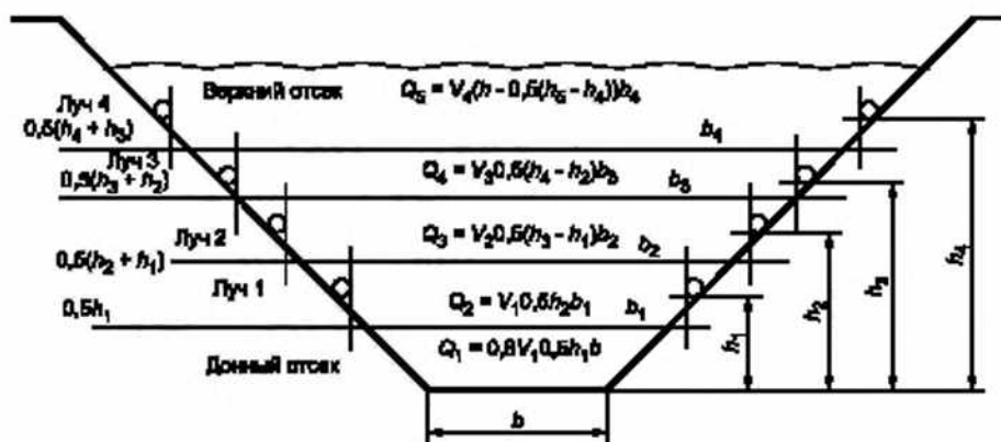
Рисунок 3 — Пример расчета расхода методом послойных сечений
