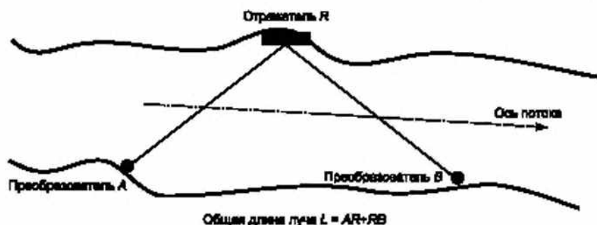
Рисунок 2 — Схема расположения преобразователей с отражением лучей
