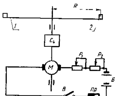
1—крестовина, 2—стойка для крепления анемометров, С4—счетчик частоты вращения крестовины, М—двигатель; P_1 , P_2 —реостаты, В—аккумуляторная батарея; В—выключатель, Пр—предохранитель
