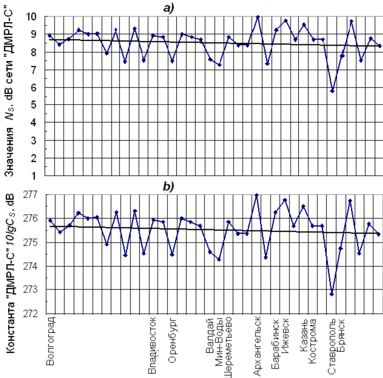
Рис. 12.11 – Значения N_C (a) и констант «ДМРЛ-С» на сети Росгидромета (b) по данным калибровки по солнечному радиоизлучению
