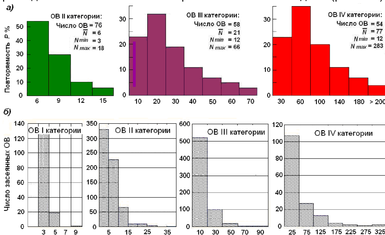
Рис. 10.9 – Расход ПГИ на засев ОБ разных категорий: а) с левосторонним развитием в Аргентине; б) правосторонним развитием на Северном Кавказе
