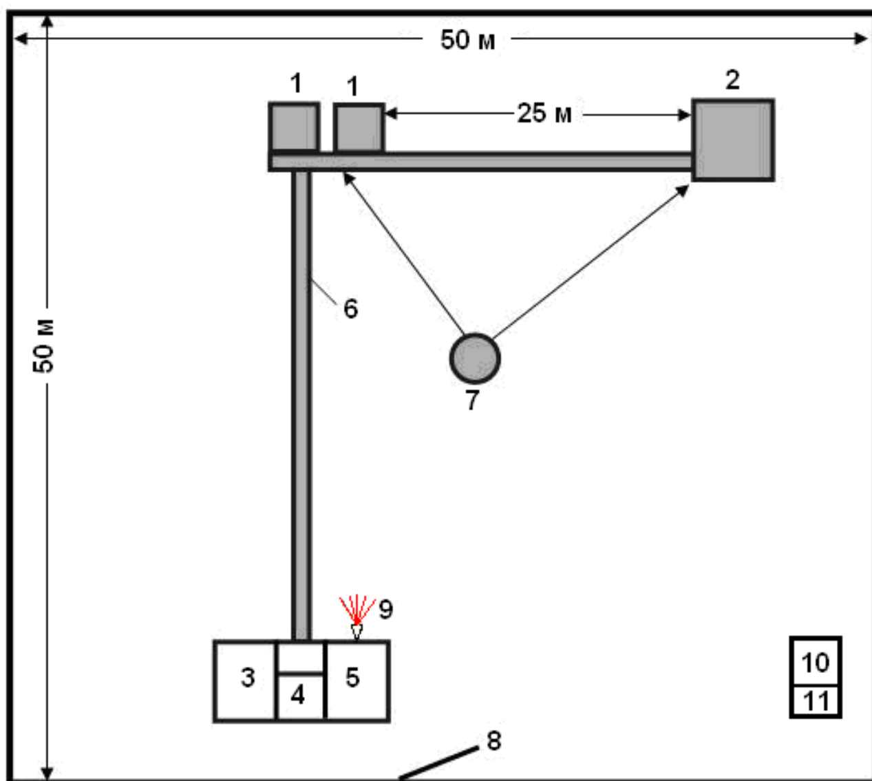
Рис. 15.4 – Примерная схема размещения объектов на ПВ: 1 – бетонированная площадка для ПУ; 2 – склад ПГИ; 3 – жилое помещение; 4 – кухня; 5 – рабочее помещение; 6 – бетонная дорожка; 7 – мачта радиосвязи; 8 – ворота; 9 – прожектор; 10 – душевая; 11 – санузел
