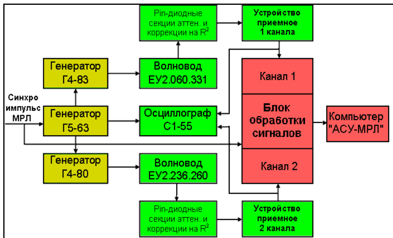
Рис. 12.6 – Блок-схема системы градуировки. измерительного тракта «АСУ-МРЛ»
