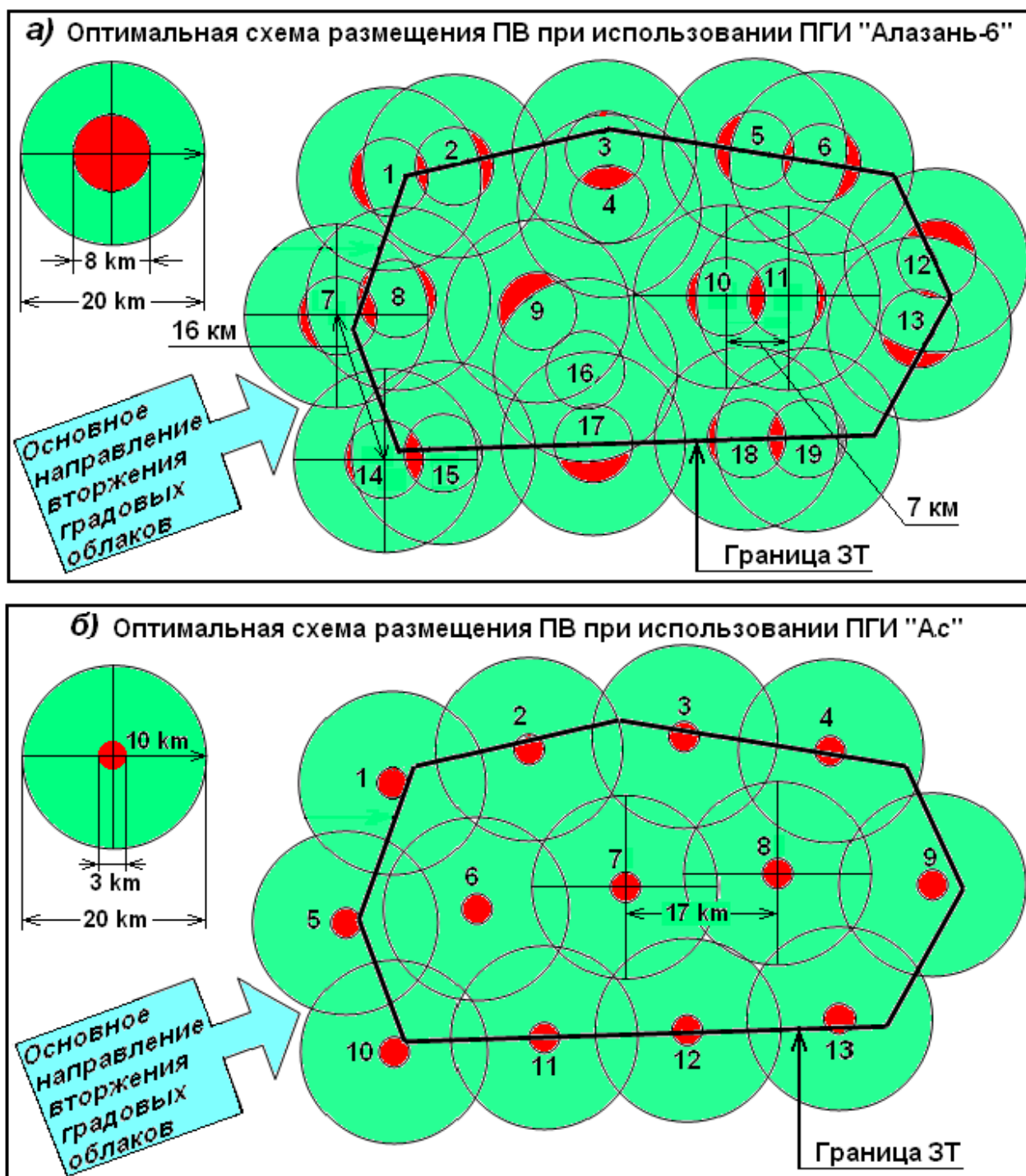
Рис. 15.2 – Оптимальная схема размещения ПВ с ПГИ «Алазань-6» и «Ас». Непростреливаемые участки выделены красным цветом
