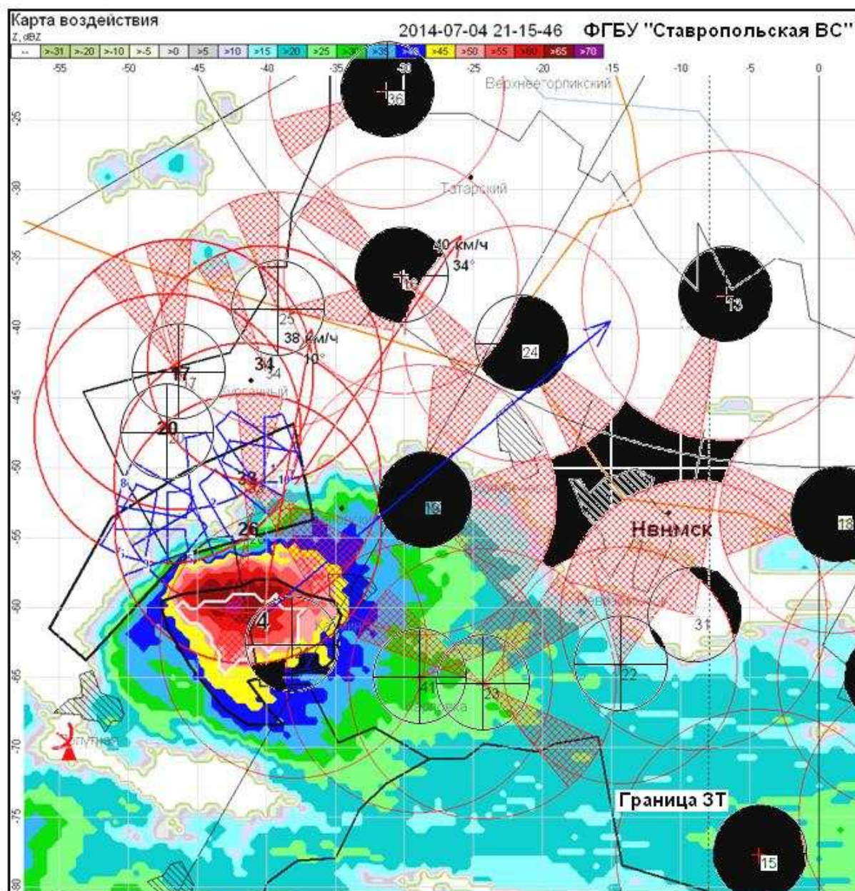
Рис. 15.3 – Фрагмент схемы размещения ПВ с запретными секторами, не простреливаемыми участками (выделены черным) и недостаточной шириной зоны предварительной обработки, приведшей к тому, что при выпадении града на ЗТ наветренный фланг суперячейкового облака остался не засеянным
