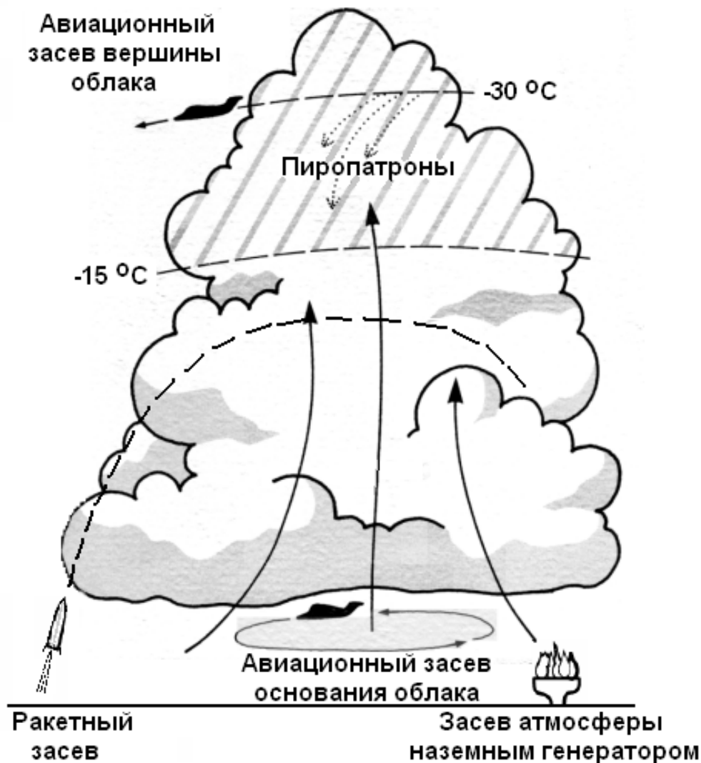
Рис. 11.6 – Ракетный, авиационный и наземный способы засева
