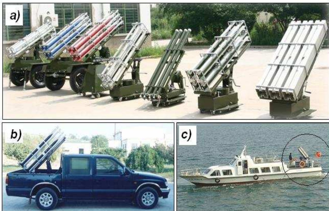
Рис. 13.9 – Ракетные установки китайского производства: а) – передвижные и стационарные; б) – автомобильная; в) – корабельная
