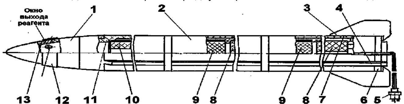
Рис. 13.12 – Устройство ПГИ «Алазань-6»: 1 – ГЧ; 2 – двигатель; 3 – перо стабилизатора; 4 – лента ВВ для дробления корпуса; 5 – вилка с проводами; 6 – блок сопловой; 7 – камера двигателя; 8 – шашка пороховая; 9 – пиротехнический замедлитель; 10 – шашка активного дыма; 11 – корпус ГЧ; 12 – защитная лента; 13 – обтекатель
