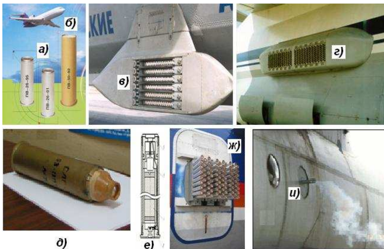
Рис. 13.3 – Российские авиационные средства засева облаков [3, 4]: а) и б) – пиропатроны «ПВ-26» и «ПВ-50»; в) и г) – кассеты для отстрела пиропатронов «АСО-24» и «КДС-155»; д) и е) – самолетные генераторы кристаллизующего аэрозоля «САГ-2» и «САГ-26»; ж) – кассета для «САГ-26»; з) – выход азотного «ГМЧЛ-А»
