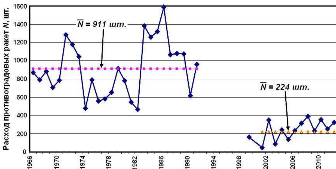
Рис. 17.13 – Расход противоголовых ракет в Молдавской ВС на защиту 100 тысяч га в период с 1966 по 2013 г.
