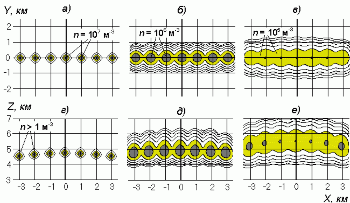
Рис. 14.9 – Горизонтальные (а – в) и вертикальные (г – е) сечения области распространения кристаллизующего аэрозоля в Cu Cong после засева артиллерийскими снарядами "Эльбрус-4" в изолиниях концентрации частиц n ( \text{м}^{-3} ) через 1 (а, г), 3 (б, д) и 5 мин (в, е)
