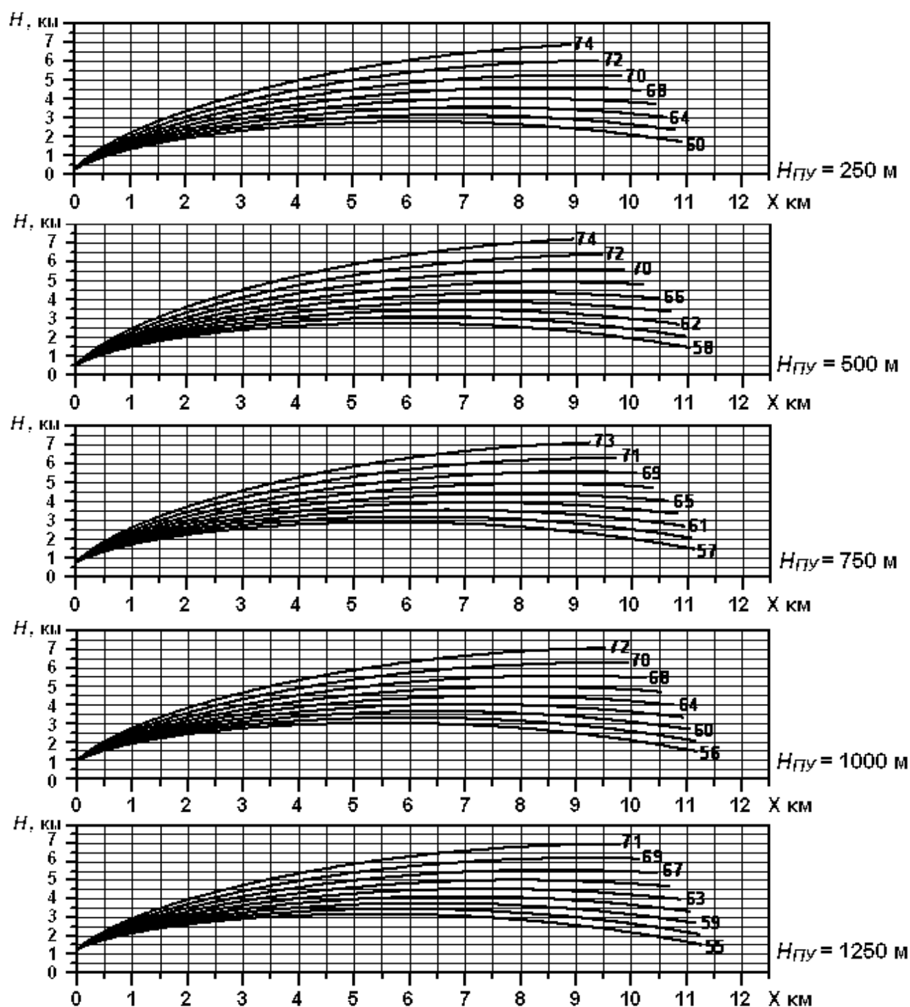
Рис. 13.17 – Траектории ПГИ «Ас» при разных углах пуска с указанной высоты над уровнем моря
