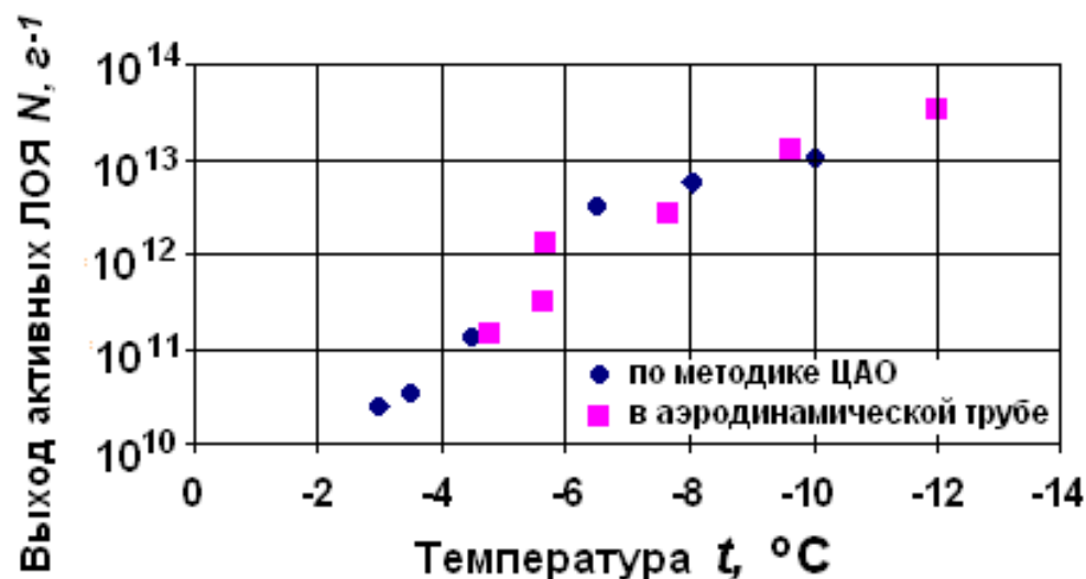
Рис. 14.7 – Выход активных ЛОЯ с 1 грамма состава «АД-1» при испытаниях по методике ЦАО и аэродинамической стенде АН Молдавии [10]
