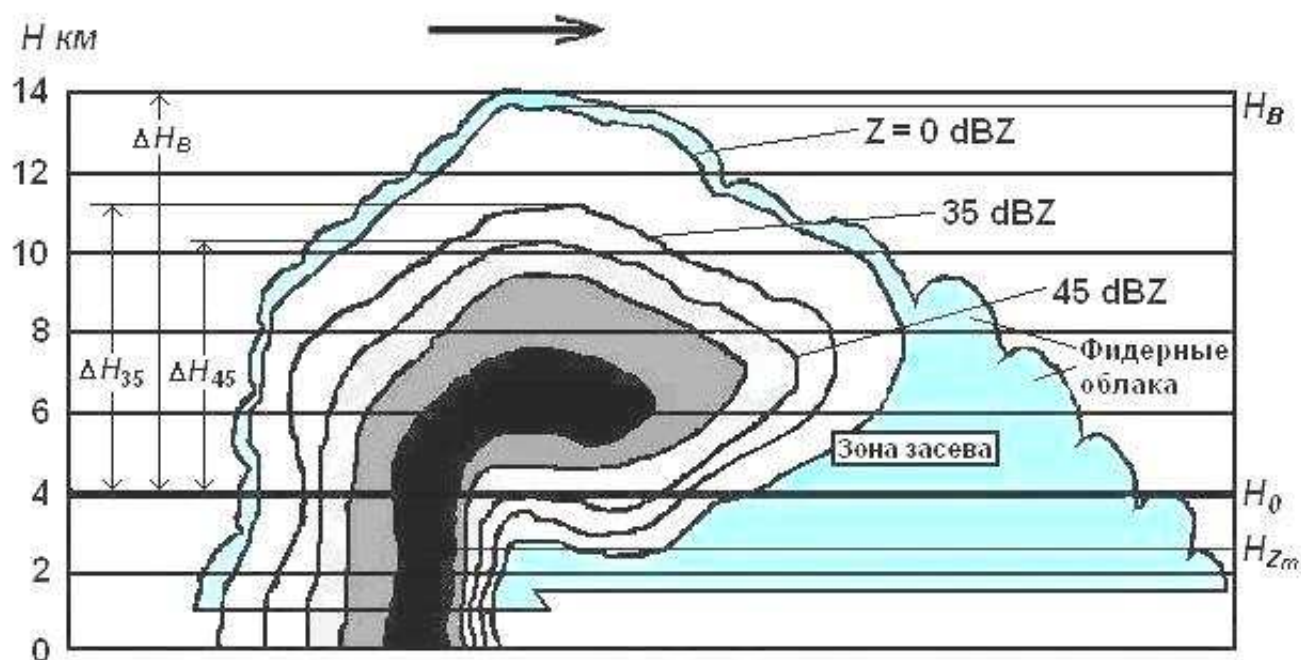
Рис. 12.5 – Схема измерения высот на вертикальном сечении градового облака
