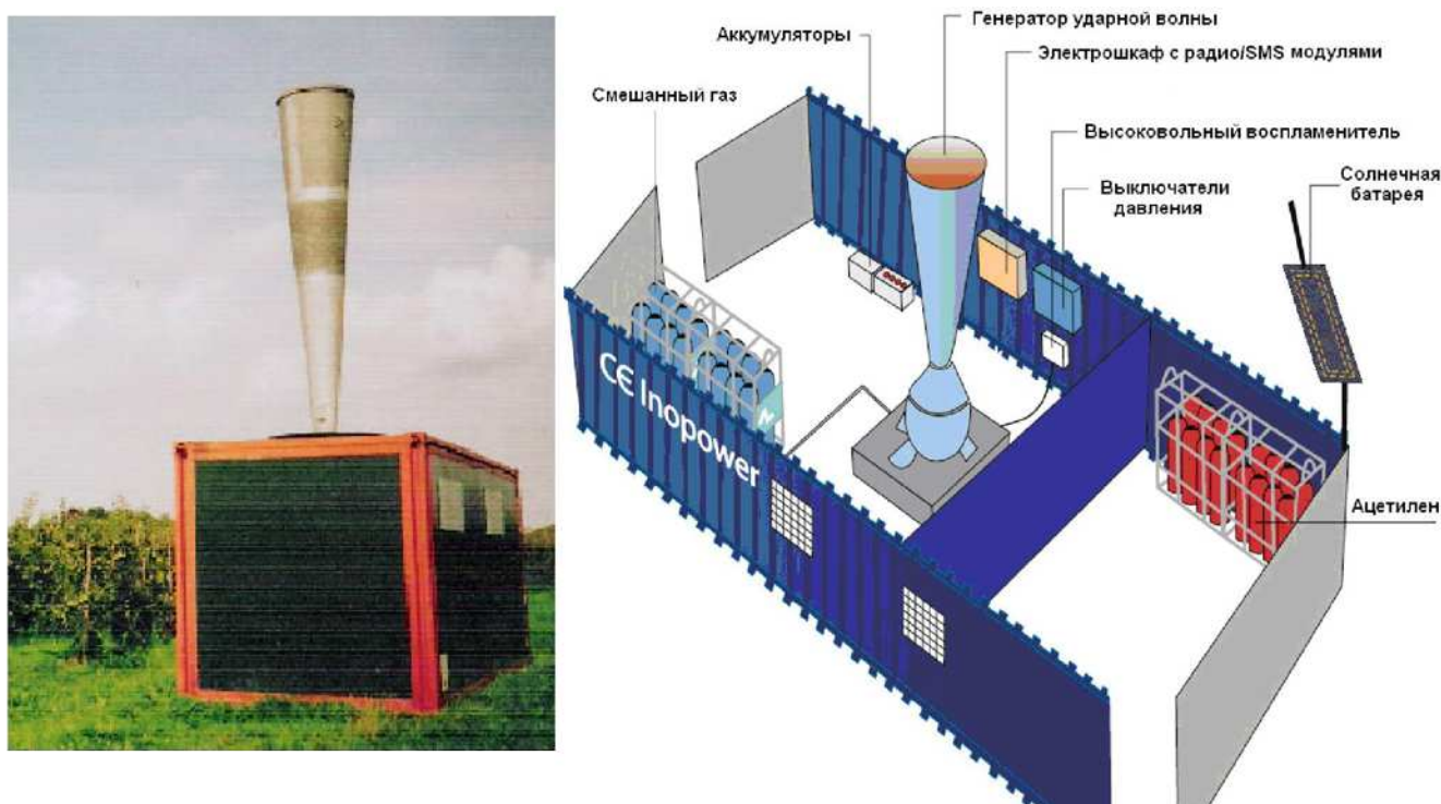
Рис. 11.2 – Ацетиленовые пушки типа «Корвалан», применяемые во Франции, Италии, Нидерландах, Аргентине, Армении и др.
