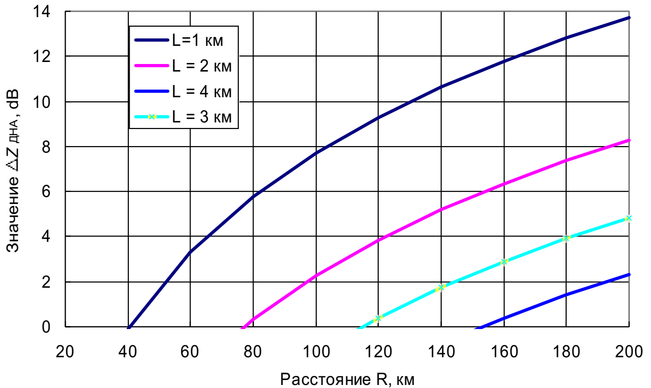
Рис. 12.4 – Зависимость поправки \Delta Z_{\text{ДНА}} от расстояния для 10 см канала МРЛ-5 для градовых облаков при \alpha = 1,5 дБ/км и указанном размере максимума отражаемости L
