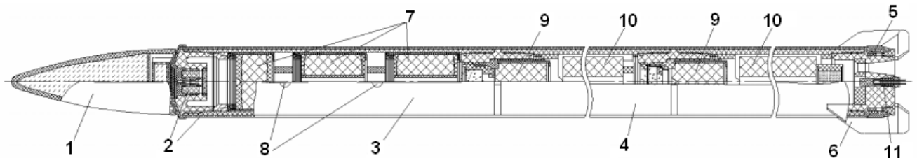
Рис. 13.15 – Малогабаритное ПГИ «Алазань-9» [16]: 1 – обтекатель; 2 – система обеспечения безопасности; 3 – головная часть; 4 – двигатель; 5 – сопловой блок; 6 – перо стабилизатора; 7 – шашка активного дыма; 8 – газовыходные отверстия; 9 – пиротехнический замедлитель; 10 – баллистический порох; 11 – электровоспламенитель
