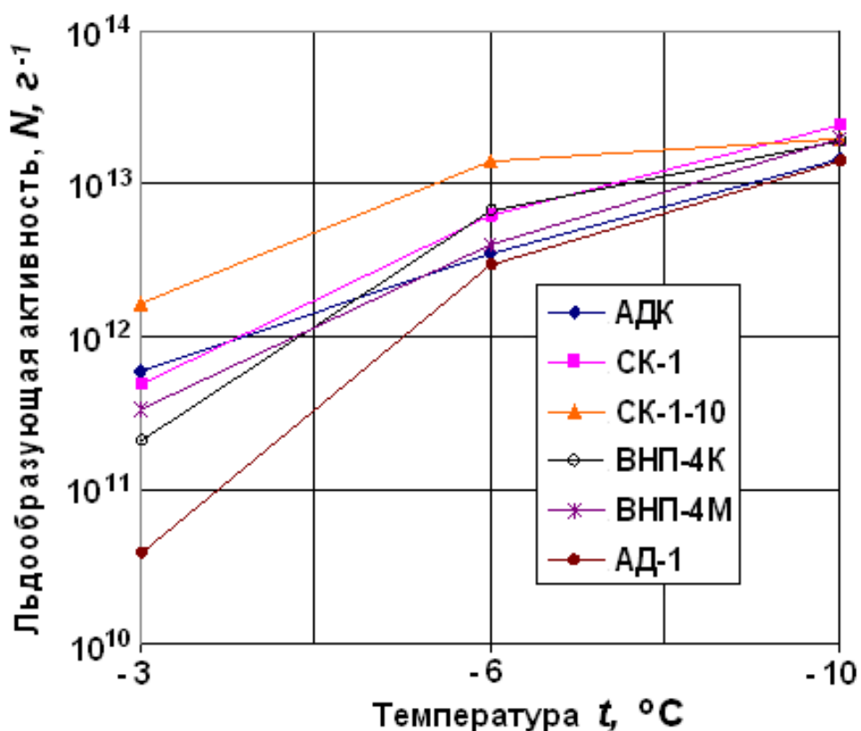
Рис. 14.4 – Результаты испытаний льдообразующей эффективности состава «АД-1» в сравнении с эффективностью новых пиросоставов [8]
