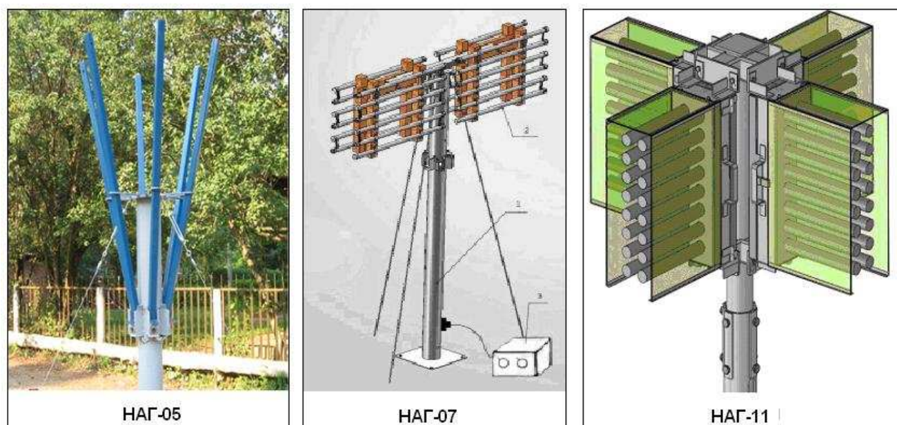
Рис. 13.5 – Наземные аэрозольные генераторы «НАГ-05» и «НАГ-11» [4]
