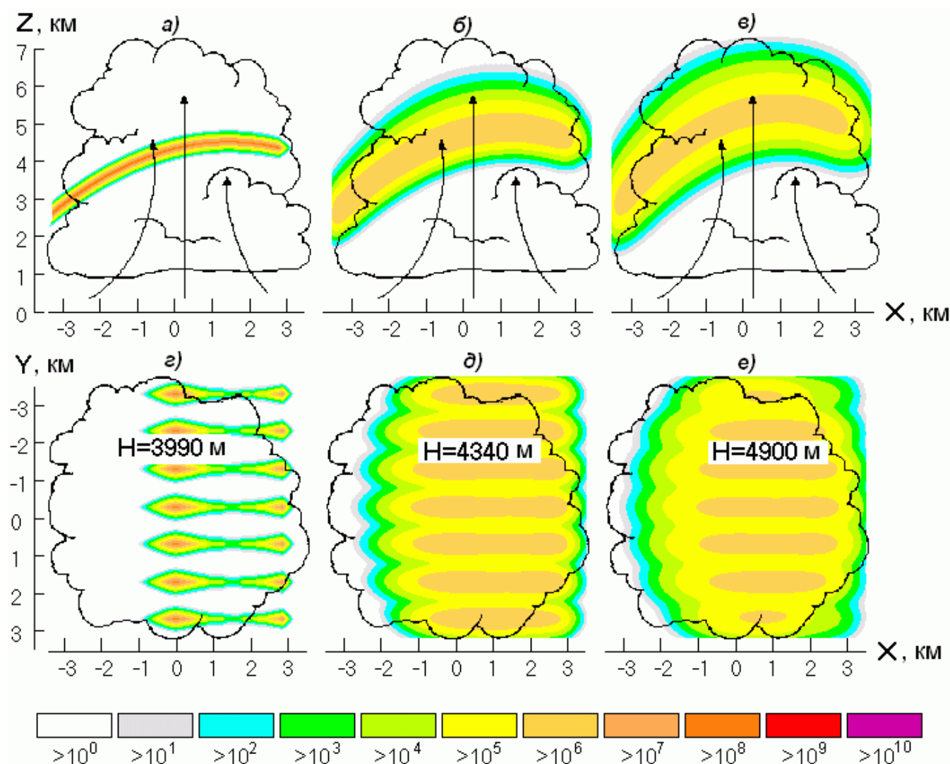
Рис. 14.8 – Вертикальные (а ÷ в) и горизонтальные (г ÷ е) сечения области распространения кристаллизующего аэрозоля в изолиниях концентрации частиц n \text{ (м}^{-3}\text{)} через 1 (а, г), 3 (б, д) и 5 мин (в, е) после засева Cu Cong с помощью ПГИ «Алазань-6»
