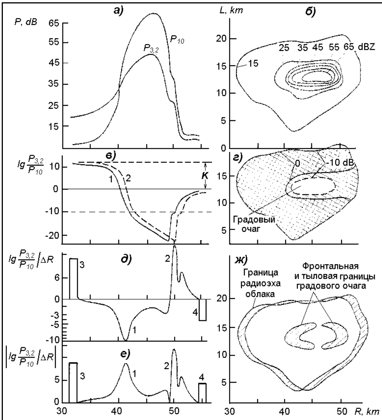
Рис. 7.23 – Форма радиоэха градового облака на индикаторах типа «А» и ИКО при различных способах отображения [27]: а) радиальное распределение мощности радиоэха на \lambda = 3,2 и 10 см; б) карта изолиний Z_{10} , dBZ; в) радиальное распределение \lg P_{3.2}(R)/P_{10}(R) без задержки (1) и с задержкой на \Delta R (2); K – полное ослабление 3.2 см. излучения на двойном пути; г) градовый очаг, выделяемый по порогам 10 \lg P_{3.2}(R)/P_{10}(R) = 0 и 10 dB; д) и е) радиальное распределение дифференциала разностного сигнала, выделяющего границы градового очага (1 и 2) и границы радиоэха (3 и 4); ж) границы градового очага на ИКО
