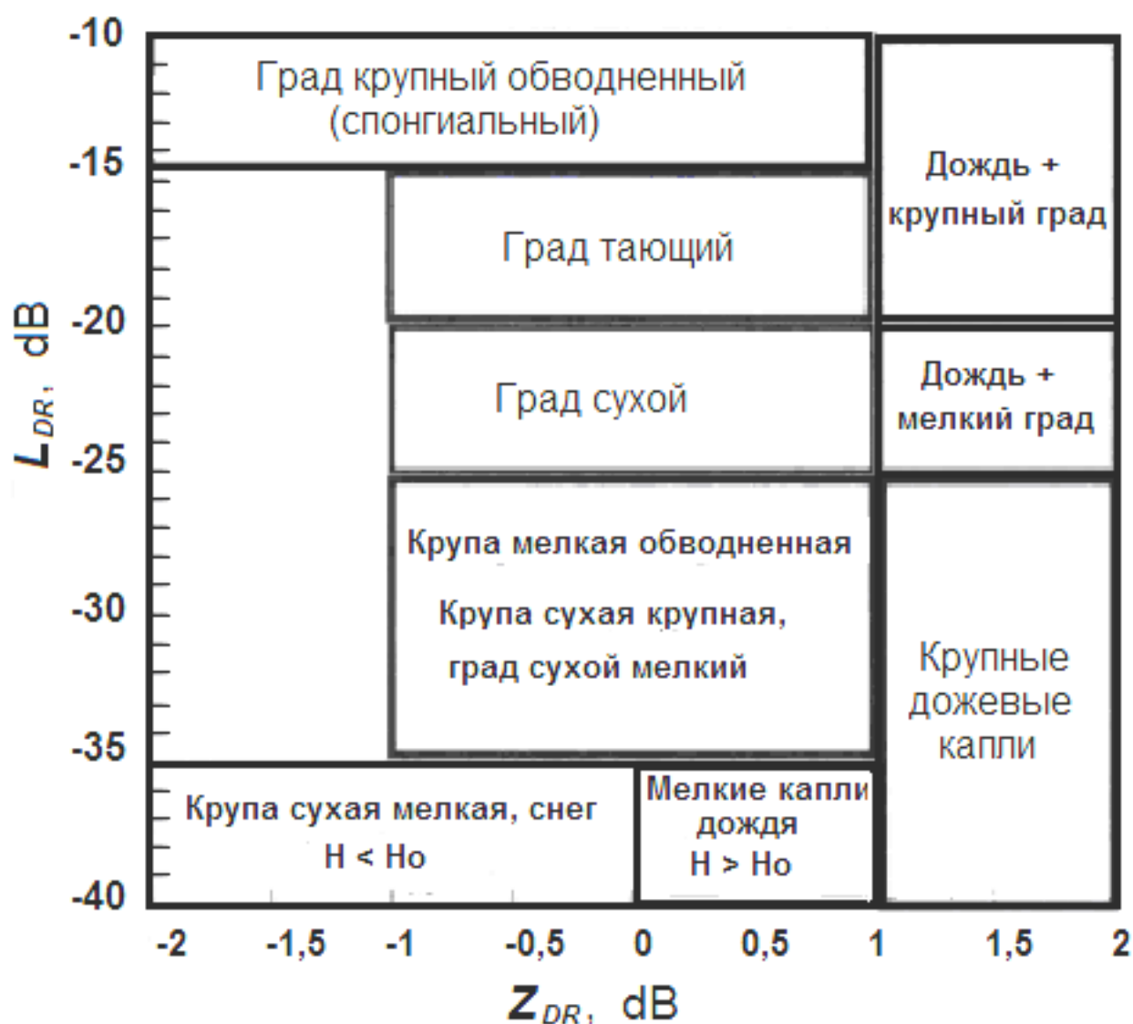
Рис. 7.24 – График распознавания вида облачных частиц по Z_{DR} и L_{DR} [29]
