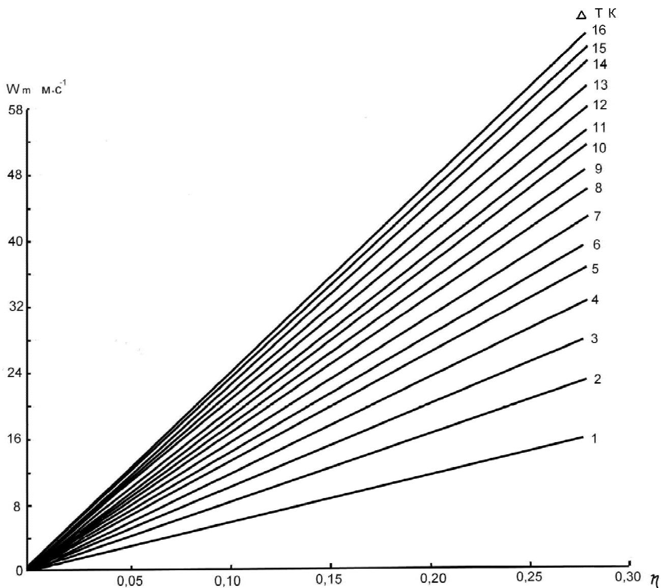
Рис. 6.6 – Зависимость W_m от \eta = \frac{T_{\text{конд}} - T_m}{T_{\text{конд}}} при разных значениях \Delta T
