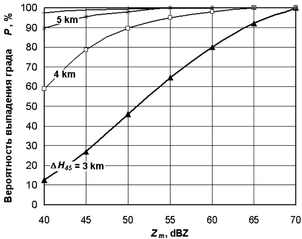
Рис. 7.13 – Вероятность выпадения града P_H в зависимости от Z_m при указанных значениях \Delta H_{45} [38]
