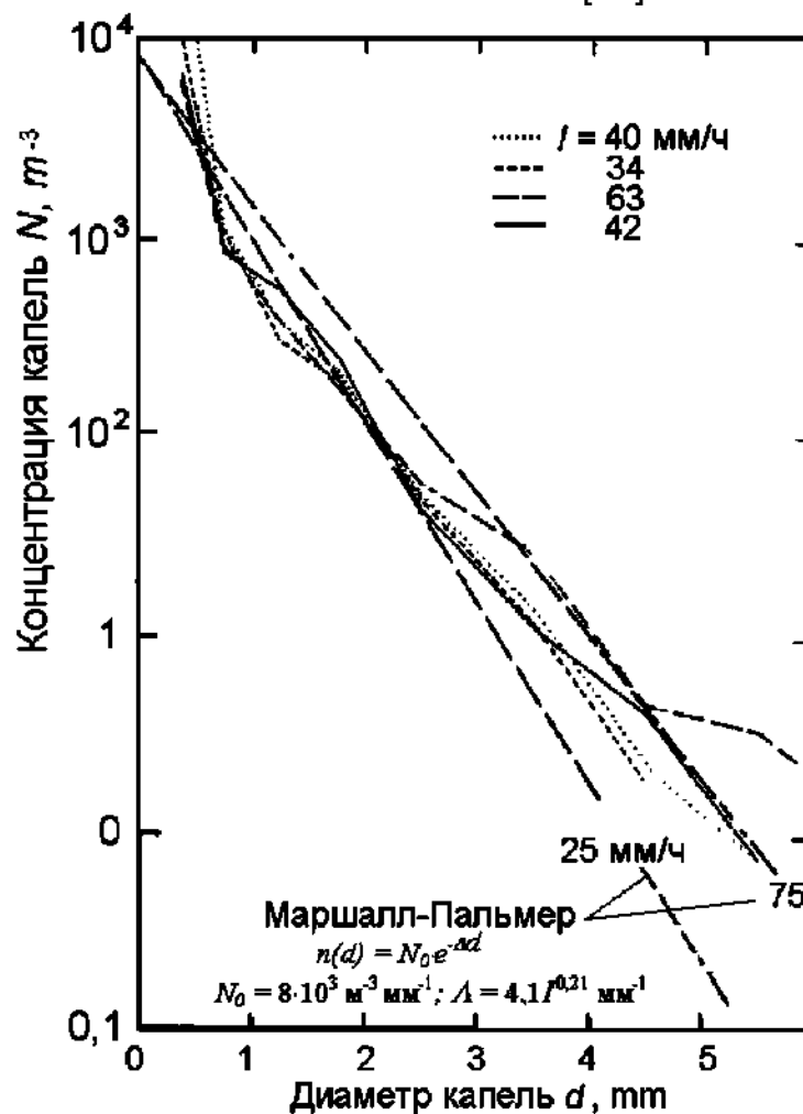
Рис. 7.6 – Спектр капель в ливневых дождях [20]
