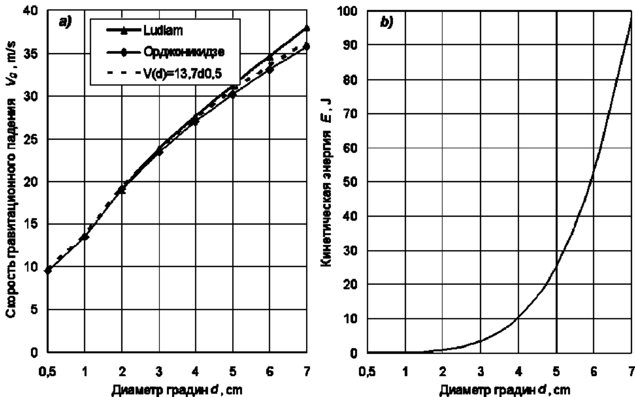
Рис. 5.12 – Зависимость от размера градин скорости их гравитационного падения (а) и кинетической энергии при безветренной ситуации (б)
