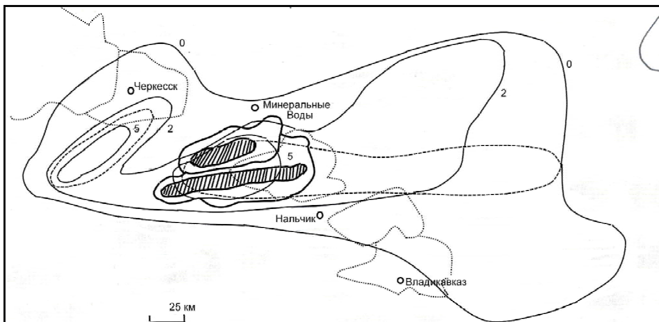
Рис. 6.12 – Определение мезорайона развития градового процесса: показаны области градиентов \Delta t_{cm}/\Delta x = 0,2 и 5 °C/100 км, штриховкой выделены полосы выпадения града [2]
