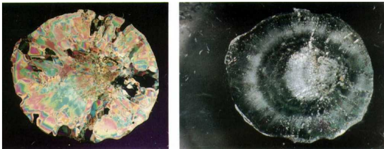
Рис. 5.11 – Структура градин в поляризованном и проходящем свете
