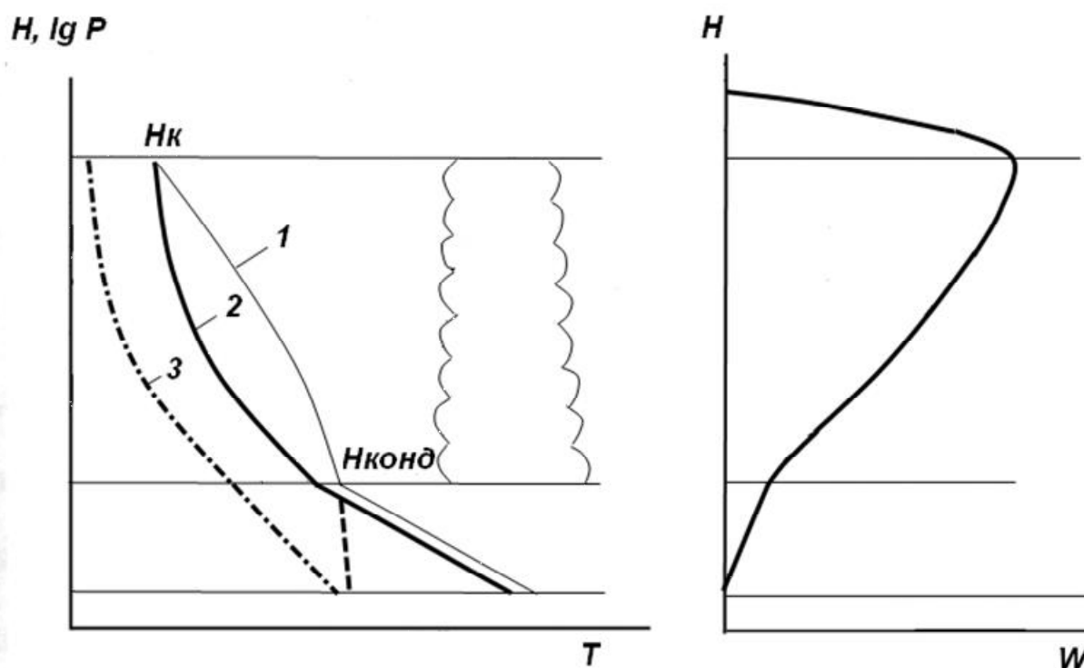
Рис. 6.2 – Определение параметров конвекции «методом частицы»: 1 – кривая состояния; 2 – кривая стратификации; 3 – кривая влажности
