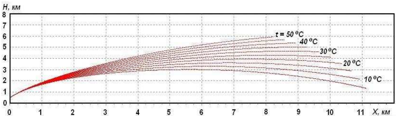
Рис. 13.17 – Траектории ПГИ «Ас» при температуре заряда от 5 до 50 °С
