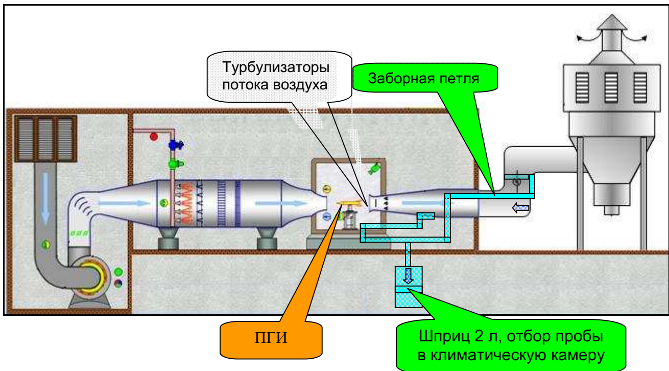
Рис. 14.5 – Схема испытаний льдообразующей эффективности ПГИ в аэродинамической трубе «НПО «Тайфун» при скоростях обдува 90 \pm 10 м/с [9]
