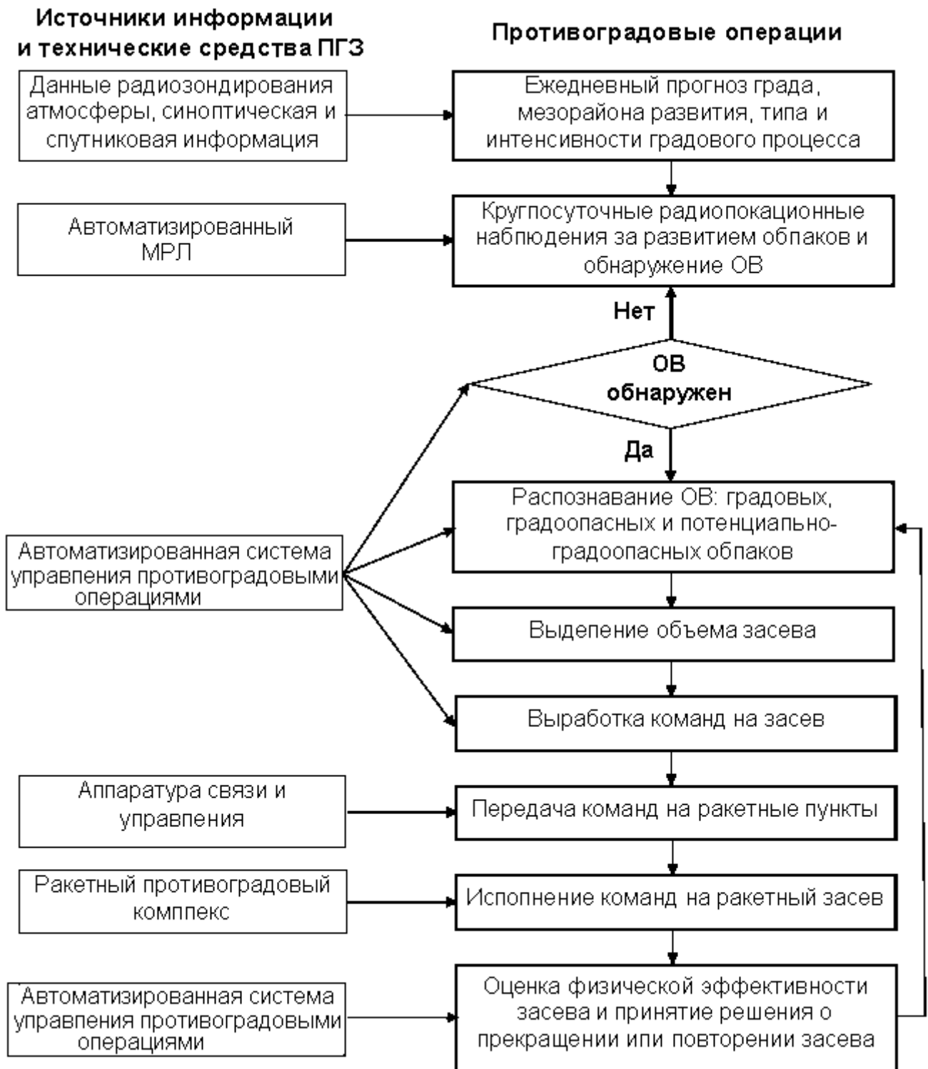
Рис. 11.7 – Блок-схема технологического процесса ПГЗ [62]
