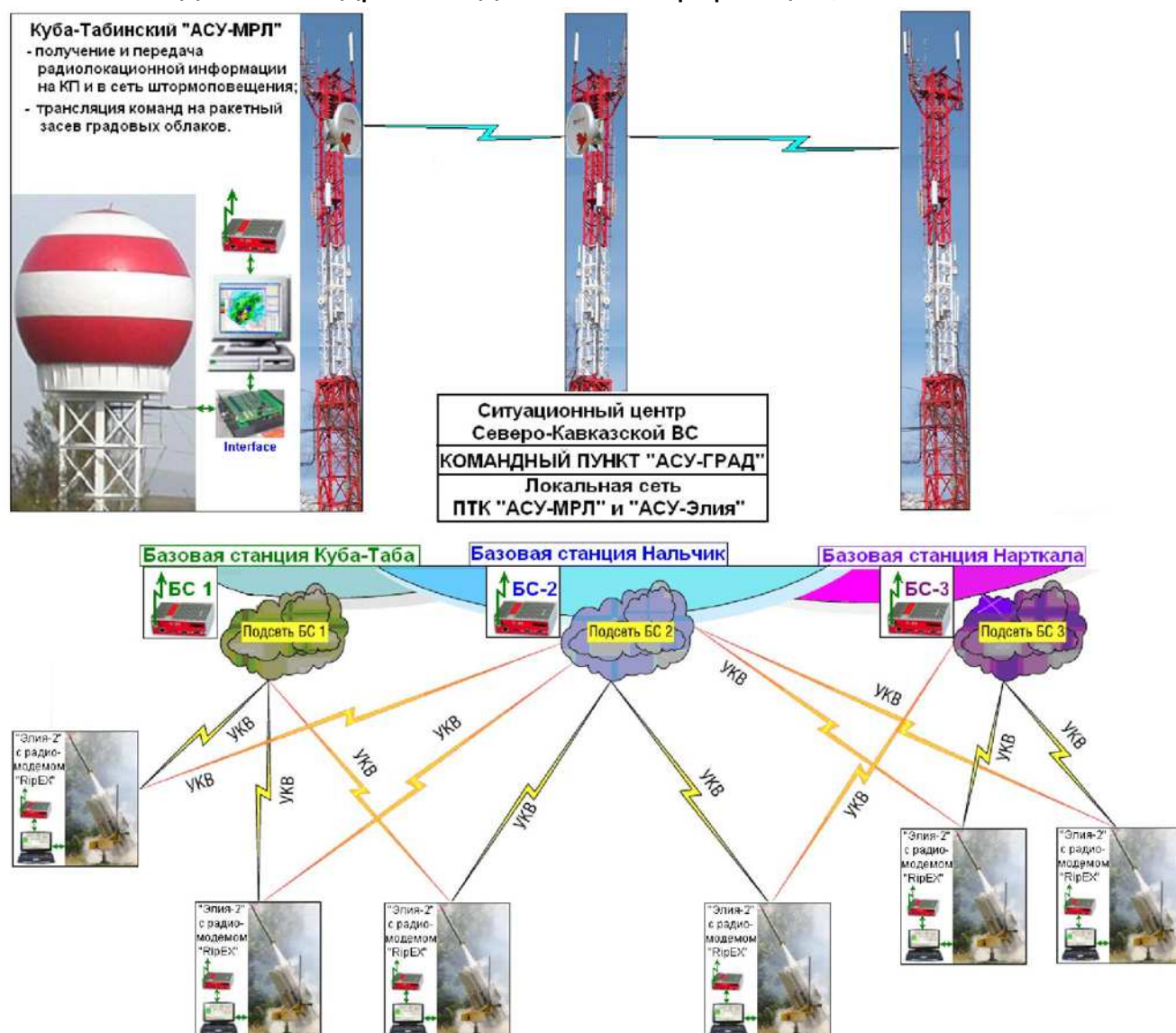
Рис. 13.20 – Блок-схема системы связи опытного образца «АСУ-Град»
