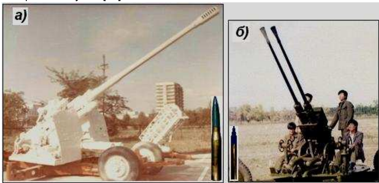
Рис. 13.7 – Артиллерийские комплексы калибра 100 и 37 мм: а) – российский комплекс «Эльбрус-4»; б) – комплекс китайского производства
