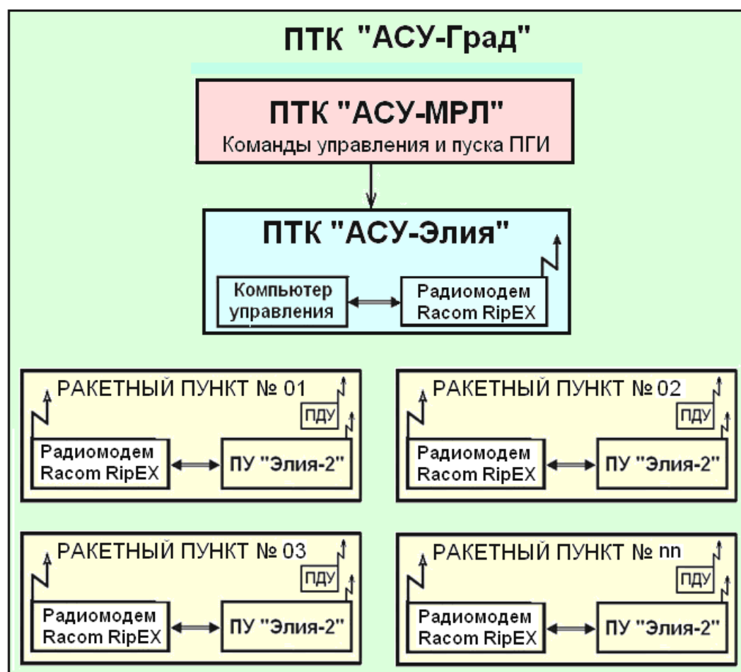
Рис. 13.18 – Блок-схема автоматизированной системы ПГЗ «АСУ-Град»
