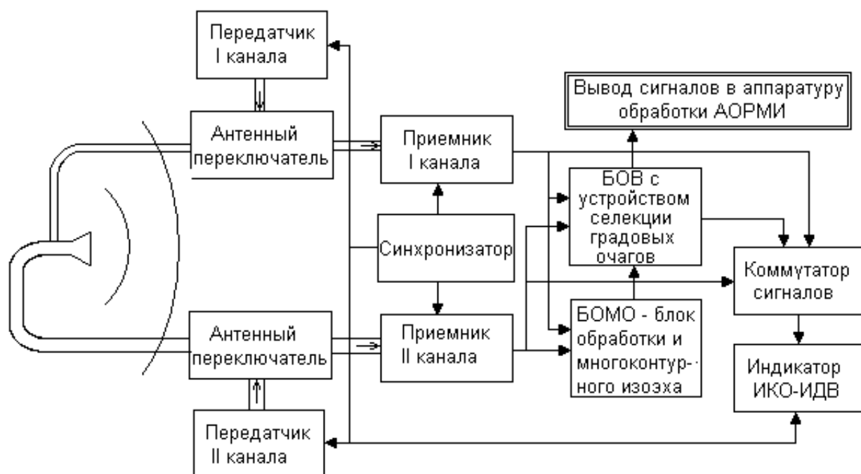
Рис. 12.1 – Блок-схема радиолокатора «МРЛ-5»
