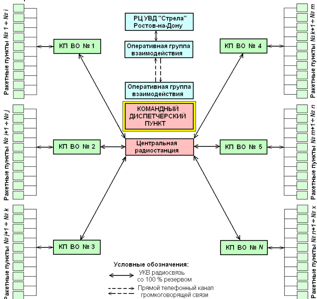
Рис. 15.5 – Примерная структура связи ВС Росгидромета
