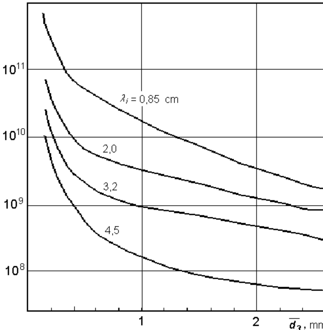
Рис. 7.9 – Связь k_{\lambda_i} / \eta_{\lambda_j} с \bar{d}_3 спектра капель на указанных \lambda_i и \lambda_j = 10 см [25]
