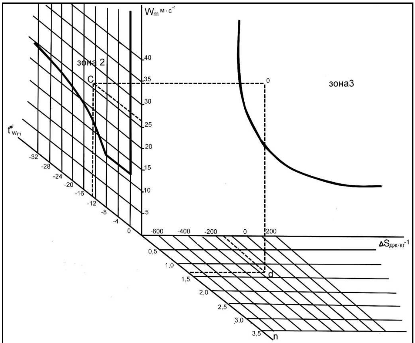
Рис. 6.10 – Зависимость интенсивности градовых процессов от термодинамических и циркуляционных характеристик атмосферы [2]: W_m – максимальная скорость восходящих потоков в облаке; t_{W_m} – температура на уровне максимальной скорости восходящих потоков в облаке; \Delta S – характеристика энергетического состояния подоблачного слоя; n – параметр, характеризующий (в долях от 10) вероятность градовых процессов в зависимости от циркуляционных характеристик атмосферы; зона 3 – область интенсивных градобитий
