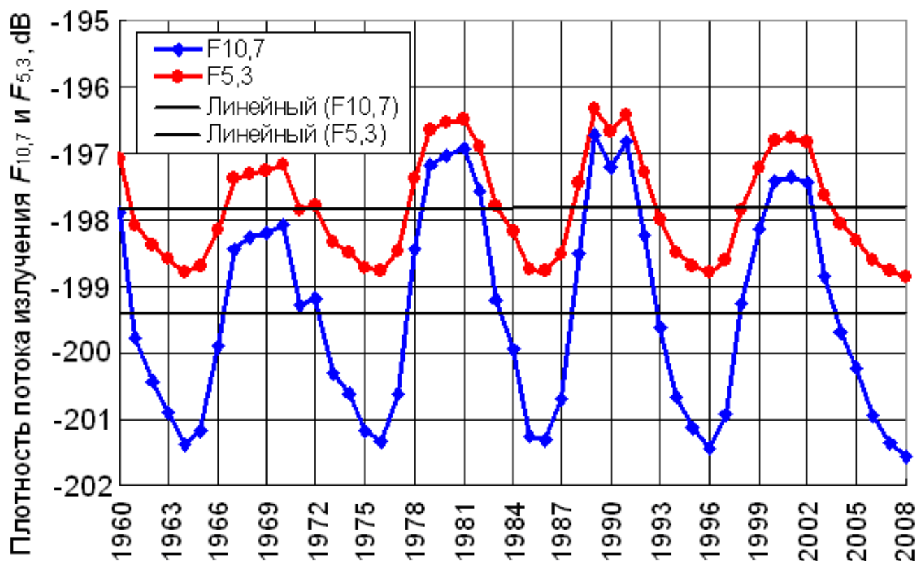
Рис. 12.9 – Временной ход значения F_{10,7} и F_{5,3} в dB в период с 1960 по 2008 г.
