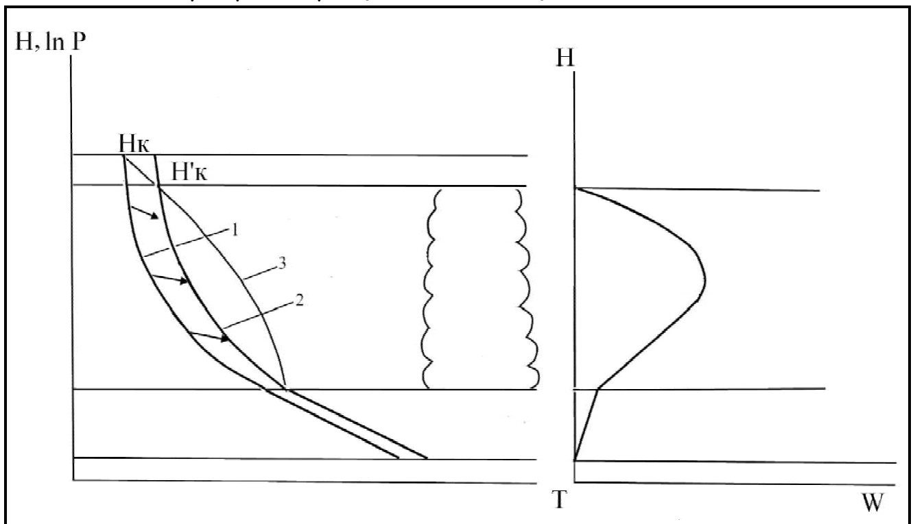
Рис. 6.3 – Определение параметров конвекции «методом слоя»: 1 – начальная кривая стратификации; 2 – кривая стратификации после развития конвекции; 3 – кривая состояния
