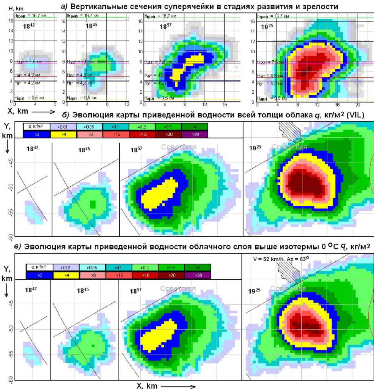
Рис. 8.12 – Эволюция структуры радиоэха суперячейки от начала развития до стадии зрелости: а) вертикальные сечения в изолиниях Z : в период зарождения в 18^{42} , в стадии развития в 18^{45} и 18^{57} и в стадии зрелости в 19^{25} ; б) и в) карты приведенной водности всей толщи и переохлажденного слоя облака
