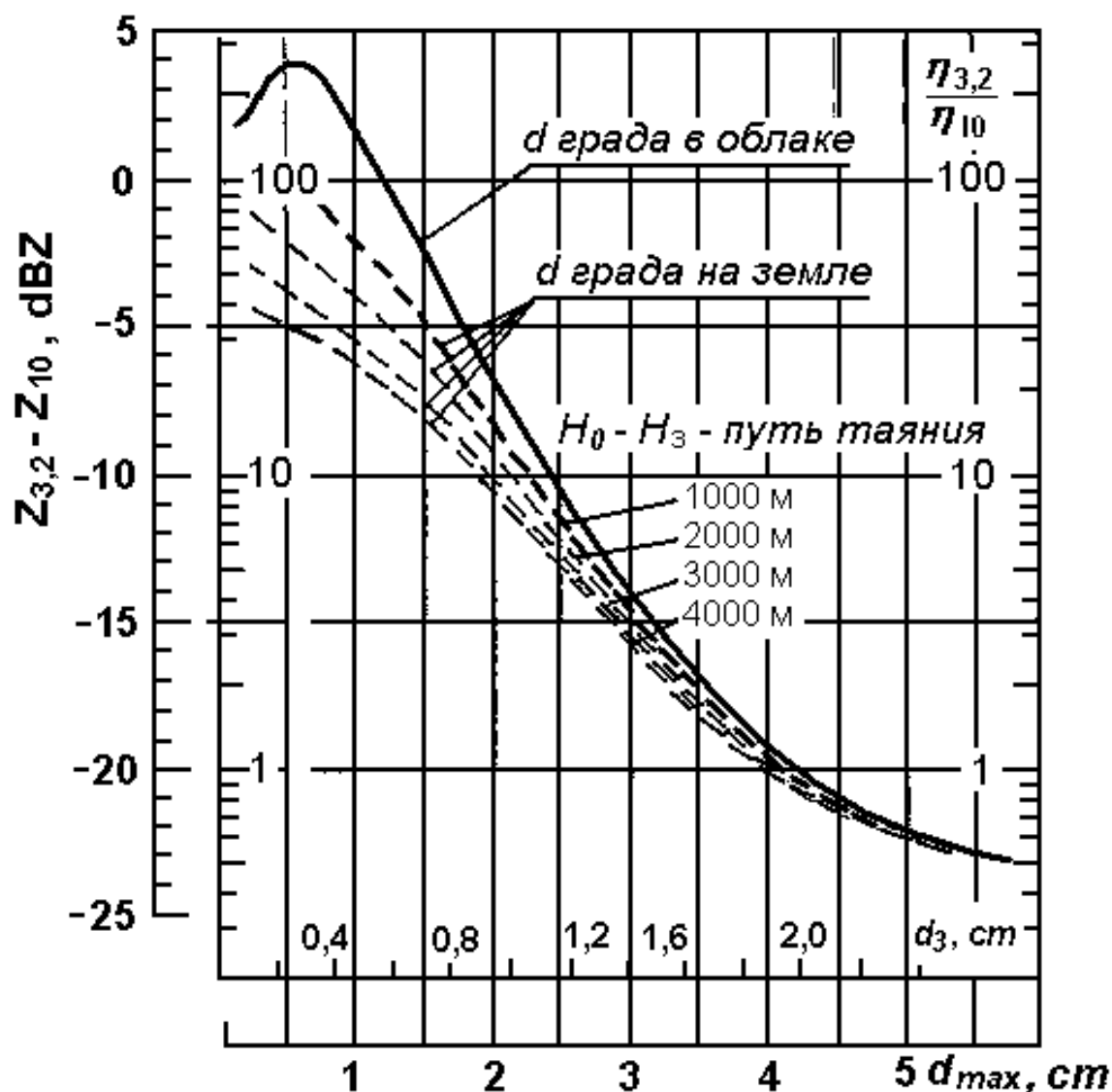
Рис. 7.22 – График определения размера града двухволновым методом: сплошная кривая – в облаках; пунктирные – в осадках с учетом таяния на пути от H_0 до
