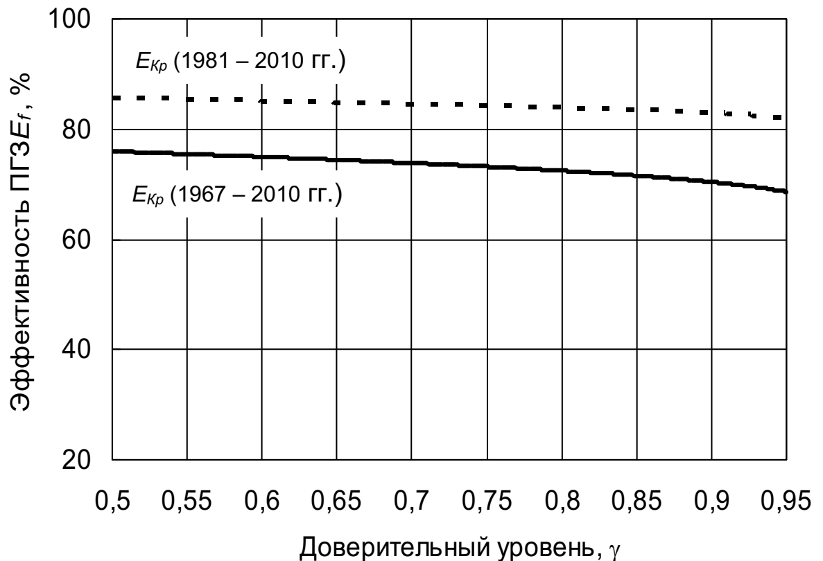
Рис. 17.18 – Верхняя граница доверительного интервала эффекта ПГЗ в СНГ в E_f в период 1967 – 2010 гг. (сплошная) и в период 1981 – 2010 гг. (пунктир)
