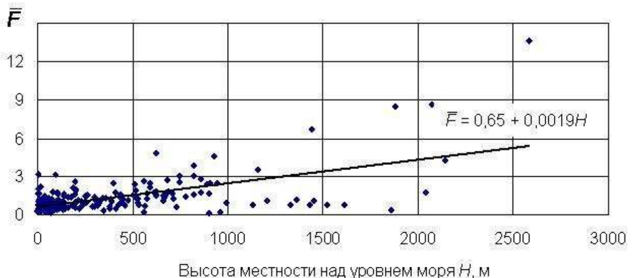
Рис. 5.2 - Зависимость частоты выпадения града от высоты [7]
