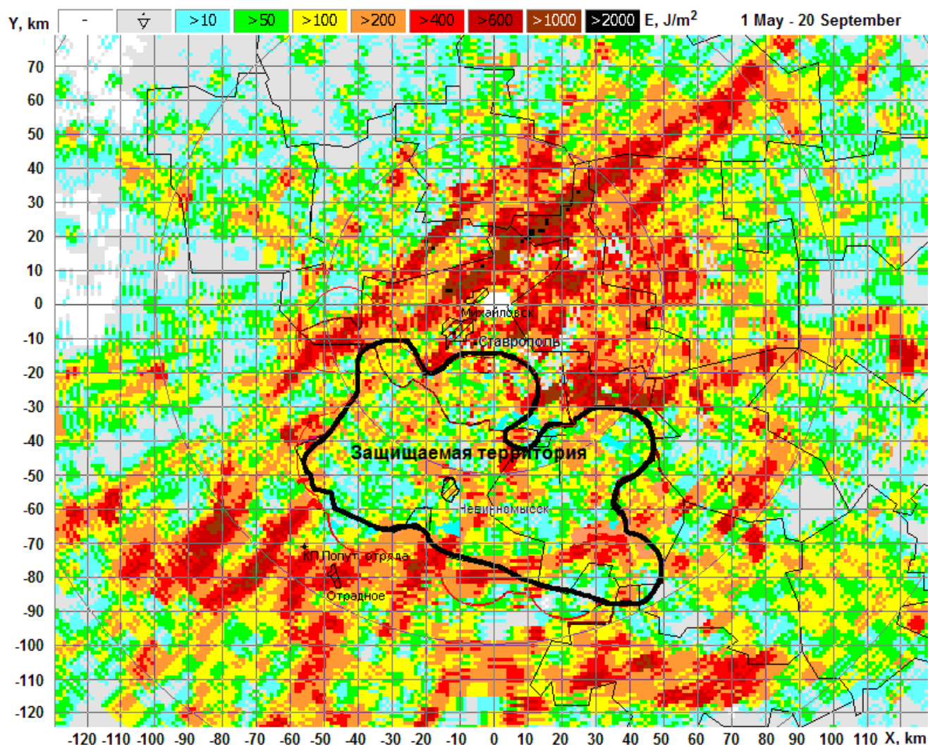
Рис. 17.10 – Карта суммарной кинетической энергии града в Ставропольском крае, просуммированной за период с 1 мая по 20 сентября 2004 г.
