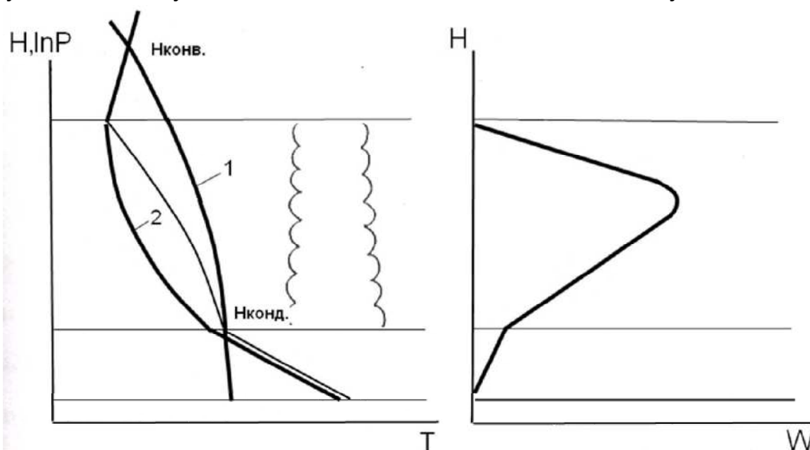
Рис. 6.4 – Определение параметров конвекции для внутримассовых процессов
