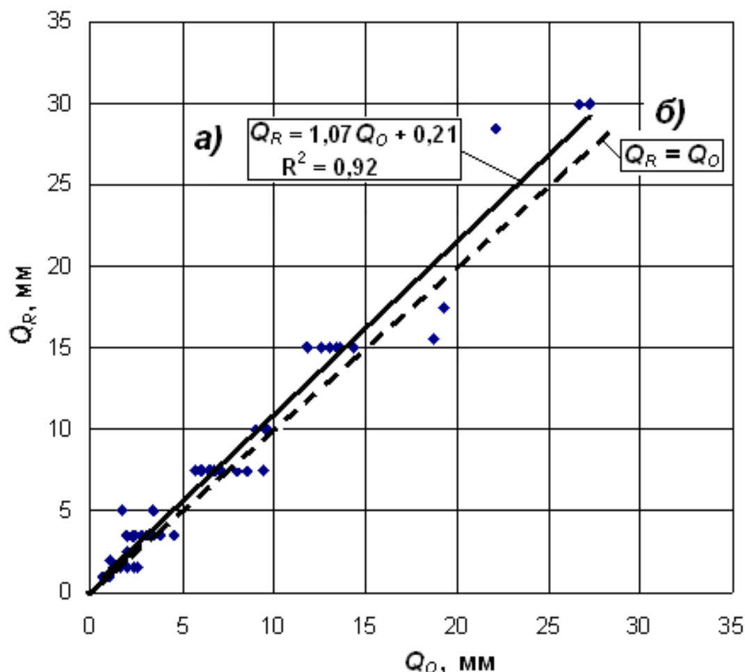
Рис. 12.8 – Количество осадков по данным «АСУ-МРЛ» Q_R и pluviографа Q_O : а) сплошная линия – линия тренда экспериментальных данных; б) линия согласования данных «АСУ-МРЛ» и pluвиографов
