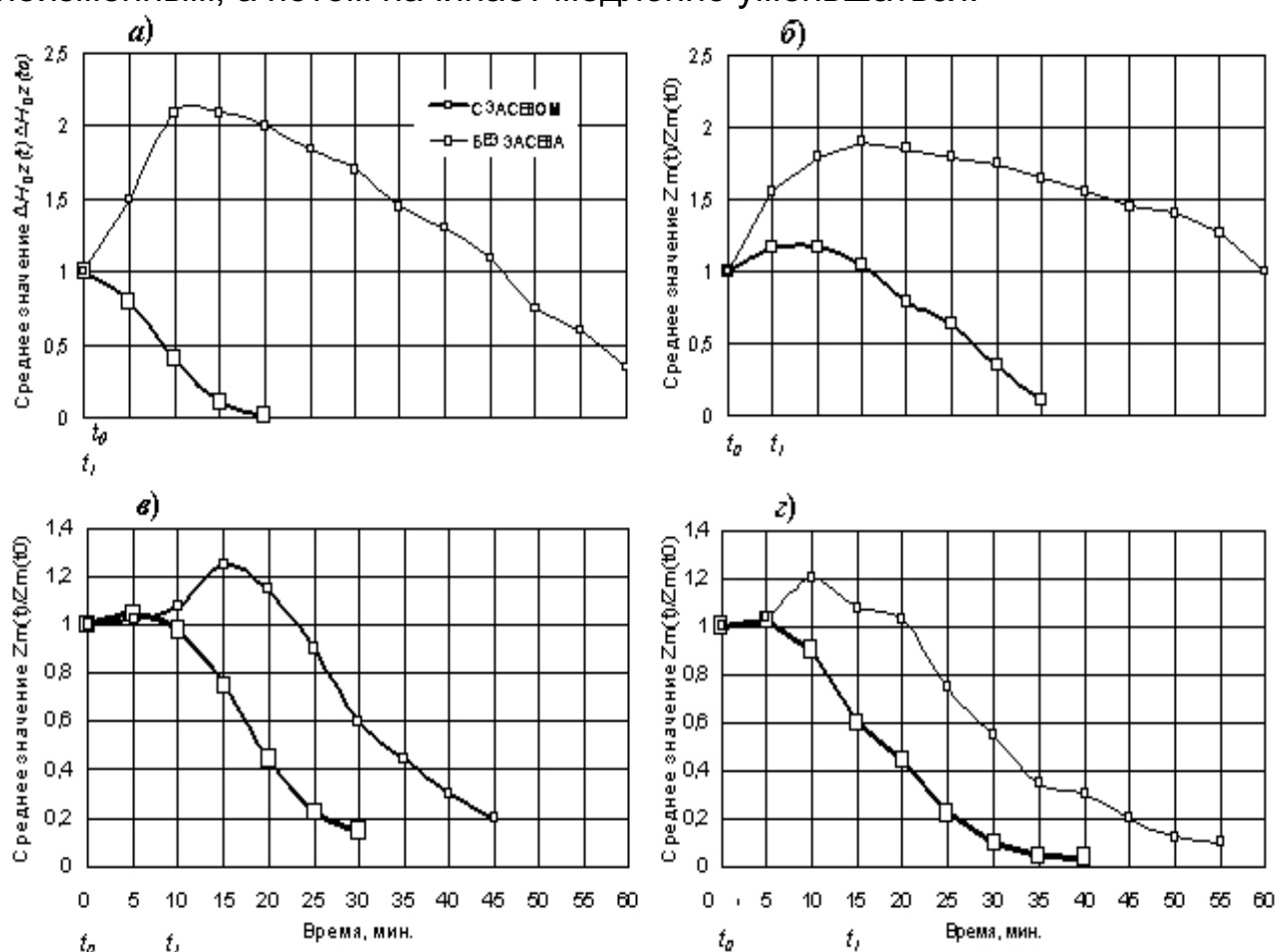
Рис. 17.3 – Эволюция во времени средних значений одномерных параметров засеянных и незасеянных ОБ I (а), II (б), III (в) и IV (г) категорий: t_0 – время начала реального и условного засева ОБ; t_1 – время окончания реального и условного засева
