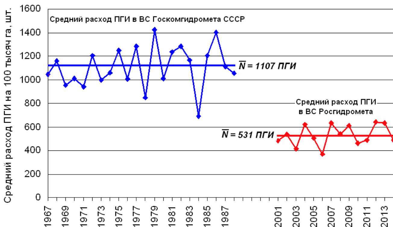
Рис. 17.12 – Средний расход ПГИ на защиту 100 тысяч га в ВС Госкомгидромета СССР и ВС Росгидромета
