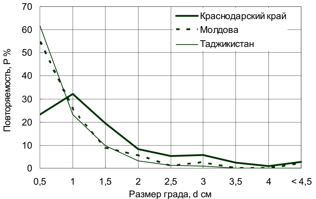
Рис. 5.10 – Повторяемость размера града в указанных регионах [7]
