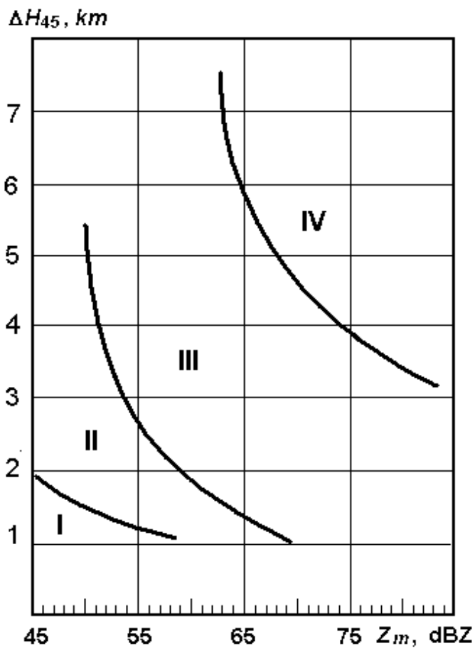
Рис. 7.14 – График разделения области ливневых (I), градоопасных (II), градовых (III) и мощных градовых (IV) облаков по значениям Z_m и \Delta H_{45} [38]
