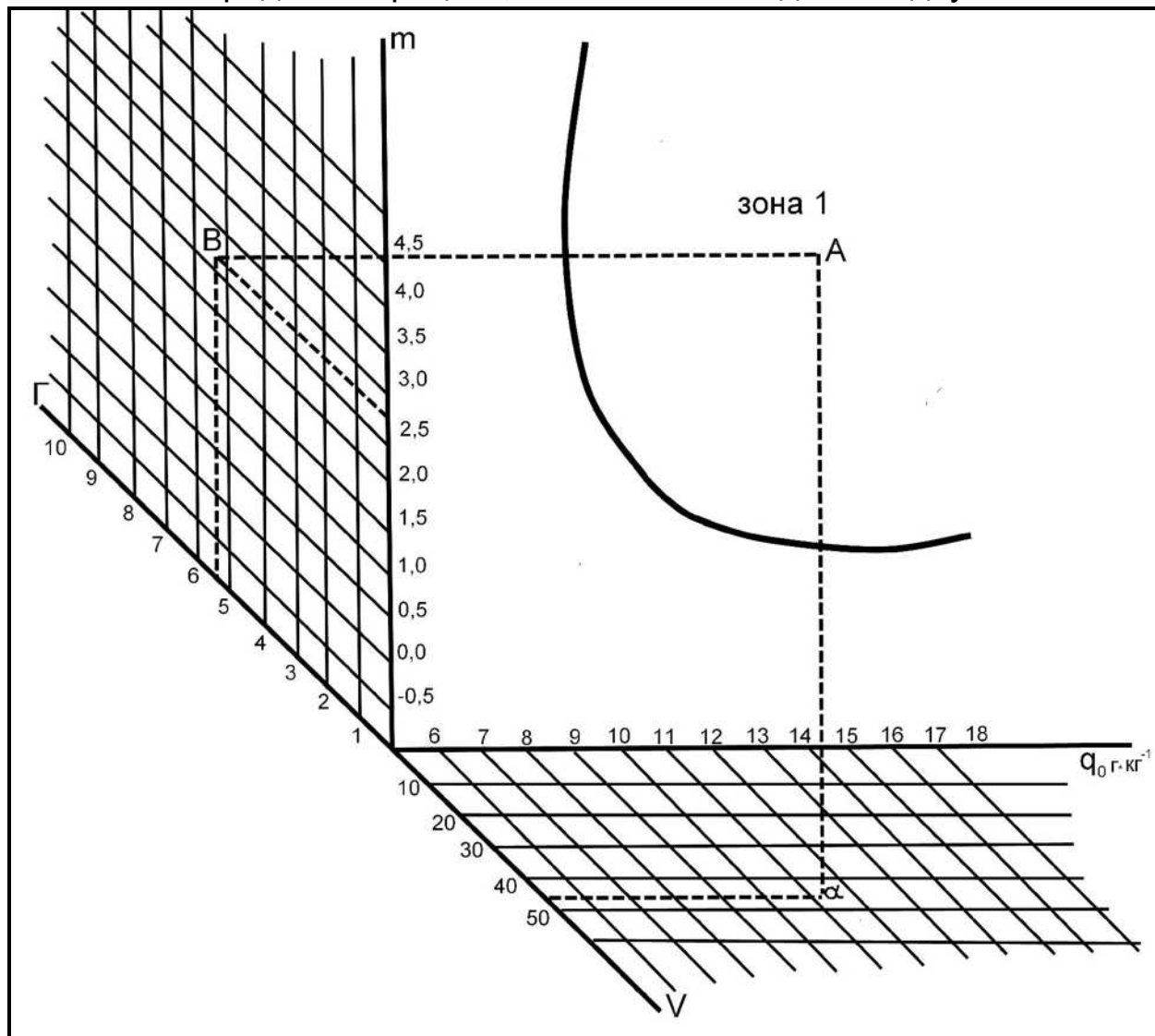
Рис. 6.9 – Зависимость интенсивности градовых процессов от термодинамических и синоптических параметров атмосферы [2]: q_0 – массовая доля влаги у земли; V – скорость перемещения фронтальной поверхности; \Gamma – градиент струйного течения; m – параметр, характеризующий вероятность ГП в зависимости от сдвига ветра в слое конвекции и направления переноса в средней тропосфере; зона 1 – область интенсивных градобитий
