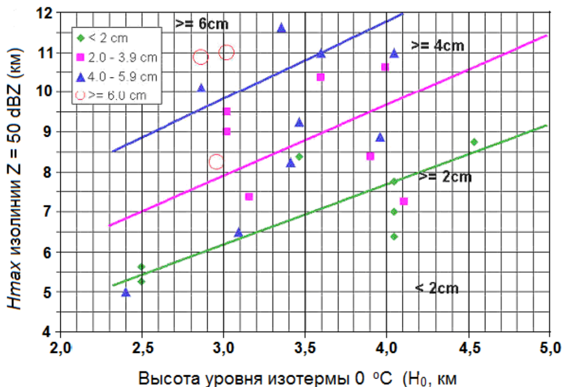
Рис. 7.28 – «Градовая номограмма» применительно к климатологии града в области Сиднея [48]
