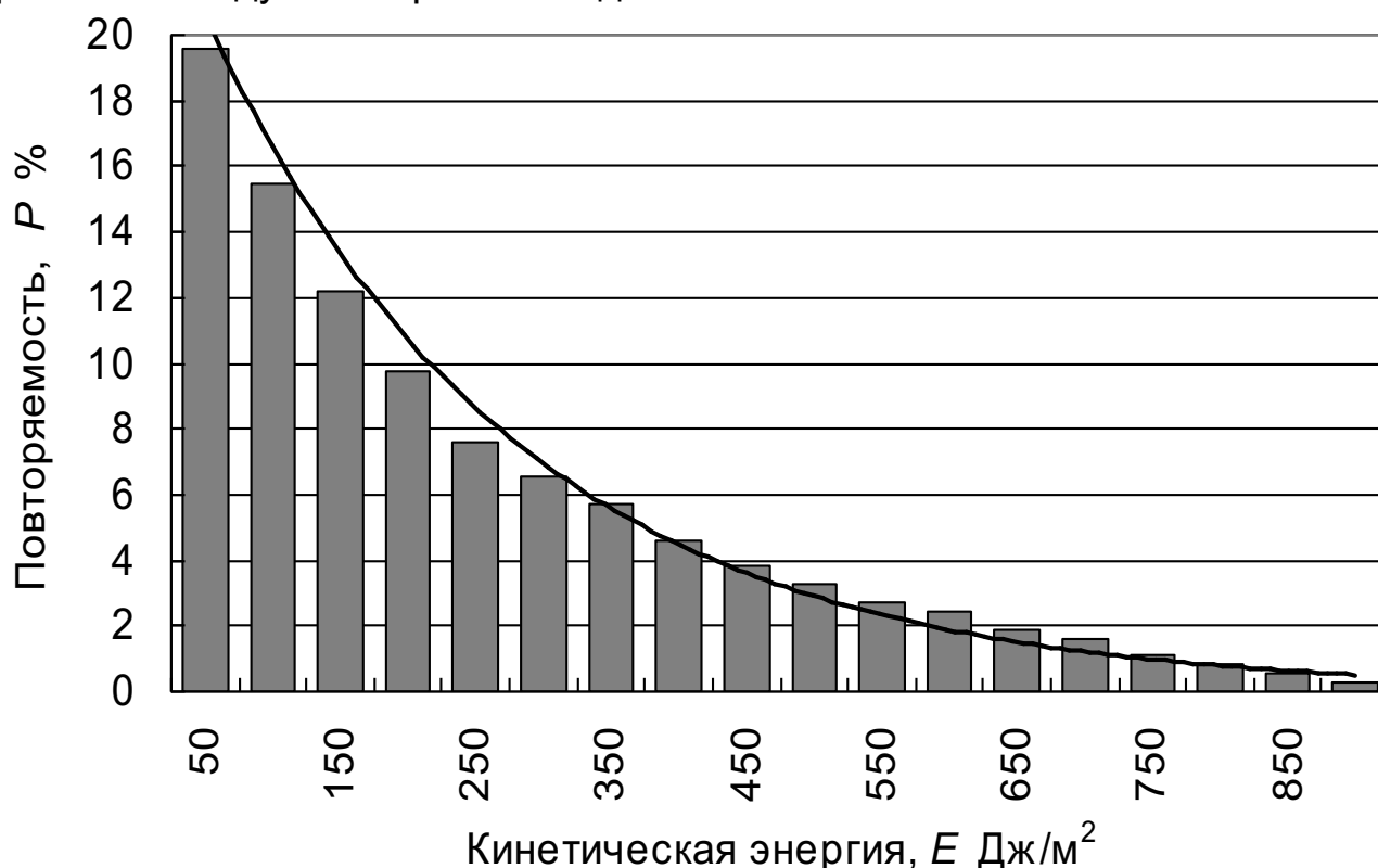
Рис. 5.13 – Повторяемость кинетической энергии града [7]
