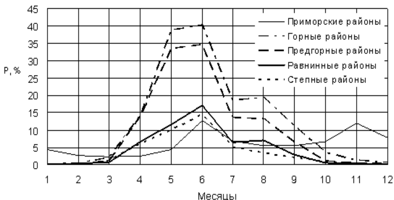
Рис. 5.6 – Сезонный ход повторяемости числа дней с градом в приморских, горных, предгорных и равнинных районах Северного Кавказа в период 1952 – 2008 гг. по данным 54 метеостанций [7]
