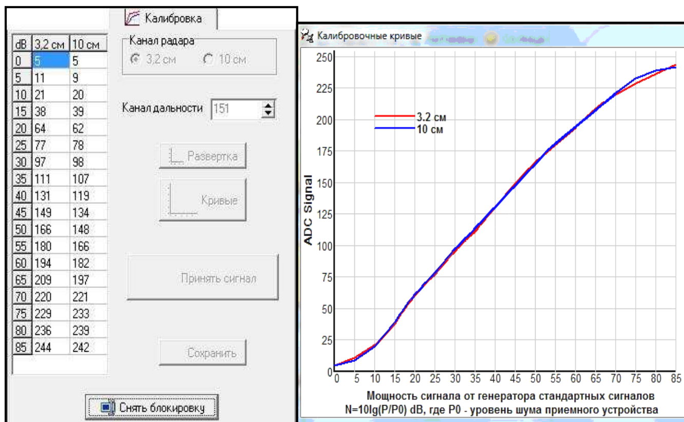
Рис. 12.7 – Панель градуировки измерительного тракта «АСУ-МРЛ» (слева) и градуировочные кривые измерительных трактов обоих каналов МРЛ-5 (справа)
