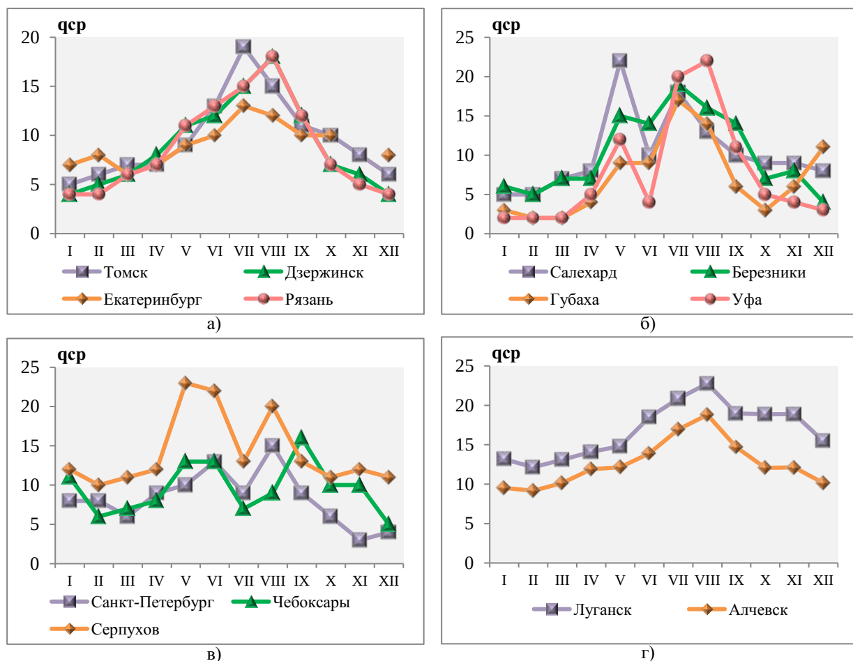
Рисунок 2.48 — Годовой ход средних за месяц концентраций формальдегида ( q_{ср} , \text{мкг/м}^3 ), в городах России в 2023 году
