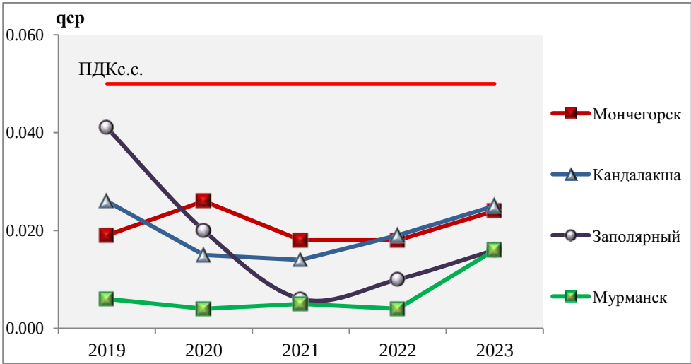
Рисунок 3.14 — Среднегодовые концентрации (qср, мг/м³) диоксида серы в период 2019–2023 гг.
