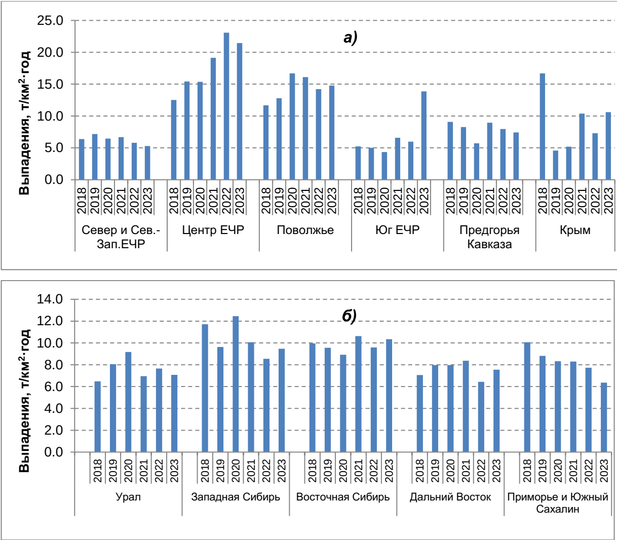
Рисунок 5.6а — Временной ход средних за год влажных выпадений суммы ионов, Р на ЕЧР (а), АЧР (б) т/км 2 ·год
