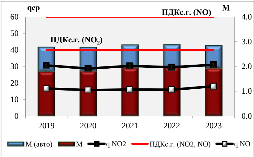
Рисунок 2.25 — Среднегодовые концентрации диоксида ( q_{NO_2} , мкг/м³), оксида азота ( q_{NO} , мкг/м³) и выбросы NO x (в пересчете на NO 2 ) от стационарных источников (M, млн т) и автотранспорта (M, млн т) NO x (в пересчете на NO 2 )
