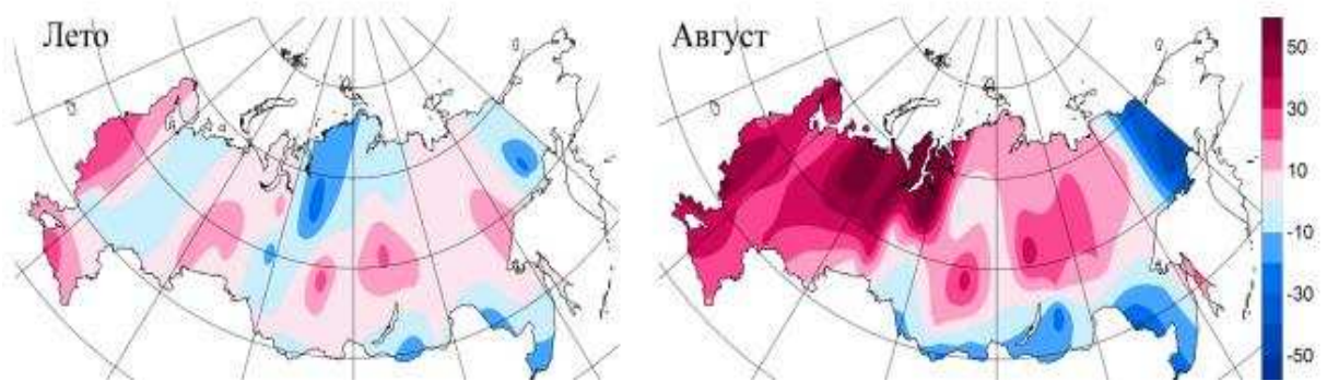
Рисунок 3.18 — Аномалии (в процентах от среднего за 1961–1990 гг.) сезонных (лето 2023 года) и месячных (август) сумм прямой солнечной радиации.
