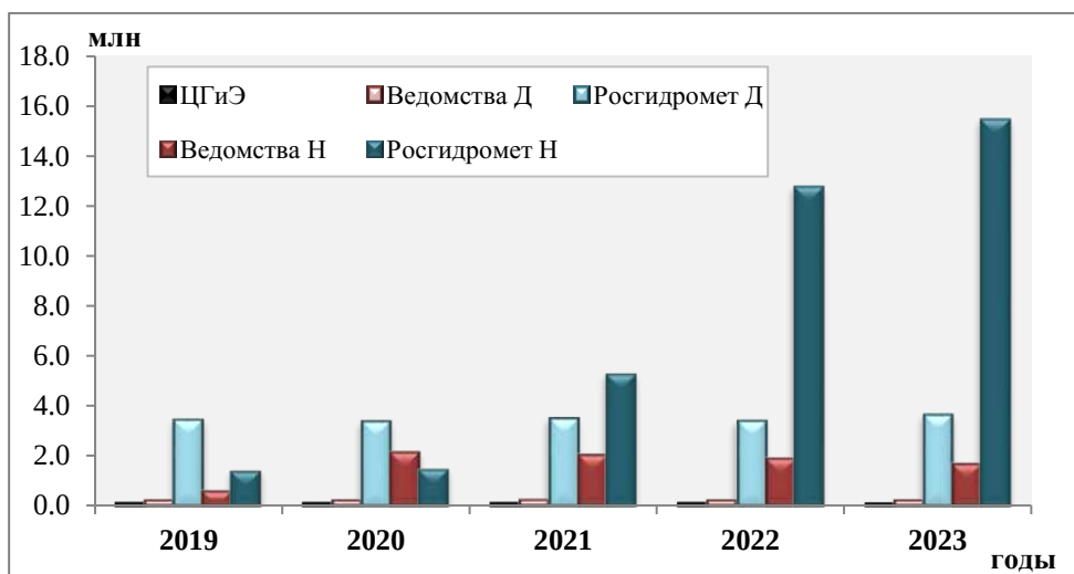
Рисунок 1.3 — Объем данных дискретных (Д) и непрерывных (Н) наблюдений (млн измерений), выполненных на сети Росгидромета, Роспотребнадзора (ЦГиЭ), других ведомств в 2019–2023 гг.
