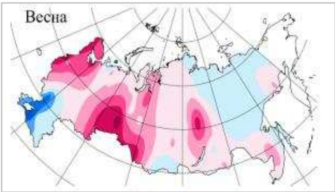
Рисунок 2.42 — Аномалии сезонных сумм прямой солнечной радиации. Весна 2023 года
