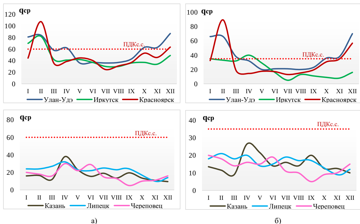
Рисунок 2.22 — Годовой ход средних за месяц концентраций ( q_{ср} , мкг/м^3 ) PM_{10} (а) и PM_{2.5} (б) в городах на территории России в 2023 году
