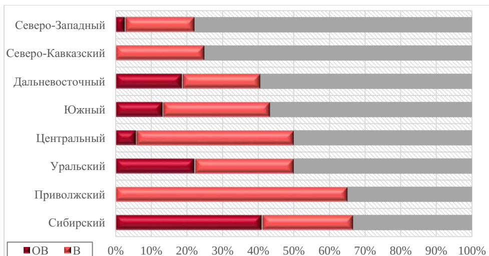
Рисунок 2.16 — Количество городов (%) с высоким (В) и очень высоким (ОВ) уровнем загрязнения воздуха в федеральных округах РФ в 2023 году
