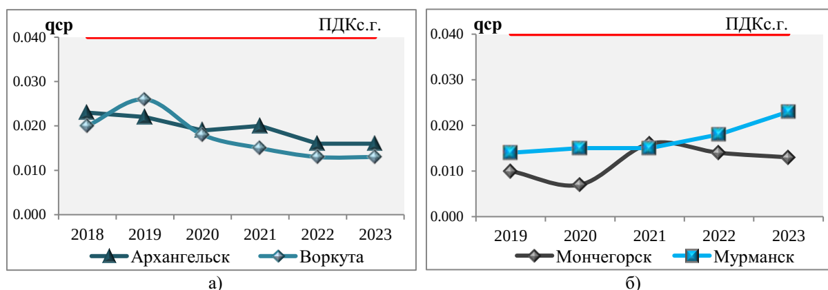
Рисунок 3.12 — Среднегодовые концентрации (qср, мг/м³) диоксида азота за период 2019–2023 гг.
