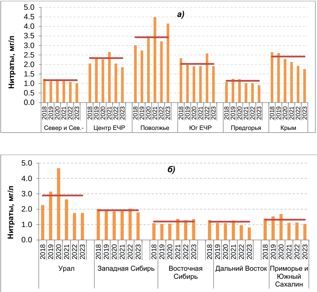
Рисунок 5.4 — Изменение средневзвешенной концентрации нитратов в осадках ЕЧР (а) и АЧР (б) Примечание: красной линией показано среднее содержание за 2018–2022 гг.
