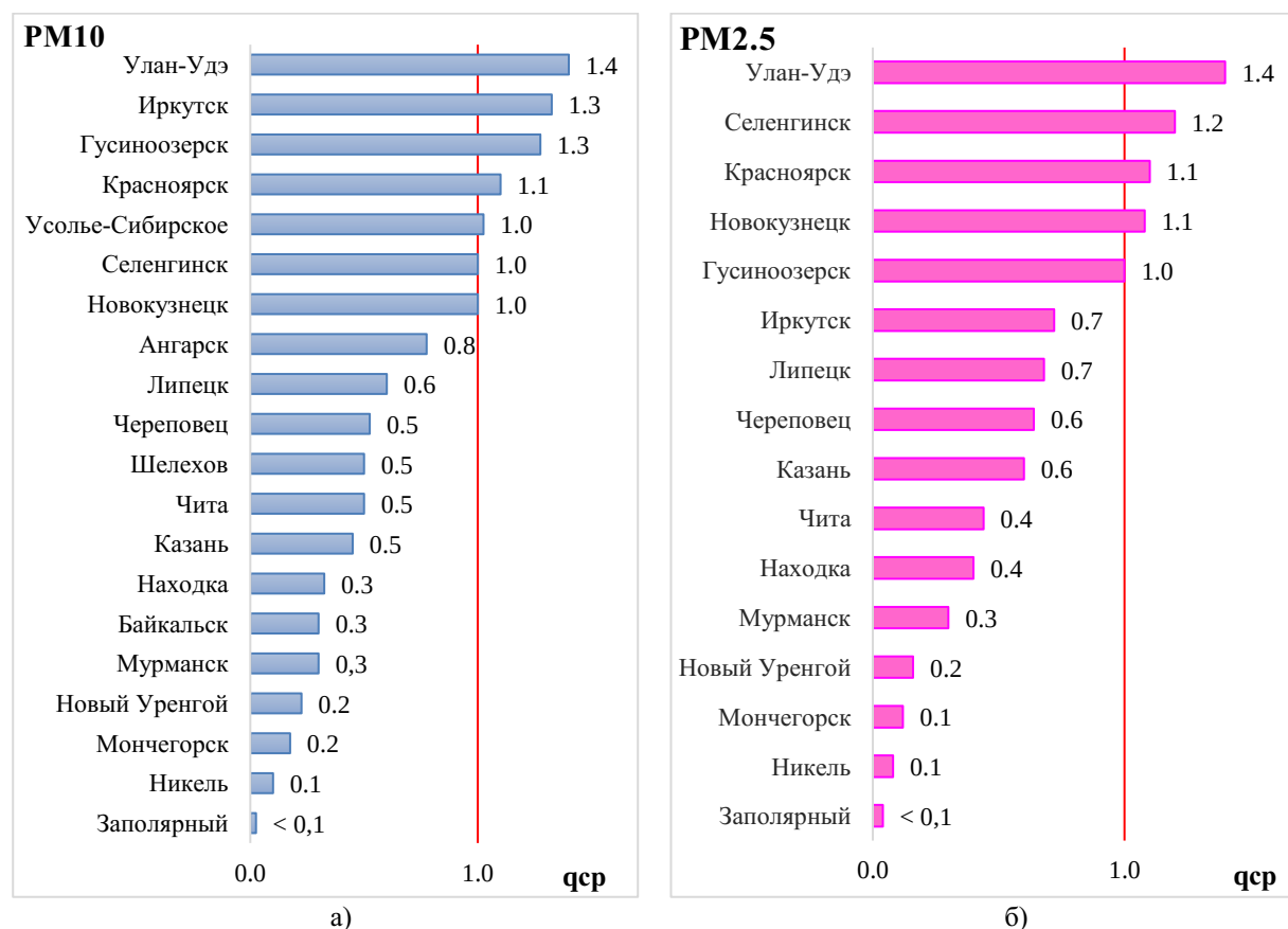
Рисунок 2.21 — Среднегодовые концентрации (qср, ПДК с.г. ) взвешенных частиц PM10 (а) и PM2.5 (б) в городах на территории России в 2023 году
