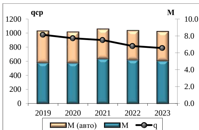
Рисунок 2.29 — Среднегодовые концентрации ( q_{\text{ср}} , \text{мкг/м}^3 ) и выбросы от стационарных источников ( M , млн т) и автотранспорта ( M , млн т) оксида углерода
