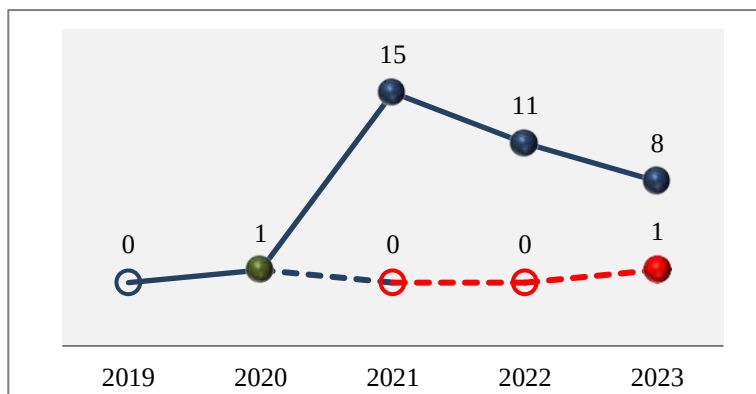
Рисунок 2.45 — Количество городов, в которых среднегодовые концентрации фенола превышали 1 ПДК с учетом прежней и новой ПДК
