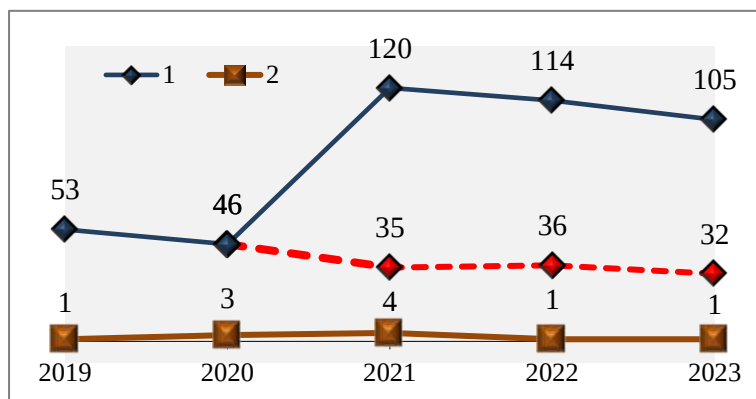
Рисунок 2.20 — Количество городов, в которых среднегодовые концентрации взвешенных веществ превышали 1 ПДК (1) с учетом прежней и новой ПДК, СИ взвешенных веществ больше 10 (2)
