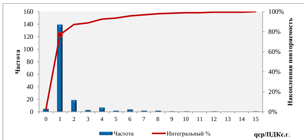
Рисунок 2.33 — Частота и накопленная повторяемость (%) среднегодовых концентраций бенз(а)пирена ( q_{cp} ) в городах России
