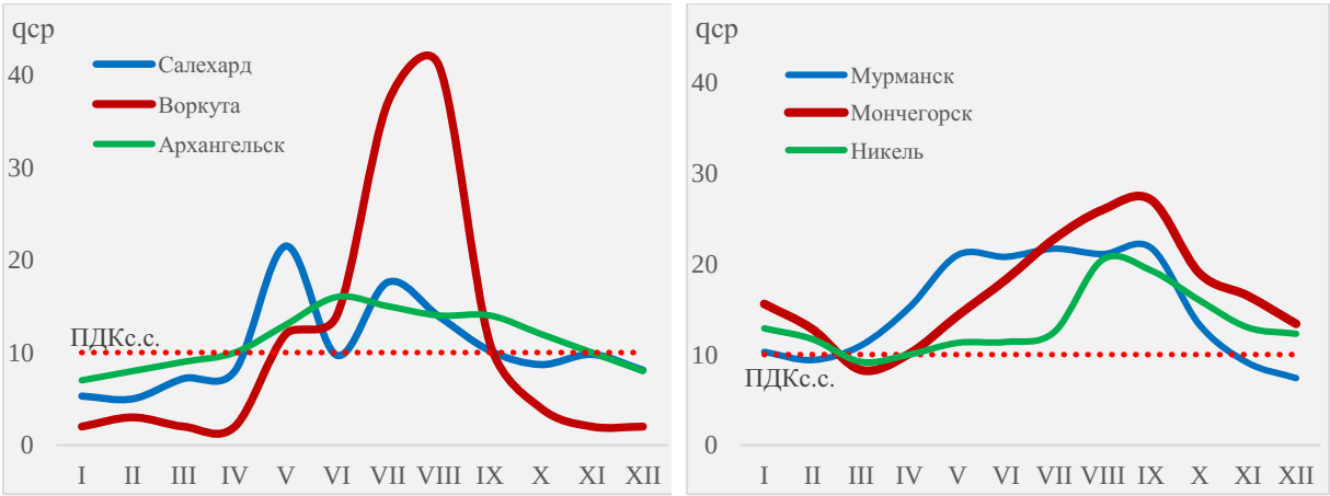
Рисунок 3.17 — Годовой ход концентраций (qср, мкг/м³) формальдегида в городах АЗРФ в 2023 году
