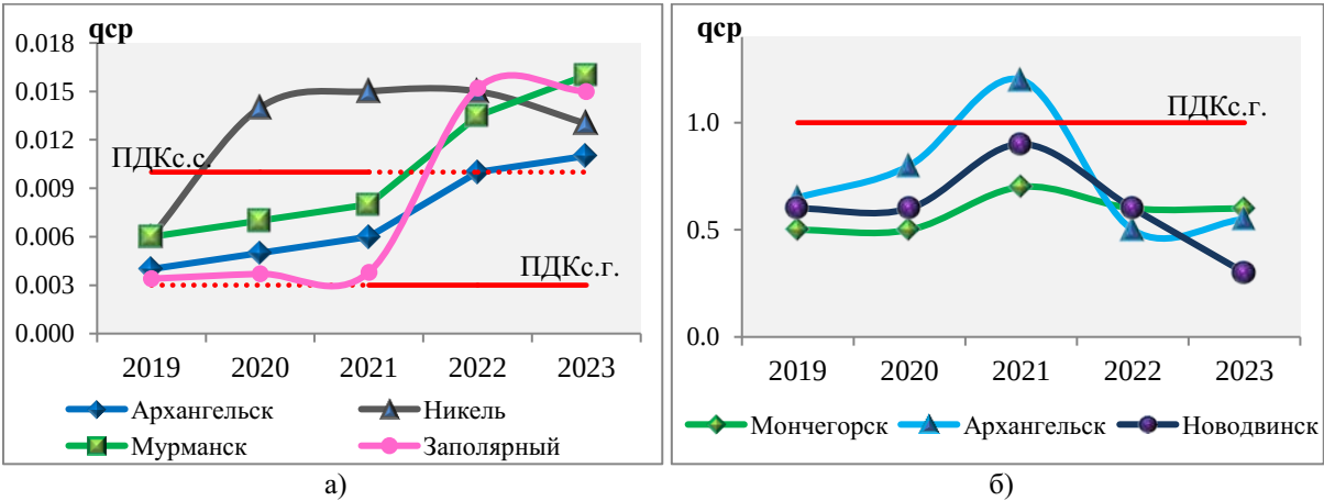
Рисунок 3.15 — Среднегодовые концентрации (qср, мг/м³) формальдегида (а) и бенз(а)пирена (qср, нг/м³) (б) в период 2019–2023 гг.
