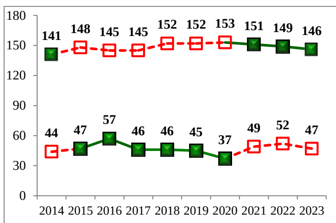
Рисунок 2.49 — Количество городов, в которых средние за год концентрации формальдегида превышают действующую в конкретный период (зеленый маркер) и отмененную (красный маркер) ПДК
