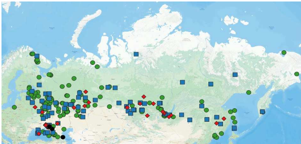
Рисунок 2.18 — Среднегодовые концентрации взвешенных веществ в городах на территории России ● — 0–1,0 ПДК, ■ — 1,1–2,0 ПДК, ◆ — 2,1–4,0 ПДК, ● — 4,1–6,4 ПДК
