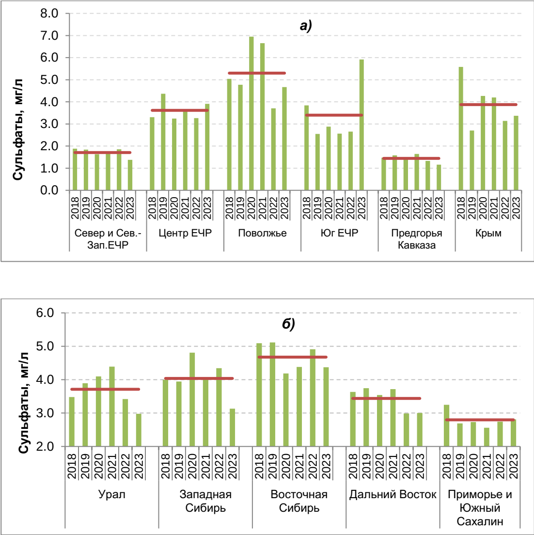
Рисунок 5.3 — Изменение средневзвешенной концентрации сульфатов в осадках ЕЧР (а) и АЧР (б)
