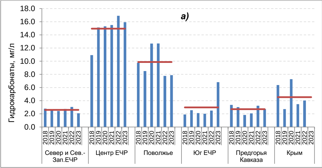
Рисунок 5.2а — Изменение средневзвешенной концентрации гидрокарбонатов в атмосферных осадках в 2023 г. на ЕЧР по сравнению со средним значением за 2018–2022 гг. Примечание: красной линией показано среднее содержание за 2018–2022 гг.
