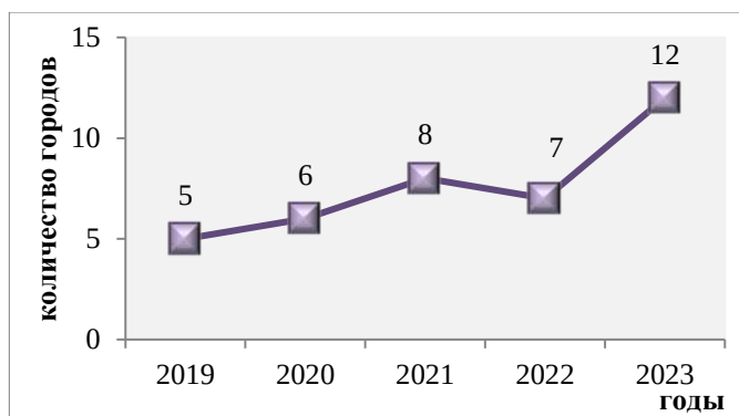
Рисунок 2.31 — Число городов, в которых среднегодовые концентрации аммиака превышают 1 ПДК
