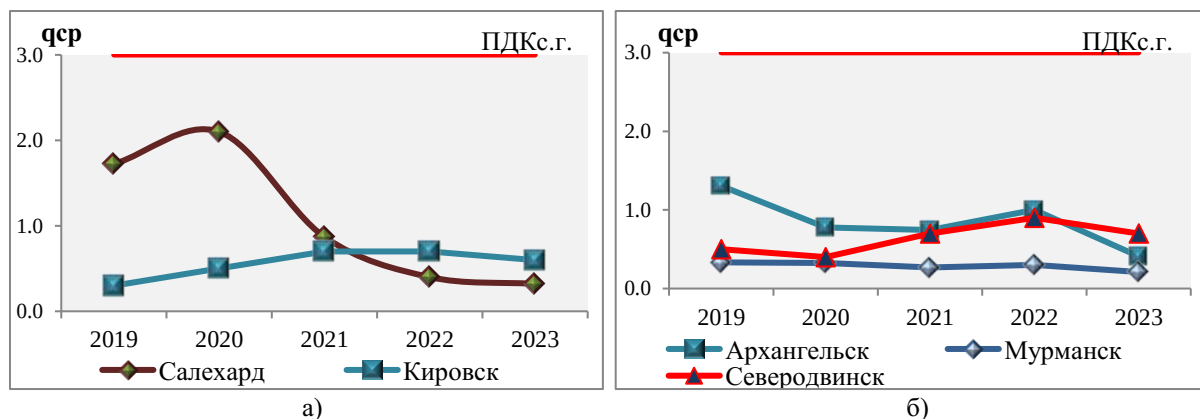
Рисунок 3.13 — Среднегодовые концентрации (qср, мг/м³) оксида углерода в период 2019–2023 гг.
