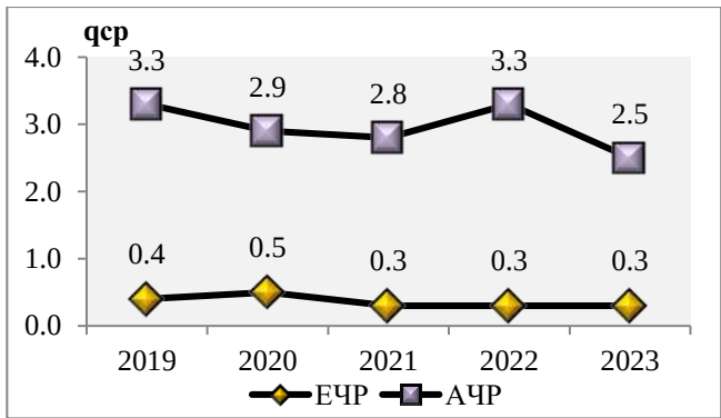
Рисунок 2.36 — Средние за год концентрации бенз(а)пирена (qср, нг/м³) на ЕЧР и АЧР за 2019–2023 гг.
