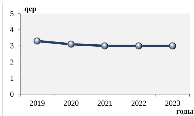
Рисунок 2.51 — Среднегодовые концентрации фторида водорода ( q_{ср} , мкг/м³)
