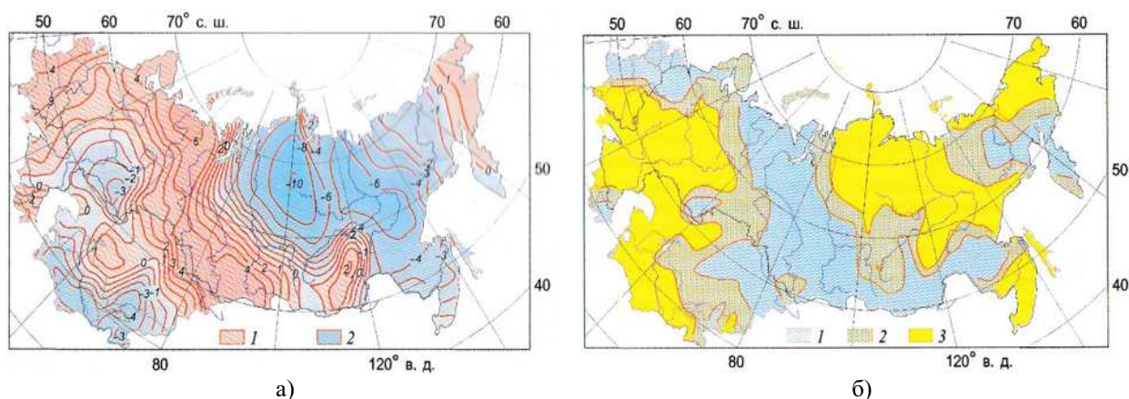
Рисунок 2.14 — Аномалии средней месячной температуры воздуха (а) и месячного количества осадков (б) в январе 2023 г.
