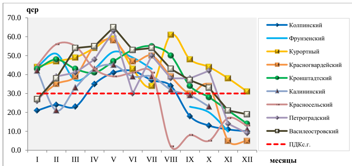
Рисунок 2.41 — Годовой ход концентраций озона ( q_{\text{ср}} , мкг/м³) на пунктах в различных районах Санкт-Петербурга
