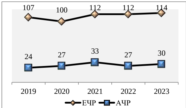
Рисунок 2.37 —Количество городов, в которых средние концентрации БП ниже ПДК на ЕЧР и АЧР за 2019–2023 гг.
