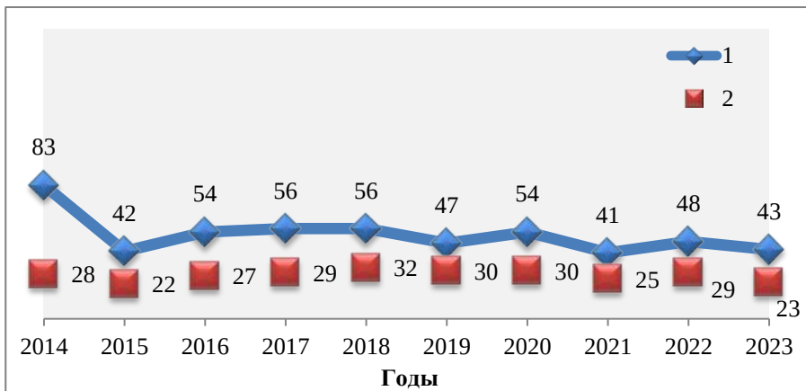
Рисунок 2.35 — Количество городов, в которых среднегодовые концентрации бенз(а)пирена превышали 1 ПДК (1), СИ бенз(а)пирена больше 10 (2) за период 2014–2023 гг.
