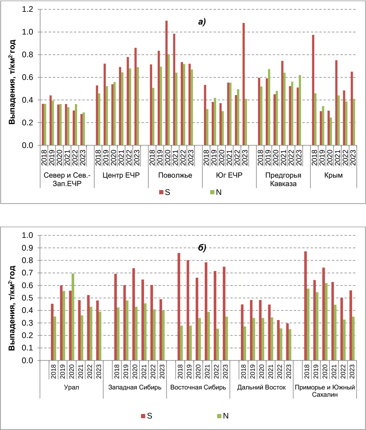
Рисунок 5.7 — Временной ход средних за год влажных выпадений суммы ионов, серы, S и суммарного азота, N (а) на ЕЧР и (б) на АЧР, т/км 2 -год
