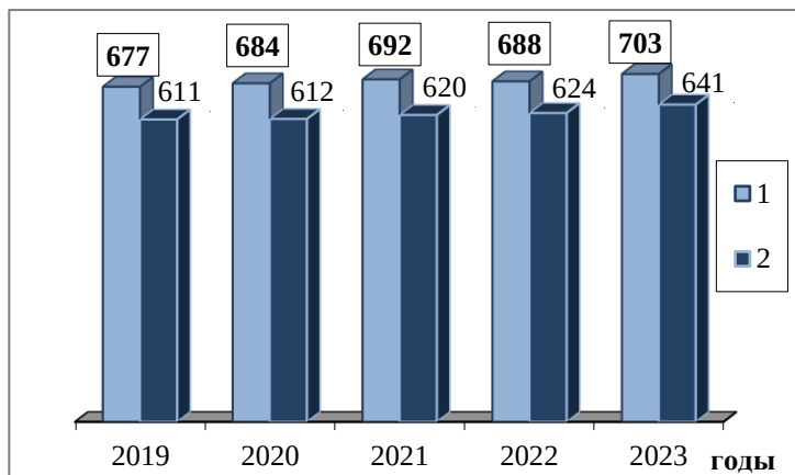
Рисунок 1.2 — Общее количество пунктов наблюдений за загрязнением атмосферного воздуха в городах (1), в том числе на сети Росгидромета (2) за период с 2019 по 2023 гг.
