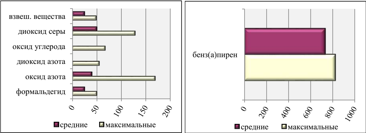
Рисунок 2.13 — Превышение (%) средних и максимальных концентраций загрязняющих веществ в городах Азиатской части территории России по отношению к тем же показателям в городах Европейской части России
