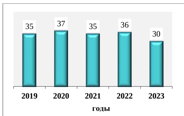
Рисунок 2.2 — Количество городов, в которых отмечались значения СИ больше 10
