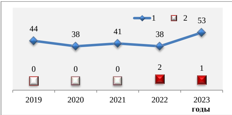
Рисунок 2.26 — Число городов, в которых среднегодовые концентрации диоксида азота превышали 1 ПДК (1), СИ диоксида азота больше 10 (2)
