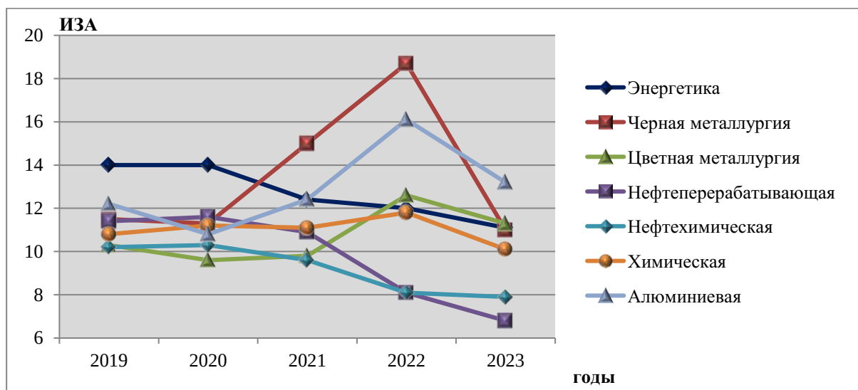
Рисунок 2.17 — Изменения ИЗА 3 за 5 лет в группах городов с крупными предприятиями различных отраслей промышленности
