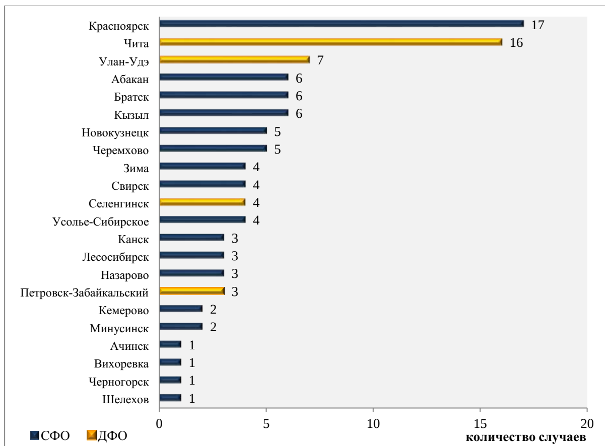
Рисунок 2.39 — Количество случаев превышений 10 ПДК среднемесячными концентрациями бенз(а)пирена в городах Сибирского (СФО) и Дальневосточного (ДФО) федеральных округов
