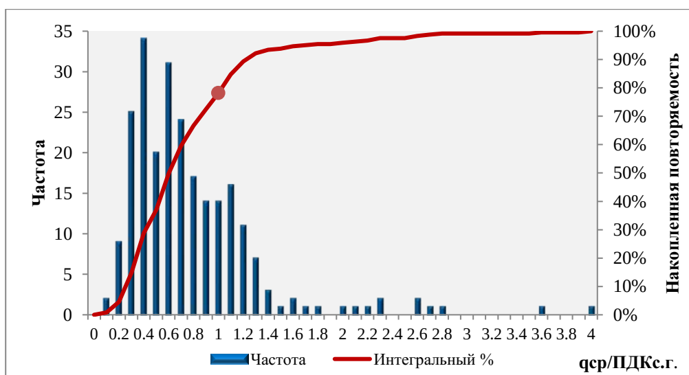
Рисунок 2.24 — Частота и накопленная повторяемость (%) среднегодовых концентраций ( q_{ср} ) диоксида азота в городах России
