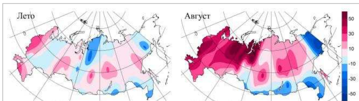
Рисунок 2.15 — Аномалии (в процентах от среднего за 1961—1990 гг.) сезонных и месячных (август) сумм прямой солнечной радиации. Лето 2023 года
