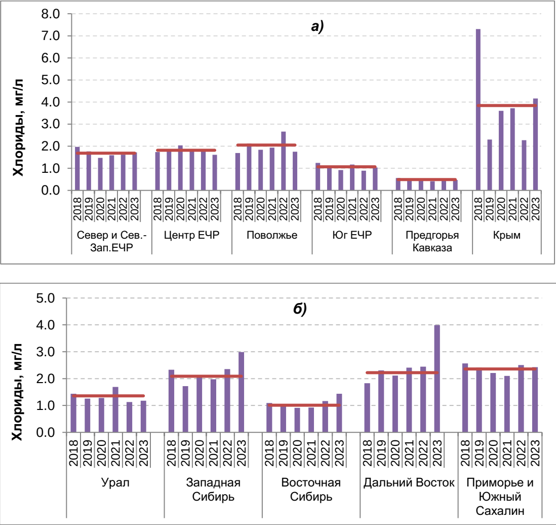
Рисунок 5.5 — Изменение средневзвешенной концентрации хлоридов в осадках ЕЧР (а) и АЧР (б) Примечание: красной линией показано среднее содержание за 2018–2022 гг.
