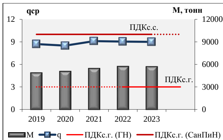
Рисунок 2.50 — Среднегодовые концентрации формальдегида ( q_{ср} , \text{мкг/м}^3 ), величины санитарно-гигиенического норматива (ПДК, \text{мкг/м}^3 ), выбросы от стационарных источников (М, тонн)
