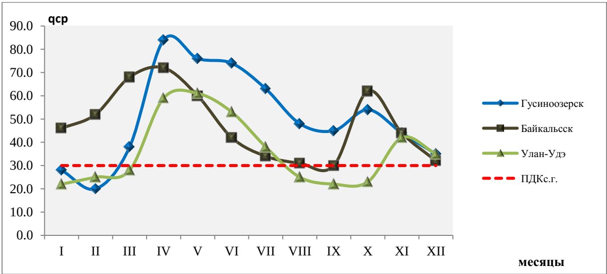
Рисунок 2.43 — Годовой ход концентраций озона (qср, мкг/м³) в городах Республики Бурятия
