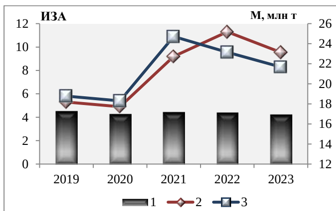
Рисунок 2.4 — Изменения выбросов от стационарных источников (М, млн т) (1), ИЗА в крупнейших городах (2) и в целом по городам России (3) за период 2019–2023 гг.
