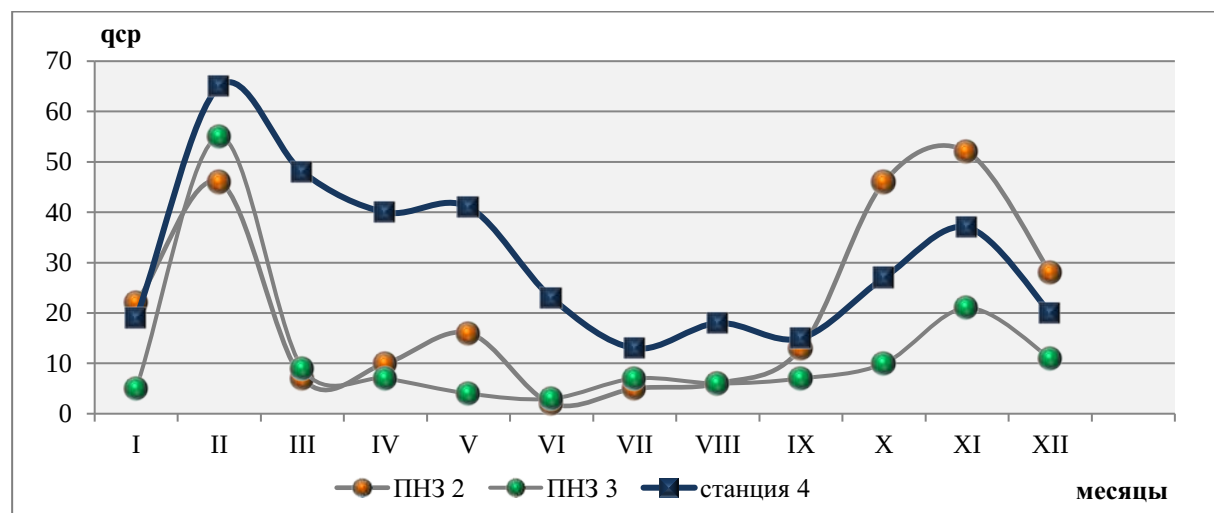
Рисунок 2.27 — Среднемесячные концентрации диоксида серы ( q_{ср} , \text{мкг/м}^3 ) по данным дискретных (ПНЗ № 2, 3) и непрерывных наблюдений (станция 4) в г. Мончегорск за 2023 г.
