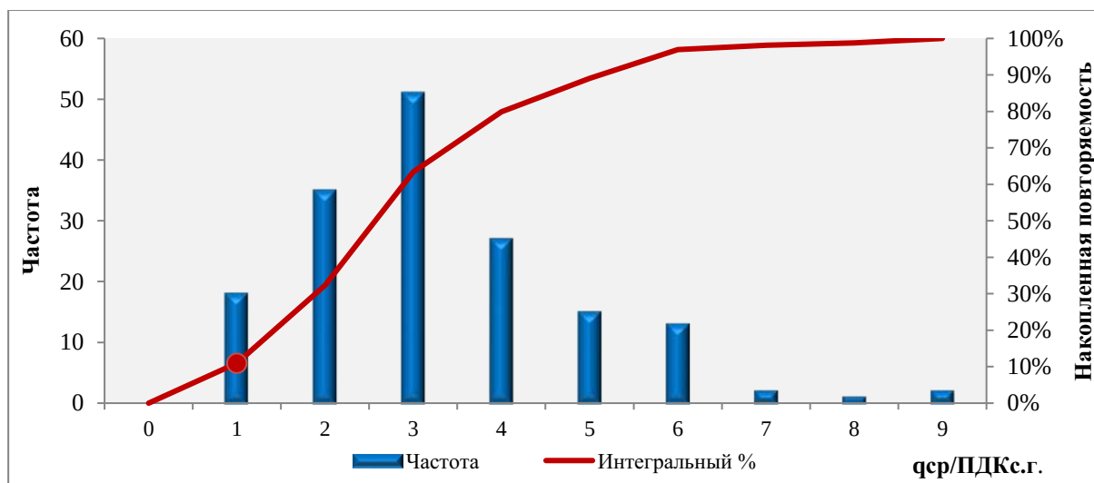
Рисунок 2.47 — Частота и накопленная повторяемость, %, среднегодовых концентраций формальдегида (qср) в городах России
