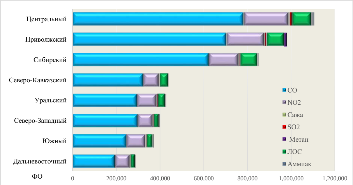
Рисунок 3.2 — Выбросы загрязняющих веществ (М, тонн) от стационарных источников (а) и автотранспорта (б) в федеральных округах РФ в 2023 году
