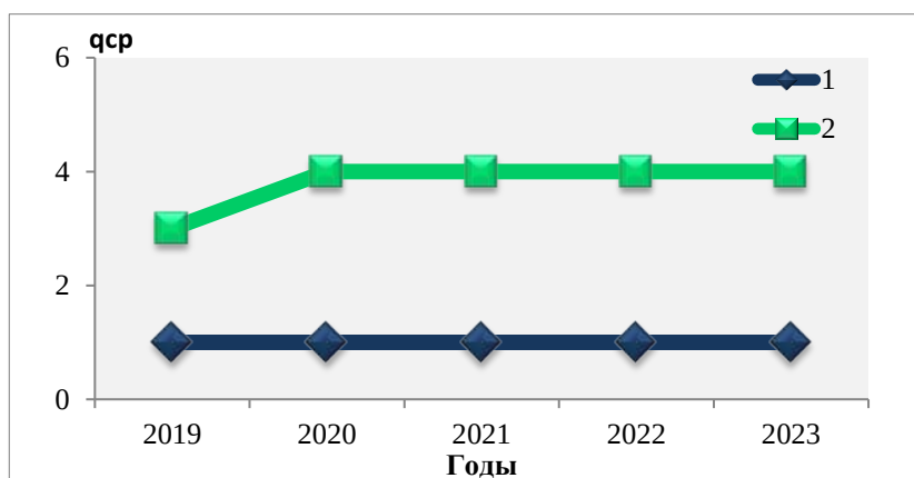
Рисунок 2.44 — Среднегодовые концентрации ( q_{\text{ср}} , мкг/м 3 ) сероводорода (1) и сероуглерода (2) за период 2019–2023 гг.
