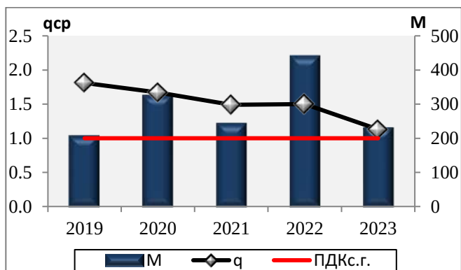
Рисунок 2.34 — Среднегодовые концентрации (qср, нг/м³) и выбросы бенз(а)пирена от стационарных источников (М, тонн)
