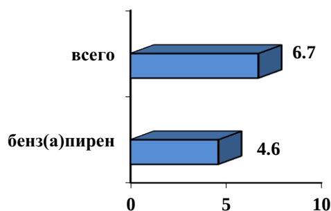
Рисунок 2.11 — Число жителей в городах (млн), находящихся под воздействием максимальных концентраций загрязняющих веществ в воздухе выше 10 ПДК
