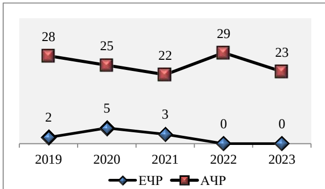
Рисунок 2.38 — Количество городов, в которых наибольшие за месяц (или за сутки) концентрации бенз(а)пирена превышали 10 ПДК на ЕЧР и АЧР за 2019–2023 гг.
