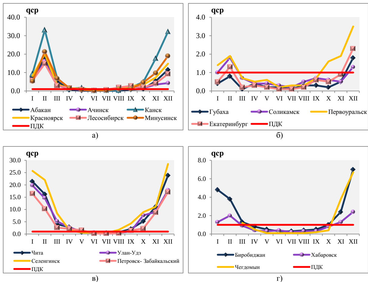
Рисунок 2.40 — Годовой ход изменений средних за месяц концентраций бенз(а)пирена (qср, нг/м³) в городах России в 2023 году
