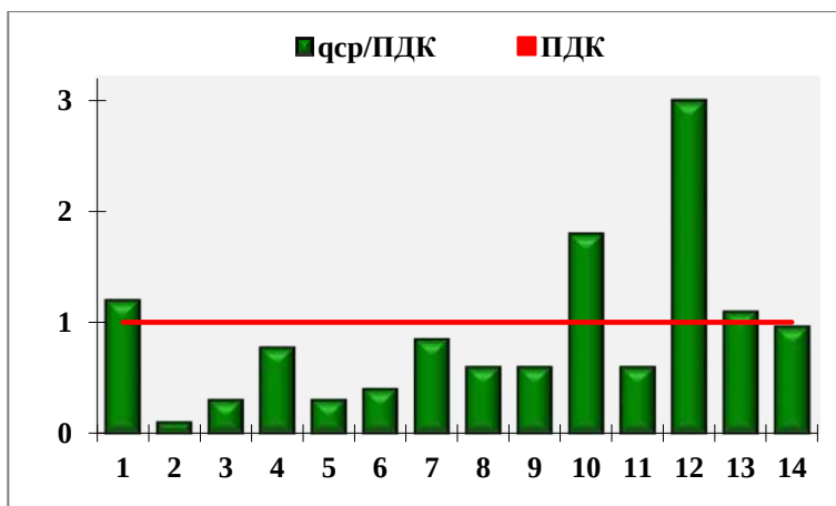
Рисунок 2.7 — Средние концентрации загрязняющих веществ q_{ср} , ПДК, в городах России: 1 — взвешенные вещества (232), 2 — диоксид серы (242), 3 — оксид углерода (237), 4 — диоксид азота (246), 5 — оксид азота (187), 6 — сероводород (120), 7 — сероуглерод (4), 8 — фенол (102), 9 — фторид водорода (31), 10 — хлорид водорода (32), 11 — аммиак (83), 12 — формальдегид (166), 13 — бенз(а)пирен (187), 14 — приземный озон (19). Цифры в скобках указывают количество городов, в которых проводились регулярные наблюдения за загрязняющими веществами.
