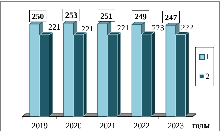
Рисунок 1.1 — Общее количество городов с наблюдениями за загрязнением воздуха (1), в том числе на сети Росгидромета (2) за период с 2019 по 2023 гг.
