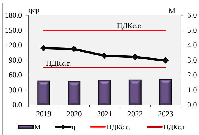
Рисунок 2.19 — Среднегодовые концентрации ( q_{ср} , \text{мкг/м}^3 ) взвешенных веществ и выбросы (M, млн т) твердых веществ от стационарных источников
