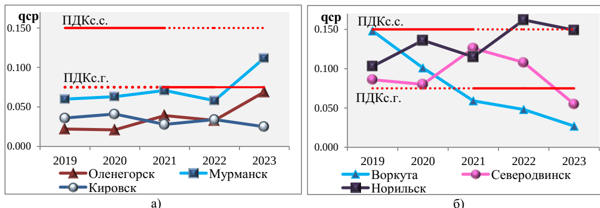
Рисунок 3.11 — Среднегодовые концентрации (qср, мг/м³) взвешенных веществ за период 2019–2023 гг.
