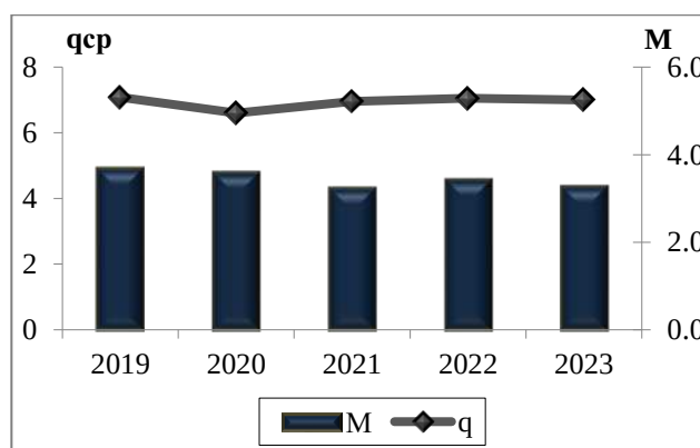
Рисунок 2.28 — Среднегодовые концентрации диоксида серы ( q_{ср} , \text{мкг/м}^3 ) и выбросы диоксида серы от стационарных источников ( M , млн т)
