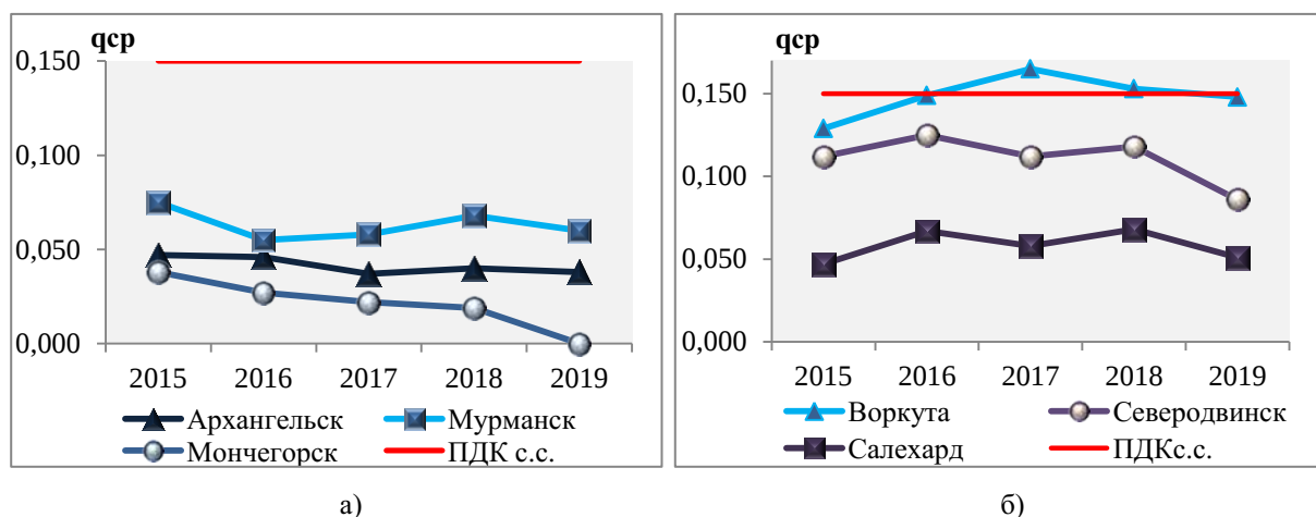
Рисунок 3.10 — Среднегодовые концентрации ( q_{ср} , mg/m^3 ) взвешенных веществ за период 2015–2019 гг.
