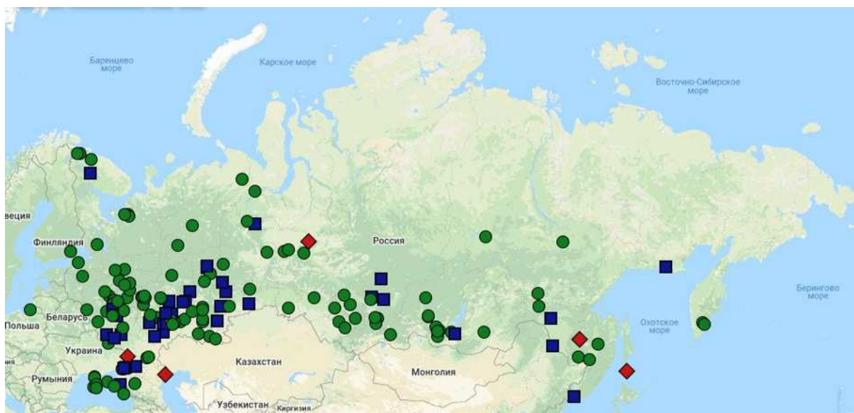
Рисунок 2.43 — Средние за год концентрации формальдегида в городах России ● - 0–1,0 ПДК, ■ - 1,1–2,0 ПДК, ◆ - 2,1–6,2 ПДК
