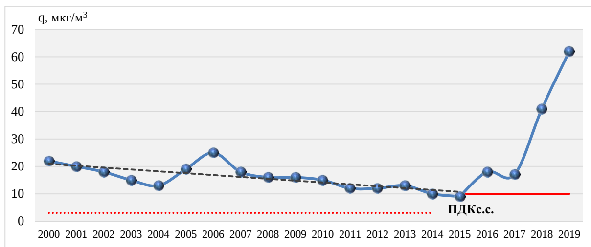
Рисунок 2.15 — Средние за год концентрации ( q , \text{мкг/м}^3 ) формальдегида в Южно-Сахалинске за период 2000–2019 гг.
