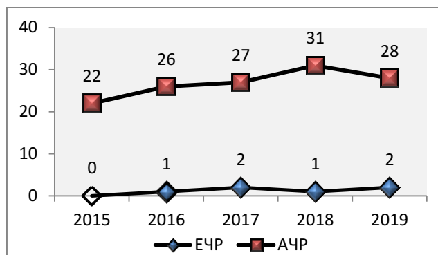
Рисунок 2.36 — Количество городов, в которых наибольшая за месяц (или за сутки) концентрации бенз(а)пирена превышала 10 ПДК на ЕЧР и АЧР за 2015–2019 гг.
