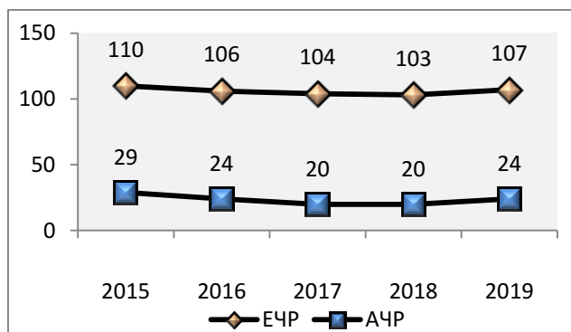
Рисунок 2.35 — Количество городов, в которых средние концентрации БП ниже ПДК на ЕЧР и АЧР за 2015–2019 гг.
