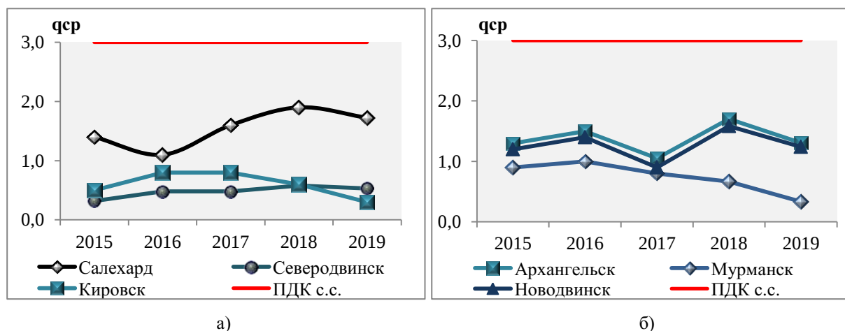
Рисунок 3.12 — Среднегодовые концентрации ( q_{ср} , mg/m^3 ) оксида углерода в период 2015–2019 гг.
