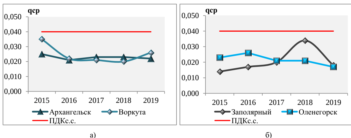
Рисунок 3.11 — Среднегодовые концентрации ( q_{ср} , mg/m^3 ) диоксида азота за период 2015–2019 гг.
