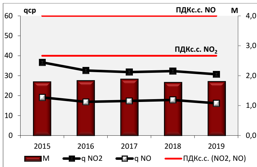
Рисунок 2.23 — Среднегодовые концентрации диоксида ( q_{NO_2} , мкг/м 3 ), оксида азота ( q_{NO} , мкг/м 3 ) и выбросы NO_x (в пересчете на NO_2 ) от стационарных источников (M, млн т)
