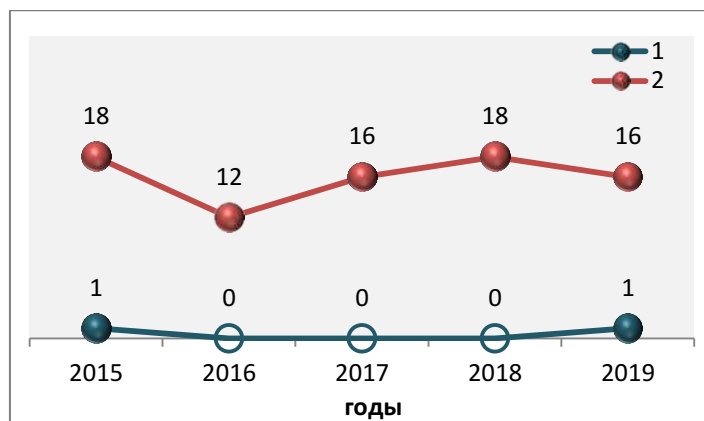
Рисунок 2.42 — Количество городов, в которых среднегодовые концентрации фенола превышают прежнюю (2) и новую (1) ПДКс.с.
