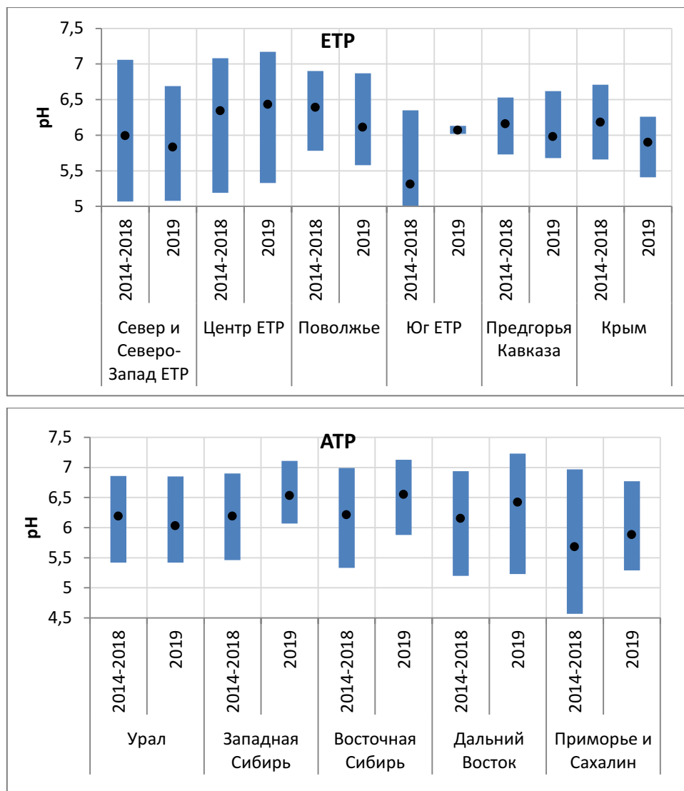
Рисунок 5.6 — Диапазон распределения среднегодовых значений pH осадков ЕТР и АТР в 2014-2018 гг. и в 2019 г.
