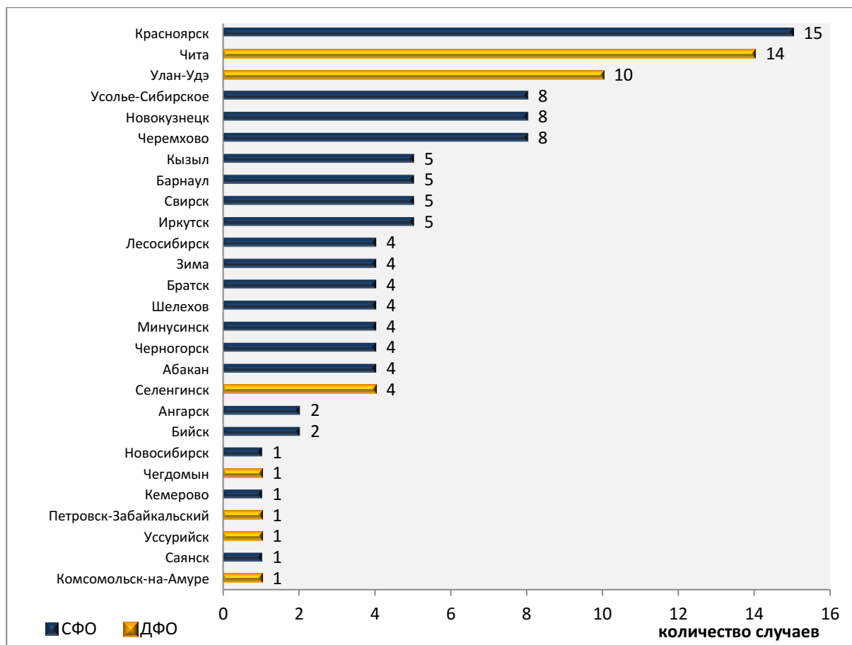
Рисунок 2.38 — Количество случаев превышений 10 ПДК среднемесячными концентрациями бенз(а)пирена в городах Сибирского (СФО) и Дальневосточного (ДФО) федеральных округов
