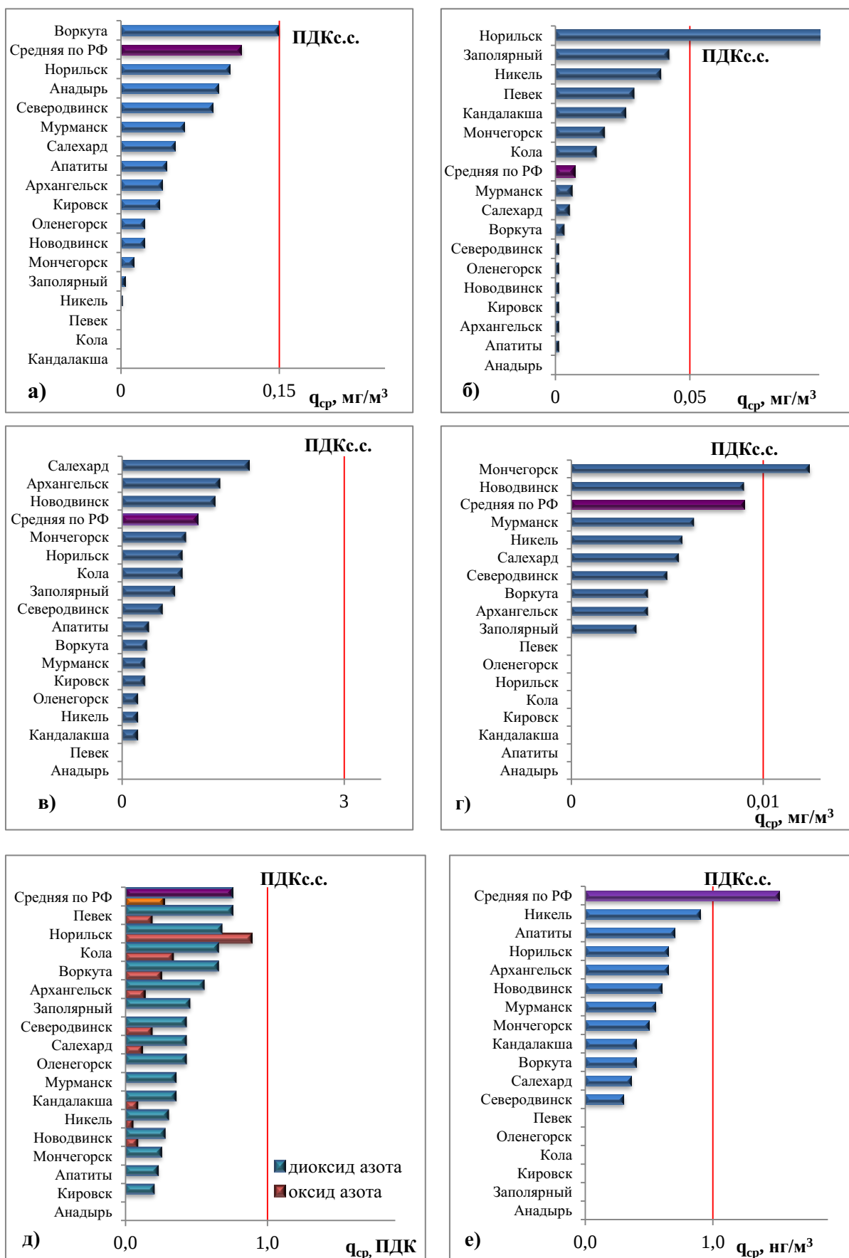
Рисунок 3.15 — Средние за год концентрации: взвешенных веществ (а), диоксида серы (б), оксида углерода (в), формальдегида (г) ( q_{ср} , мг/м 3 ), диоксида и оксида азота (д) ( q_{ср} , ПДК), бенз(а)пирена (е) ( q_{ср} , нг/м 3 ), в городах АЗРФ и в целом по России в 2019 году
