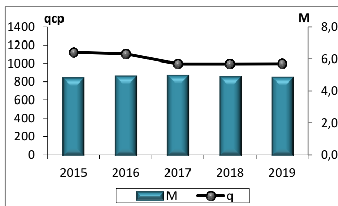
Рисунок 2.27 — Среднегодовые концентрации ( q_{\text{ср}} , \text{мкг/м}^3 ) и выбросы оксида углерода от стационарных источников (M, млн т)
