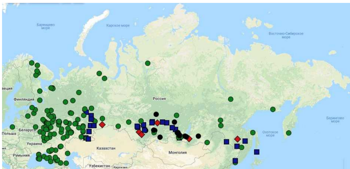
Рисунок 2.30 — Среднегодовые концентрации бенз(а)пирена в городах на территории России ● - 0–1,0 ПДК, ■ - 1,1–3,0 ПДК, ◆ - 3,1–5,0 ПДК, ● - 5,1–18,0 ПДК
