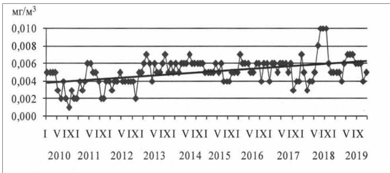
Рисунок 3.8 — Средние за месяц концентрации формальдегида, \text{мг/м}^3 , в Санкт-Петербурге [26]
