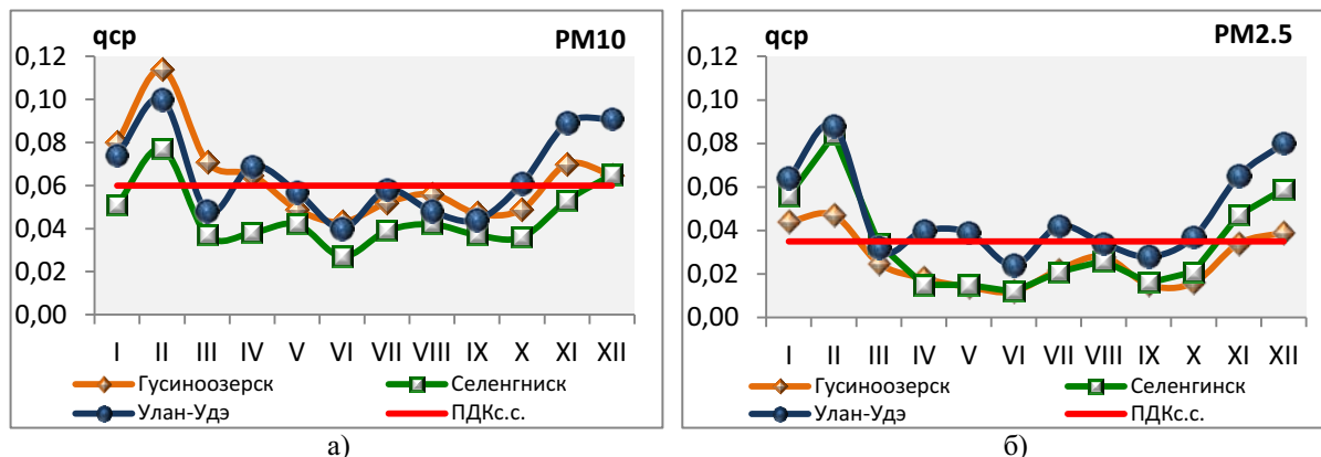
Рисунок 2.20 — Годовой ход изменений средних за месяц концентраций ( q_{ср} , мг/м^3 ) PM_{10} (а) и PM_{2.5} (б) в Гусиноозерске, Селенгинске и Улан-Удэ в 2019 году
