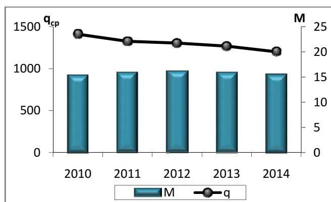
Рисунок 2.24 — Среднегодовые концентрации ( q_{ср} , мкг/м³) и суммарные выбросы (М, млн. т) оксида углерода
