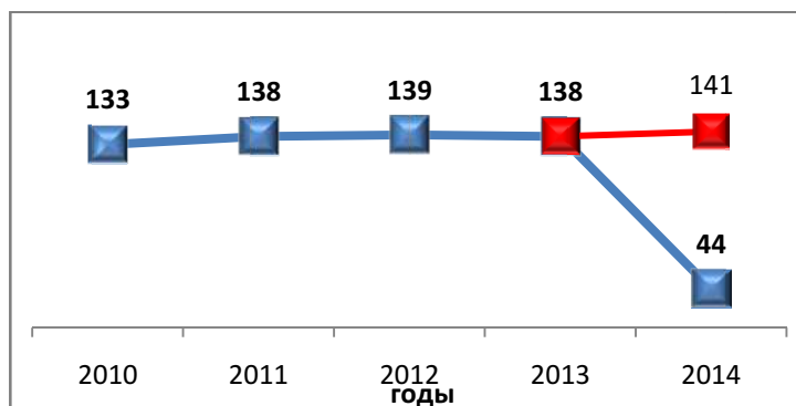
Рисунок 2.47 — Количество городов, в которых среднегодовые концентрации формальдегида превышают 1 ПДК
