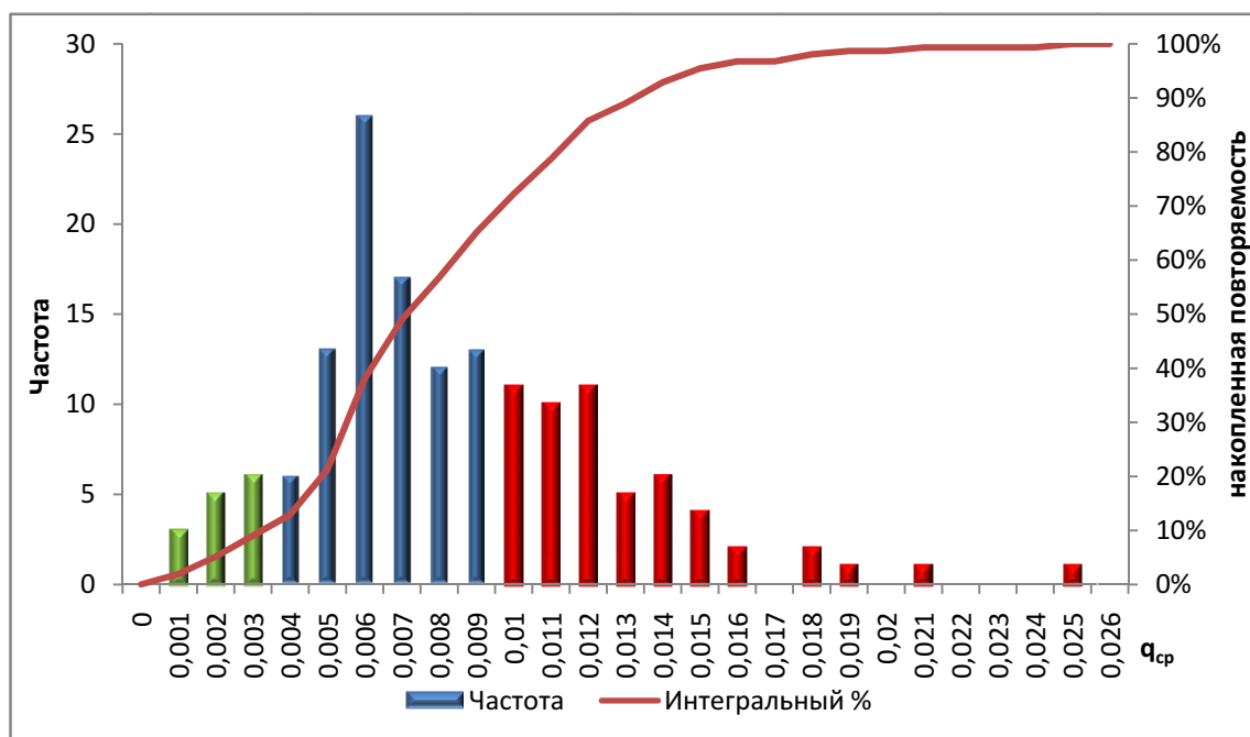
Рисунок 2.45 — Частота и накопленная повторяемость, %, среднегодовых концентраций формальдегида ( q_{ср} , мг/м³) в городах России
