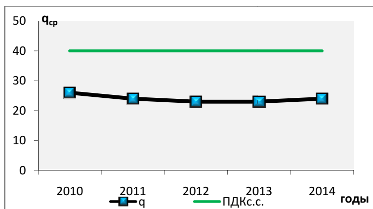
Рисунок 2.25 — Среднегодовые концентрации аммиака ( q_{ср} , мкг/м³)
