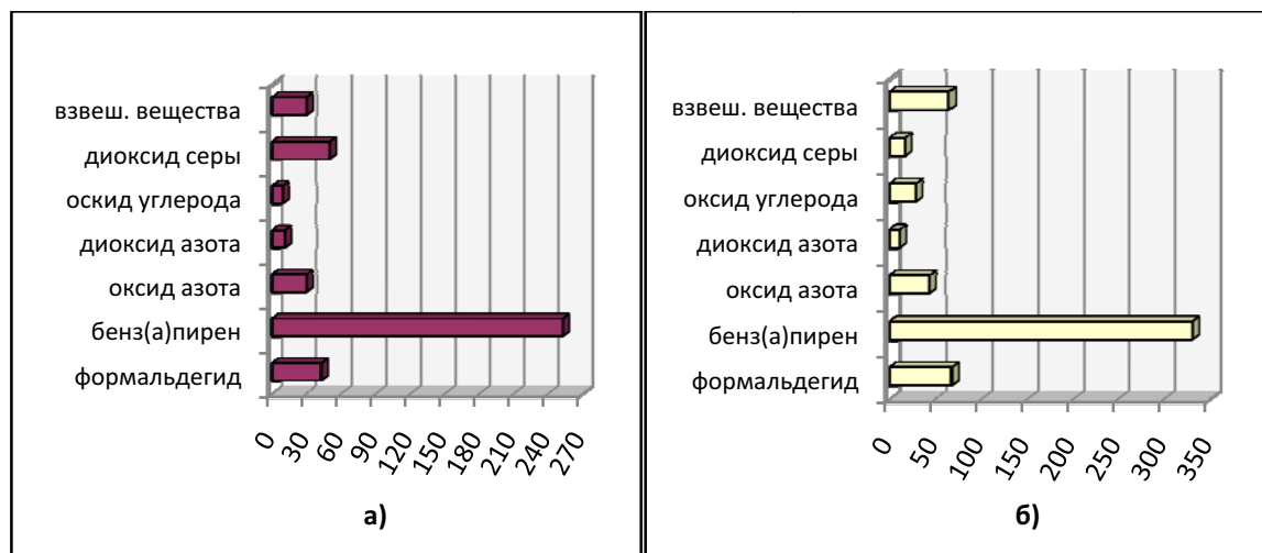
Рисунок 2.13 — Превышение (%) средних (а) и максимальных (б) концентраций примесей в городах Азиатской части территории России по отношению к тем же показателям в городах Европейской части России
