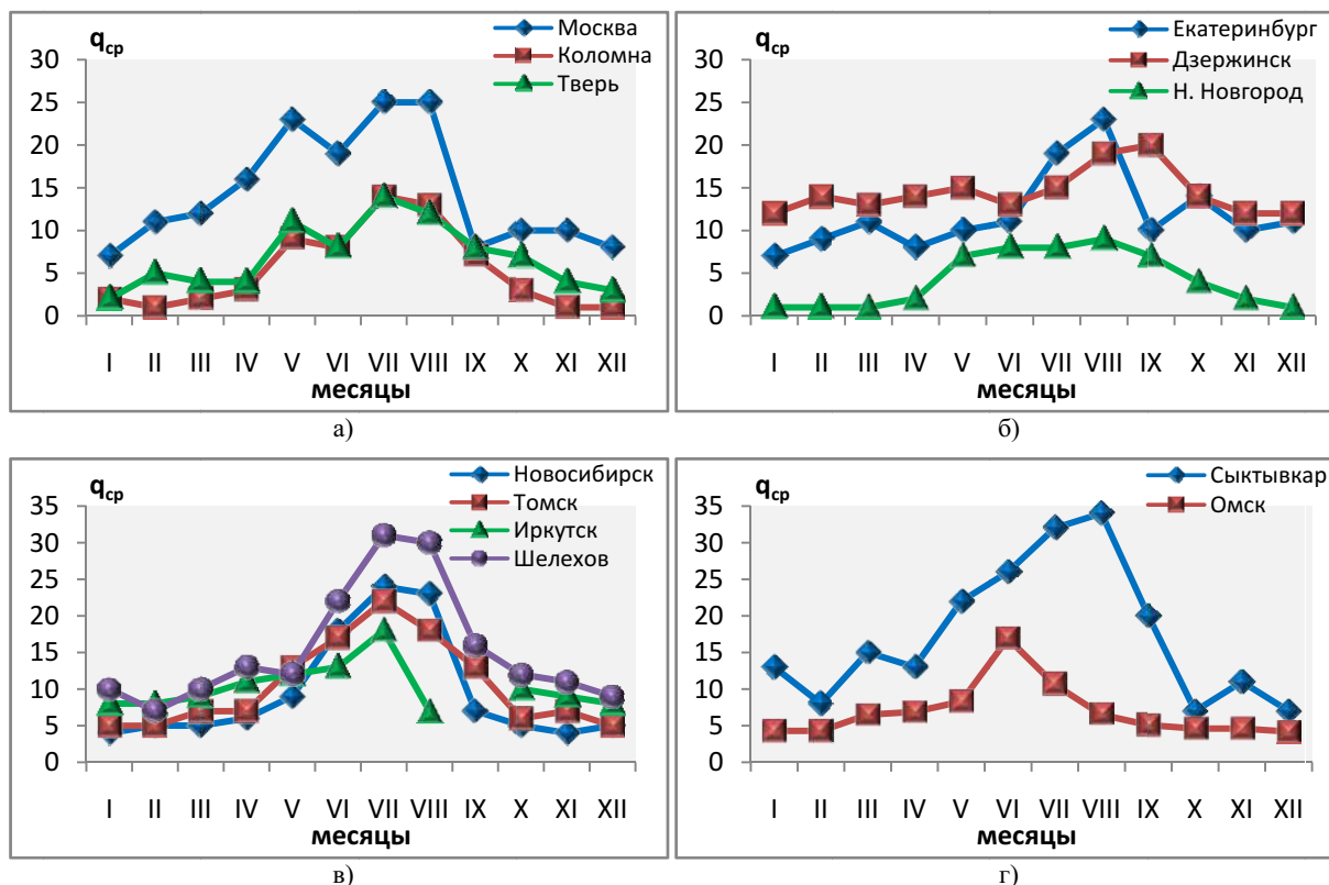
Рисунок 2.46 — Годовой ход средних за месяц концентраций формальдегида ( q_{cp} , мкг/м^3 ) в городах России в 2014 году
