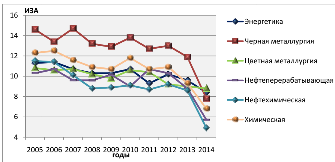
Рисунок 2.14 — Изменения ИЗА за 10 лет в группах городов с крупными предприятиями различных отраслей промышленности
