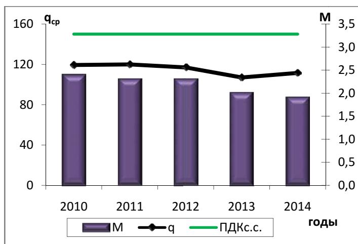
Рисунок 2.16 — Среднегодовые концентрации ( q_{cp} , мкг/м³) взвешенных веществ и суммарные выбросы (M, млн. т) твердых веществ
