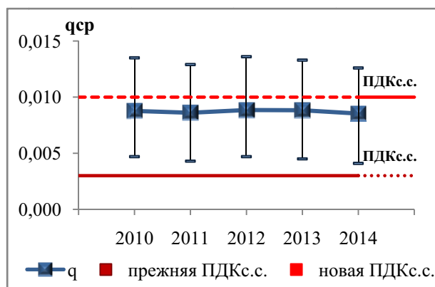
Рисунок 2.48 — Среднегодовые концентрации формальдегида ( q_{ср} , мг/м^3 ), их стандартные отклонения и величины санитарно-гигиенического норматива, ПДК с.с. , мг/м^3 .
