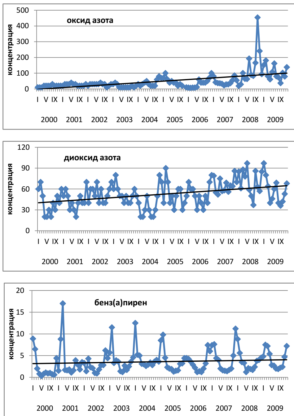
Рисунок — Средние за месяц концентрации оксида и диоксида азота, \mu\text{г}/\text{м}^3 , бенз(а)пирена, \text{нг}/\text{м}^3 , в Красноярске
