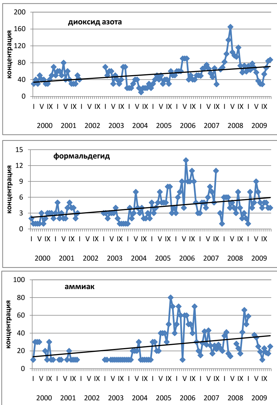
Рисунок — Средние за месяц концентрации примесей, мкг/м³, в Нижнем Новгороде
