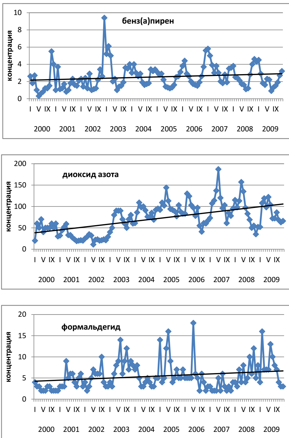
Рисунок — Средние за месяц концентрации бенз(а)пирена, \text{нг/м}^3 , диоксида азота и формальдегида, \text{мкг/м}^3 , в Казани
