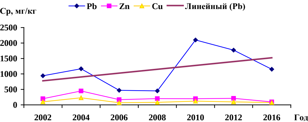
Р и с у н о к 6 – Динамика средних массовых долей ТМ в почве УМН-1 г. Свирск Иркутской области, расположенного в 0,5 км на юг от ЗАО «Актех-Байкал»
