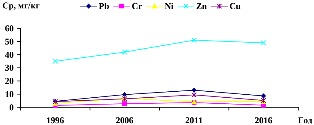
Р и с у н о к 5 – Динамика средних массовых долей ТМ в почвах территории г. Нижний Тагил: а) кислоторастворимых, б) подвижных
