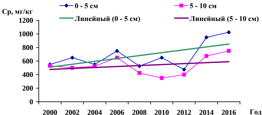
Р и с у н о к 7 – Динамика средней массовой доли фтора по валу в слое почвы от 0 до 5 см и от 5 до 10 см в районе г. Братск (пробы отобраны на удалении 2 (С), 8 (СВ), 12 (ВСВ) и 30 (СВ) км от ОАО «РУСАЛ Братск», направления указаны в скобках)
