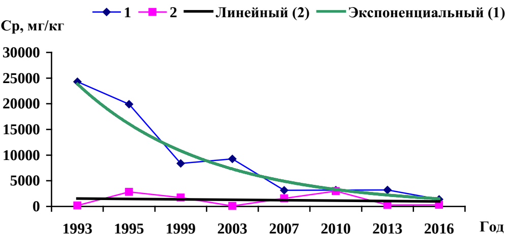
Р и с у н о к 8 – Динамика средних массовых долей НП в почвах нефтяного пятна (1) и за его пределами по разным направлениям до 250 м (2) вблизи пос. Тыреть Заларинского района Иркутской области
