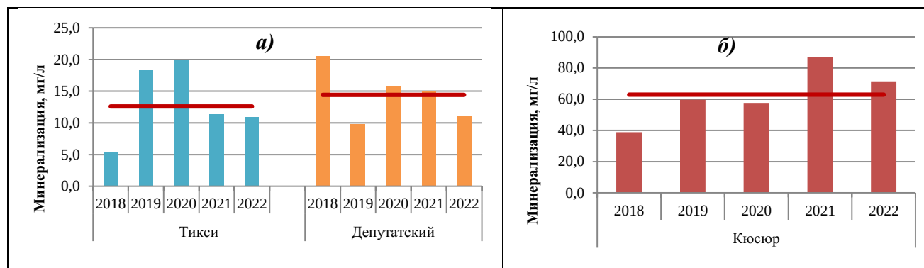
Рис. 4.42. Изменение средневзвешенной минерализации осадков на территории Якутии, 2018-2022 гг.
