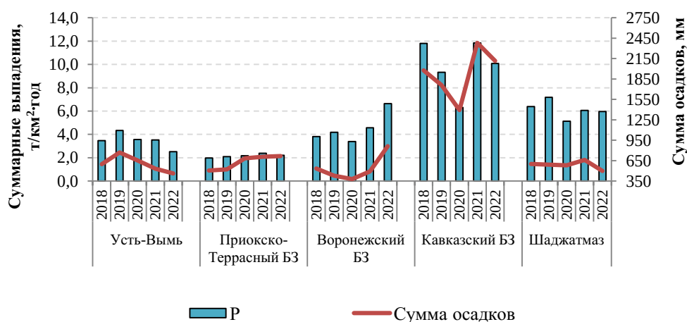
Рис. 2.23. Суммарные влажные выпадения на ЕЧР, 2018-2022 гг.
