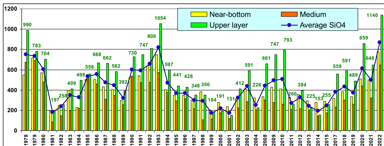
Рис. 3.60. Многолетняя динамика среднего значения содержания силикатов (мкг/дм 3 ) в приповерхностном, промежуточном и придонном слоях вод Двинского залива Белого моря в 1978-2022 гг.
