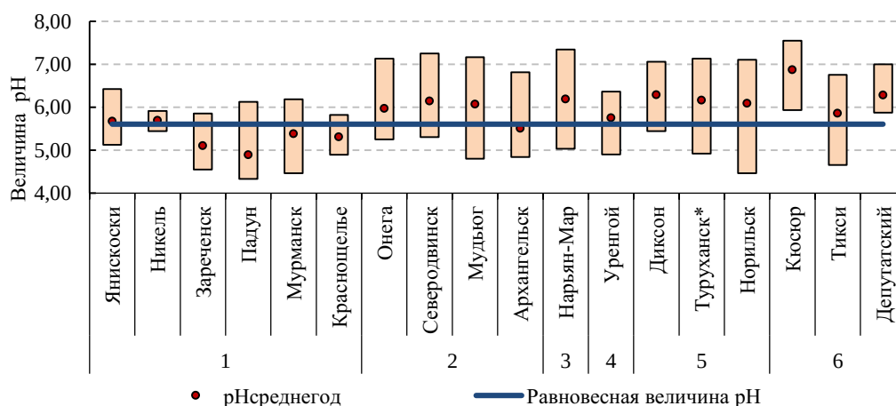
Рис. 4.43. Диапазон изменений значений pH суммарных ежемесячных проб осадков на арктических станциях в 2022 г.
