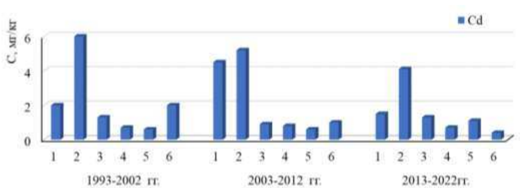
Рис. 3.22. Динамика средних по отраслям промышленности массовых долей кадмия, усредненных за разные периоды наблюдений, в почвах 5-километровых зон вокруг предприятий черной металлургии (1), цветной металлургии (2), машиностроения и металлообработки (3), топливной и энергетической промышленности (4), химической и нефтехимической промышленности (5), строительной промышленности и производства стройматериалов (6)
