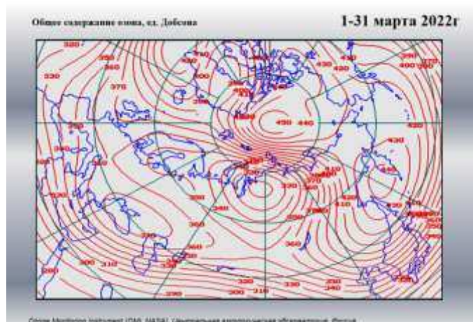
Рис. 2.13. Среднемесячное поле ОСО в марте 2022 г. над территорией Российской Федерации
