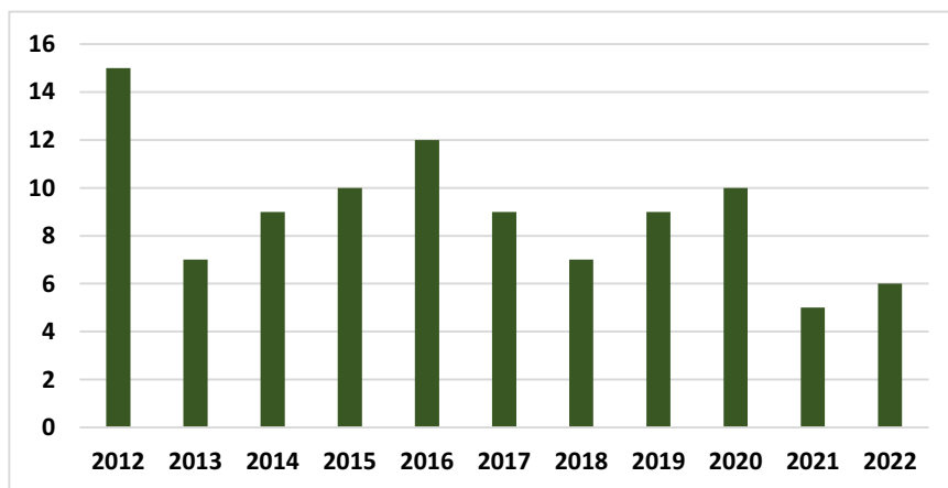
Рис. 3.28. Количество субъектов, на территориях которых отмечалось высокое содержание суммарного ДДТ в период 2012-2022 гг.
