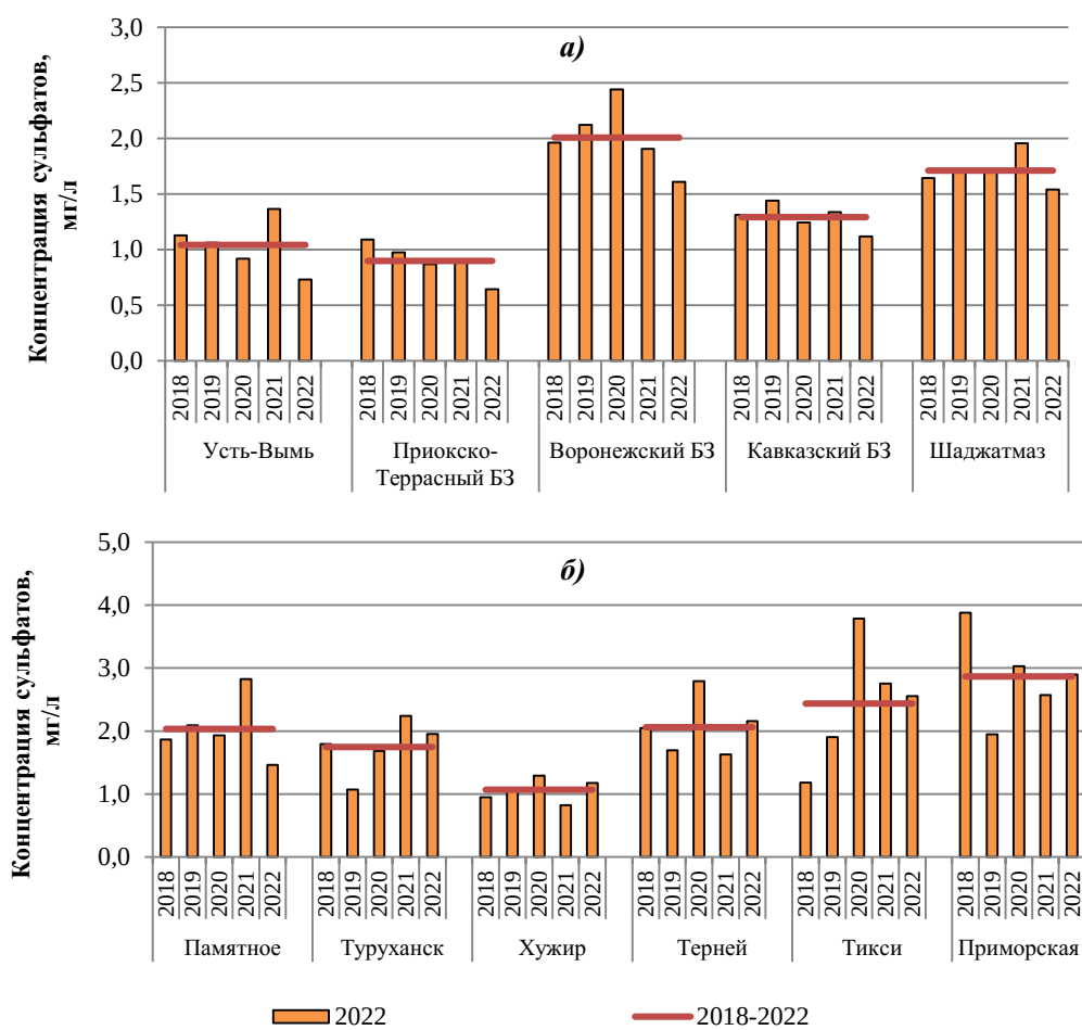
Рис. 2.20. Изменение средневзвешенной концентрации сульфатов в осадках фоновых станций ЕЧР (а) и АЧР (б), 2018-2022 гг.
