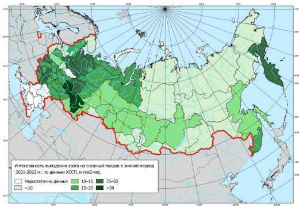
Рис. 2.33. Интенсивность выпадения азота на снежный покров в зимний период 2021-2022 гг.
