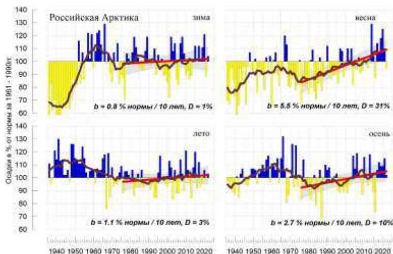
Рис. 4.34. Сезонные суммы осадков (% нормы) в Российской Арктике в 1936-2022 гг. Жирная темная кривая - 11летнее скользящее среднее. Показан линейный тренд за 1976-2022 гг.
