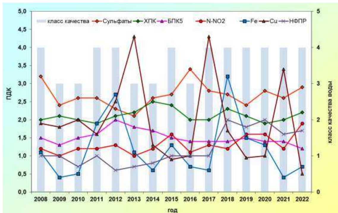
Рис. 3.40. Изменение среднегодовых концентраций отдельных загрязняющих веществ и показателей качества воды р. Дон, ниже г. Ростов-на-Дону за многолетний период
