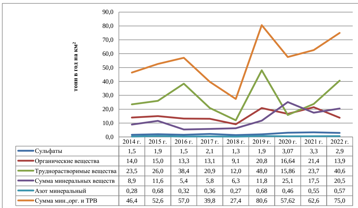
Рис. 4.11. Поступление веществ из атмосферы на ст. Байкальск
