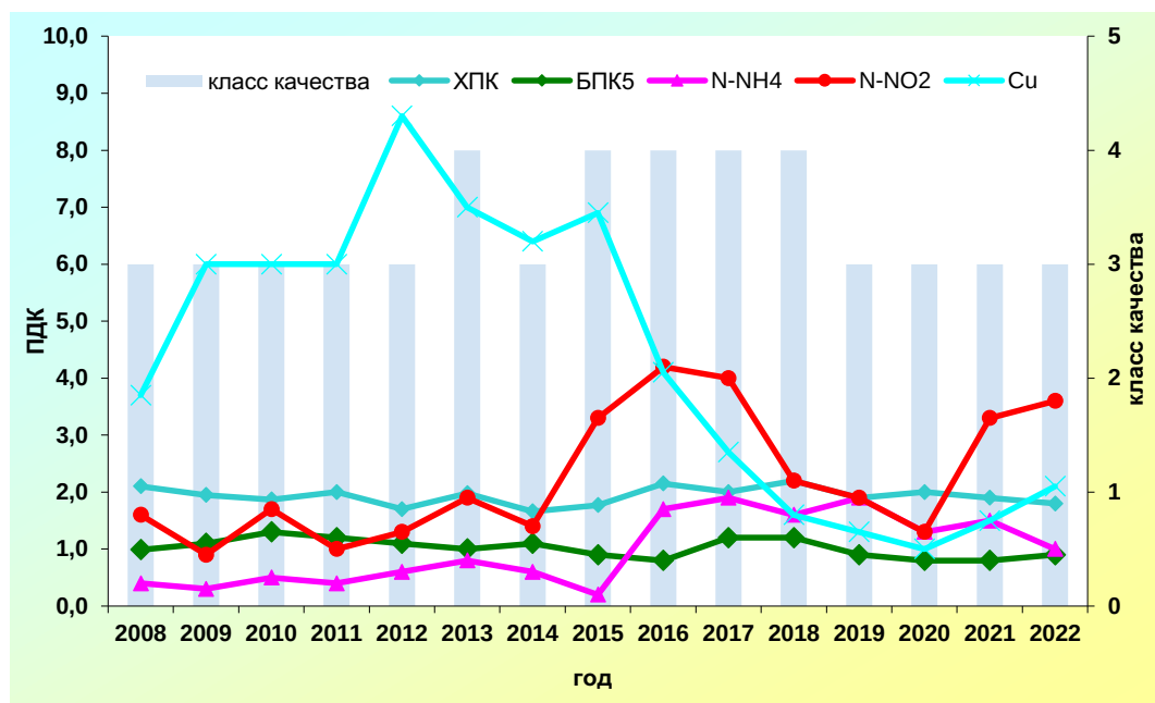
Рис. 3.34. Изменение среднегодовых концентраций отдельных загрязняющих веществ и показателей качества воды Чебоксарского водохранилища, 4,2 км ниже г. Нижний Новгород за многолетний период
