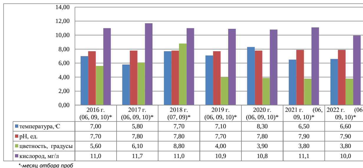
Рис. 4.15. Общая гидрохимическая характеристика воды в районе продольного разреза оз. Байкал
