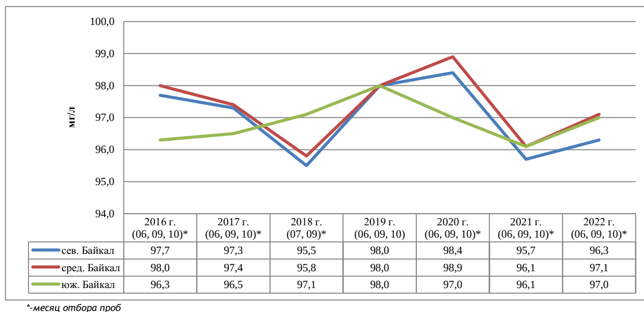
Рис. 4.16. Минерализация воды озера по котловинам продольного разреза
