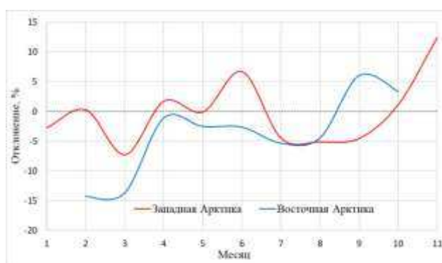
Рис. 4.37. Отклонения от нормы среднемесячных значений ОСО для восточного и западного секторов Арктики в 2022 г.
