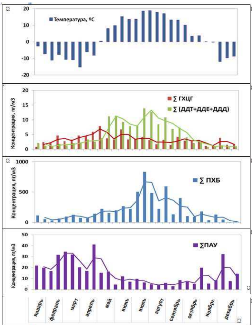
Рис. 4.22. Ход приземной температуры и концентраций ΣГХЦГ, ΣДДТ, ΣПХБ, ΣПАУ в г. Байкальске в 2022 г.
