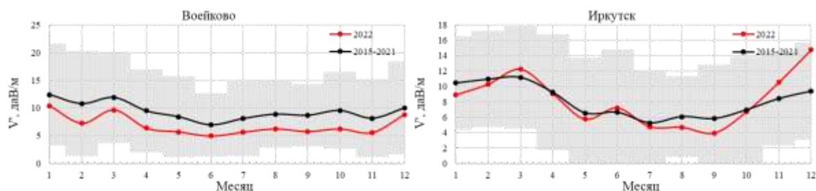
Рис. 2.9. Годовой ход V' по станциям Воейково, Иркутск в 2022 г. на фоне осредненного годового хода V' за период 2015-2021 гг.
