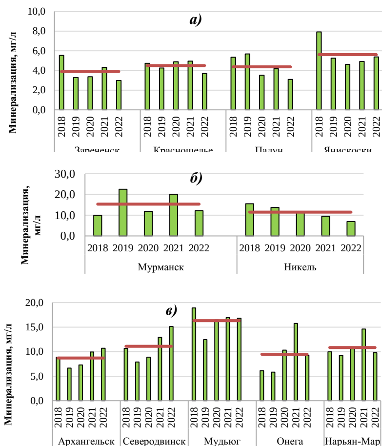
Рис. 4.40. Изменение средневзвешенной минерализации осадков на Европейской территории Арктики, 2018-2022 гг.
