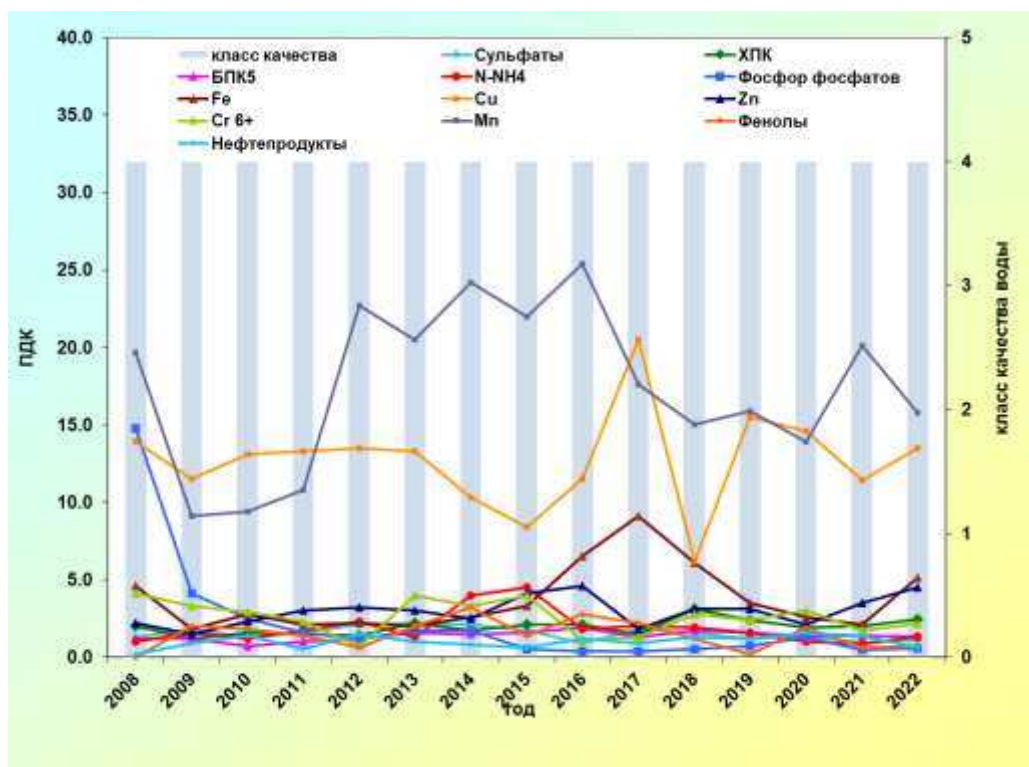
Рис 3.38. Изменение среднегодовых концентраций отдельных загрязняющих веществ и показателей качества воды р. Чусовая, 1,7 км ниже г. Первоуральск за многолетний период
