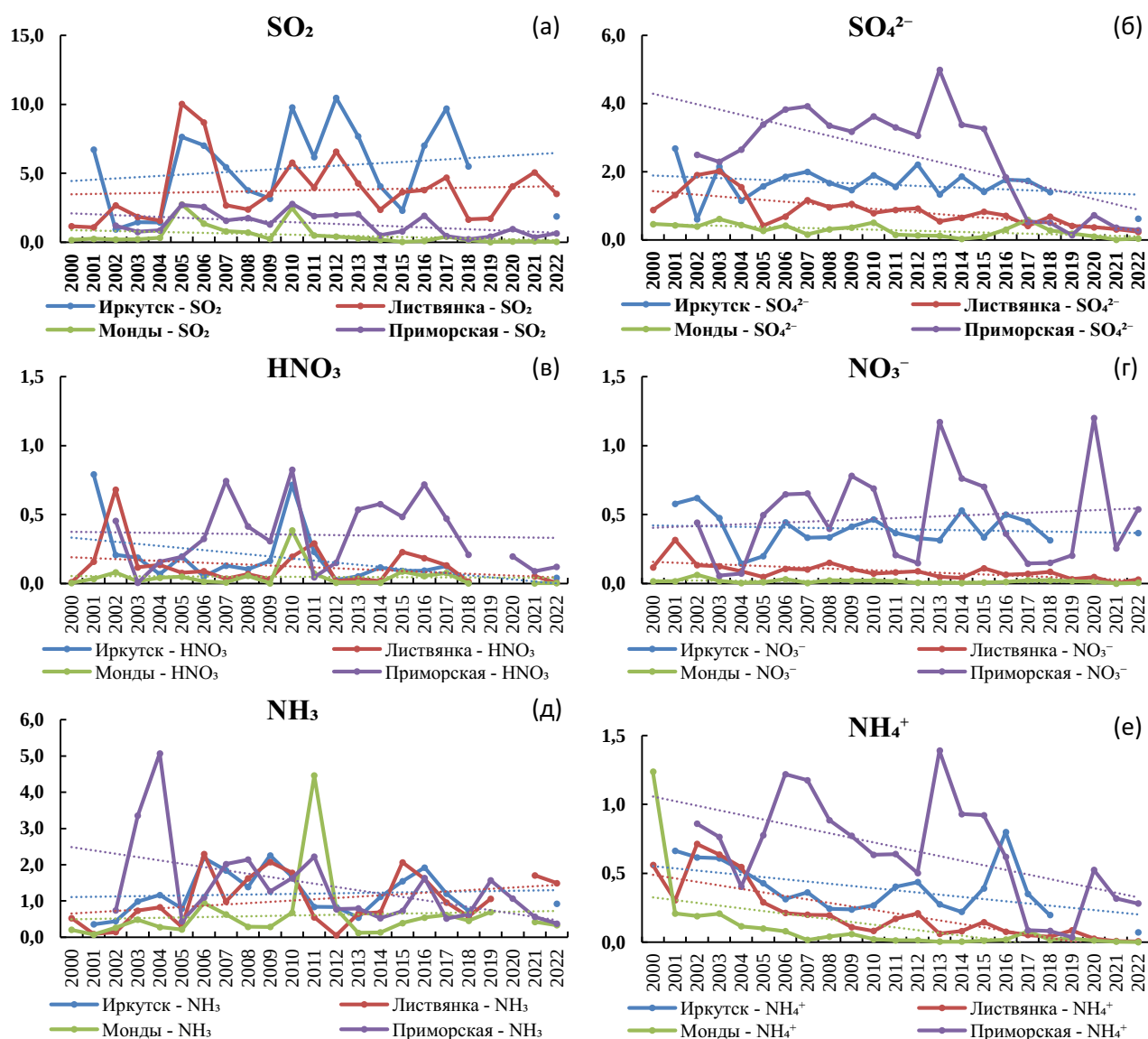
Рис. 2.38. Изменения средних годовых концентрации соединений серы (а, б) и азота (в, г, д, е) в атмосферном воздухе на станциях ЕАНЕТ ( \text{мкг м}^{-3} )
