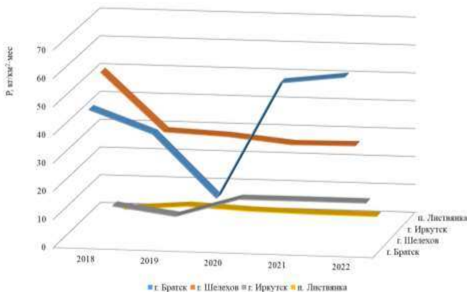
Рис. 3.25. Динамика среднегодовых значений плотностей атмосферных выпадений фторидов ( P , \text{кг}/\text{км}^2 \cdot \text{мес} ) в населенных пунктах Иркутской области
