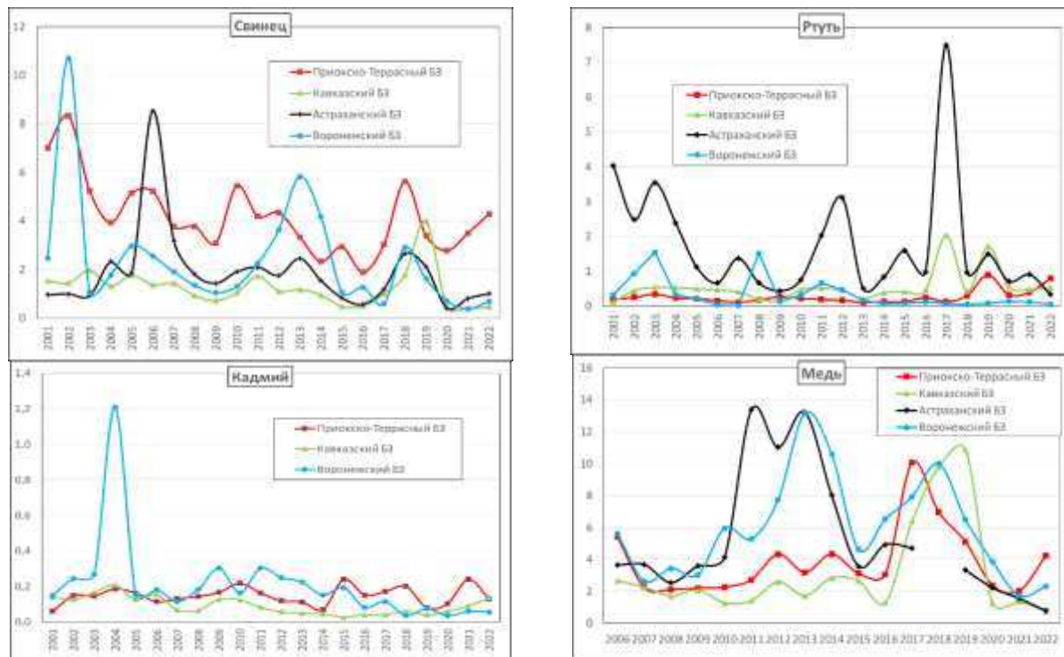
Рис. 2.35. Изменения среднего содержания тяжелых металлов в атмосферных осадках фоновых районов в 2001-2022 гг.
