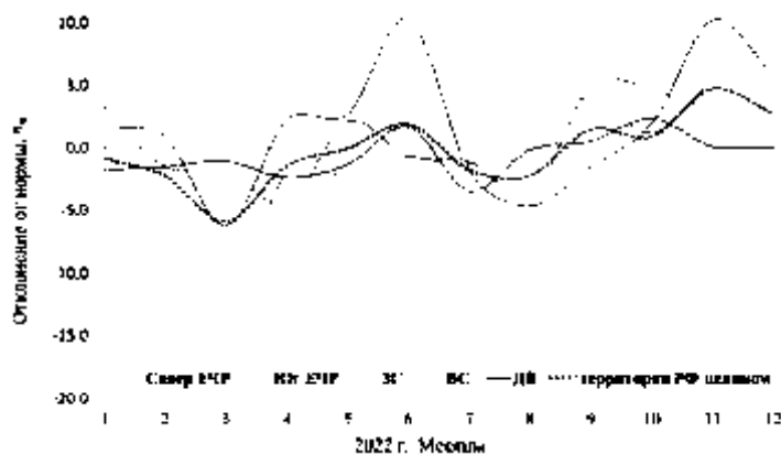
Рис. 2.16. Отклонения среднемесячных значений ОЗО от норм по регионам РФ в 2022 г. (Север ЕЧР - Север Европейской части России, Юг ЕЧР - Юг Европейской части России, ЗС - Западная Сибирь, ВС - Восточная Сибирь, ДВ - Дальний Восток)
