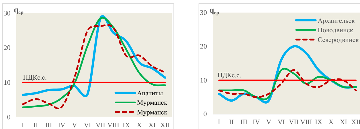
Рис. 4.48. Годовой ход концентраций формальдегида в городах АЗРФ в 2022 г., q_{\text{ср}} , мкг/м 3
