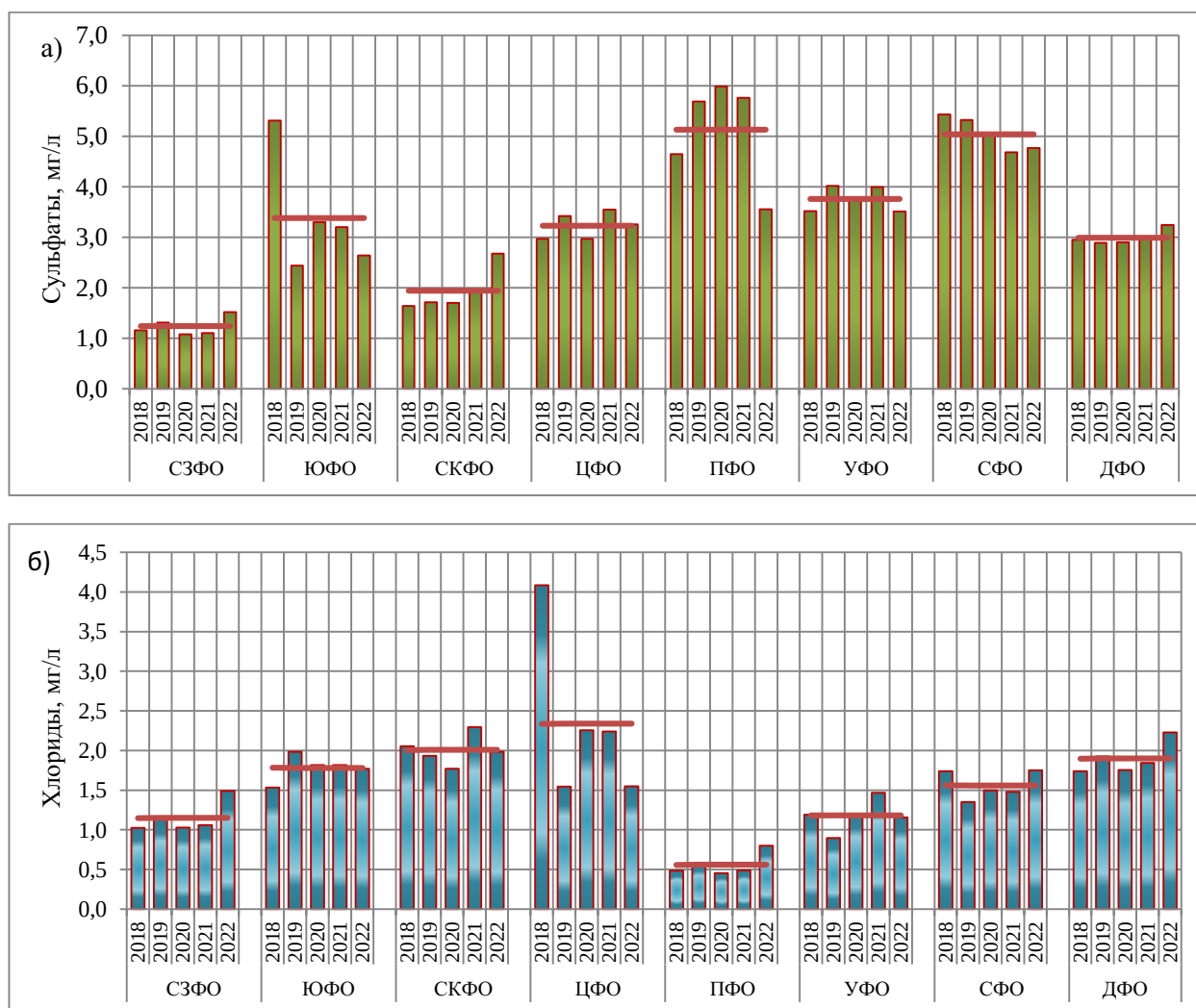
Рис. 2.29 (начало). Изменение средневзвешенной концентрации ионов (а - сульфатов, б - хлоридов, в - нитратов, г - гидрокарбонатов) в атмосферных осадках по федеральным округам, 2018-2022 гг.
