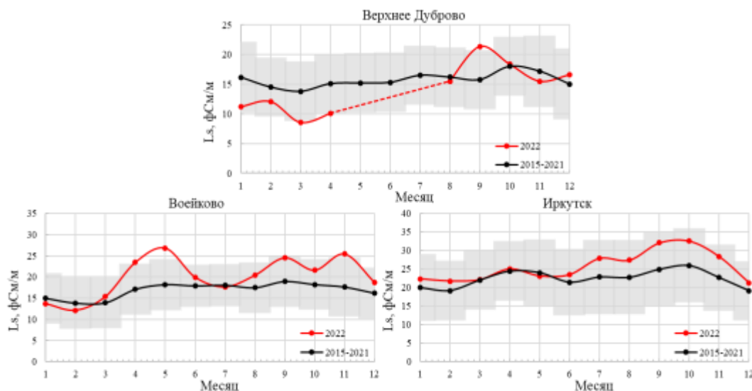
Рис. 2.10. Годовой ход L_s на станциях Верхнее Дуброво, Воейково, Иркутск в 2022 г. на фоне осредненного годового хода L_s за период 2015-2021 гг. Цветным фоном обозначены границы стандартного отклонения \pm\sigma от среднего значения за 2015-2021 гг.
