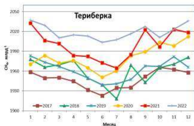
Рис. 2.2. Сезонный ход концентрации \text{CH}_4 на станции Териберка
