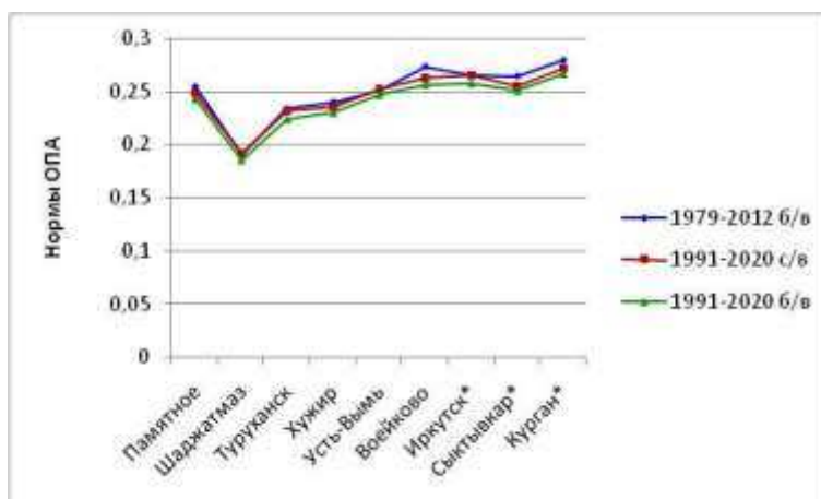
Рис. 2.6. 30-летние нормы ОПА, рассчитанные для каждой станции фоновой мониторинга за 1979-2012 гг. (без учета 1983-1984 гг.) и 1992-1993 гг. (6/в); за 1991-2020 гг. (полностью (с/в) и за 1991-2020 гг. (без учета 1983-1984 гг.) и 1992-1993 гг. (6/в)
