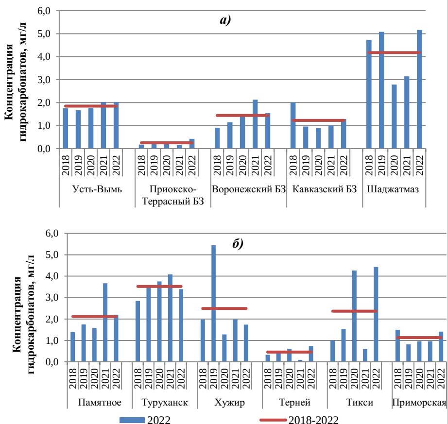
Рис. 2.19. Изменение средневзвешенной концентрации гидрокарбонатов в осадках фоновых станций ЕЧР (а) и АЧР (б), 2018-2022 гг.
