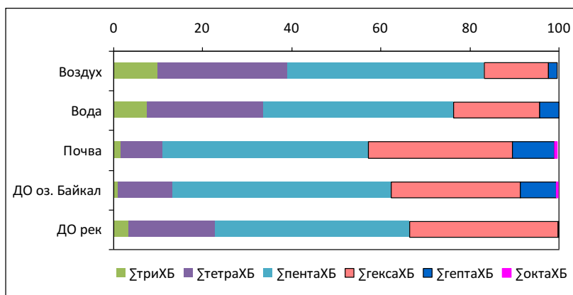
Рис. 4.21. Конгенерный состав ПХБ в пробах окружающей среды
