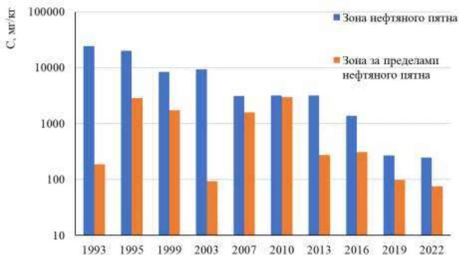
Рис. 3.26. Многолетняя динамика изменений содержания нефтепродуктов в почвах п. Тыреть Заларинского района Иркутской области
