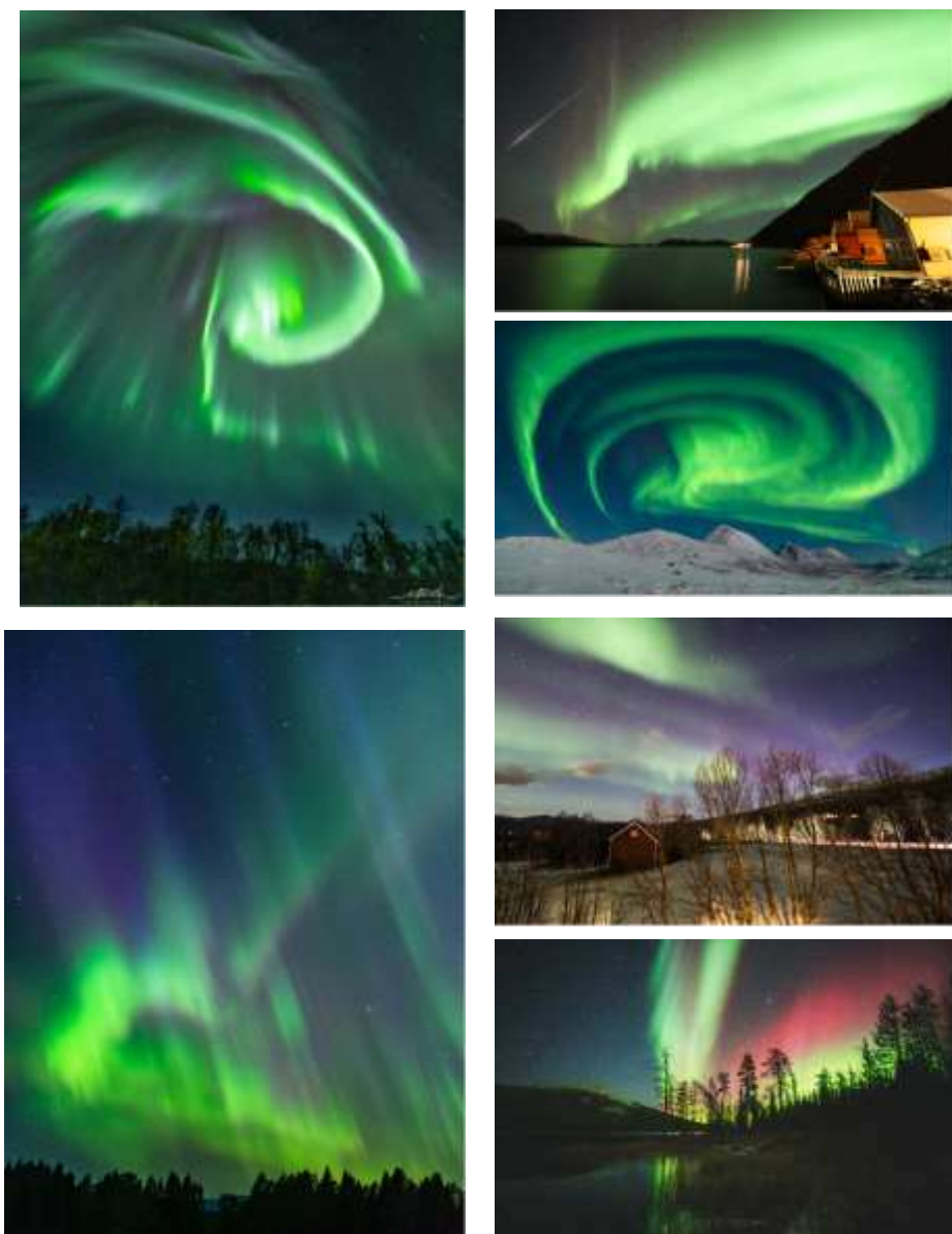
Рис. 1.4. Примеры наблюдения полярных сияний в разных регионах арктической зоны в период с сентября по ноябрь 2022 г.
