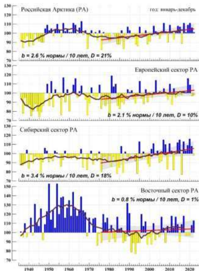
Рис. 4.33. Годовые (январь-декабрь) суммы осадков (% нормы) в Российской Арктике и ее секторах в 1936-2022 гг. Жирная темная кривая - 11летнее скользящее среднее. Показан линейный тренд за 1976-2022 гг.
