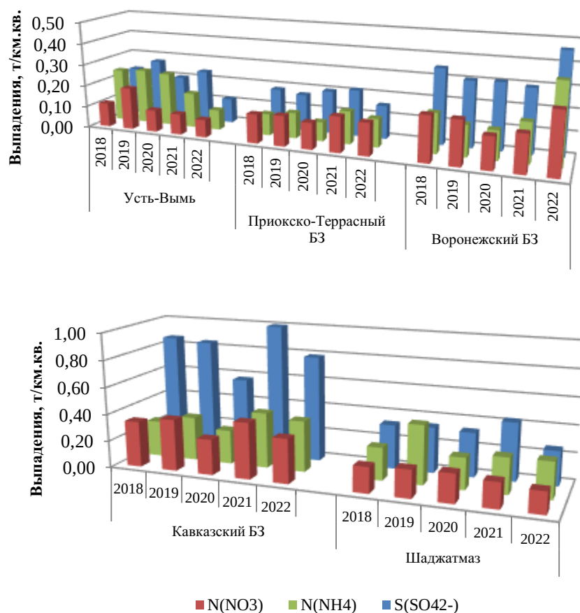
Рис. 2.25. Выпадения серы (S), азота нитратного (N(NO 3 )) и азота аммонийного (N(NH 4 )) с атмосферными осадками на станциях ЕЧР в период с 2018 по 2022 гг.
