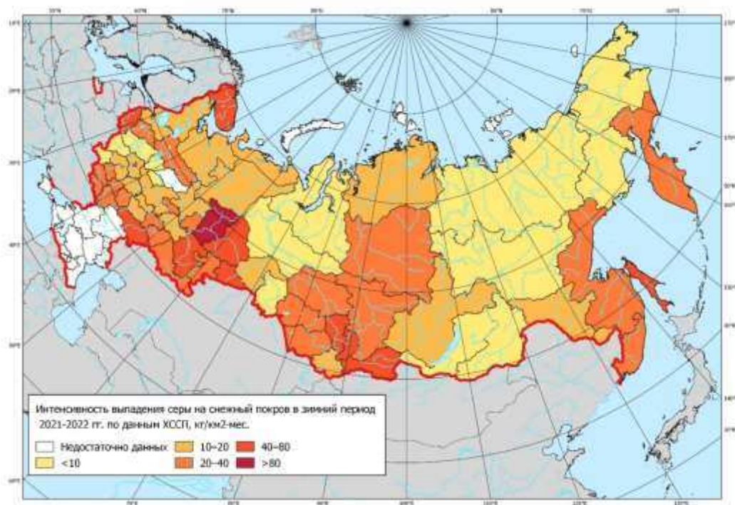
Рис. 2.32. Интенсивность выпадения серы на снежный покров в зимний период 2021-2022 гг.
