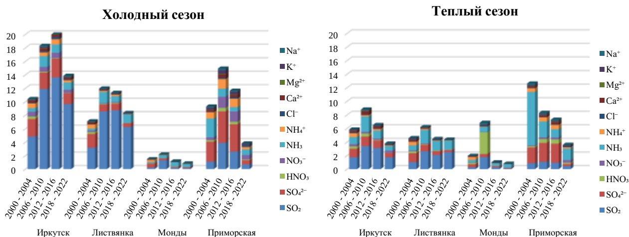
Рис. 2.39. Изменение средних пятилетних значений содержания кислотообразующих веществ в общем составе аэрозолей и газов ( \text{мкг м}^{-3} ) на станциях ЕАНЕТ в холодный (слева) и теплый (справа) периоды в 2000-2022 гг.
