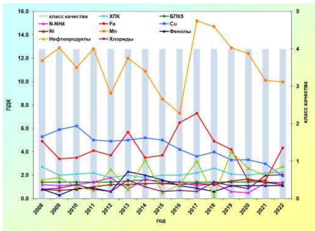
Рис 3.39. Изменение среднегодовых концентраций отдельных загрязняющих веществ и показателей качества воды р. Белая, 10,5 км ниже г. Sterlitamak за многолетний период
