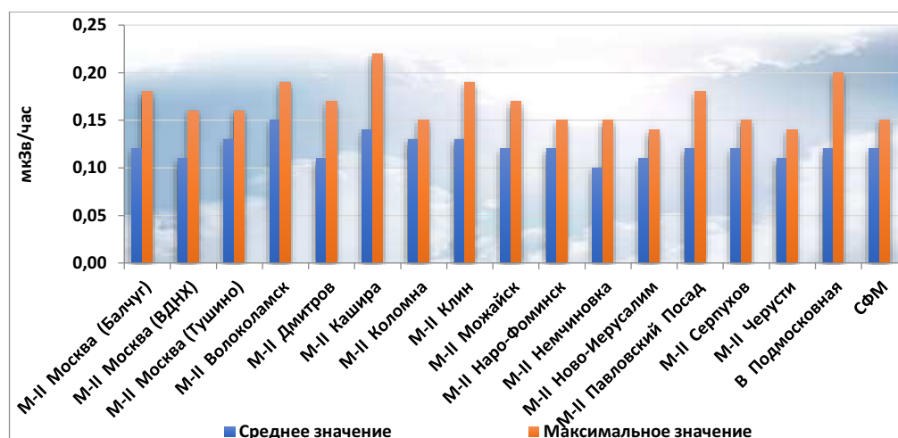
Рис. 4.8. Мощность амбиентного эквивалента дозы гамма-излучения (МАЭД) в 2022 г.
