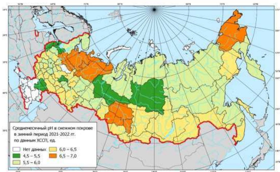
Рис. 2.34. pH снежного покрова в зимний период 2021-2022 гг.
