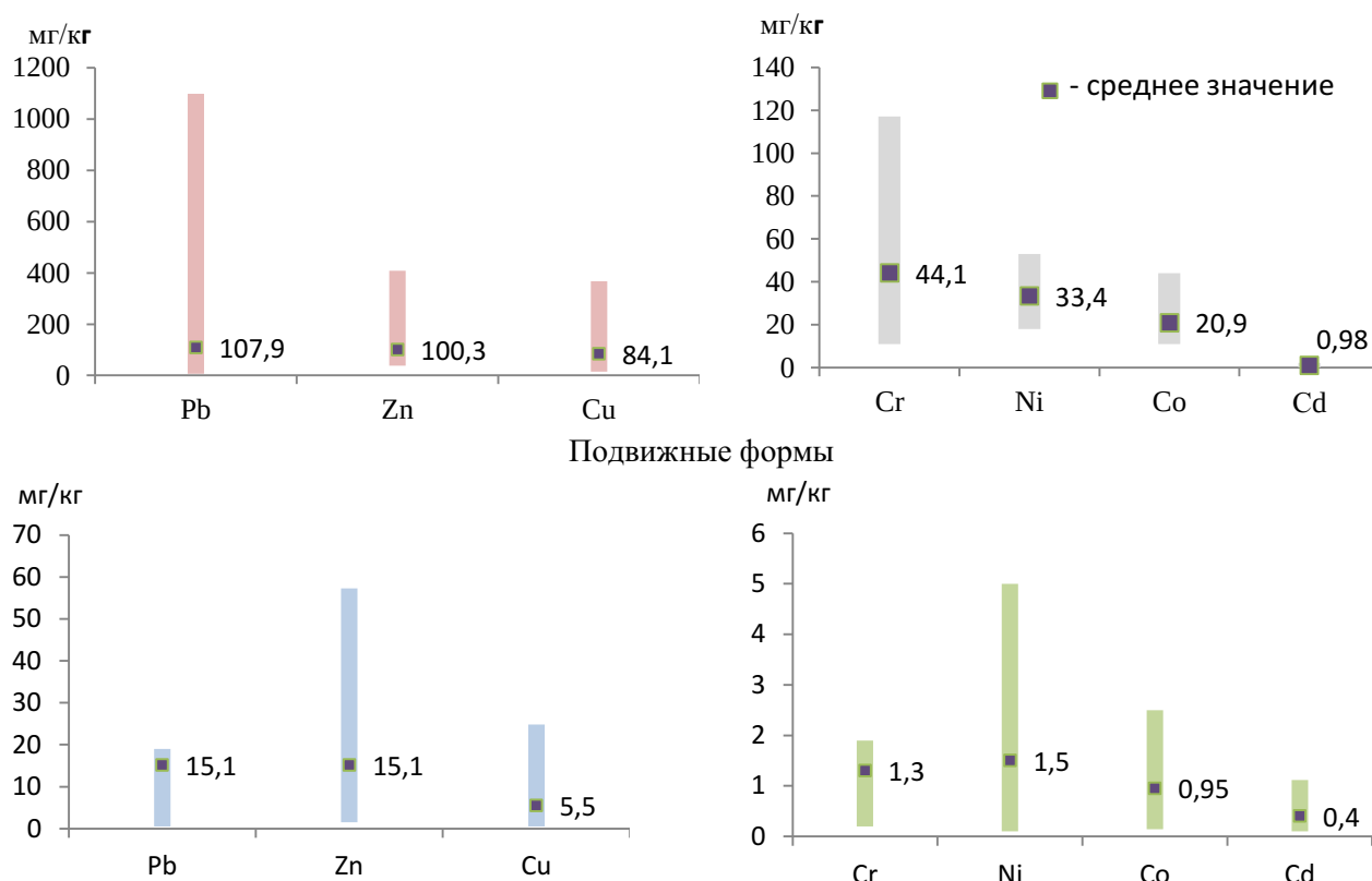
Рис. 2.42. Диапазон варьирования и среднее содержание кислоторастворимых и подвижных форм металлов в почве фонового участка п. Мариинск (Свердловская область) по данным наблюдений 1999-2022 г.
