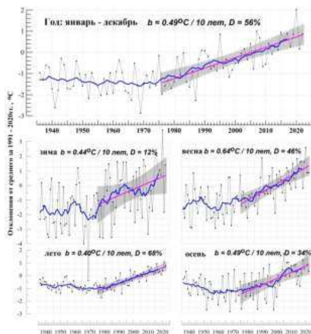
Рис. 1.8. Средние годовые (вверху) и сезонные аномалии температуры приземного воздуха (°C), осредненные по территории РФ, 1936-2022 гг.
