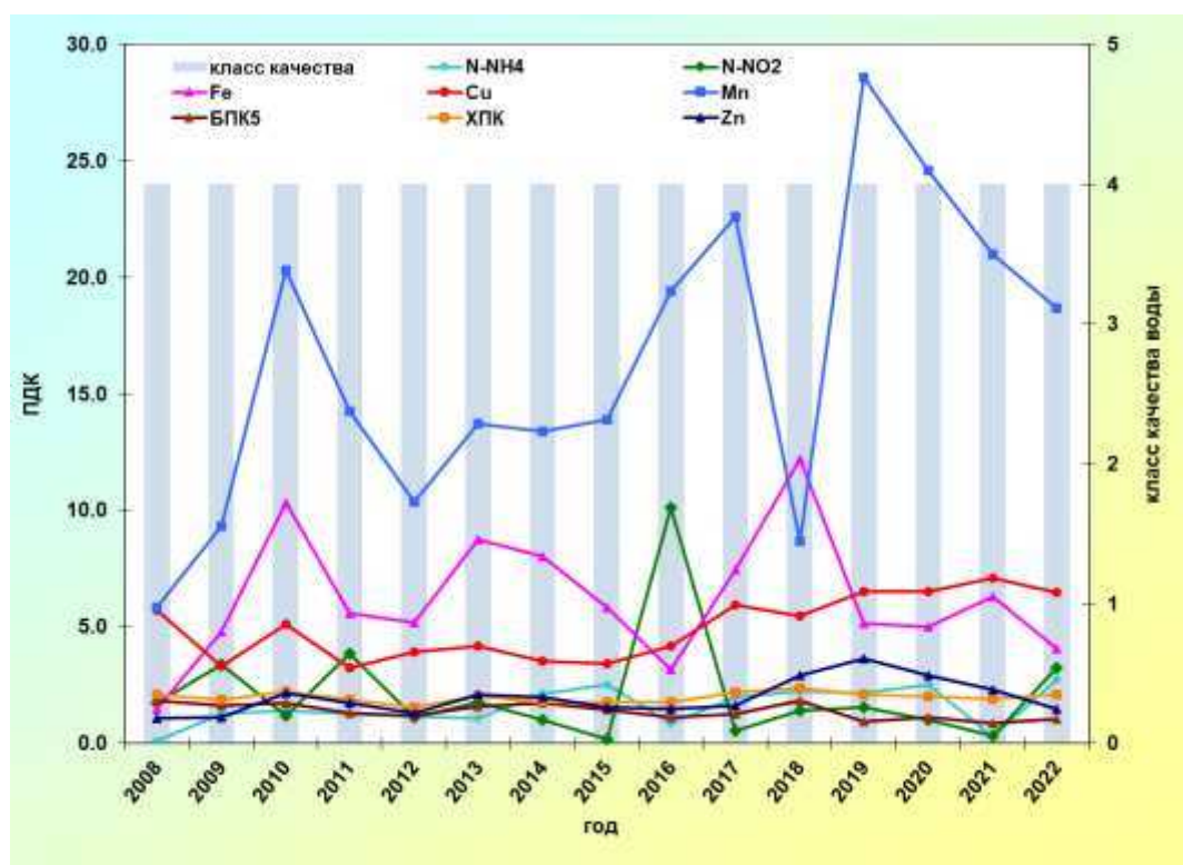
Рис. 3.30. Изменение среднегодовых концентраций отдельных загрязняющих веществ и показателей качества воды р. Охта, 0,05 км выше устья, в черте г. Санкт-Петербург, в многолетнем плане
