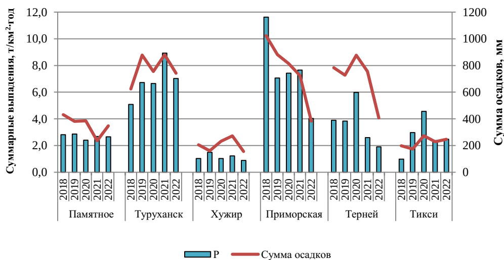
Рис. 2.24. Суммарные влажные выпадения на АЧР, 2018-2022 гг.
