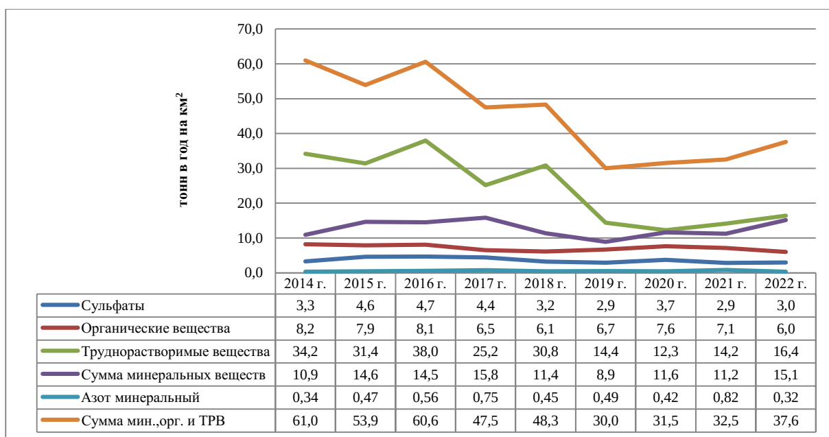
Рис. 4.13. Поступление веществ из атмосферы на ст. Большое Голоустное
