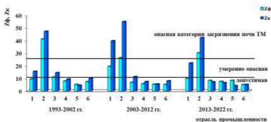
Рис. 3.21. Динамика средних по отраслям промышленности усреднённых за несколько лет показателей загрязнения почв комплексом ТМ Z_f и Z_k вокруг предприятий черной металлургии (1), цветной металлургии (2), машиностроения и металлообработки (3), топливной и энергетической промышленности (4), химической и нефтехимической промышленности (5), строительной промышленности и производства строительных материалов (6), усреднённых за несколько лет
