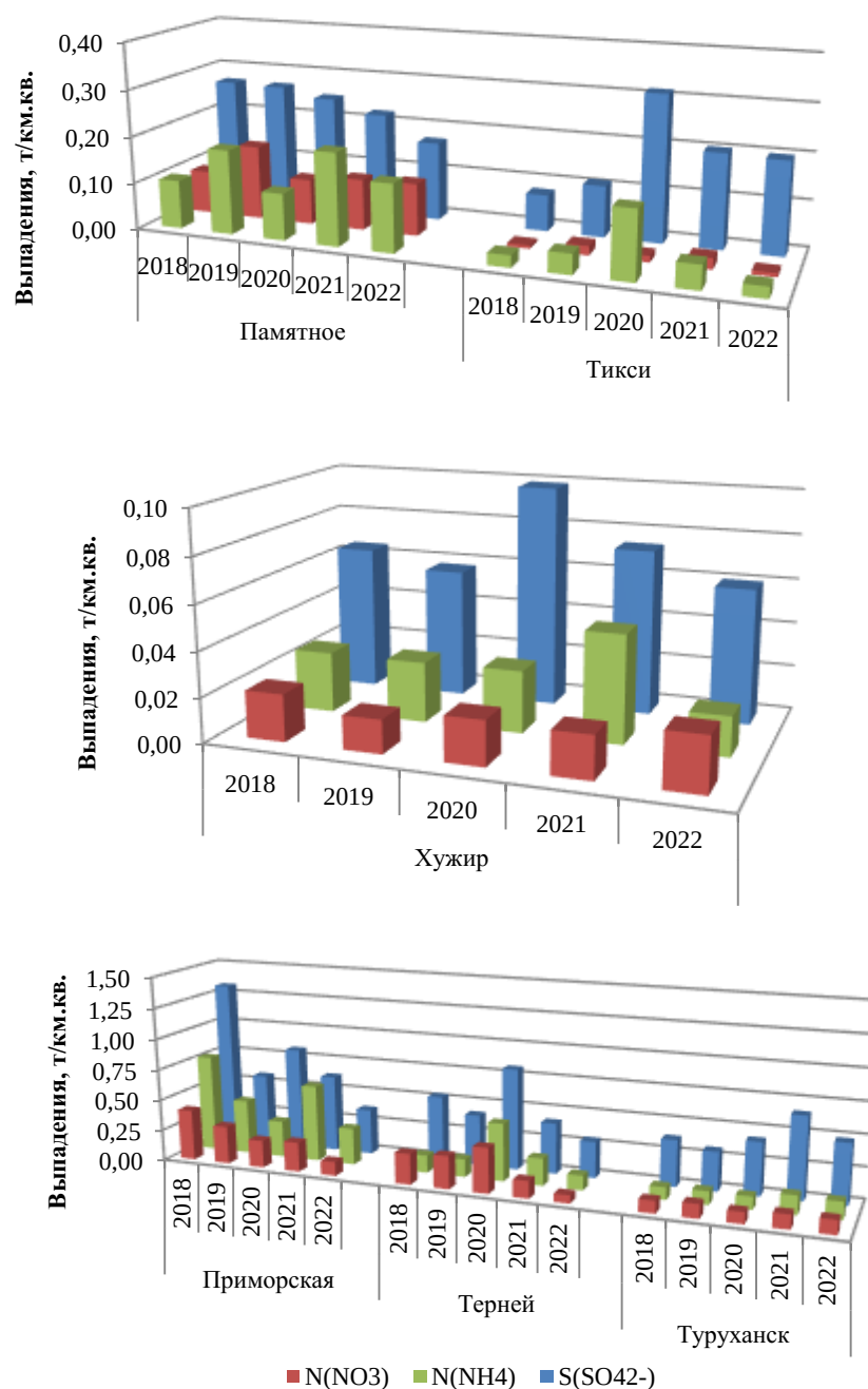
Рис. 2.26. Выпадения серы (S), азота нитратного (N(NO 3 )) и азота аммонийного (N(NH 4 )) с атмосферными осадками на станциях АЧР в период с 2018 по 2022 гг.
