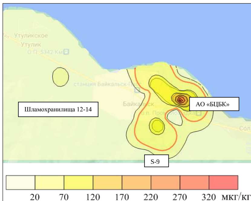
Рис. 4.26. Изолинии концентраций бенз(а)пирена в почве
