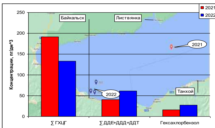
Рис. 4.23. Среднее содержание хлорорганических пестицидов в воде Южной котловины оз. Байкал
