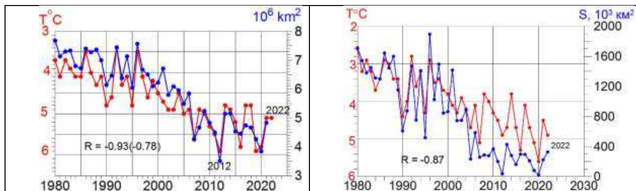
Рис. 4.36. Площадь, занятая морским льдом в сентябре и температура воздуха летом в Северном Ледовитом океане (слева) и в морях СМП в сентябре (справа)
