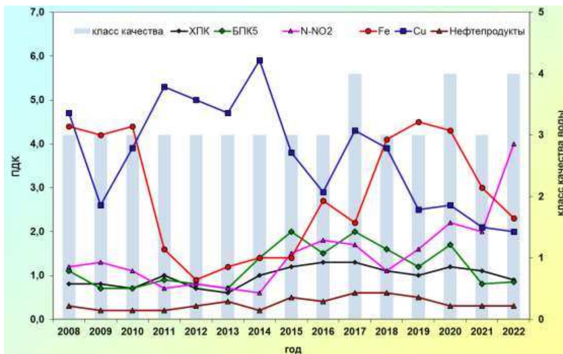
Рис. 3.41. Изменение среднегодовых концентраций загрязняющих веществ и показателей качества воды р. Кубань, 24,5 км ниже г. Краснодар за многолетний период
