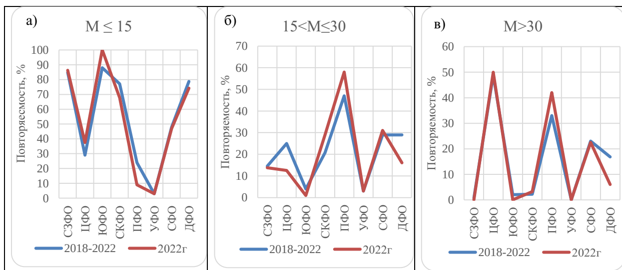
Рис. 2.28. Повторяемость (%) минерализации осадков (M) по диапазонам в период 2018-2022 гг. и в 2022 г.
