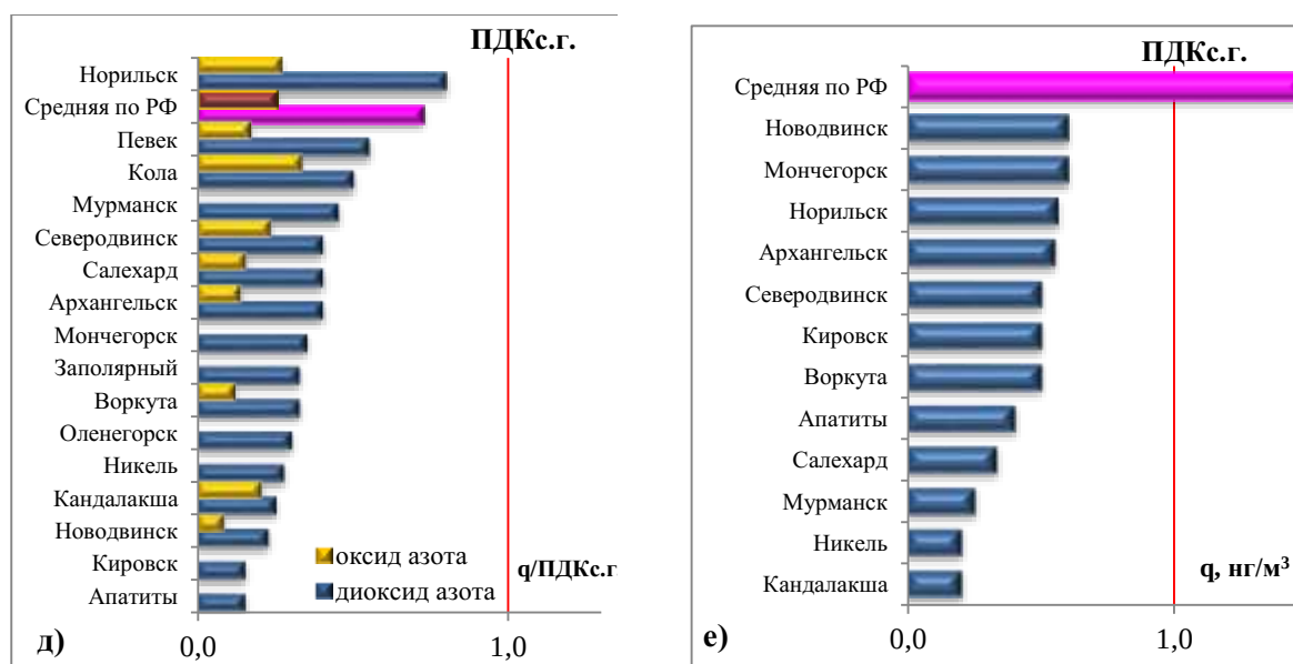
Рис. 4.47. Средние за год концентрации: взвешенных веществ (а), диоксида серы (б), оксида углерода (в), q , \text{мг}/\text{м}^3 , формальдегида (г), диоксида и оксида азота (д), q , ПДКс.г., бенз(а)пирена (е), q , \text{нг}/\text{м}^3 , в городах АЗРФ и в целом по России в 2022 г.
