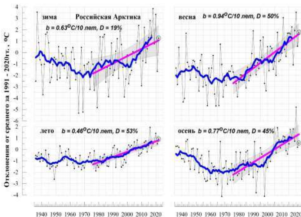
Рис. 4.31. Сезонные аномалии температуры воздуха в Российской Арктике в 1936-2022 гг. Жирная синяя кривая - 11-летнее скользящее среднее. Показан линейный тренд за 1976-2022 гг. с 95%-й доверительной полосой
