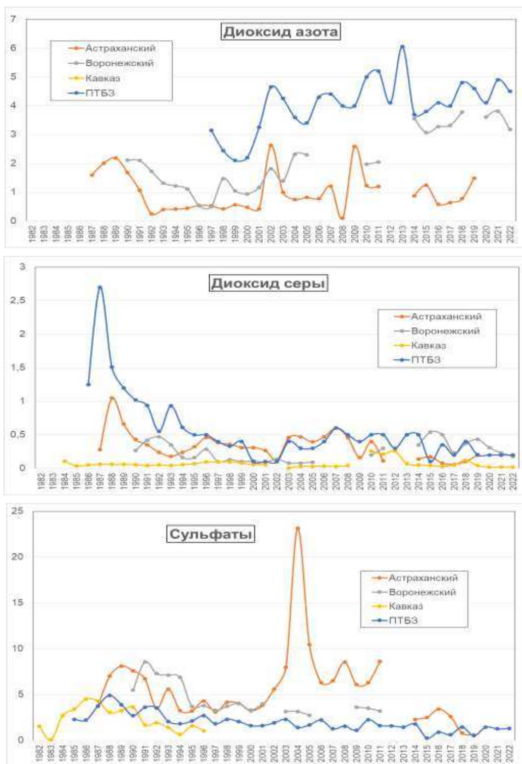
Рис. 2.18. Изменения среднегодового содержания диоксида серы, сульфатов и диоксида азота в атмосферном воздухе фоновых районов ( \text{мкг}/\text{м}^3 )
