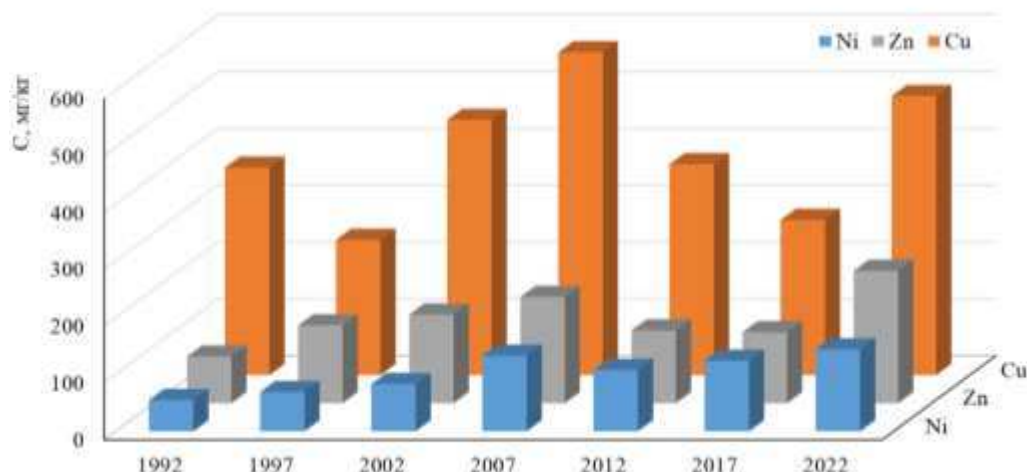
Рис. 3.24. Содержание некоторых тяжелых металлов в почвах г. Верхняя Пышма Свердловской области (0–10 км от АО «Уралэлектромедь»)
