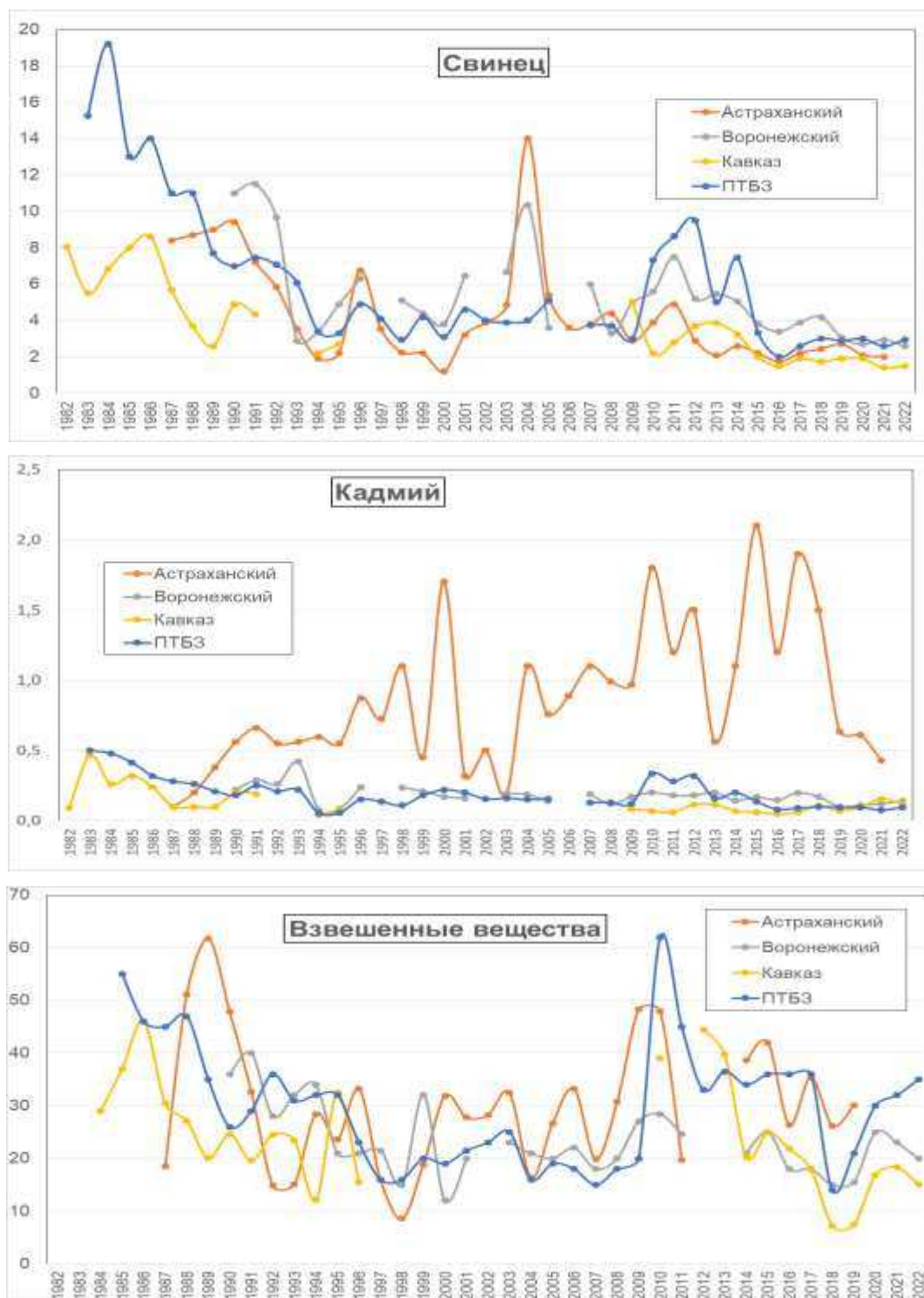
Рис. 2.17. Изменения среднегодового содержания свинца, кадмия ( \text{нг}/\text{м}^3 ), взвешенных веществ и ( \text{мкг}/\text{м}^3 ) в атмосферном воздухе фоновых районов
