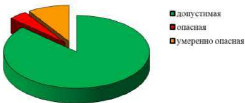
Рис. 3.23. Доля обследованных в 2013-2022 гг. населенных пунктов, почвы которых относятся к разным категориям загрязнения
