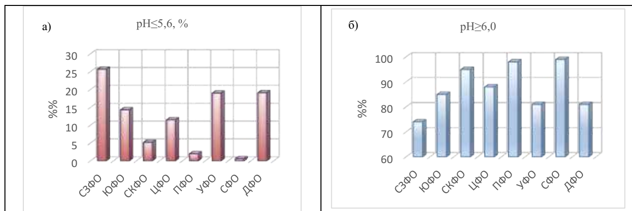
Рис. 2.30. Повторяемость величины pH в атмосферных осадках ФО: а) pH≤5,6 ед. pH, %; б) pH≥6,0 ед. pH, %
