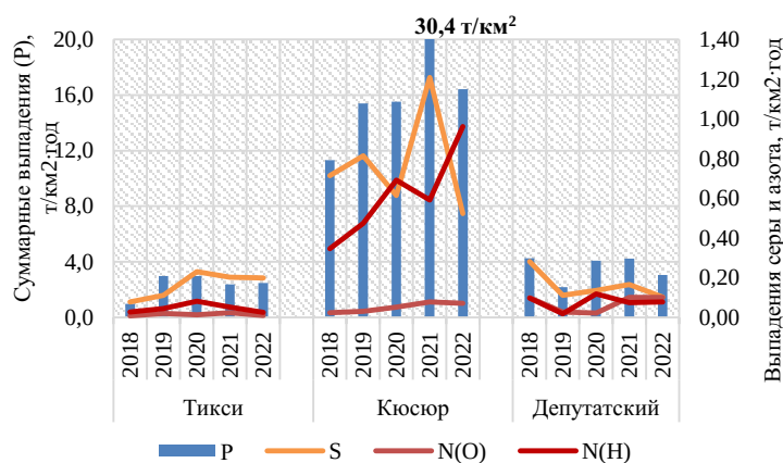
Рис. 4.46. Межгодовой ход суммарных влажных выпадений (P) и выпадений серы (S), нитратного (N(O)) и аммиачного (N(H)) азота в Республике Саха (Якутия)
