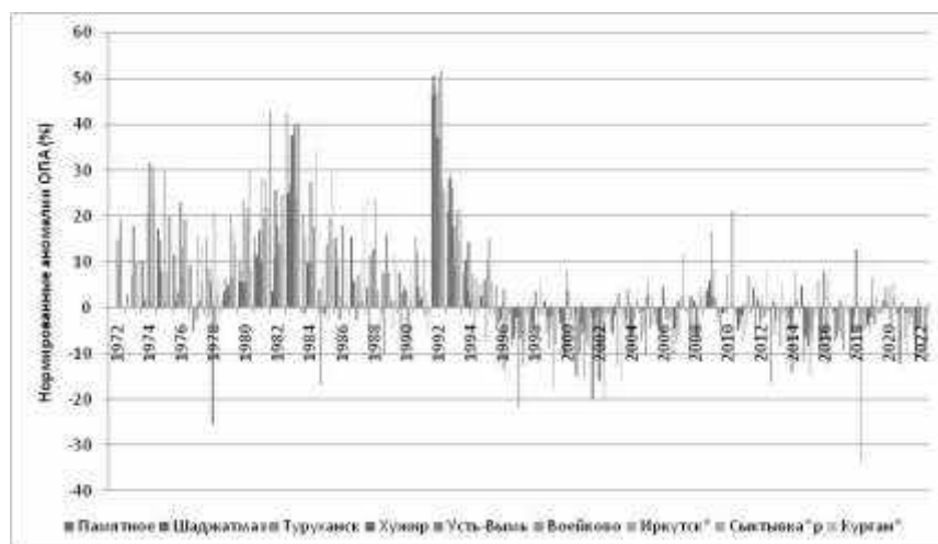
Рис. 2.8. Нормированные аномалии ОПА(%) на станциях фоновой мониторинга
