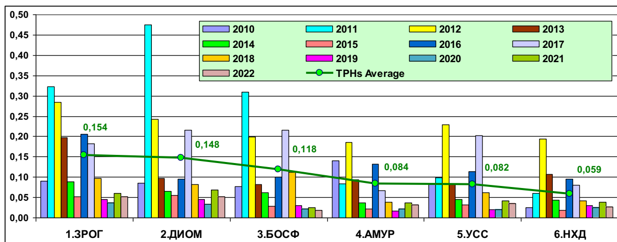
Рис. 3.64. Межгодовые изменения среднегодовой концентрации нефтяных углеводородов (мг/дм 3 ) в водах залива Петра Великого Японского моря: 1. ЗРОГ — бухта Золотой Рог, 2. ДИОМ — бухта Диомид, 3. БОСФ — пролив Босфор Восточный, 4. АМУР — Амурский залив, 5. УСС — Уссурийский залив, 6. НХД — залив Находка.
