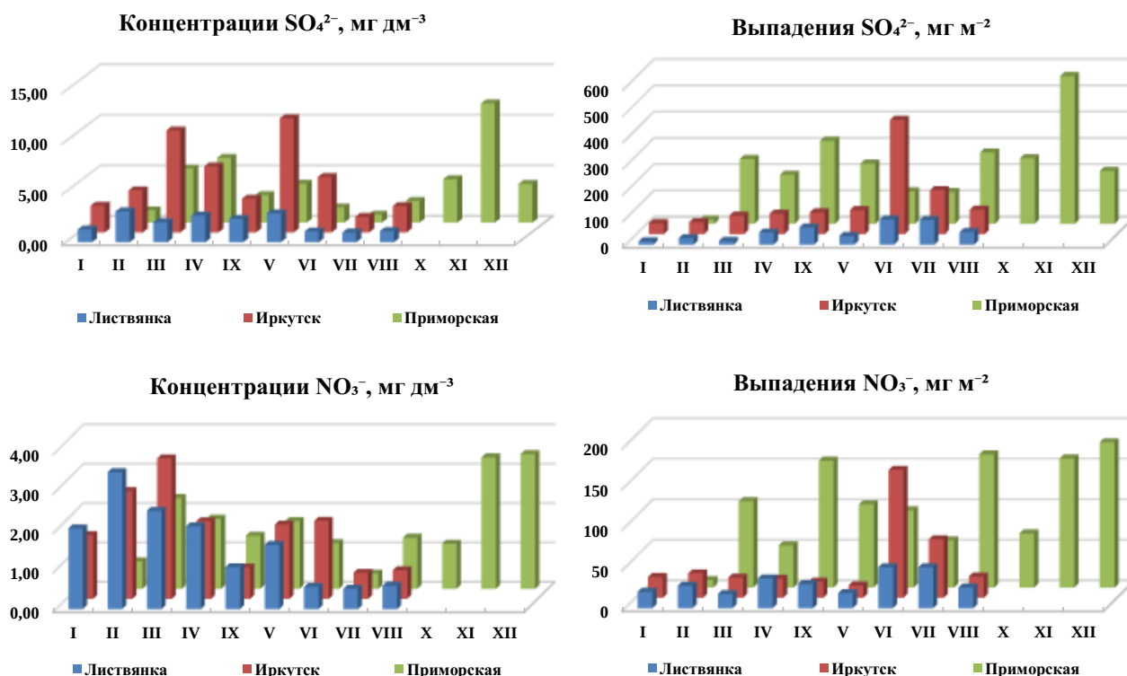
Рис. 2.40 (начало). Годовой ход концентраций (слева) и выпадений (справа) основных кислотообразующих ионов с осадками на станциях ЕАНЕТ в 2022 г.
