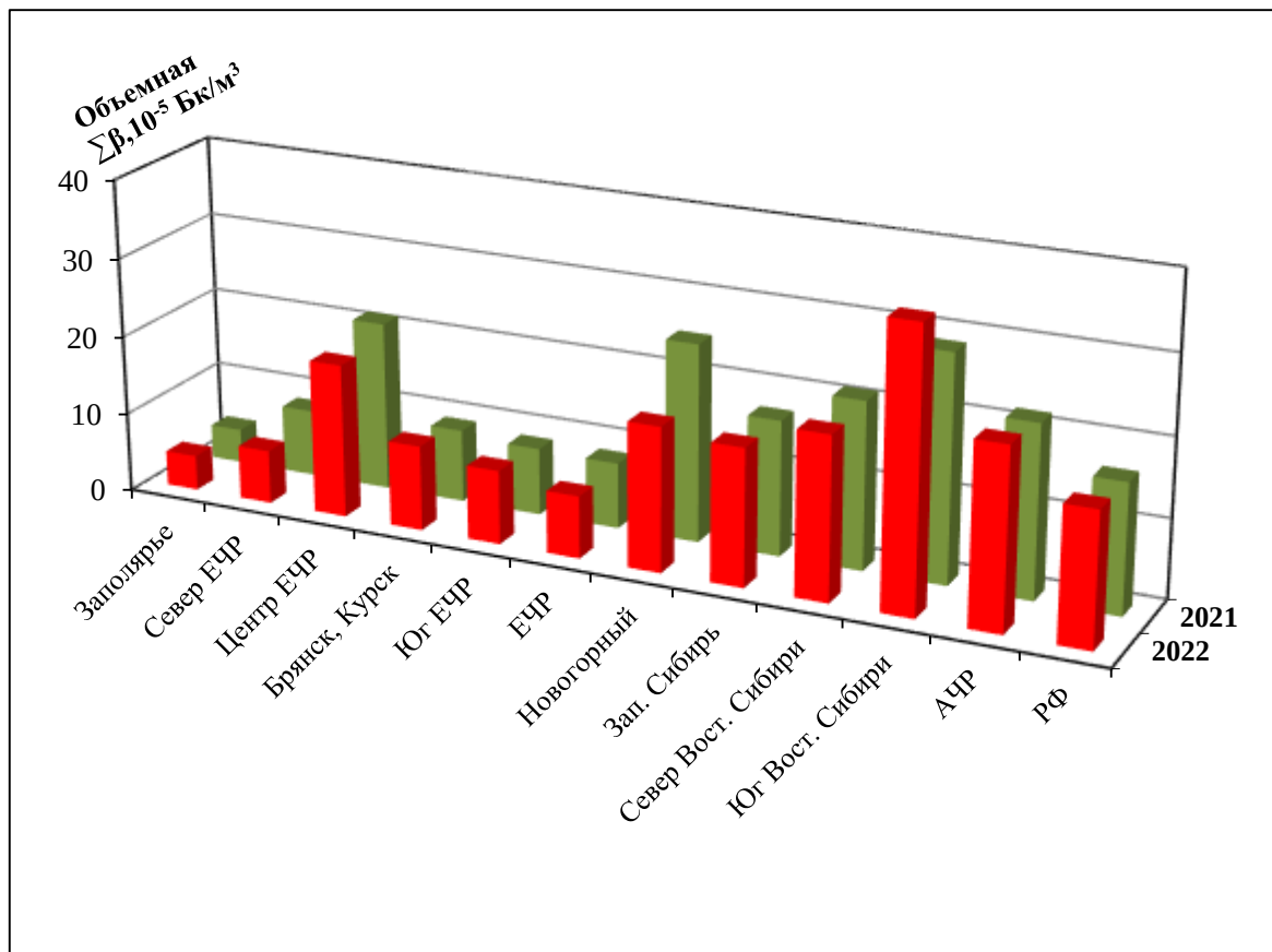
Рис. 2.43. Средние значения объемной \Sigma B в приземном слое атмосферы на территории РФ в 2021-2022 гг., 10^{-5} Бк/м 3
