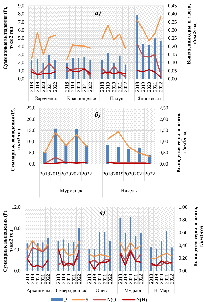
Рис. 4.44. Межгодовой ход суммарных влажных выпадений (P) и выпадений серы (S), нитратного (N(O)) и аммиачного (N(H)) азота на территориях Мурманской обл. (а,б), Архангельской обл. и Ненецкого АО (в)
