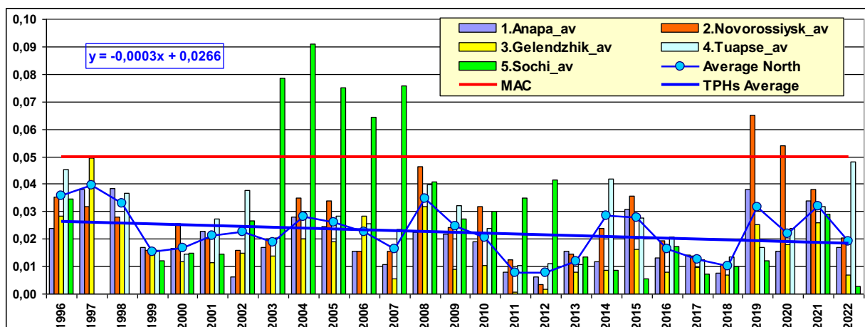
Рис. 3.57. Динамика средней концентрации нефтяных углеводородов (мг/дм³) в прибрежных водах Кавказа в 1996-2022 гг. Сокращения: Average North - средняя величина в северной части Кавказского побережья; ПДК - предельно допустимая концентрация (ПДК); Trend Average North - тренд концентрации НУ в северной части побережья.
