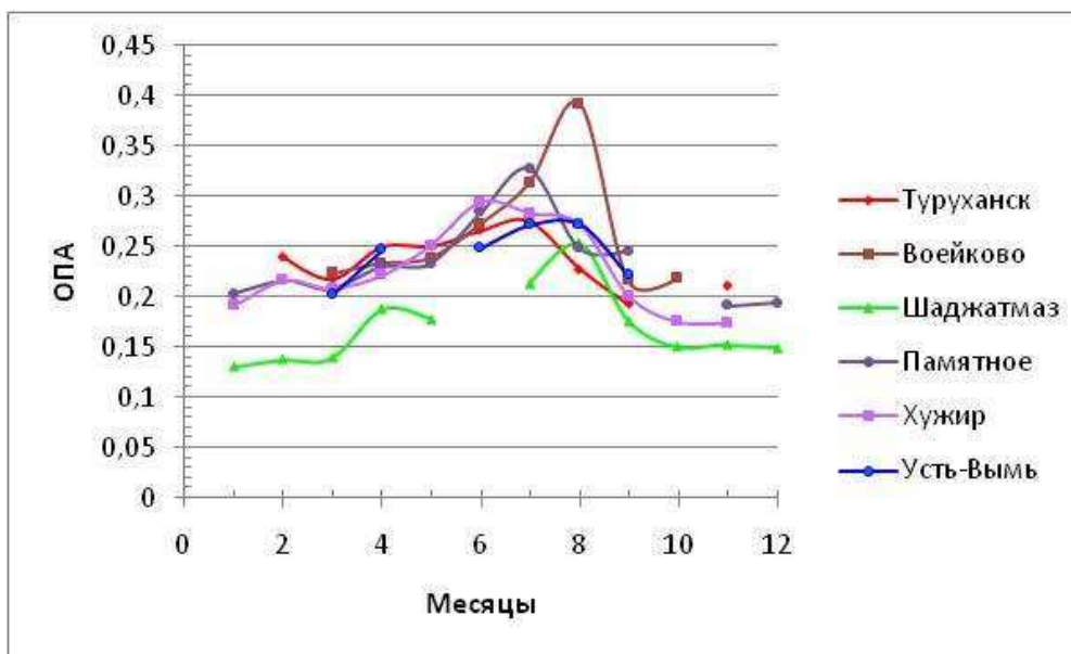
Рис. 2.5. Годовой ход ОПА в 2022 г. на региональных станциях фоновых мониторинга
