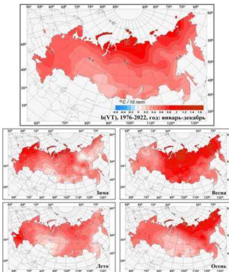
Рис. 1.10. Распределение коэффициентов линейного тренда среднегодовой и средних сезонных значений температуры приземного воздуха на территории России за период 1976-2022 гг. (в ^{\circ}\text{C}/10 лет)
