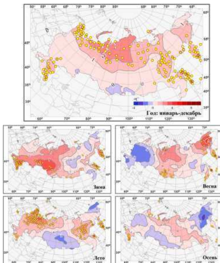
Рис. 1.9. Аномалии средней годовой и сезонных температур приземного воздуха на территории России в 2022 г. (отклонения от средних за 1991-2020 гг.) с указанием локализации экстремальных аномалий. Кружками белого и желтого цвета показаны станции, на которых наблюденная температура оказалась ниже 5-го или выше 95-го перцентилля, рассчитанного за 1936-2021 гг.
