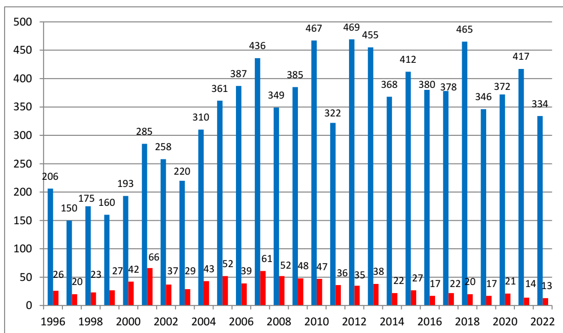
Рис. 1.6. Распределение гидрометеорологических ОЯ по годам: общее количество (синий) и количество непредусмотренных ОЯ (красный)
