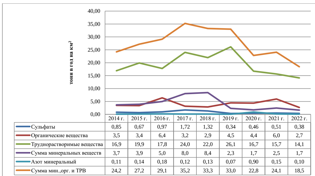
Рис. 4.14. Поступление веществ из атмосферы на ст. Хужир
