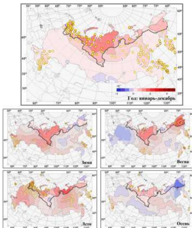
Рис. 4.29. Годовые (январь-декабрь) и сезонные аномалии температуры воздуха в Российской Арктике Аномалии (°C) рассчитаны относительно норм периода 1991-2020 гг. Желтыми кружками показаны аномалии выше 95-го перцентиля.
