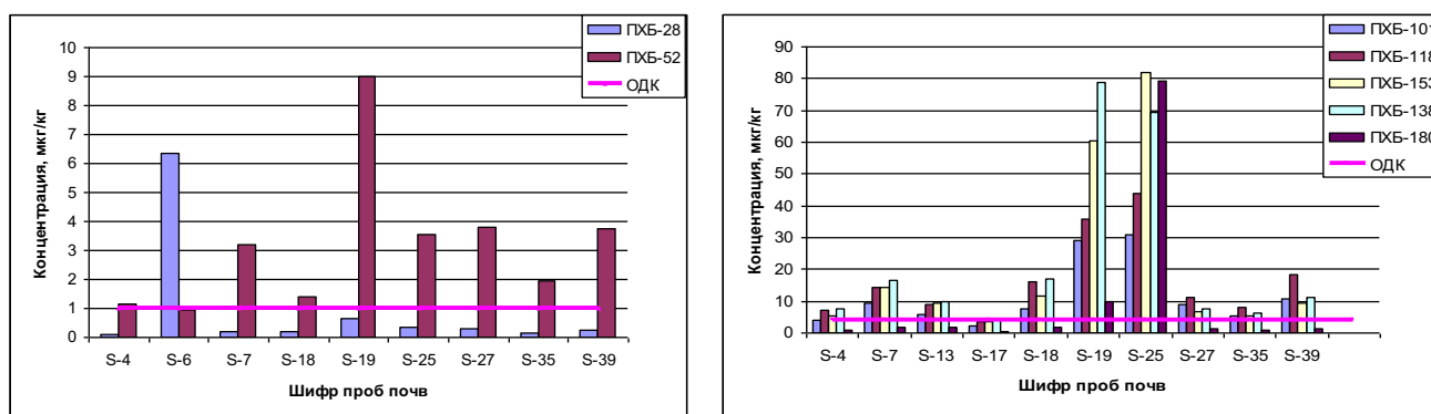
Рис. 4.24. Концентрации индивидуальных нормируемых ПХБ, выявленные в наиболее загрязненных пробах почв
