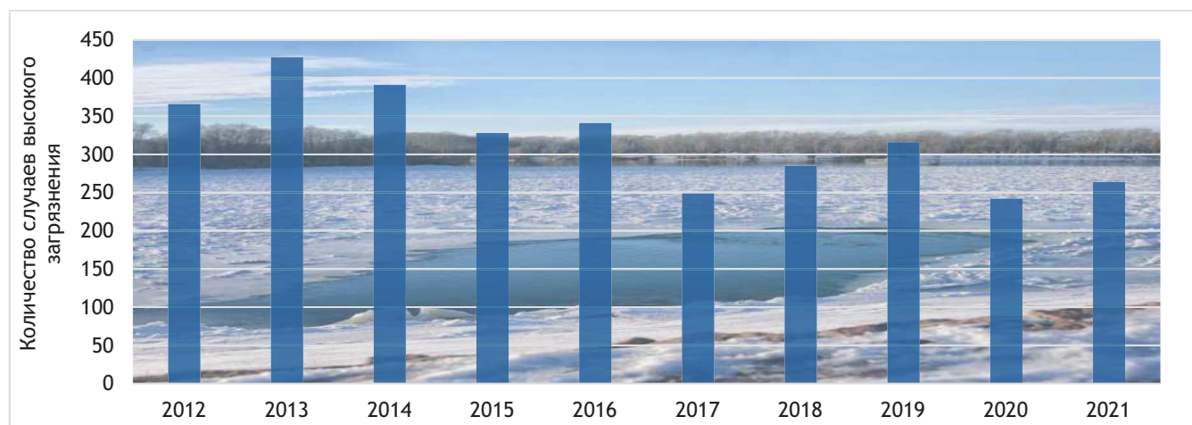
Рис. 4.4. Количество случаев высокого загрязнения воды водотоков Московского региона
