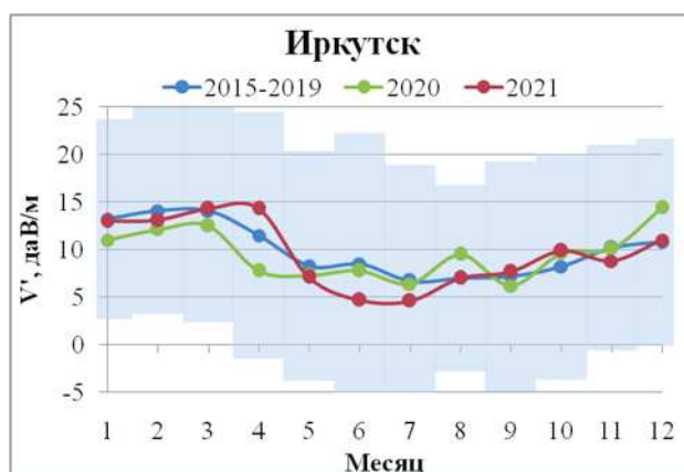
Рис. 2.8. Годовой ход V' по станциям Воейково, Иркутск в 2021 г. в сравнении с 2020 г. и на фоне осредненного годового хода V' за период 2015-2019 гг.
