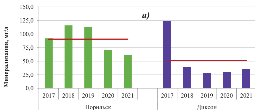
Рис. 4.40 (начало). Изменение средневзвешенной минерализации осадков на территории Красноярского края (а, б) и Ямало-Ненецкого АО (в), 2017-2021 гг.
