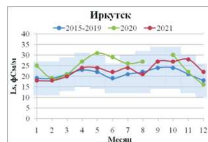
Рис. 2.9. Годовой ход L s на станциях Верхнее Дуброво, Воейково, Иркутск в 2021 г. в сравнении с 2020 г. и на фоне осредненного годового хода L s за период 2015-2019 гг.
