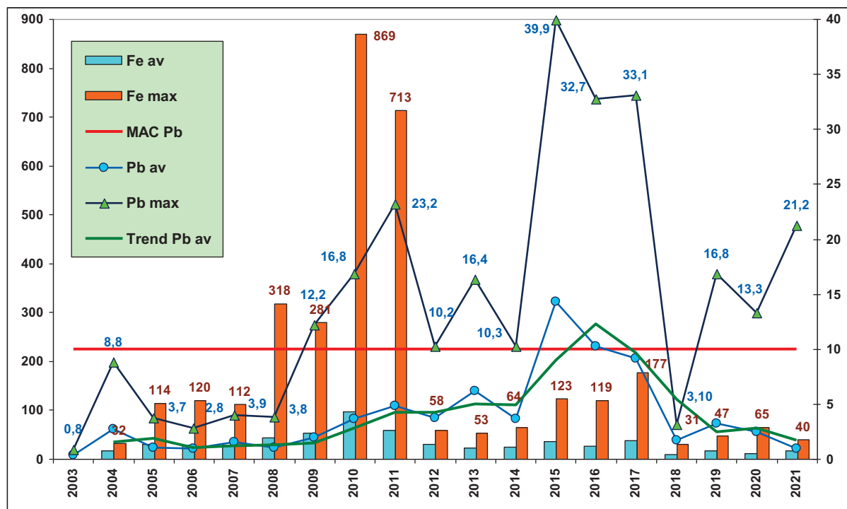
Рис. 3.64. Средняя и максимальная концентрации железа и свинца (мкг/дм 3 ) в прибрежных водах района Адлер-Сочи в 2003-2021 гг.
