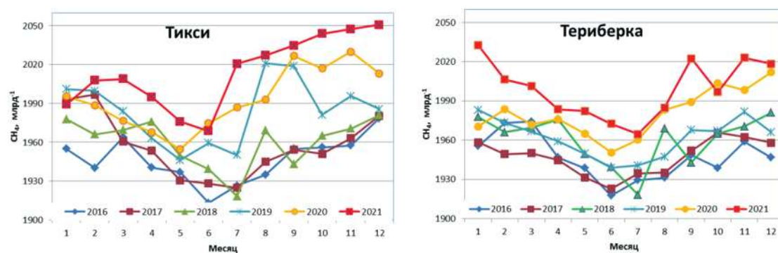
Рис. 2.2. Сезонный ход концентраций CH 4 на станциях Тикси и Териберка
