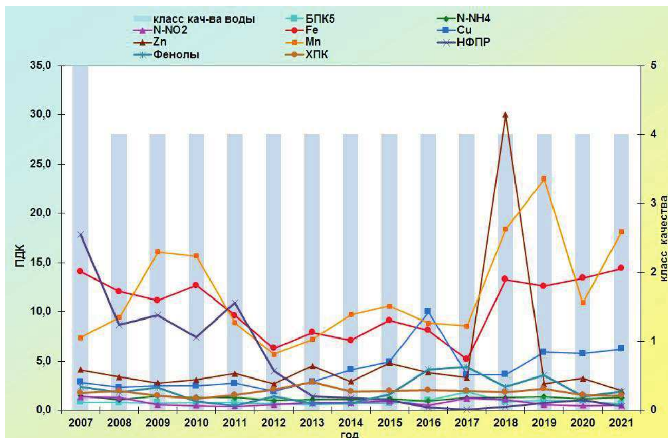
Рис. 3.43. Изменение среднегодовых концентраций отдельных загрязняющих веществ и показателей качества воды р. Обь ниже г. Салехарда за многолетний период
