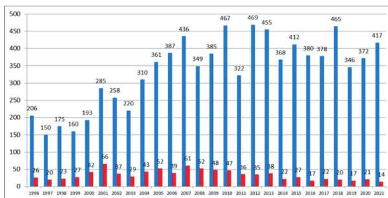
Рис. 1.5. Распределение гидрометеорологических ОЯ по годам: общее количество (синий) и количество непредусмотренных ОЯ (красный)
