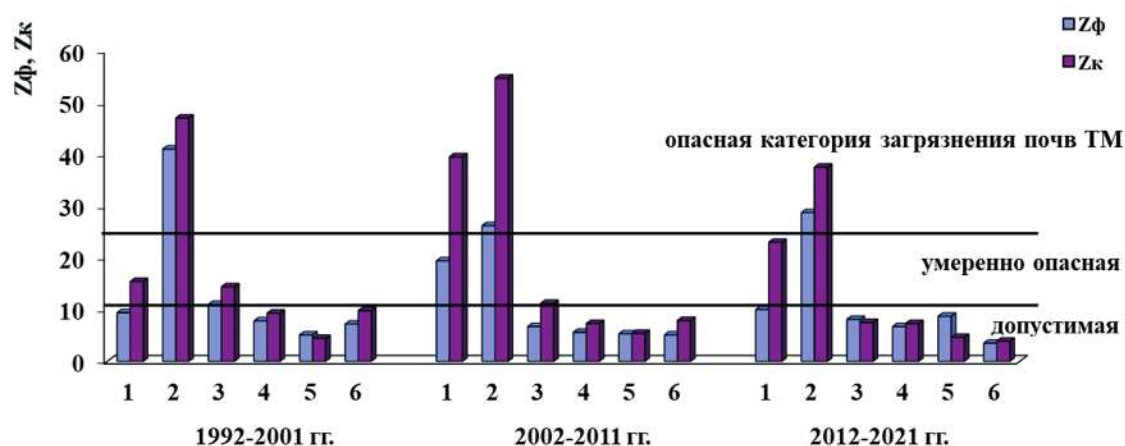
Рис. 3.23. Динамика усреднённых за несколько лет показателей загрязнения почв комплексом ТМ Z_f и Z_k вокруг предприятий черной металлургии (1), цветной металлургии (2), машиностроения и металлообработки (3), топливной и энергетической промышленности (4), химической и нефтехимической промышленности (5), строительной промышленности и производства стройматериалов (6)
