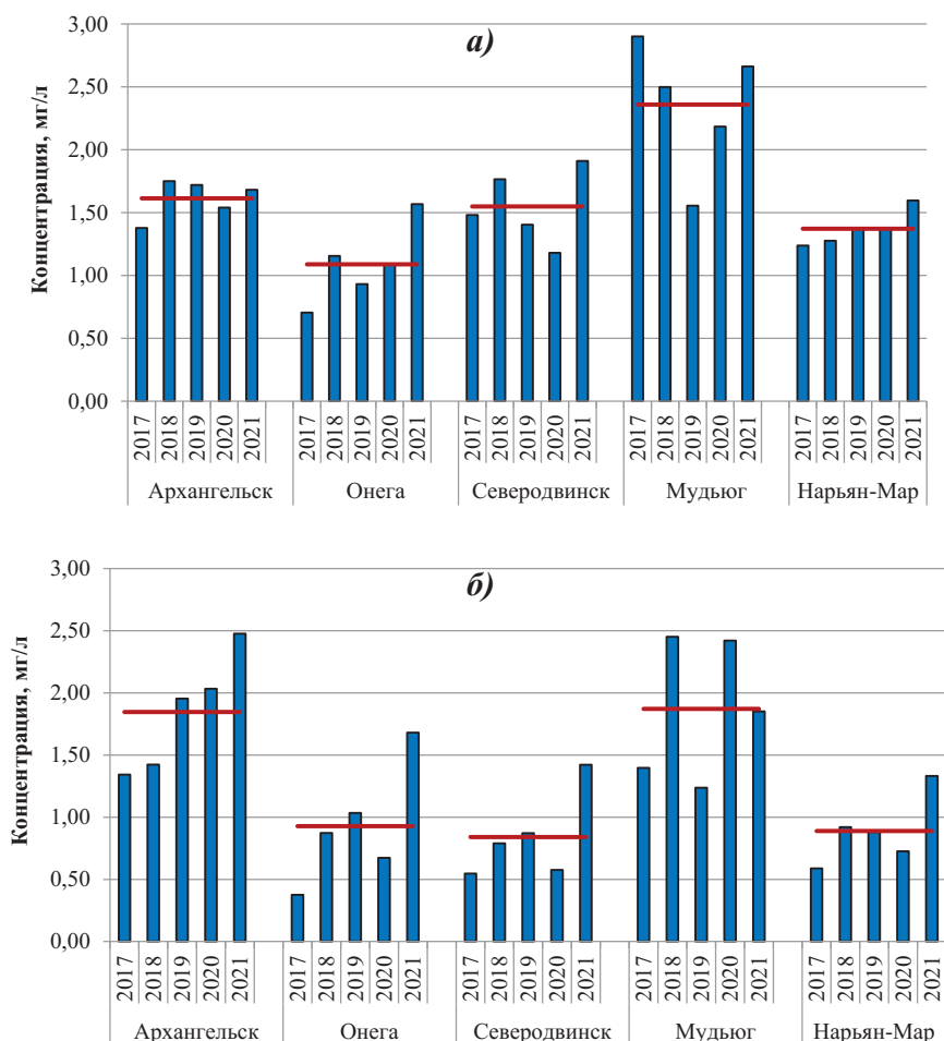
Рис. 4.39. Изменение средневзвешенной концентрации сульфатов (а) и нитратов (б) в осадках Архангельской обл. и Ненецкого АО в 2017-2021 гг.
