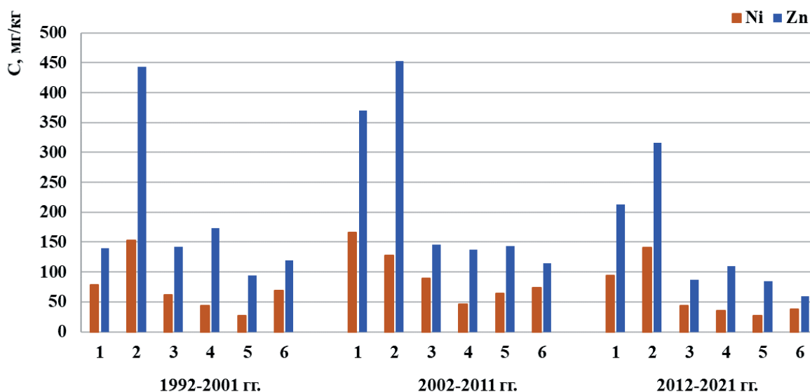
Рис. 3.24. Динамика массовых долей никеля и цинка, усредненных за разные периоды наблюдений, в почвах 5-километровых зон вокруг предприятий черной металлургии (1), цветной металлургии (2), машиностроения и металлообработки (3), топливной и энергетической промышленности (4), химической и нефтехимической промышленности (5), строительной промышленности и производства стройматериалов (6)
