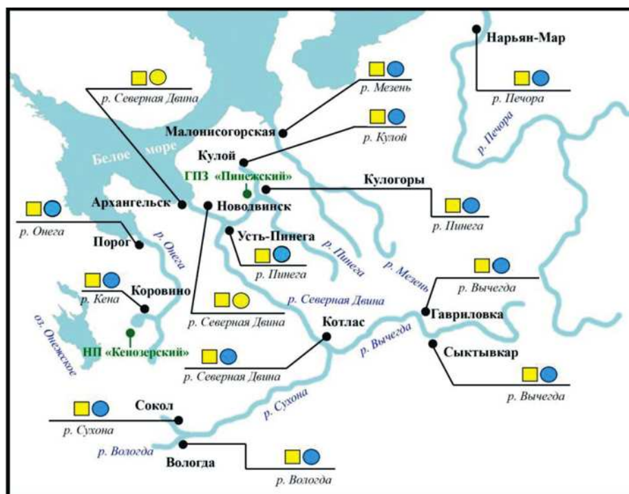
Рис. 4.56. Качество водотоков Севера ЕЧР по гидробиологическим показателям в 2021 г. Обозначения такие же, как на рис. 4.55
