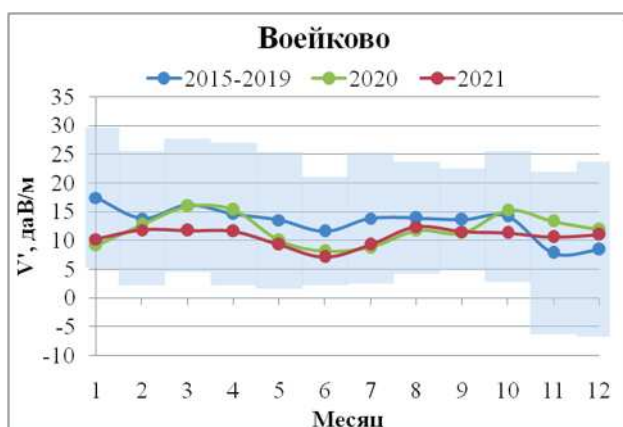
Рис. 2.8. Годовой ход V' по станциям Воейково, Иркутск в 2021 г. в сравнении с 2020 г. и на фоне осредненного годового хода V' за период 2015-2019 гг.
