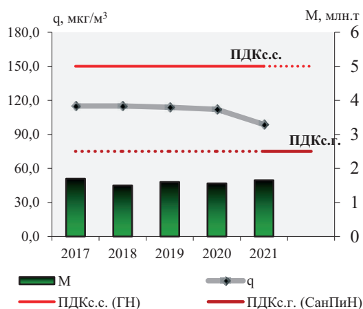
Рис. 3.9. Среднегодовые концентрации ( q , мкг/м³) и выбросы от стационарных источников ( M , млн. т) твердых веществ
