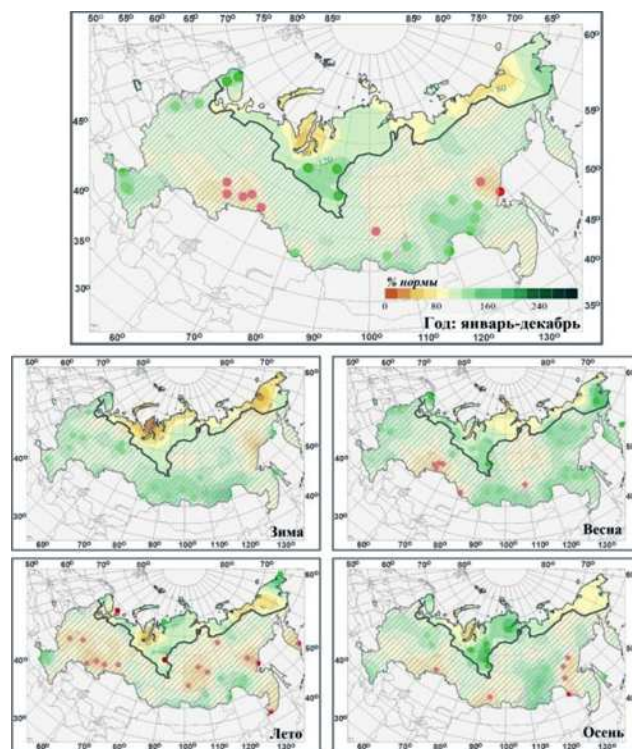
Рис. 4.28. Годовые (январь-декабрь) и сезонные суммы осадков (% от нормы периода 1961-1990 гг.) в Российской Арктике. Зелеными кружками показаны станционные аномалии выше 95-го перцентиля, красными - ниже 5-го.
