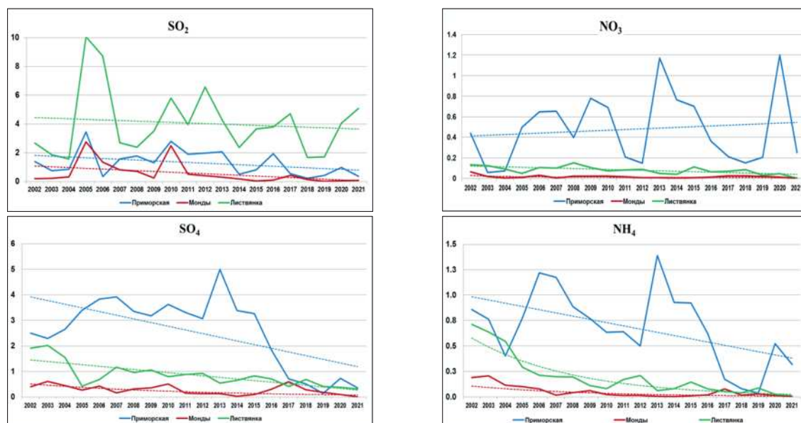
Рис. 2.28. Изменения средних годовых концентрации соединений серы (слева) и азота (справа) в воздухе на станциях ЕАНЕТ (мкг/м³)
