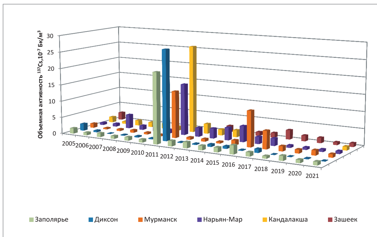
Рис. 4.58. Объемная активность ^{137}\text{Cs} в приземной атмосфере в пунктах наблюдения Сухопутных территорий Арктики и в среднем по Заполярье в 2005-2021 гг., 10^{-7} Бк/м 3
