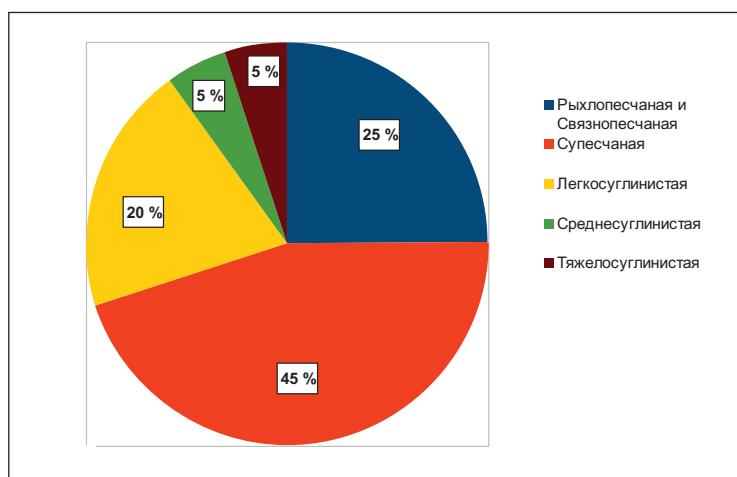
Рис. 4.20. Разновидности почв на территории г. Байкальска
