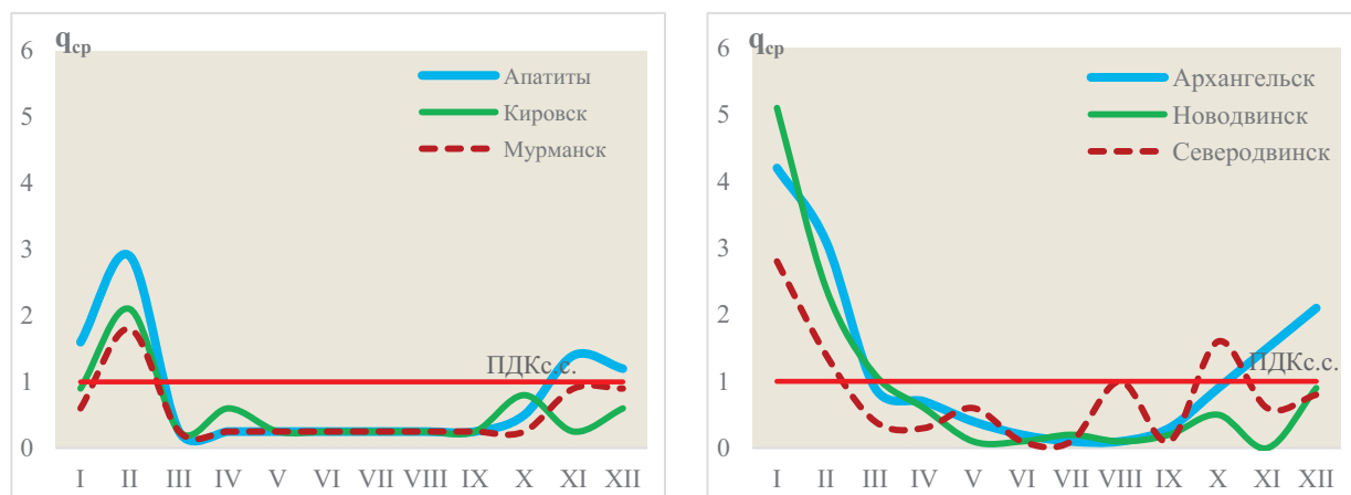
Рис. 4.47. Годовой ход бенз(а)пирена в городах АЗРФ в 2021 г., q_{cp} , нг/м³
