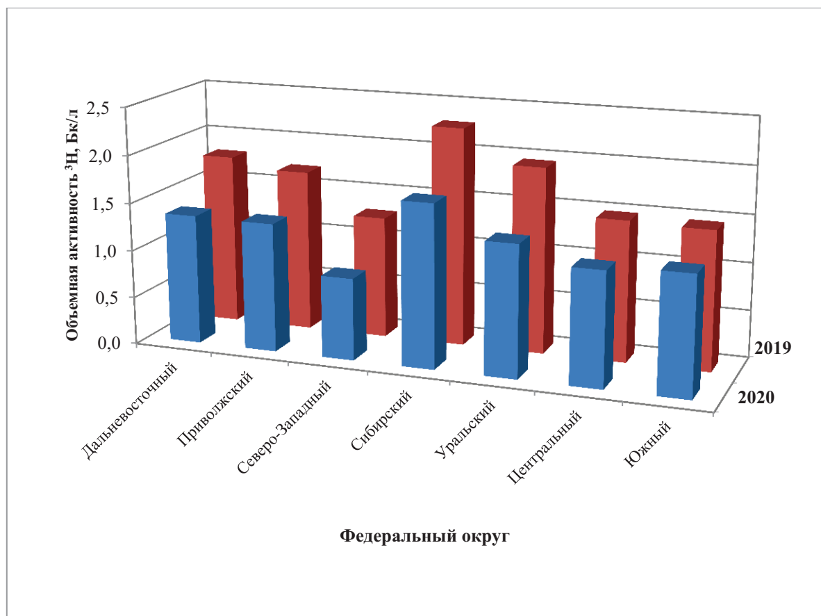
Рис. 2.40. Среднегодовая объемная активность ^3\text{H} в атмосферных осадках на территории федеральных округов РФ в 2020-2019 гг., Бк/л
