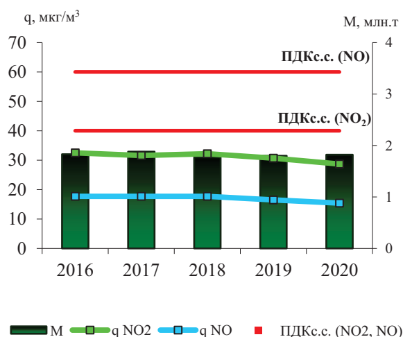
Рис. 3.12. Среднегодовые концентрации диоксида ( q\text{NO}_2 , мкг/м³) и оксида азота ( q\text{NO} , мкг/м³) и выбросы от стационарных источников ( M , млн. т) \text{NO}_x (в пересчете на \text{NO}_2 )
