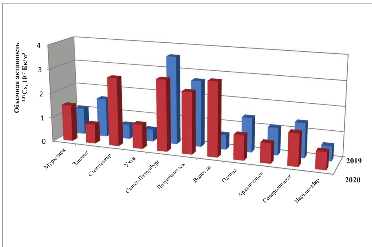
Рис. 2.37. Среднегодовая объемная активность ^{137}\text{Cs} в населенных пунктах СЗФО в 2019-2020 гг., 10^{-7} Бк/м 3
