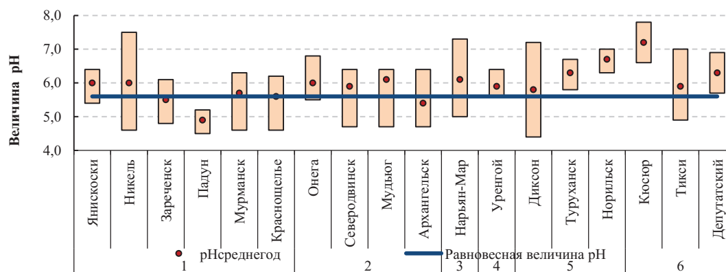
Рис. 4.37. Диапазон изменений значений pH суммарных ежемесячных проб осадков на арктических станциях в 2020 г.
