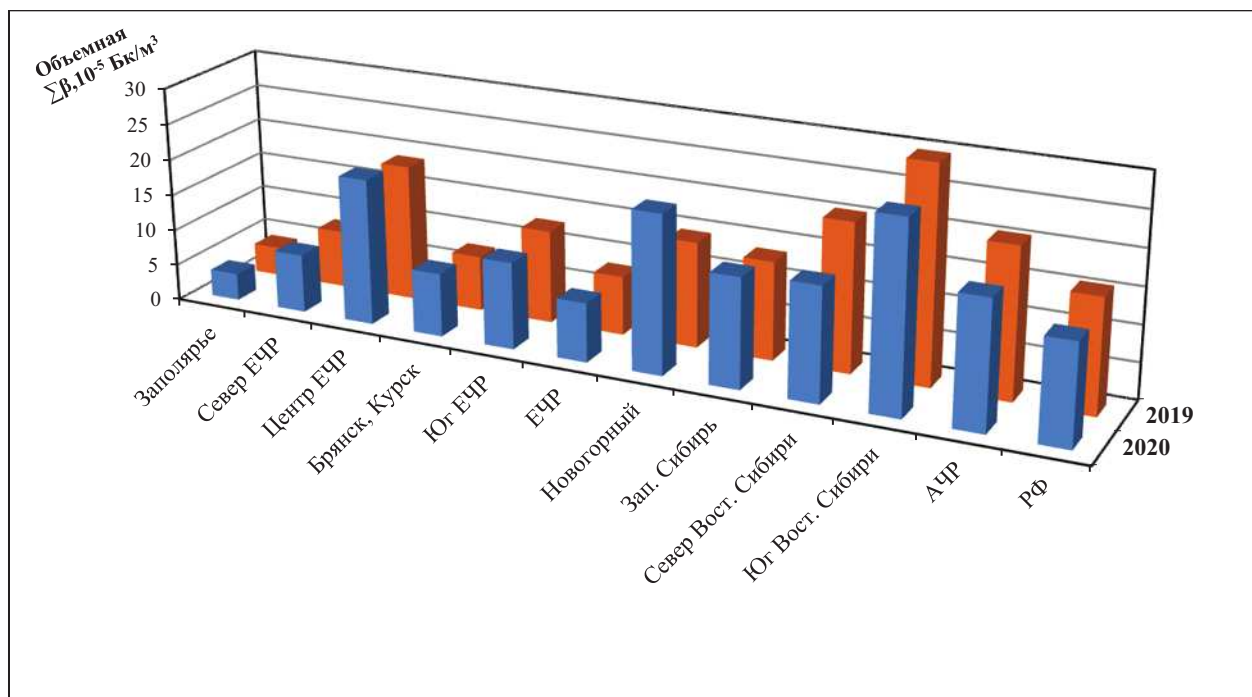
Рис. 2.36. Средние значения объемной ΣВ в приземном слое атмосферы на территории РФ в 2019-2020 гг., 10^{-5} Бк/м 3
