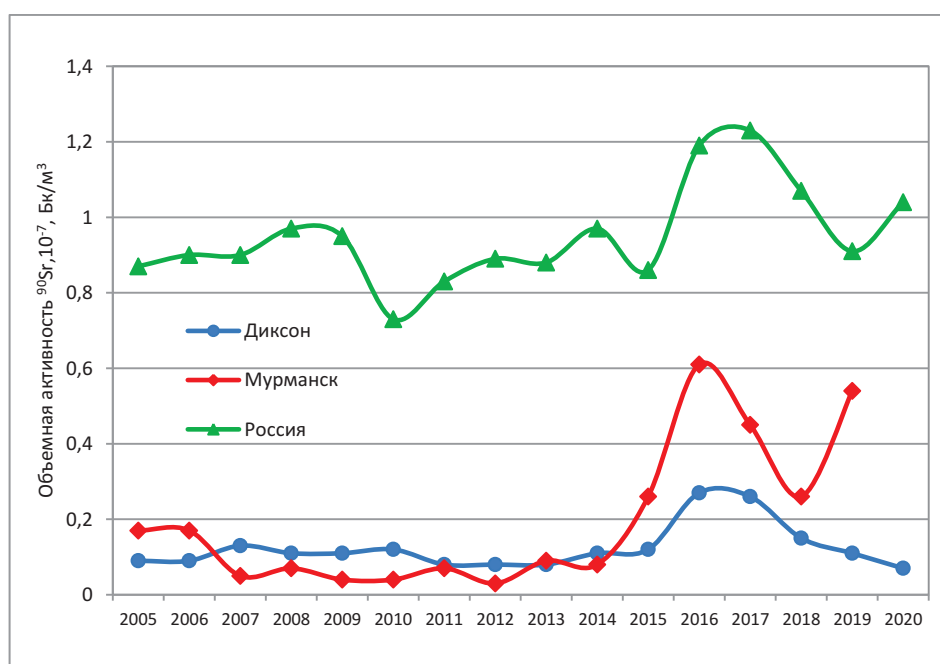
Рис. 4.55. Динамика объемной активности ^{90}\text{Sr} в воздухе на о. Диксоне, в Мурманске и средневзвешенной по России в 2005-2020 гг.
