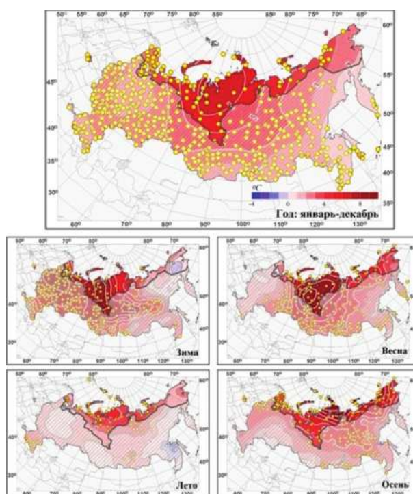
Рис. 4.24. Годовые (январь-декабрь) и сезонные аномалии температуры воздуха в Российской Арктике. Аномалии (°C) рассчитаны относительно норм периода 1961-1990 гг. Желтыми кружками показаны аномалии выше 95-го процентиля
