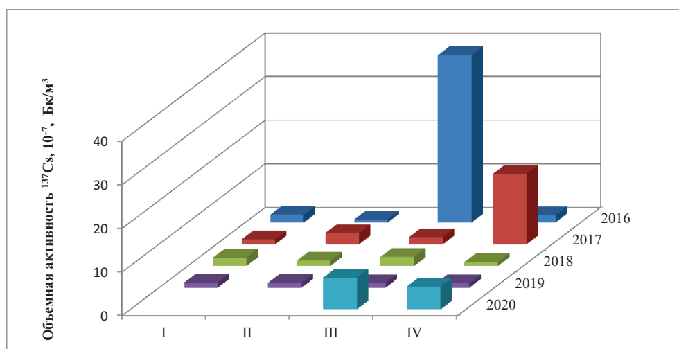
Рис. 4.54. Динамика средней за квартал величины объемной активности ^{137}\text{Cs} в воздухе в Мурманске в 2016-2020 гг.
