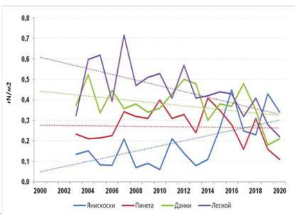
Рис. 2.28. Многолетние выпадения суммарного азота (нитратного и аммонийного) из атмосферы с осадками на станциях ЕМЕП (г N/м 2 /год)
