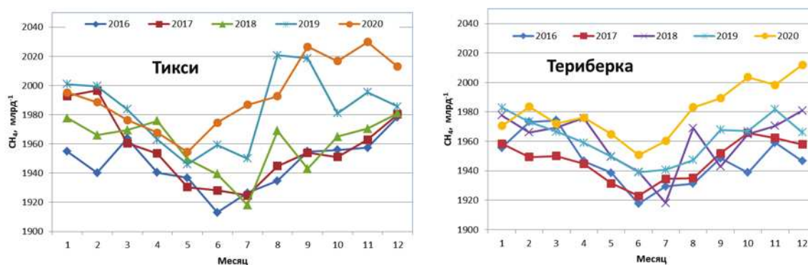
Рис. 2.2. Сезонный ход концентрации CH 4 на станциях Тикси и Териберка
