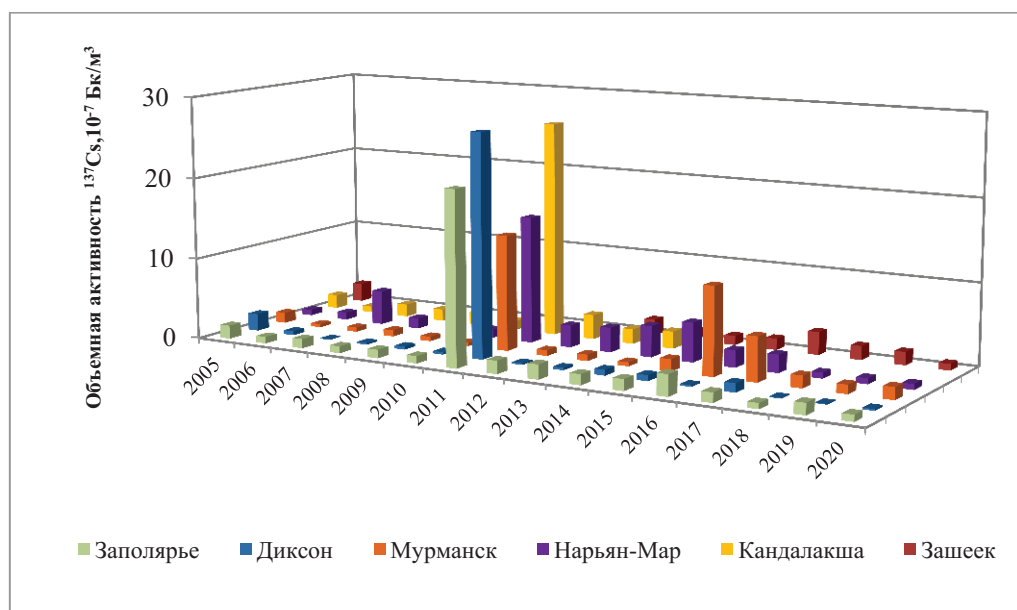
Рис. 4.53. Объемная активность ^{137}\text{Cs} в приземной атмосфере в пунктах наблюдения Сухопутных территорий Арктики и в среднем по Заполярье в 2005-2020 гг., 10^{-7} Бк/м 3
