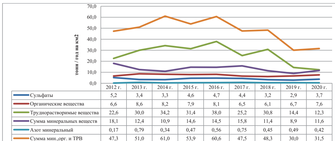
Рис. 4.16. Динамика поступления химических веществ из атмосферы на ст. Большое Голоустное
