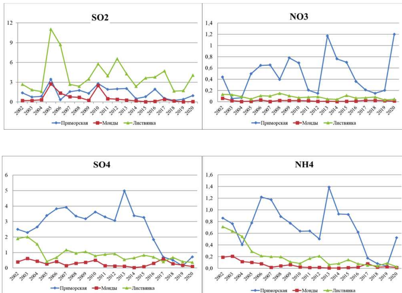
Рис. 2.30. Изменения средних годовых концентрации соединений серы (слева) и азота (справа) в воздухе на станциях ЕАНЕТ (мкг/м 3 )
