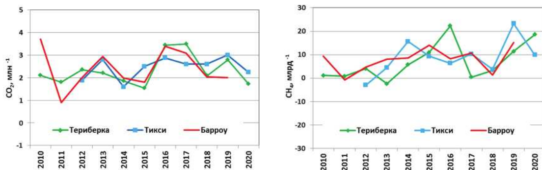
Рис. 2.1. Межгодовые изменения концентрации CO 2 и CH 4
