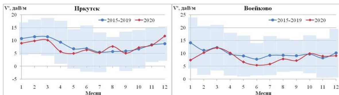
Рис. 2.8. Годовой ход V' по станциям атмосферно - электрической сети Воейково и Иркутск в 2020 г. на фоне осредненного годового хода V' за период 2015-2019 гг.
