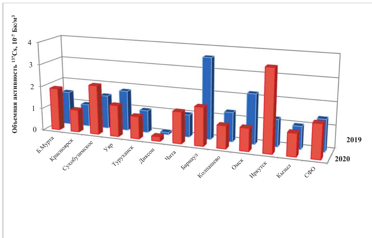
Рис. 2.38. Среднегодовая объемная активность ^{137}\text{Cs} в населенных пунктах СФО в 2019-2020 гг., 10^{-7} Бк/м 3
