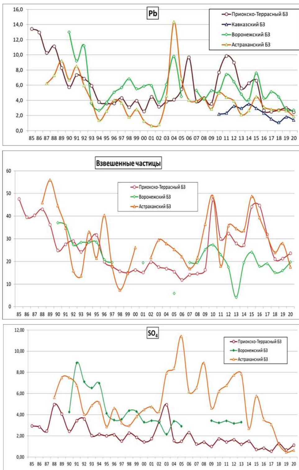
Рис. 2.14. Многолетнее изменение среднегодового содержания свинца ( \text{нг}/\text{м}^3 ), взвешенных частиц и сульфатов ( \text{мкг}/\text{м}^3 )
