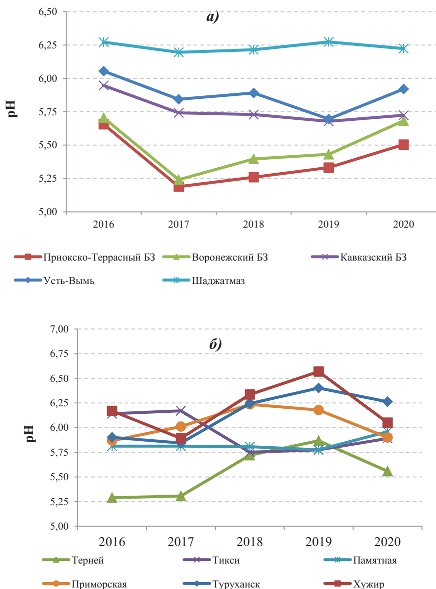
Рис. 2.17. Изменение среднегодовых значений pH атмосферных осадков фоновых станций на ЕЧР (а) и АЧР (б) в период с 2016 по 2020 гг.
