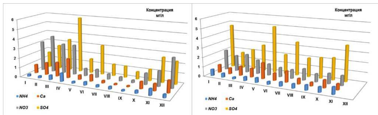
Рис. 2.31 (начало). Годовой ход концентраций (верхний) и выпадений (нижний) основных кислотообразующих ионов с осадками в районе оз. Байкал (ст. Листвянка, слева) и на Дальнем Востоке (ст. Приморская, справа) в 2020 г.
