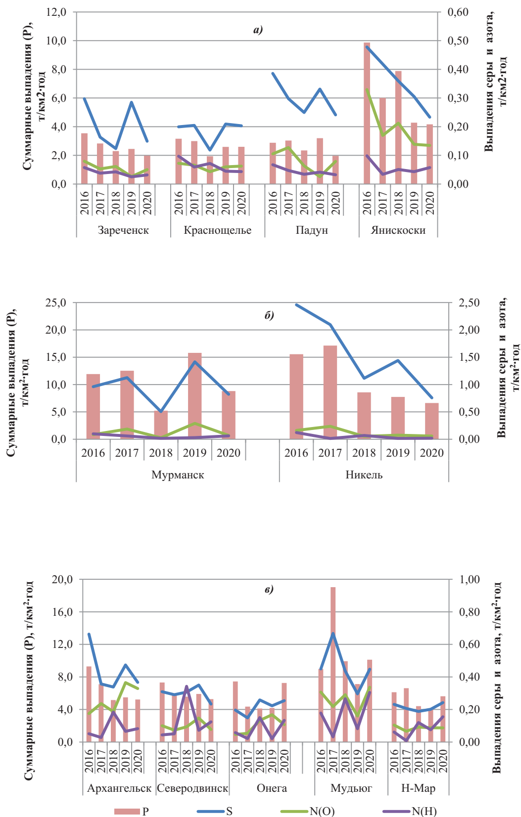
Рис. 4.38. Межгодовой ход суммарных влажных выпадений (P) и выпадений серы (S), нитратного (N(O)) и аммиачного (N(H)) азота на территории Мурманской обл. (а, б), Архангельской обл. и Ненецкого АО (в)
