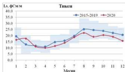
Рис. 4.33. Годовой ход L_s на станциях Тикси и Диксон за 2020 г. на фоне осредненного годового хода L_s за предшествующий период
