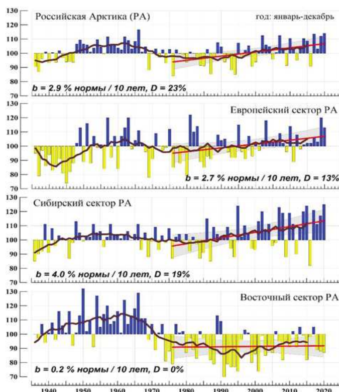
Рис. 4.29. Годовые (январь-декабрь) суммы осадков (% нормы) в Российской Арктике и ее секторах в 1936-2020 гг. Жирная черная кривая - 11-летнее скользящее среднее. Показан линейный тренд за 1976-2020 гг.
