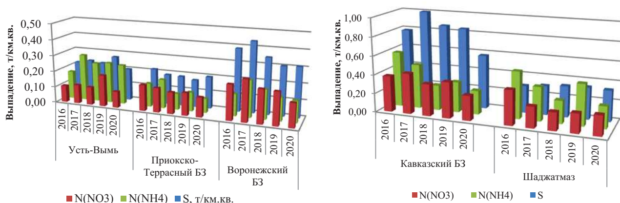
Рис. 2.18. Выпадения серы (S), азота нитратного ( \text{N}(\text{NO}_3) ) и азота аммонийного ( \text{N}(\text{NH}_4) ) с атмосферными осадками на ЕЧР в период с 2016 по 2020 гг.
