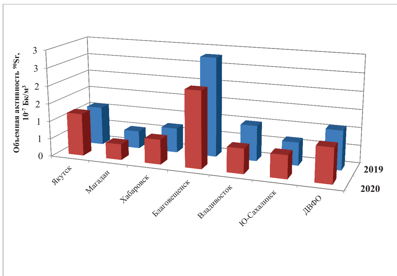
Рис. 2.39. Среднегодовая объемная активность ^{90}\text{Sr} в населенных пунктах ДВФО в 2019-2020 гг., 10^{-7} Бк/м 3
