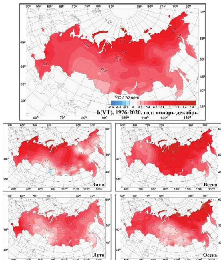
Рис. 1.9. Распределение коэффициентов линейного тренда среднегодовой и средних сезонных значений температуры приземного воздуха на территории России за период 1976-2020 гг. ( ^{\circ}\text{C}/10 лет).
