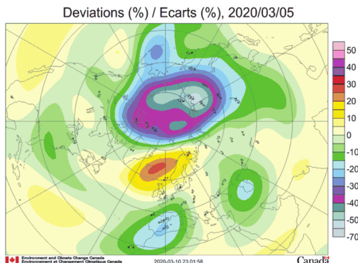
Рис. 2.13. Поле ОСО над Северным полушарием 05.03.2020 г. по данным канадского центра по окружающей среде и изменениям климата https://exp-studies.tor.ec.gc.ca .
