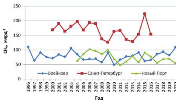
Рис. 2.3. Среднегодовое превышение концентрации CH 4 над фоновым уровнем
