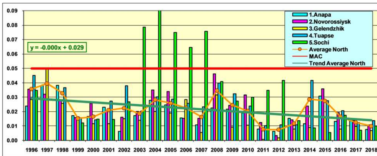
Рис. 3.59. Динамика среднегодовой концентрации нефтяных углеводородов (мг/дм³) в прибрежных водах Кавказа в 1996-2018 гг. Сокращения: Average North - средняя величина в северной части Кавказского побережья; MAC - предельно допустимая концентрация; Trend Average North - тренд концентрации НУ в северной части побережья.
