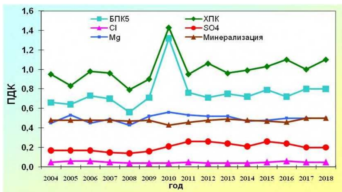
Рис. 2.35 (начало). Изменение среднегодовых концентраций отдельных ингредиентов и качество воды р. Лесной Воронеж выше г. Мичуринск в многолетнем плане
