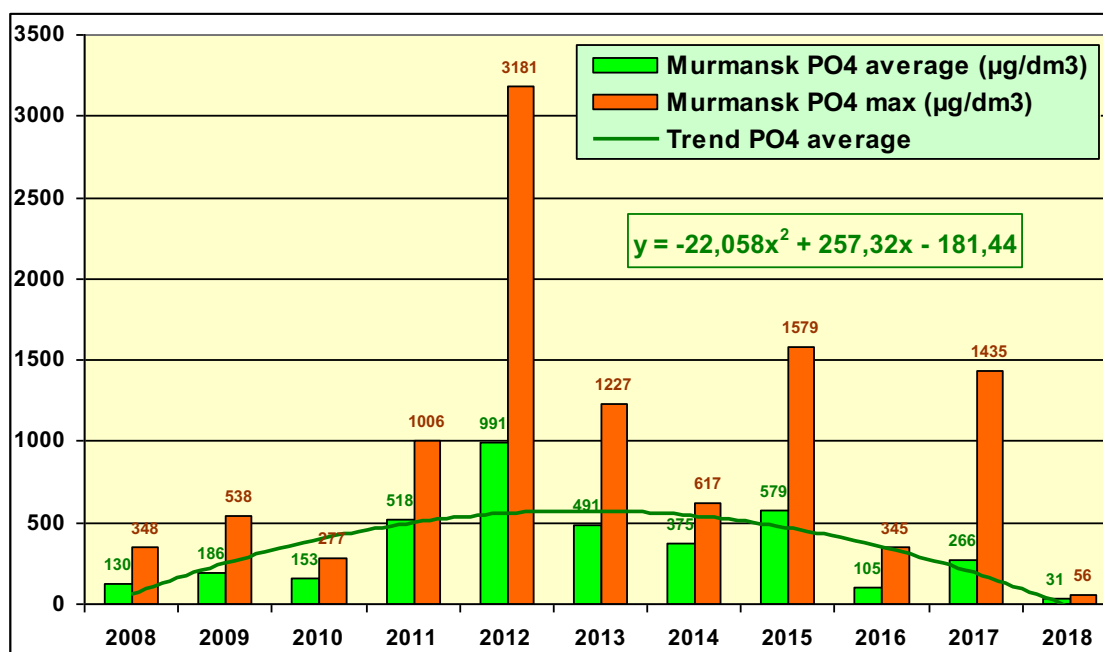
Рис. 3.65. Динамика среднегодовой и максимальной концентраций неорганического фосфора Р-Р О4 (мкг/дм³) в водах водпоста торгового порта г. Мурманска в 2008-2018 гг.
