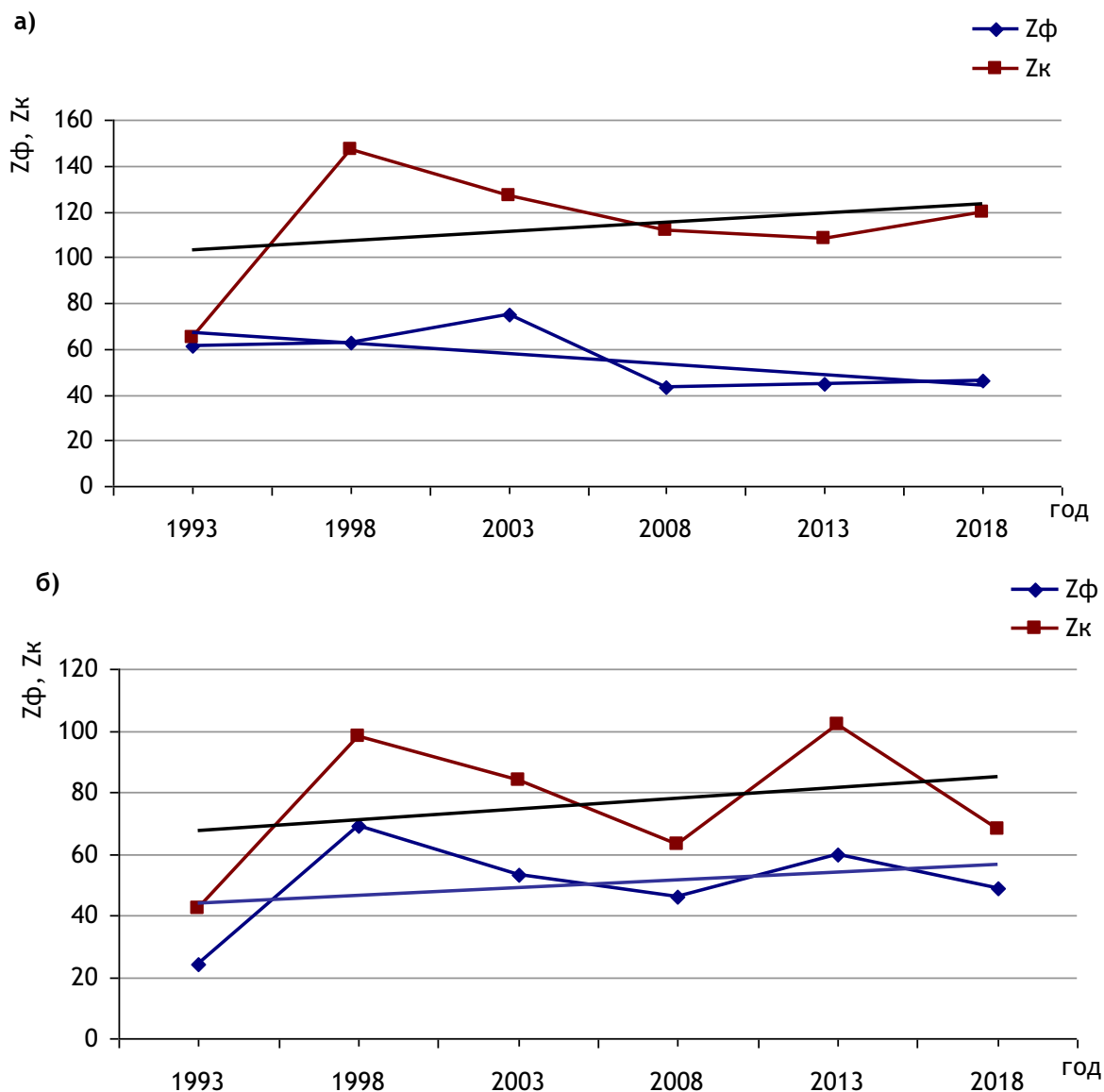
Рис. 3.22. Динамика изменений показателей загрязнения почв Z_f и Z_k комплексом тяжелых металлов г. Кировград (а) и г. Реж (б) в 1993-2018 гг.
