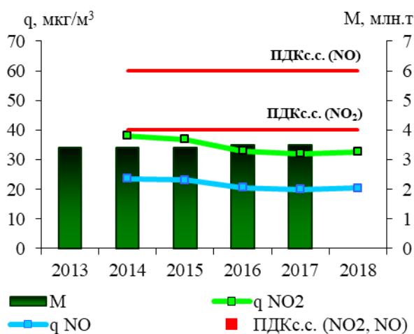
Рис. 3.12. Среднегодовые концентрации диоксида ( qNO_2 , мкг/м³) и оксида азота ( qNO , мкг/м³) и суммарные выбросы ( M , млн. т) NO_x (в пересчете на NO_2 )
