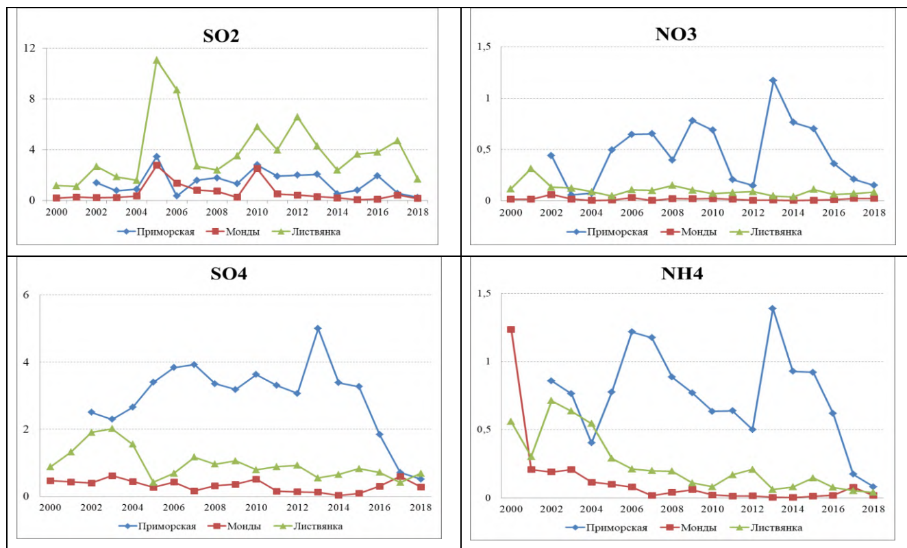
Рис. 2.31. Изменения средних годовых концентрации соединений серы (слева) и азота (справа) в воздухе на станциях ЕАНЕТ ( \mu\text{г}/\text{м}^3 )
