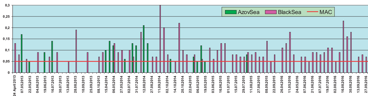
Рис. 3.62. Максимальное содержание нефтяных углеводородов (мг/дм 3 ) в черноморских водах с соленостью более 13‰ и менее соленых азовских морских водах в Керченском проливе в 2013–2016 гг.
