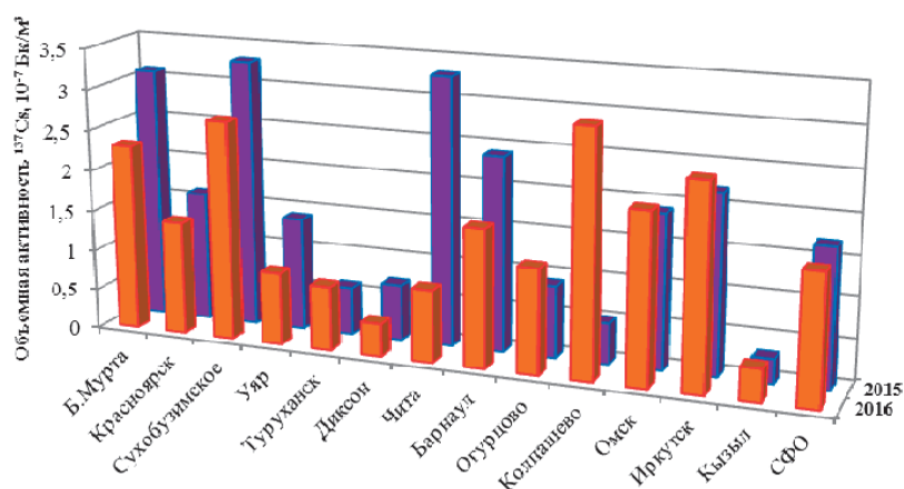
Рис. 2.46. Среднегодовая объемная активность ^{137}\text{Cs} в населенных пунктах СФО в 2015–2016 гг., 10^{-7} \text{ Бк/м}^3
