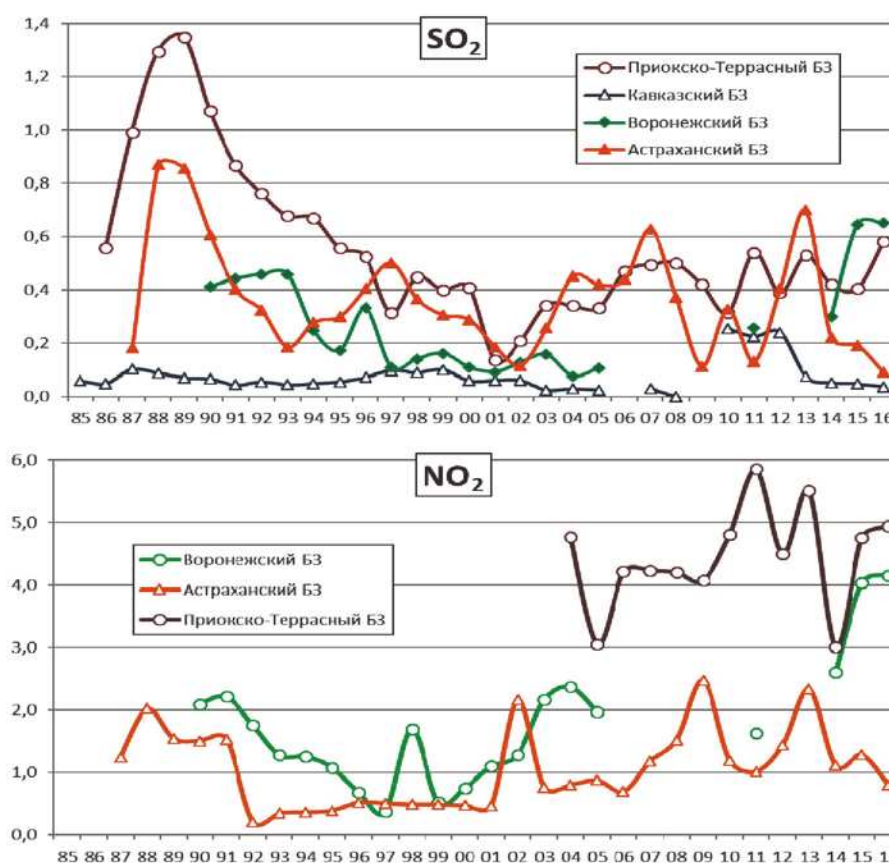
Рис. 2.15. Изменение фоновых содержания диоксида серы и диоксида азота в атмосферном воздухе фоновых районов (мкг/м 3 )
