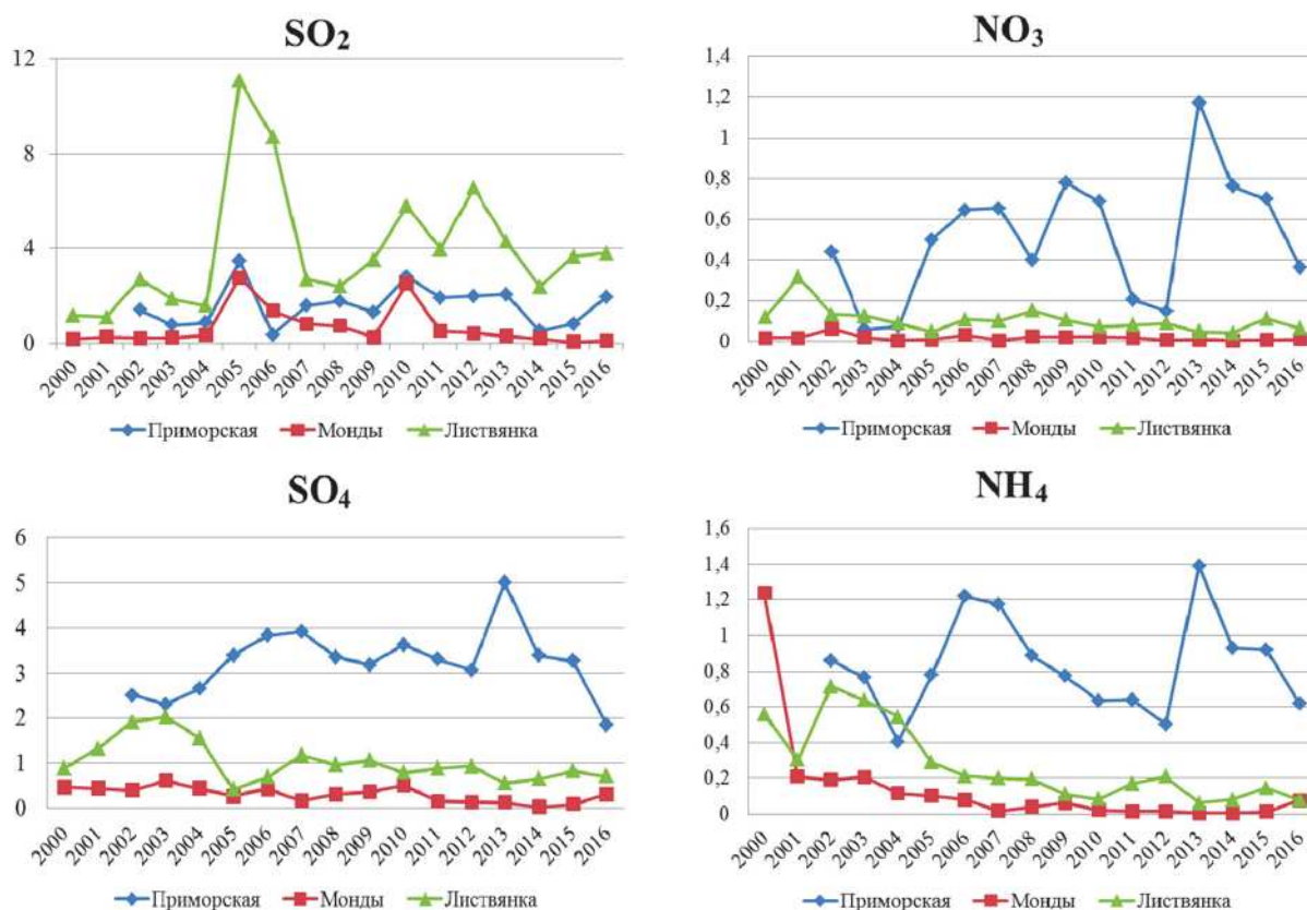
Рис. 2.37. Изменения средних годовых концентрации соединений серы (слева) и азота (справа) в воздухе на станциях ЕАНЕТ ( \mu\text{кг}/\text{м}^3 )
