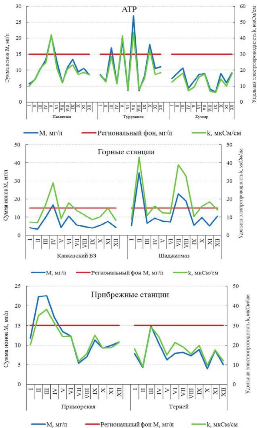
Рис. 2.17. Годовой ход минерализации и удельной электропроводности атмосферных осадков на станциях фонового мониторинга, 2016 г.
