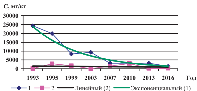
Рис. 3.27. Динамика средних массовых долей НП в почвах нефтяного пятна (1) и за его пределами по разным направлениям до 250 м (2) вблизи п. Тьреть Заларинского района Иркутской области
