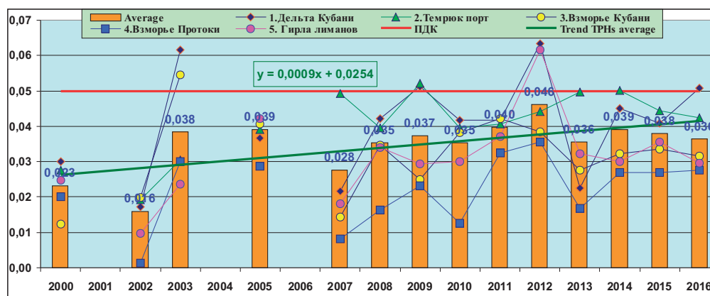
Рис. 3.60. Многолетняя динамика средней концентрации нефтяных углеводородов (мг/дм³) в водах дельты Кубани и Темрюкского залива Азовского моря
