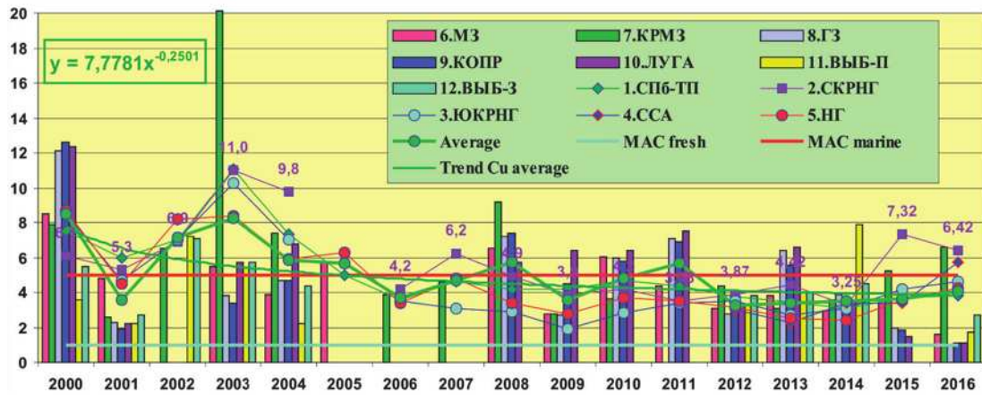
Рис. 3.63. Многолетняя динамика средней концентрации меди (мкг/дм³) в водах восточной части Финского залива в 2000–2016 г.
