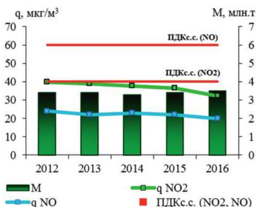
Рис. 3.12. Среднегодовые концентрации диоксида ( q_{NO_2} ) и оксида азота ( q_{NO} ) и суммарные выбросы ( M ) NO_x (в пересчете на NO_2 )
