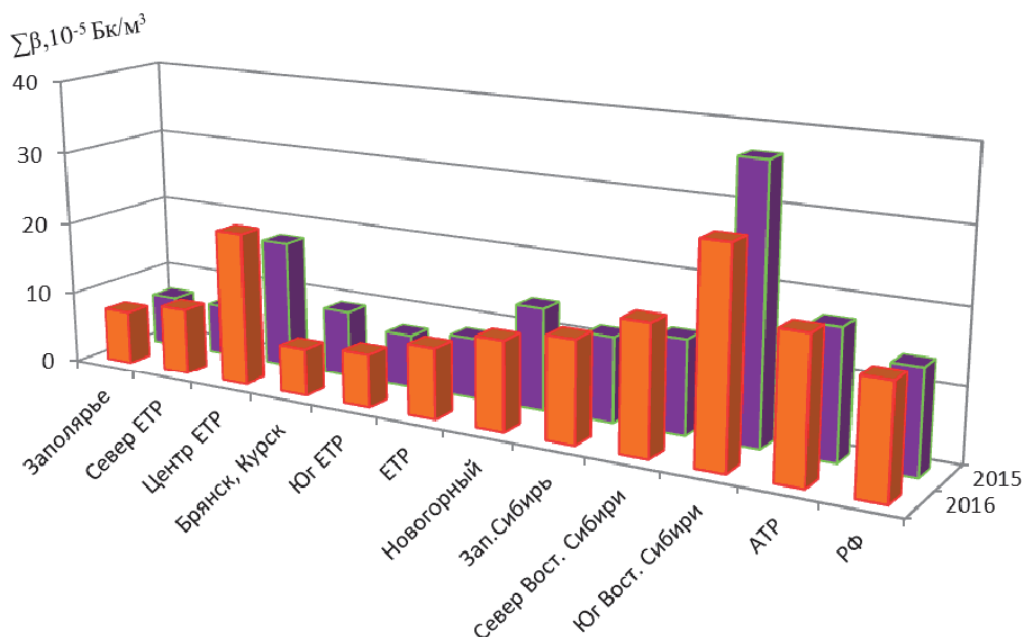
Рис. 2.44. Средние значения объемной \Sigma\beta в приземном слое атмосферы на территории РФ в 2015–2016 годах, 10^{-5} \text{ Бк/м}^3
