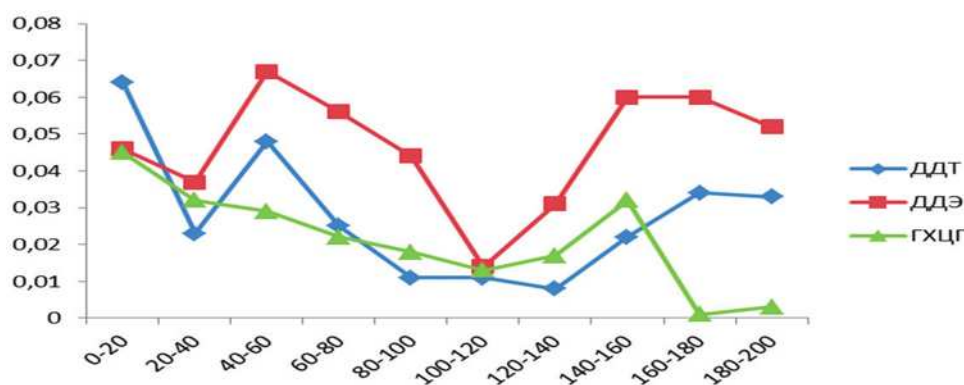
Рис. 3.28. Распределение хлорорганических пестицидов по почвенному профилю в результате многолетней вертикальной миграции
