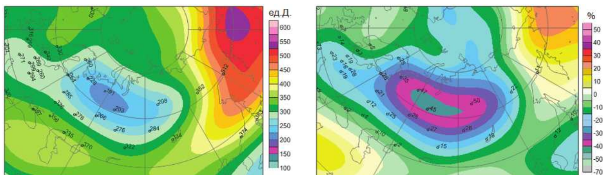
Рис. 2.10. Поле общего содержания озона (ед.Д.; слева) 28 января 2016 г. и его отклонения(%; справа) от средних многолетних (1978–1988 гг.) значений по данным WUODC, Канада
