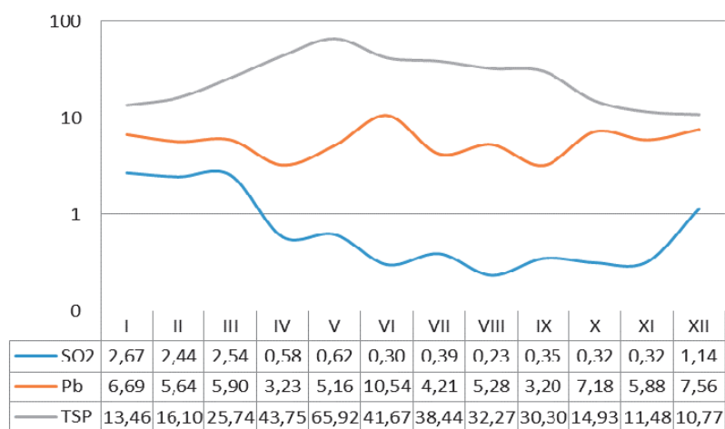
Рис. 2.16. Сезонный ход загрязняющих веществ в Приокско-Террасном БЗ, осредненный за 2003–2016 гг. (свинец – \text{нг/м}^3 , диоксид серы и взвешенные частицы – \text{мкг/м}^3 )
