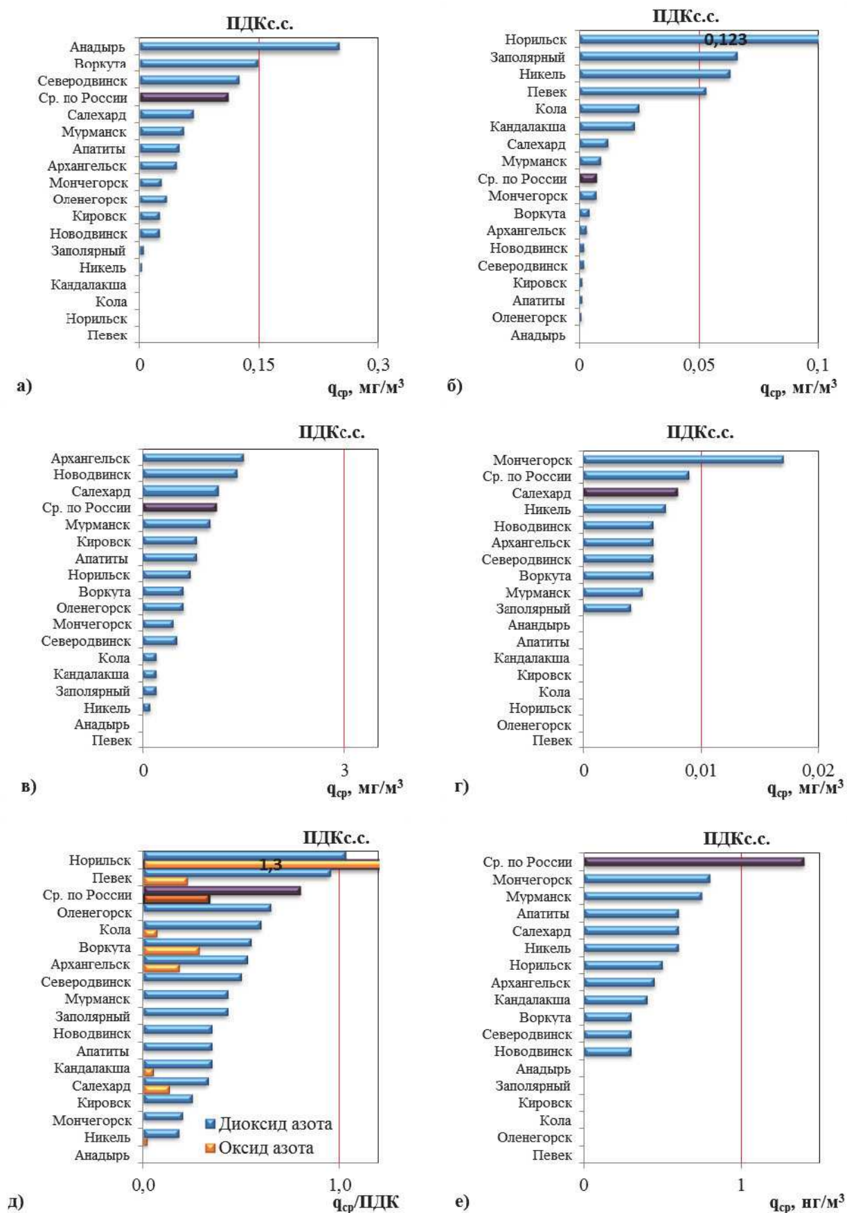
Рис. 4.35. Средние за год концентрации: взвешенных веществ (а), диоксида серы (б), оксида углерода (в), формальдегида (г), q_{ср} , мг/м 3 , диоксида и оксида азота (д), q_{ср} , ПДК, бенз(а)пирена (е), q_{ср} , нг/м 3 , в городах АЗРФ и в целом по России
