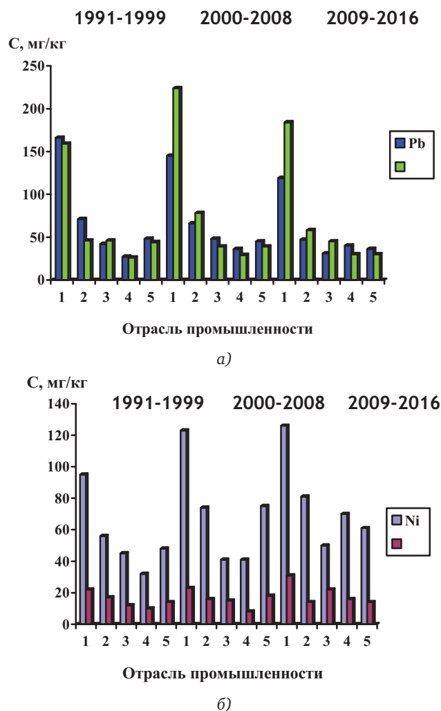
Рис. 3.24. Динамика средних по отраслям промышленности массовых долей, усредненных за определенные периоды:
