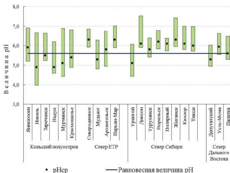
Рис. 4.28. Диапазоны изменения средней за год величины pH_{ср} , 2016 г.
