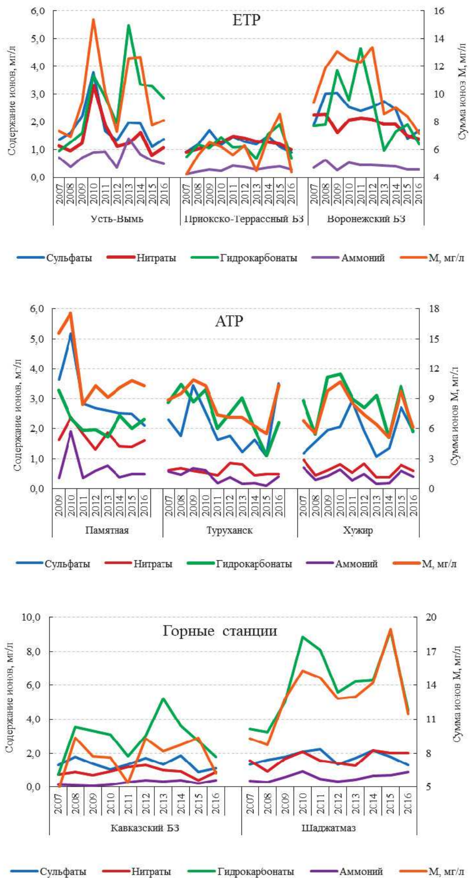
Рис. 2.18 (начало). Десятилетний ход содержания ионов и минерализации в осадках, 2007–2016 гг.
