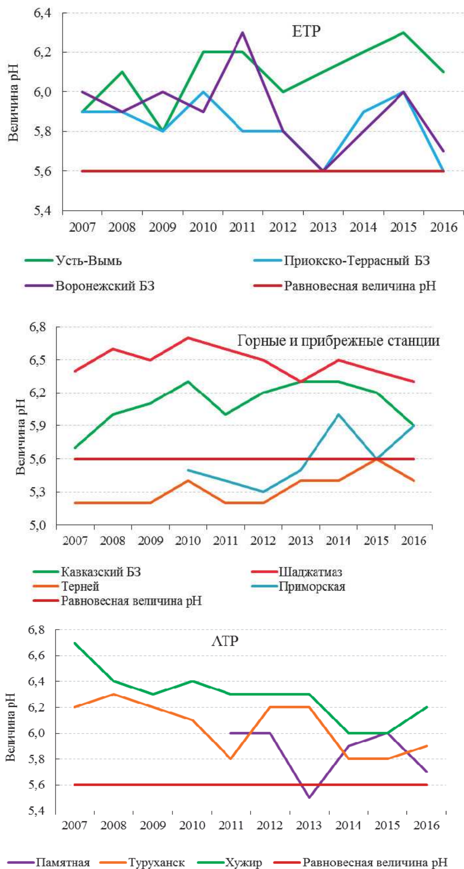
Рис. 2.19. Изменение со временем средней за год величины pH на станциях фонового мониторинга, 2007–2016 гг.
