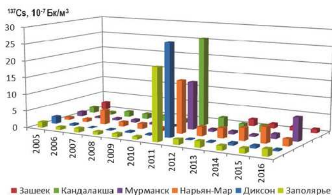
Рис. 4.37. Объемная активность ^{137}\text{Cs} в приземной атмосфере в пунктах наблюдения Сухопутных территорий Арктики и в среднем по Заполярье в 2005–2016 годах, 10^{-7} Бк/м 3
