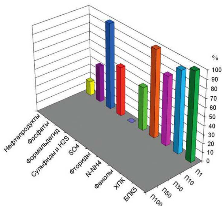
Рис. 3.40. Повторяемость числа случаев превышения ПДК разного уровня загрязняющими веществами в воде р. Вихорева, 7 км ниже с. Кобляково в 2016 г.
