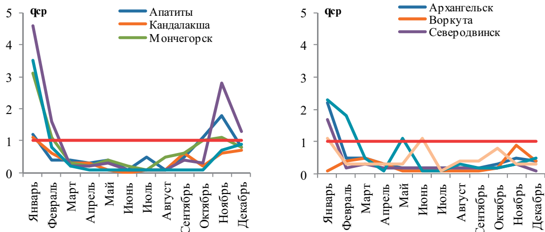
Рис. 4.36. Годовой ход бенз(а)пирена в городах АЗРФ в 2016 году, q_{cp} , нг/м 3
