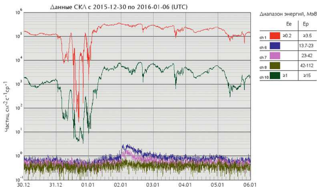
Рис. 1.5. Вторжение потоков протонов солнечных космических лучей (СКЛ) в январе 2016 года. Поток электронного и протонного излучения (5-минутные данные). Источник данных: КА «Электрон-Л» №1
