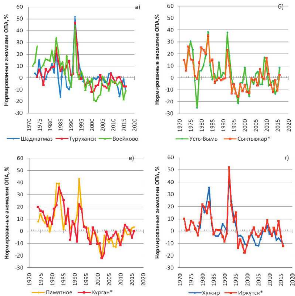
Рис. 2.6. Межгодовая изменчивость нормированных аномалий ОПА (%) на станциях фонового мониторинга атмосферы
