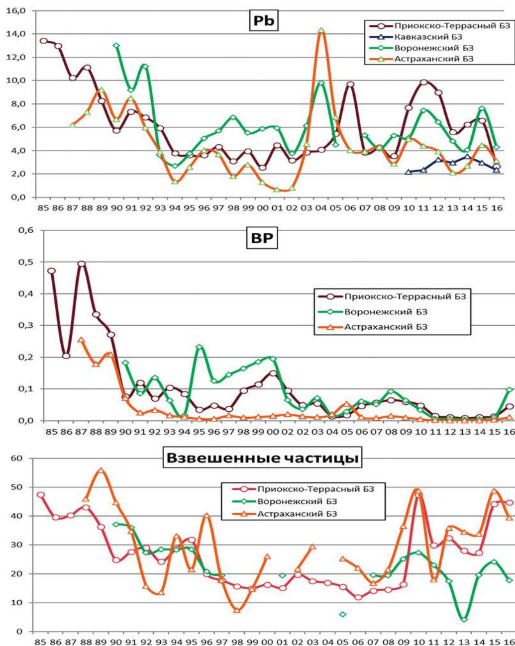
Рис. 2.14. Изменение фонового содержания свинца, 3,4-бензпирена (нг/м³) и взвешенных частиц (мкг/м³) в атмосферном воздухе фоновых районов
