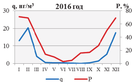
Рис. 3.23. Изменение среднемесячных концентраций бенз(а)пирена, q , нг/м 3 , и повторяемости приземной и приподнятой инверсий, P , %, в Магнитогорске в 2016 году
