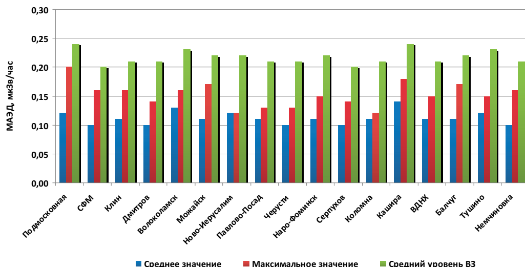
Рис. 4.14. Мощности амбиентного эквивалента дозы (МАЭД) на станциях Московского региона в 2016 году
