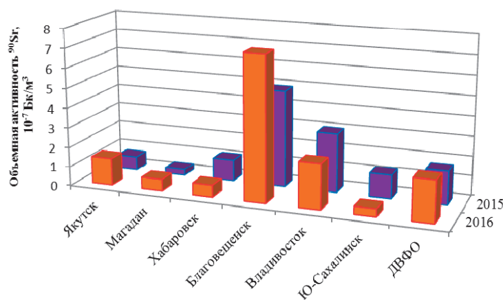
Рис. 2.47. Среднегодовая объемная активность ^{90}\text{Sr} в населенных пунктах ДВФО в первом полугодии 2015 года и первом полугодии 2016 года, 10^{-7} Бк/м 3
