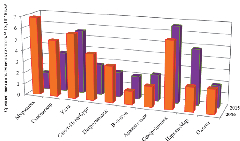
Рис. 2.45. Среднегодовая объемная активность ^{137}\text{Cs} в населенных пунктах СЗФО в 2015–2016 годах, 10^{-7} \text{ Бк/м}^3
