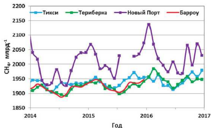
Рис. 4.25. Концентрация CH 4 для арктических станций РФ в сравнении со станцией Барроу
