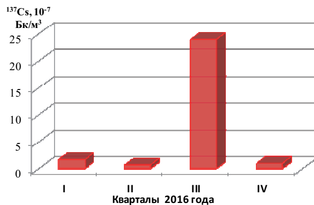
Рис. 4.38. Динамика средней за квартал величины объемной активности ^{137}\text{Cs} в воздухе в Мурманске в 2016 году
