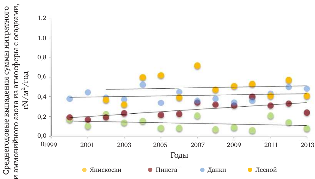
Рис. 2.36. Среднегодовые выпадения суммы нитратного и аммонийного азота из атмосферы с осадками, гN/м²/год
