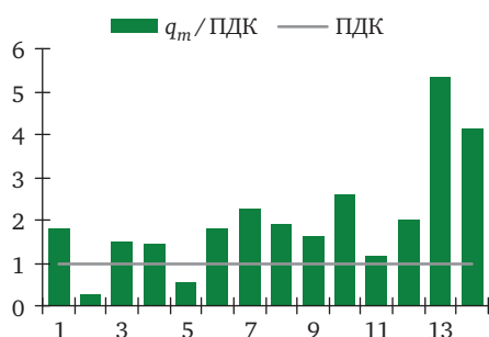
Рис. 3.17. Средние из максимальных концентрации загрязняющих веществ в городах России
