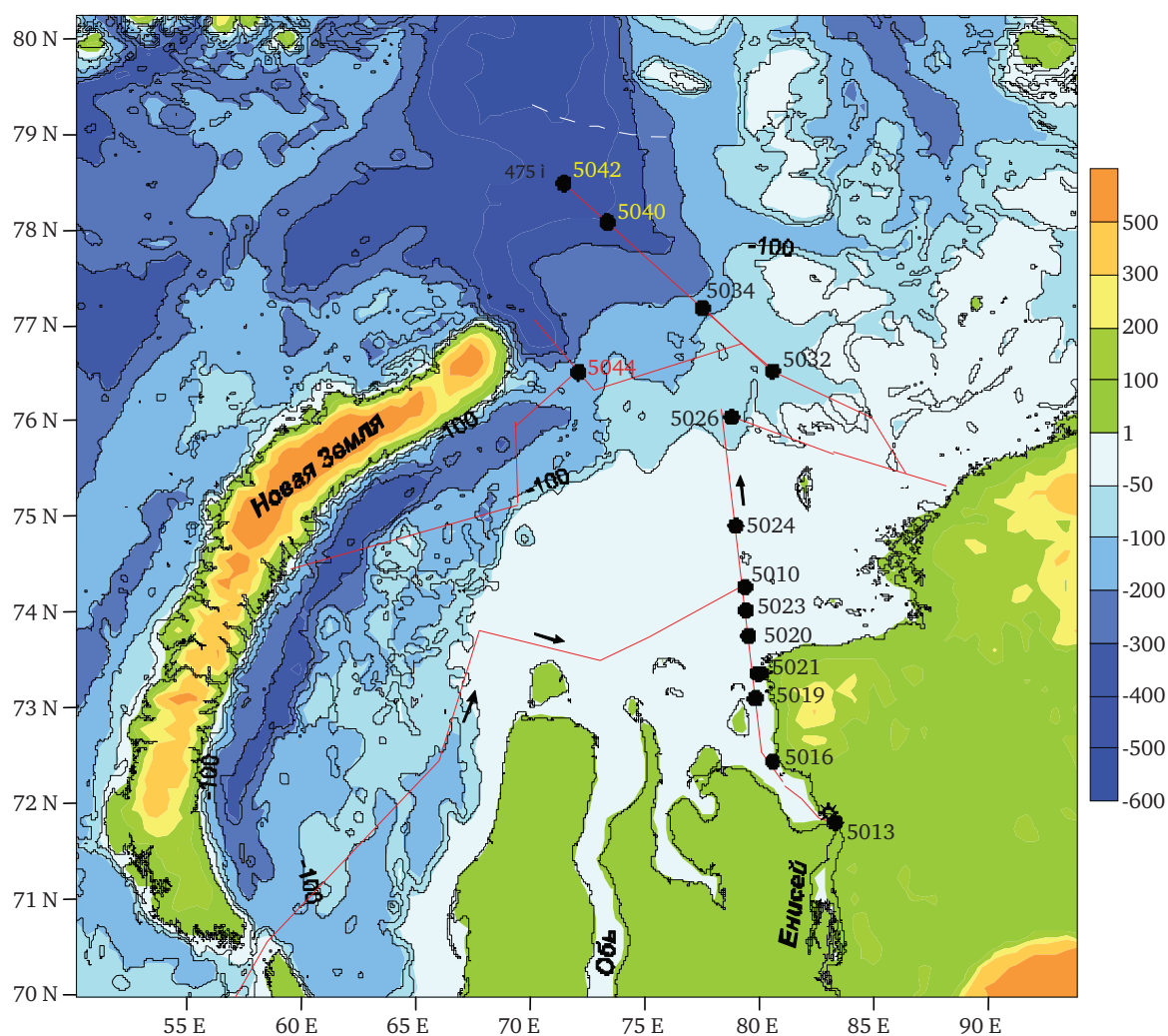
Рис. 3.58. Расположение станций. Нумерация станций: на карте порядковый № для НИС АМК – например, № 5026, в тексте – № 26
