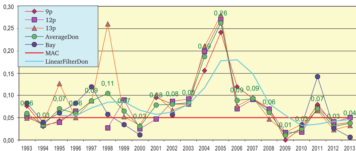
Рис. 3.56. Динамика средней концентрации нефтяных углеводородов (мг/дм³) в протоках дельты реки Дон в 1993–2013 гг.
