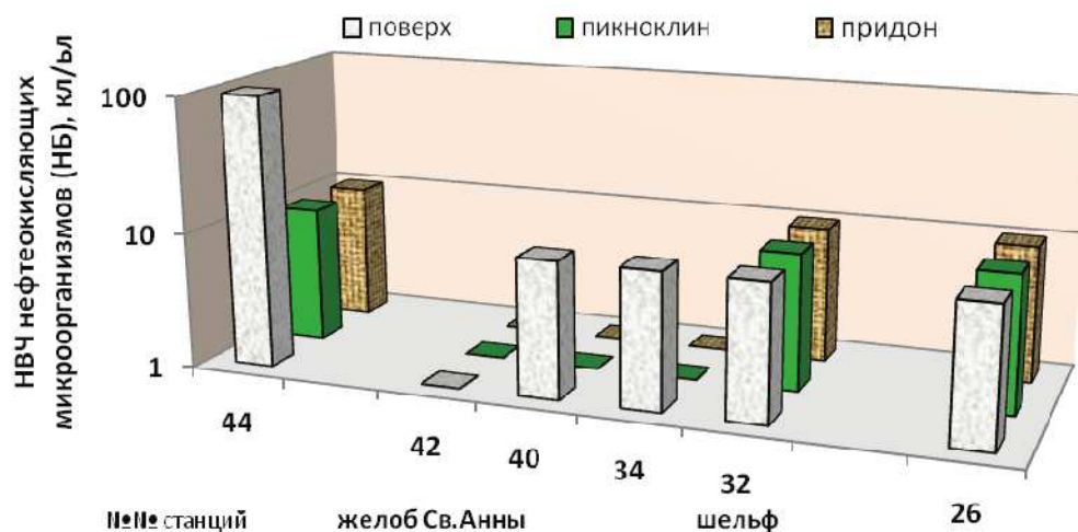
Рис. 3.60. Наиболее вероятная численность микроорганизмов нефтеокисляющих микроорганизмов (НВЧ НБ, кл/мл) в водах северо-западной части Карского моря (2011 г). Районы: ст. 26 – шельф; ст. 32-42 – желоб Св. Анны; ст. 44 – северное побережье Новой Земли
