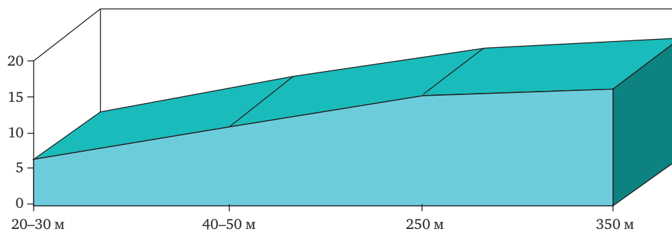
Рис. 4.12. Изменение суммарного показателя покрытия-встречаемости лишайников на липах при удалении от метрополитана (Воробьевская набережная)
