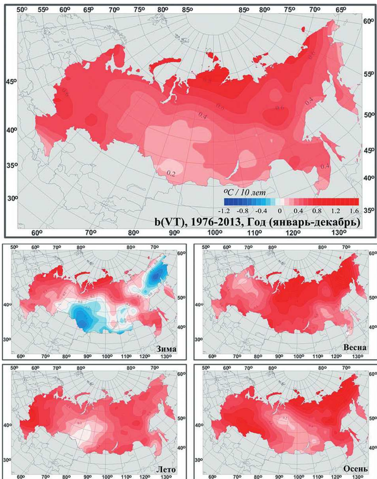
Рис. 1.10. Распределение коэффициентов линейного тренда среднегодовой и средних сезонных значений температуры приземного воздуха на территории РФ за период 1976–2013 гг. (в °C/10 лет)
