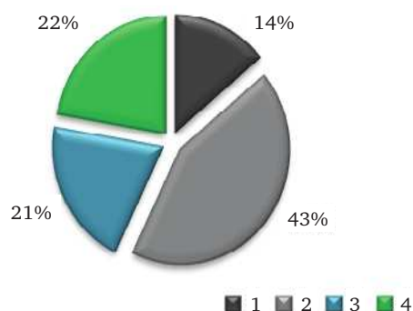
Рис. 3.14. Количество городов (%), где ИЗА ≥ 14 (1), 7–13 (2), 5–6 (3), ≤ 5 (4)
