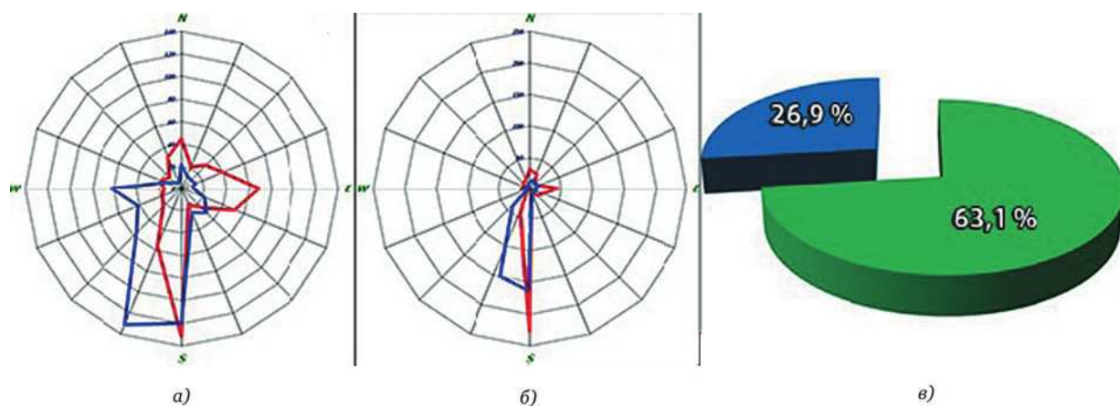
Рис. 4.27. Векторная диаграмма направлений атмосферного переноса, 2010 – 2011 гг. (красная линия), 2012–2013 гг. (синяя линия): а – для средних значений концентрации ЭГР; б – для случаев AMDEs ( < 1 \text{ нг/м}^3 ); в – круговая диаграмма, вклад случаев AMDEs – 26,9% (синий сектор), вклад средних значений – 63,1%
