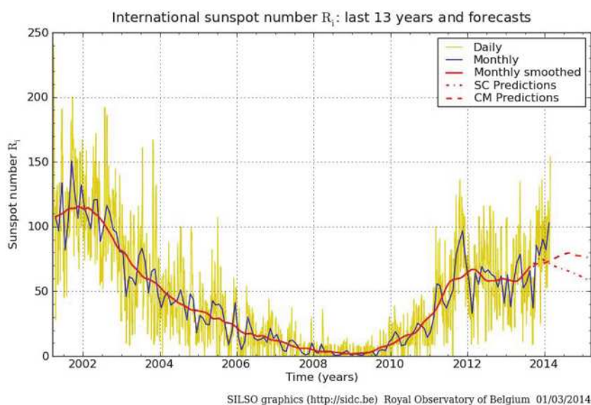
Рис. 1.2. График изменения среднемесячных значений чисел Вольфа
