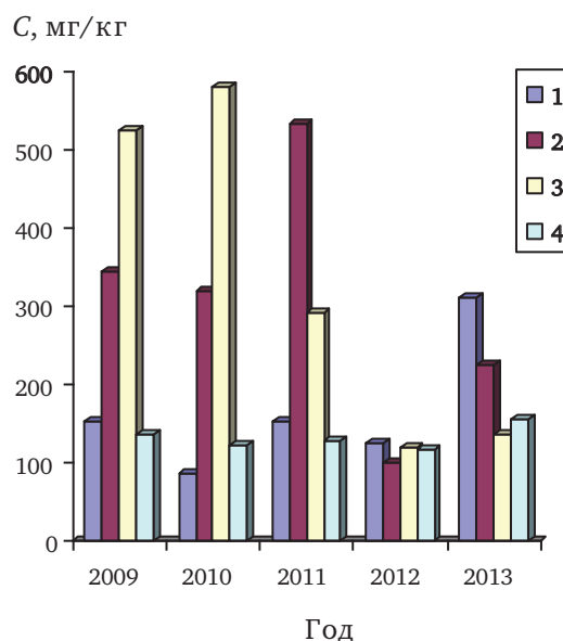
Рис. 3.22. Динамика средних массовых долей НП в поверхностном слое почв ПМН в городах Кемерово (1), Набережные Челны (2), Нижнекамск (3), Новокузнецк(4)
