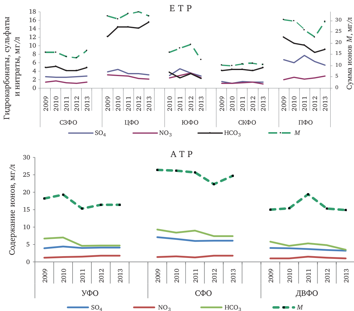
Рис. 2.27. Ход изменения со временем по ФО суммы ионов M , сульфатов SO_4^{2-} , гидрокарбонатов HCO_3^- и нитратов NO_3^- (ЕТР и АТР)
