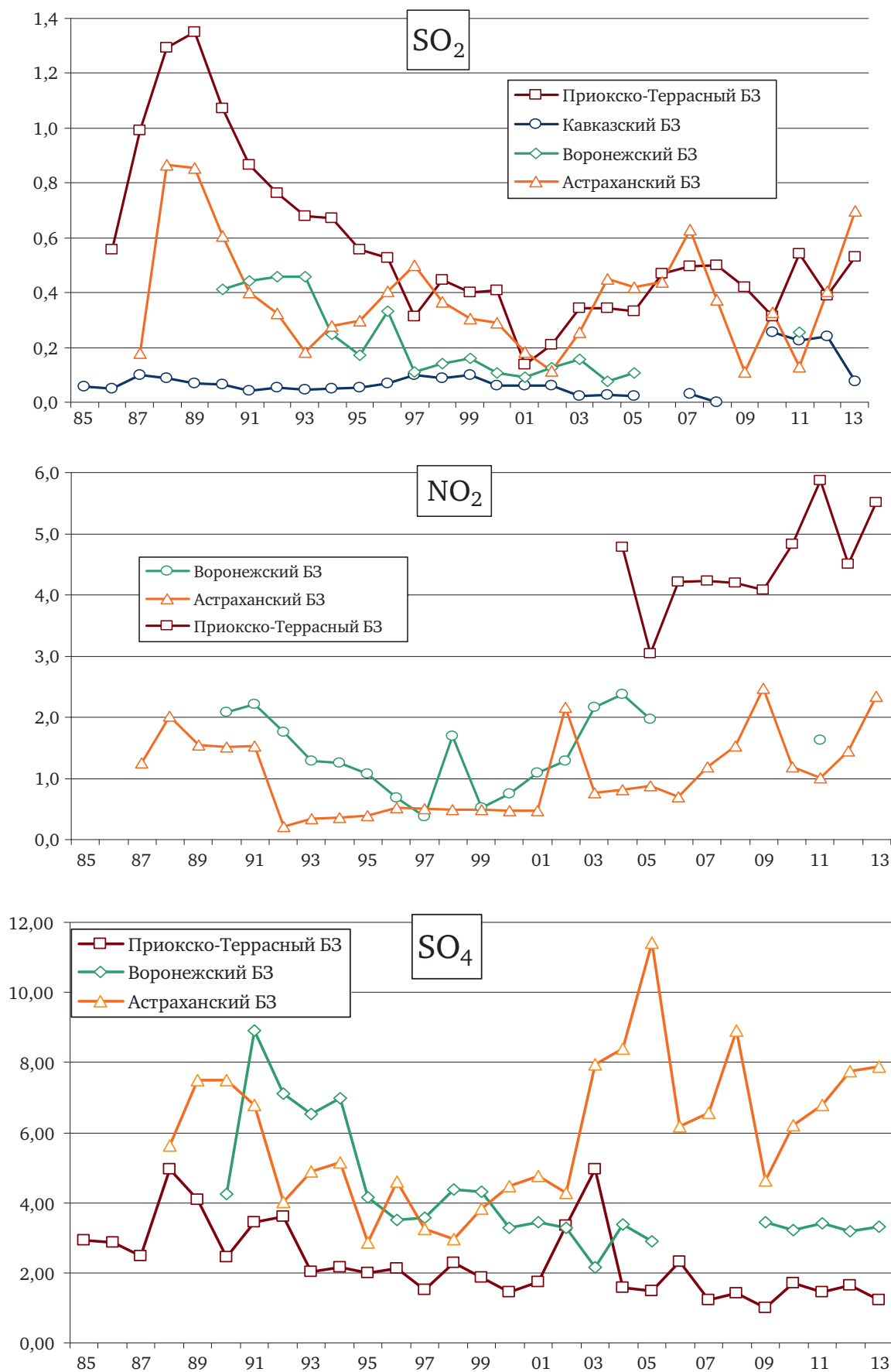
Рис. 2.23. Изменение фоновое содержания диоксида серы, диоксида азота и сульфатов в атмосферном воздухе фоновых районов (мкг/м 3 )
