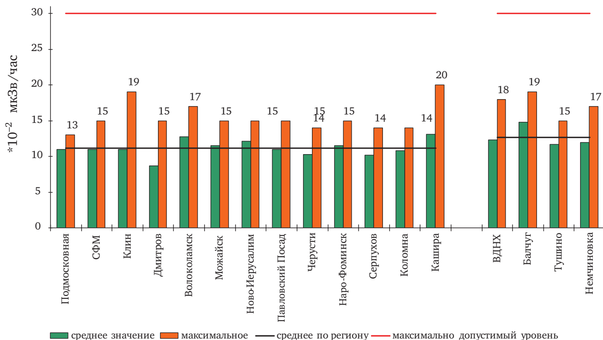
Рис. 4.11. Мощность экспозиционной дозы (МЭД) на станциях Московского региона в 2013 г.
