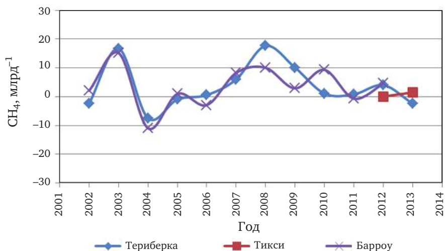
Рис. 2.8. Межгодовой рост концентрации \text{CH}_4
