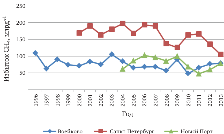
Рис. 2.9. Среднегодовое превышение концентрации \text{CH}_4 над фоновым уровнем
