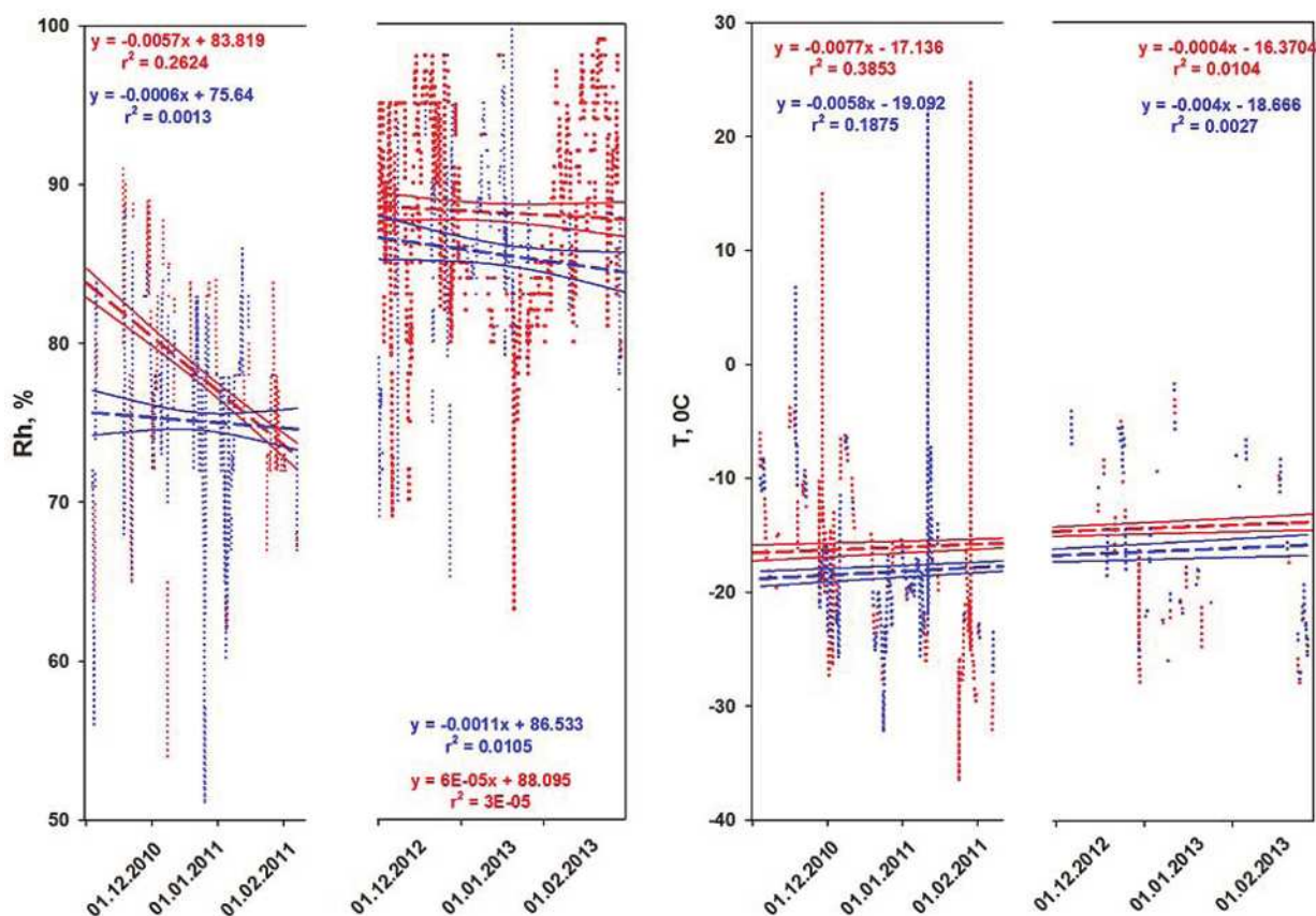
Рис. 4.25. Временной ряд значений относительной влажности и температуры в приземном слое атмосферы для зимних периодов с 2011 г. по 2013 г. как в случае регистрации AMDEs (синий) так и в случае отсутствия AMDEs (красный) ( C_{Hg} > 1,0 \text{ нг/м}^3 ); линейная аппроксимация тренда (синяя штриховая линия) для случаев AMDEs и (красная штриховая линия) для случаев, когда отсутствовали AMDEs
