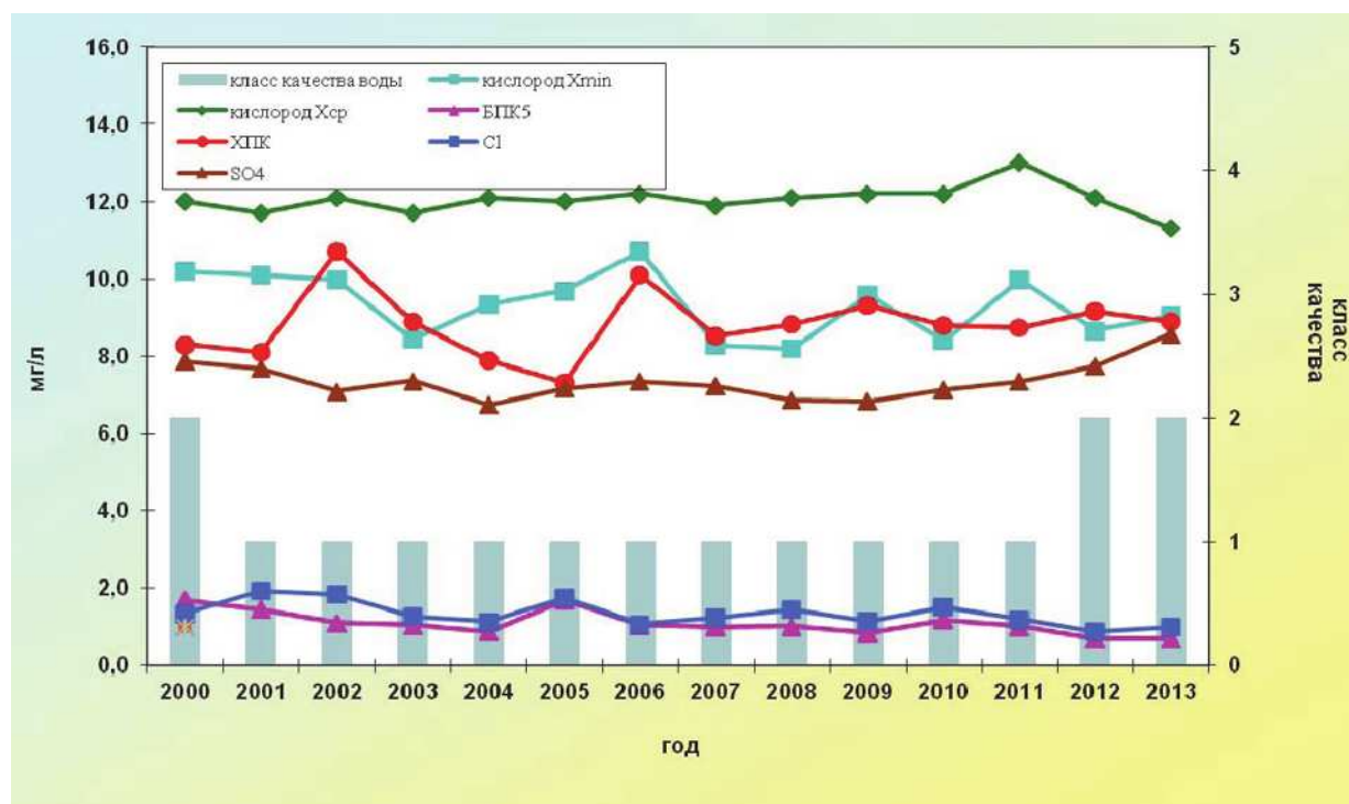
Рис. 2.54. Изменение класса качества и среднегодовых концентраций отдельных ингредиентов и показателей качества воды Иркутского водохранилища, ОГП-1 Исток Ангары за многолетний период
