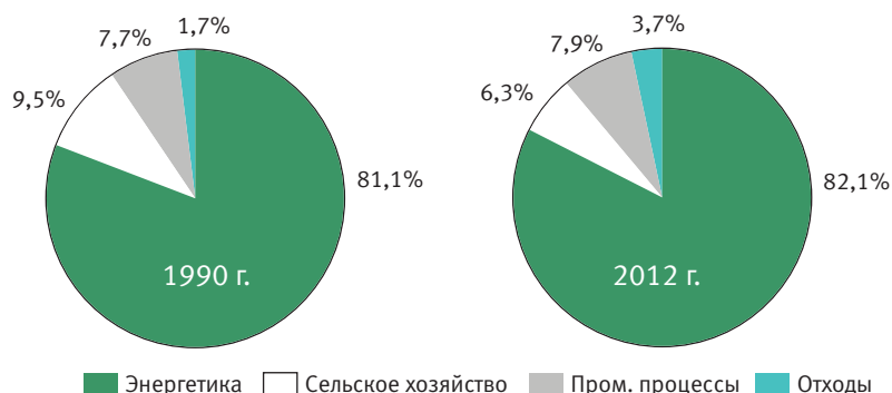
Рис. 2.3. Распределение общего выброса парниковых газов (CO 2 -экв.) по секторам в 1990 и 2012 гг. (без учета сектора «Землепользование, изменение землепользования и лесное хозяйство»)
