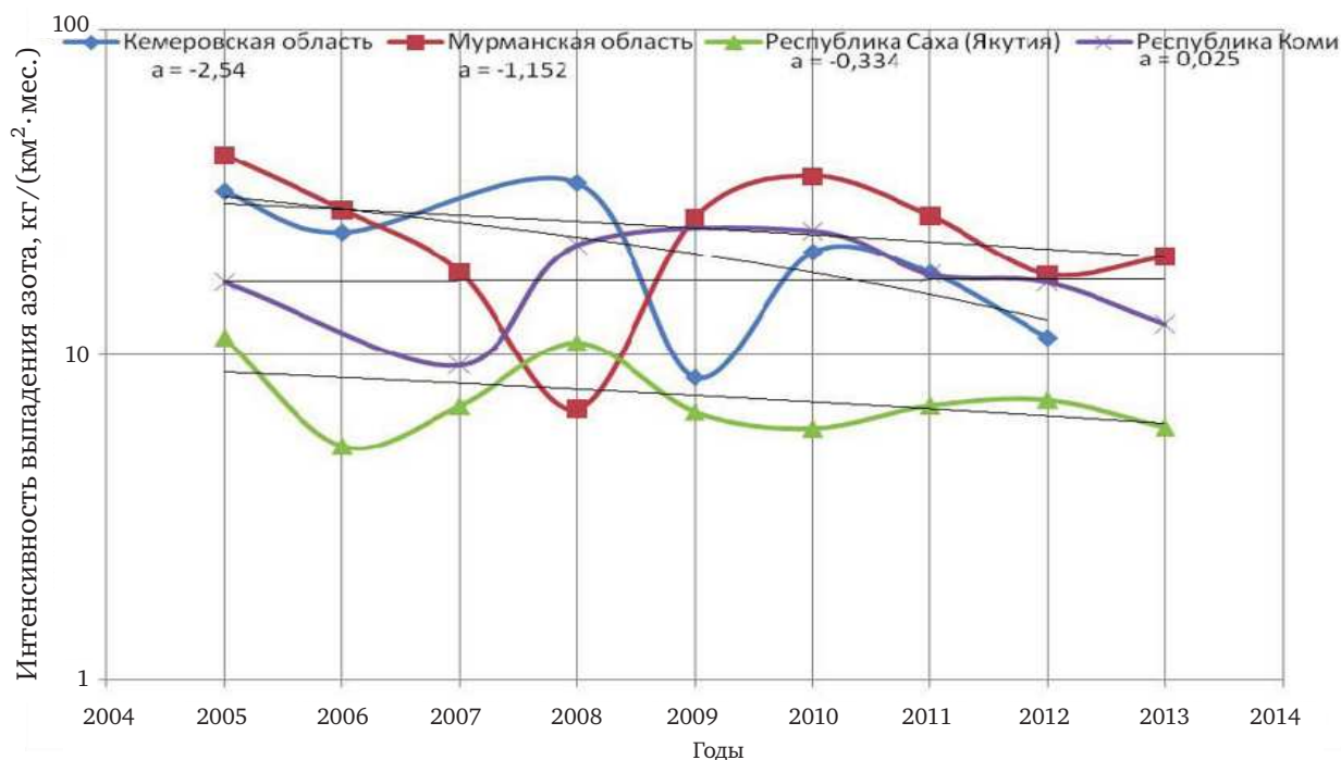
Рис. 2.32. Интенсивность выпадений серы P_S в промышленных и фоновых регионах на ЕТС и АТС по данным мониторинга химического состава снежного покрова в 2005–2013 гг.
