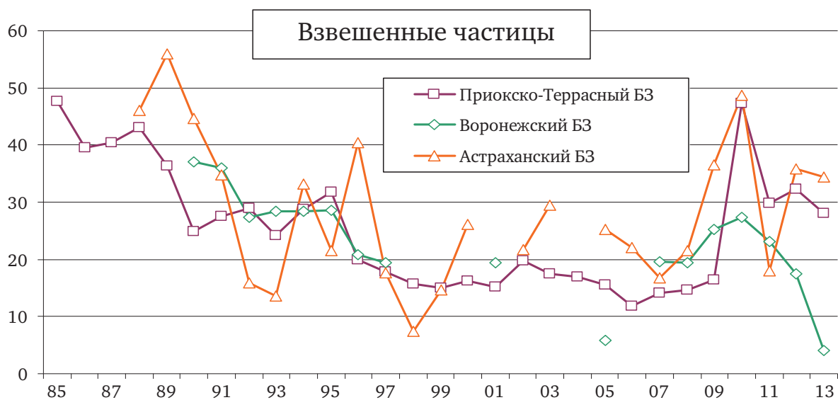
Рис. 2.22. Изменение фоновых содержания свинца ( \text{мкг/м}^3 ), 3,4-бензпирена ( \text{нг/м}^3 ) и взвешенных частиц ( \text{мкг/м}^3 ) в атмосферном воздухе фоновых районов
