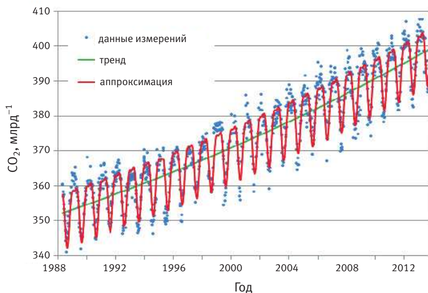
Рис. 2.5. Результаты мониторинга содержания CO 2 на станции Териберка
