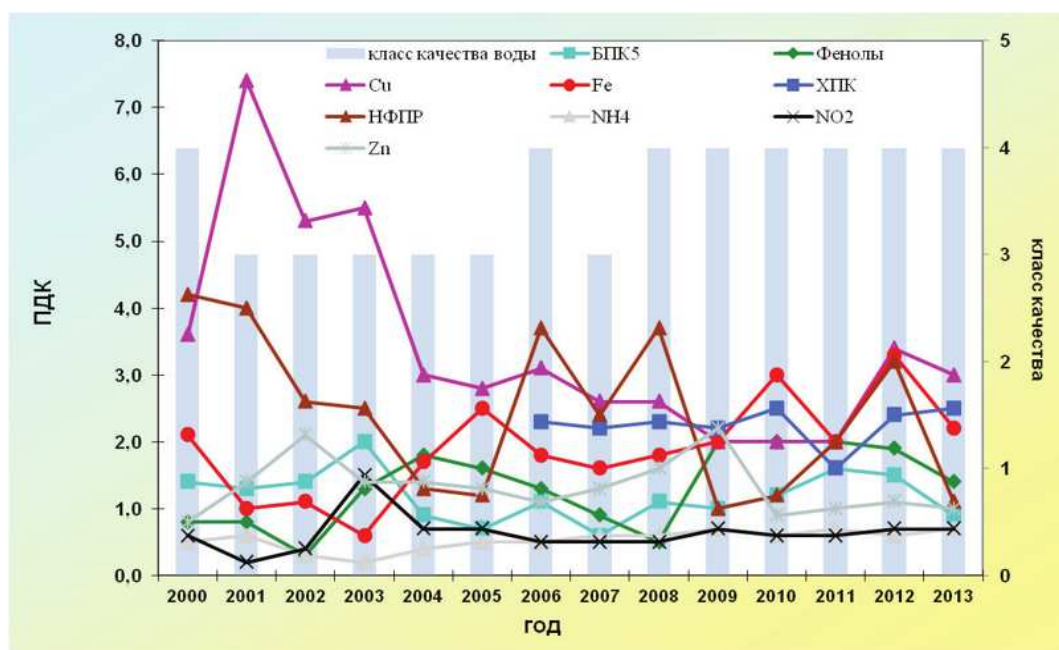
Рис. 3.37. Изменение среднегодовых концентраций отдельных ингредиентов и качества воды Верхне-Волжских водохранилищ: з – Горьковское вдхр., г. Тутаев, 6 км ниже города
