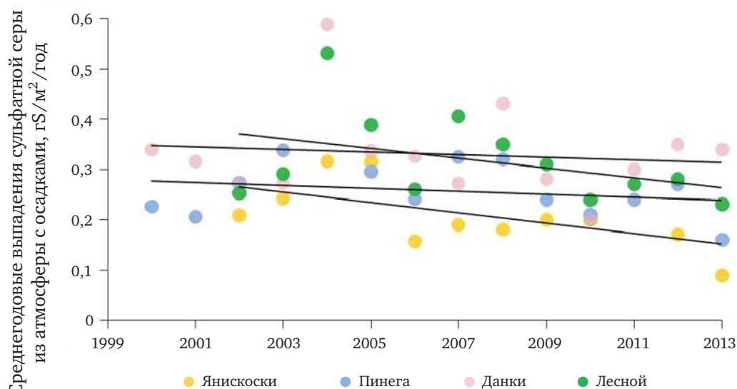
Рис. 2.35. Среднегодовые выпадения сульфатной серы из атмосферы с осадками, гS/м²/год
