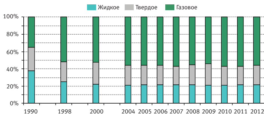
Рис. 2.2. Изменение вклада отдельных видов топлива в выброс CO 2 от сжигания ископаемого топлива (сектор «Энергетика»)
