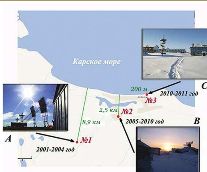
Рис. 4.22. (А) Место установки анализатора с 2001 по 2004 гг., (В) с 2005 по 2010 гг., (С) с 2010 по 2013 гг.
