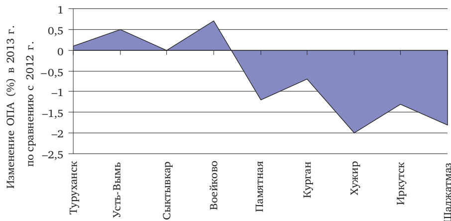
Рис. 2.11. Изменения ОПА на станциях фоновых мониторинга в 2013 г. по сравнению с предыдущим 2012 г.
