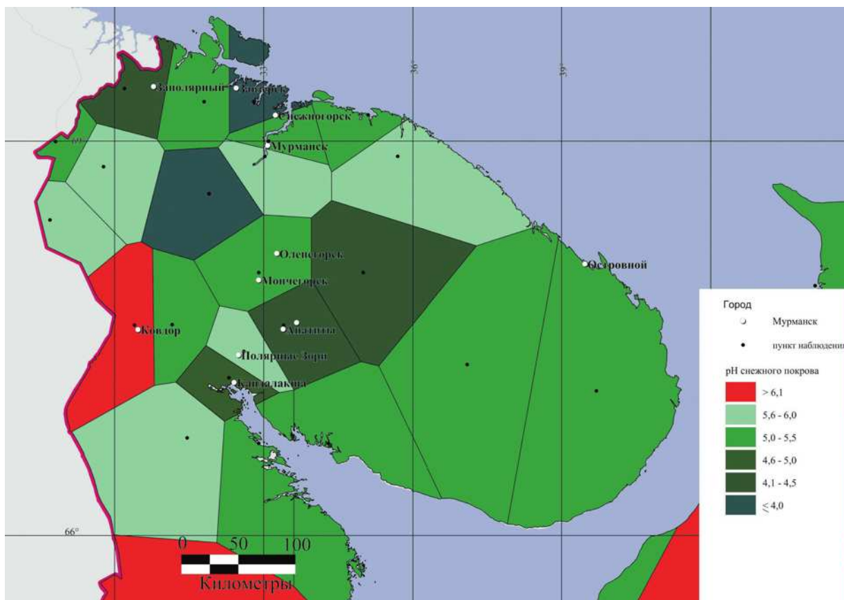
Рис. 2.28. Распределение pH снежного покрова на территории Мурманской области по данным наблюдений в 2013 г. (полигоны Вороного)
