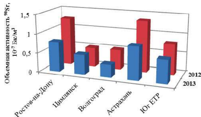
Рис. 2.62. Среднегодовая объемная активность ^{90}\text{Sr} в населенных пунктах ЮФО в 2012–2013 годах, 10^{-7} \text{ Бк/м}^3
