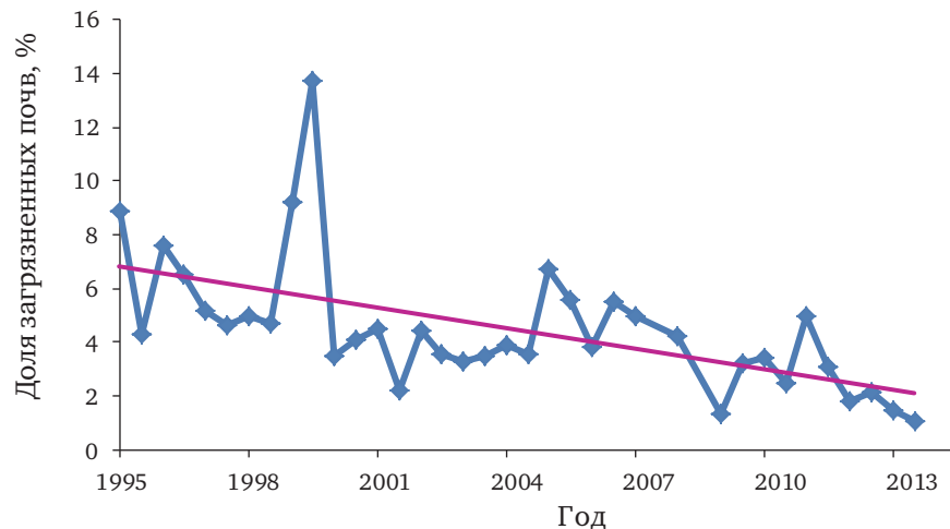
Рис. 3.24. Доля загрязненных почв, % от обследованной площади
