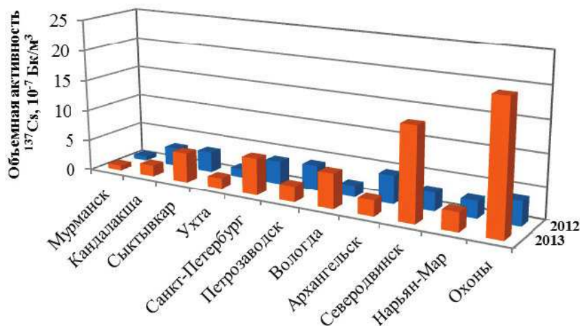
Рис. 2.60. Среднегодовая объемная активность ^{137}\text{Cs} в населенных пунктах СЗФО в 2012–2013 годах, 10^{-7} Бк/м 3
