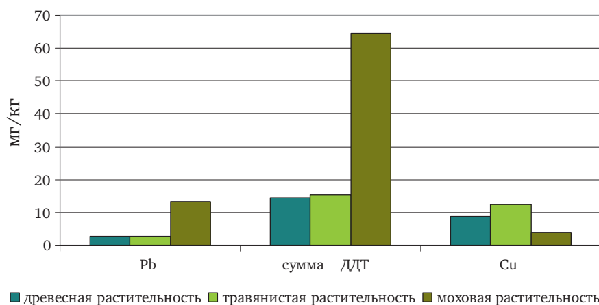
Рис. 2.45. Среднее содержание загрязняющих веществ в растительности древесного, травянистого и мохового ярусов станций комплексного фоновой мониторинга в 2013 г.
