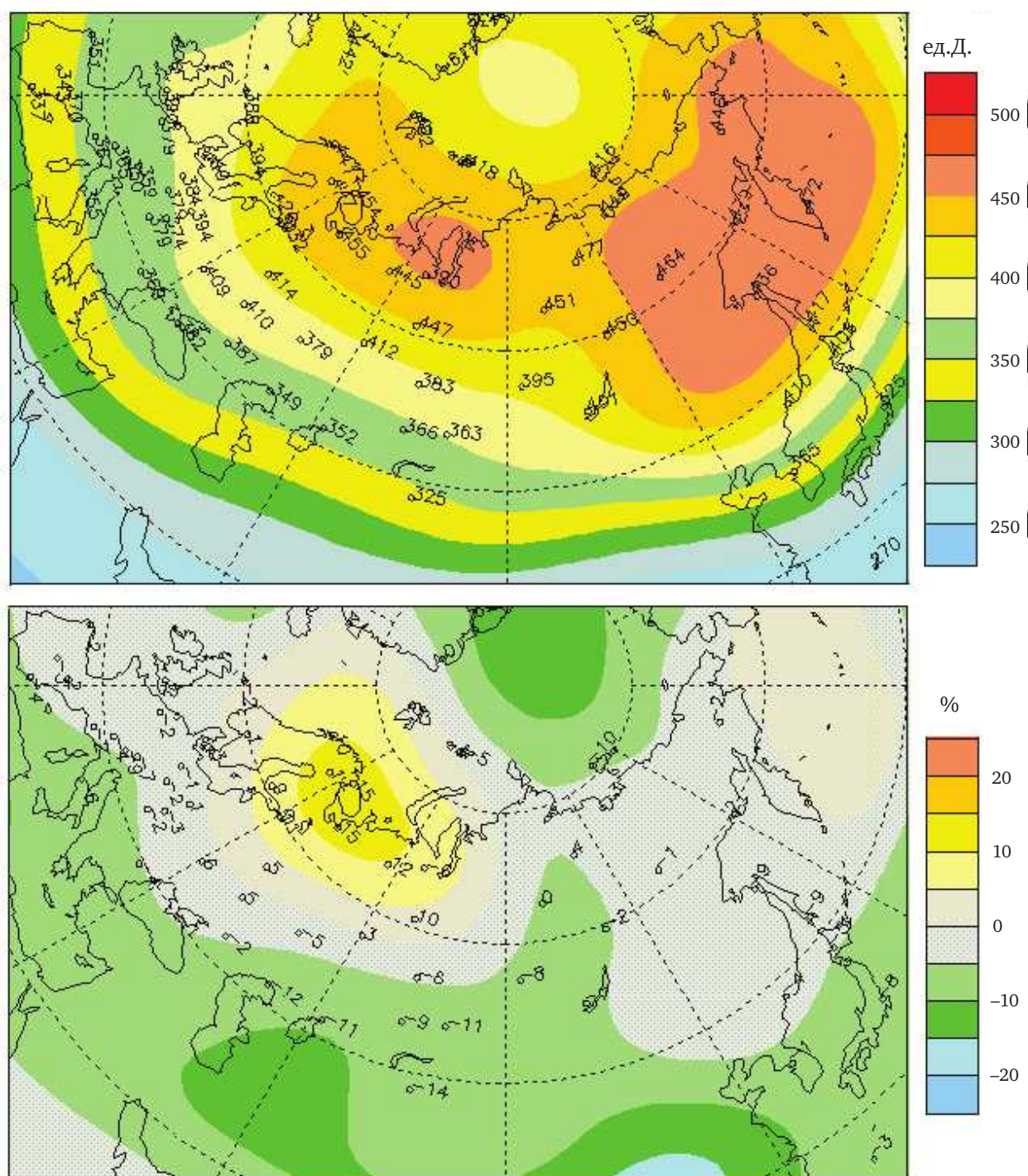
Рис. 2.19. Поле общего содержания озона (ед.Д.; верху) в марте 2013 г. и его отклонения (%) в от средних многолетних (1978–1988 гг.) значений по данным WUODC, Канада
