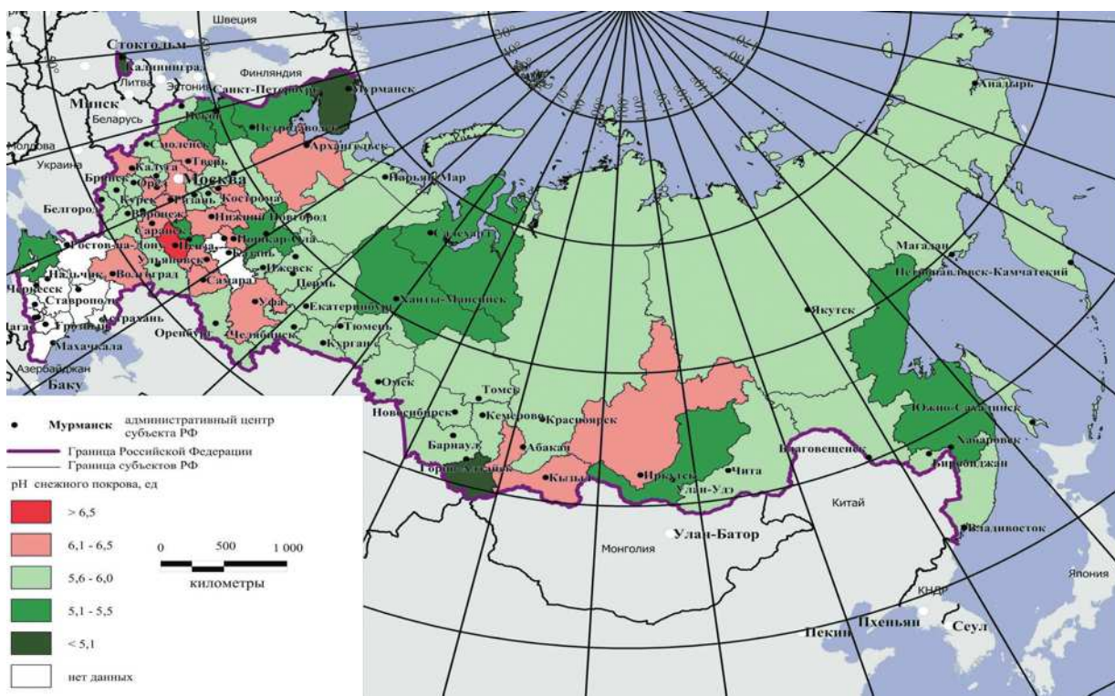
Рис. 2.29. Средние показатели кислотности pH снежного покрова в регионах РФ по данным мониторинга в 2013 г.
