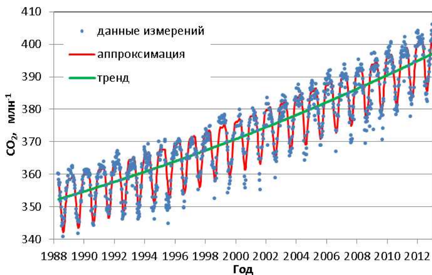
Рис. 2.5. Результаты наблюдений за содержанием \text{CO}_2 на станции Териберка
