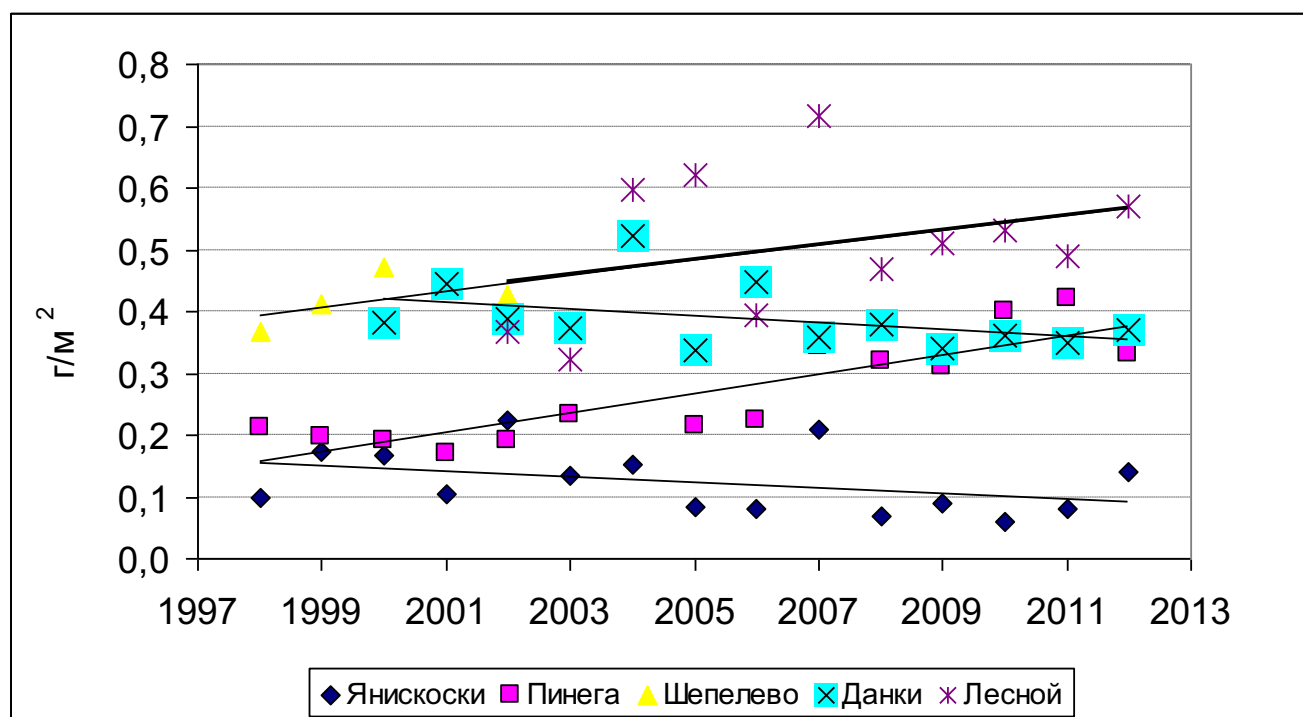
Рис. 2.35. Среднегодовые выпадения суммы нитратного и аммонийного азота из атмосферы с осадками, г N/m^2/год
