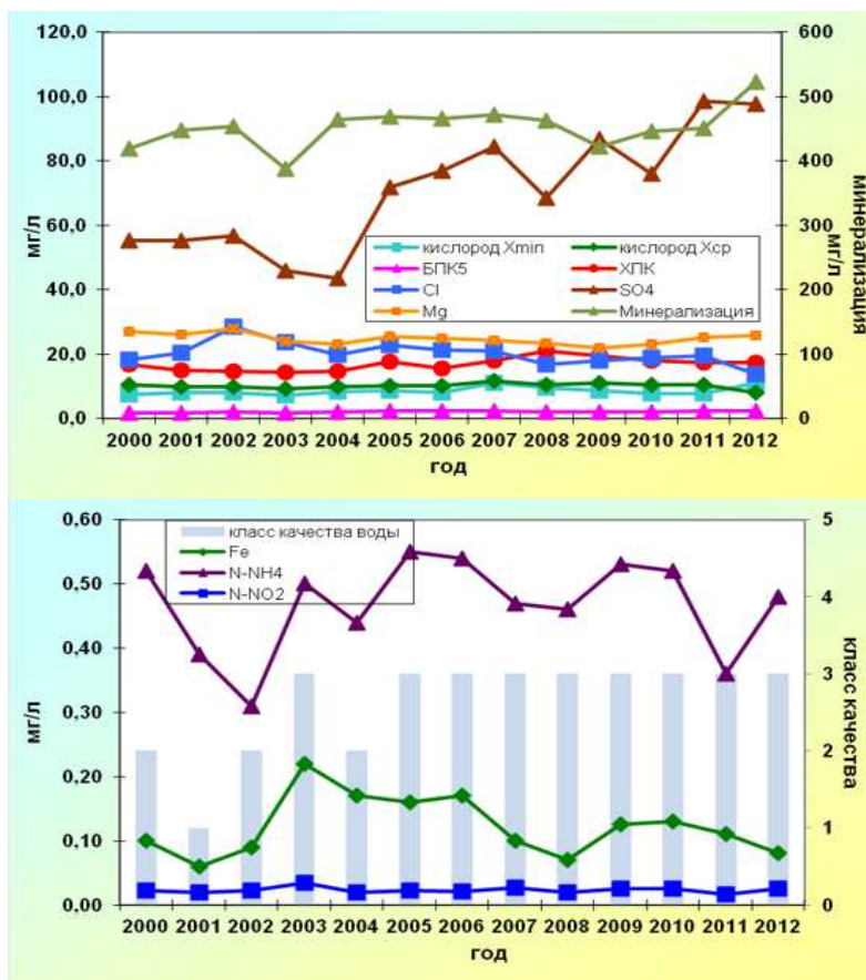
Рис. 2.48. Изменение среднегодовых концентраций основных ингредиентов и качества воды верхнего течения р. Дон в районе г. Данков
