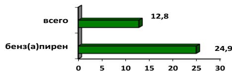
Рис. 3.19. Число жителей в городах (млн.), находящихся под воздействием максимальных концентраций примесей в воздухе выше 10 ПДК (всего) и 5 ПДК бенз(а)пирена
