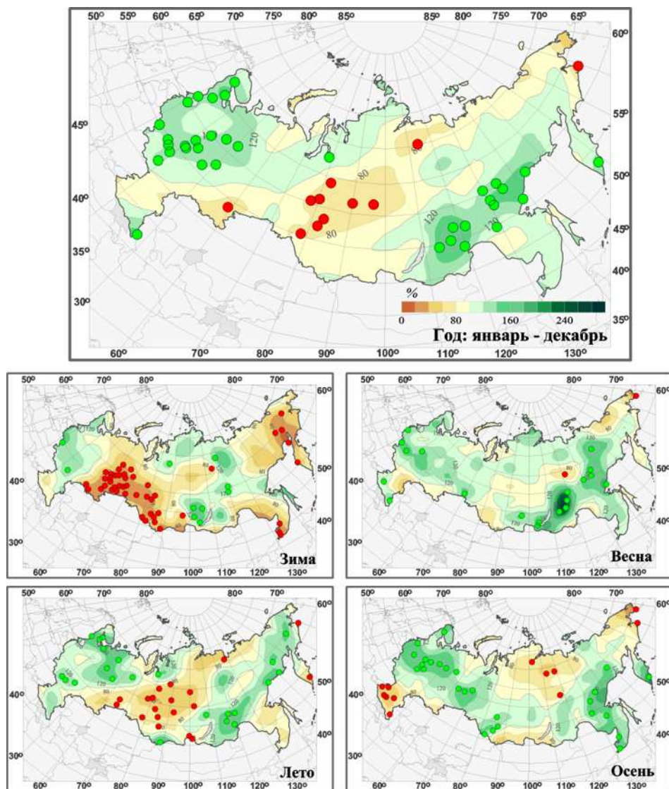
Рис. 1.10. Аномалии годовых и сезонных сумм осадков на территории России в 2012 г. (% от нормы 1961-1990 гг.). Кругами красного и зеленого цвета показаны станции, на которых осадки оказались соответственно ниже 5-го или выше 95-го процентиля.
