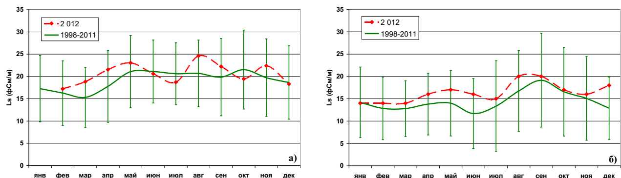
Рис. 2.15. Годовой ход L_s по станциям (а) Воейково, (б) Иркутск в 2012 г. по сравнению с осредненными значениями за предшествующий 15-летний период наблюдений. Вертикальными отрезками обозначен доверительный интервал ( \pm \sigma ) относительно среднего значения для периода с 1998 по 2011 гг.
