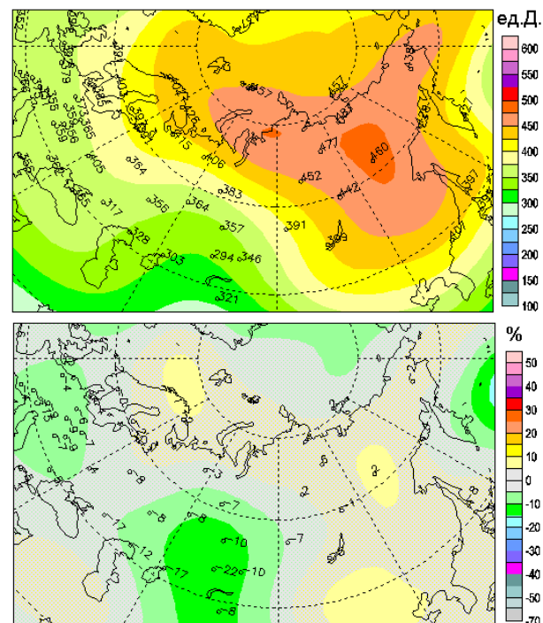
Рис. 2.17. Поле общего содержания озона (ед. Д.; сверху) в апреле 2012 г. и его отклонения (%) от соответствующих средних значений за 1978-1988 гг. по данным WOUDC, Канада
