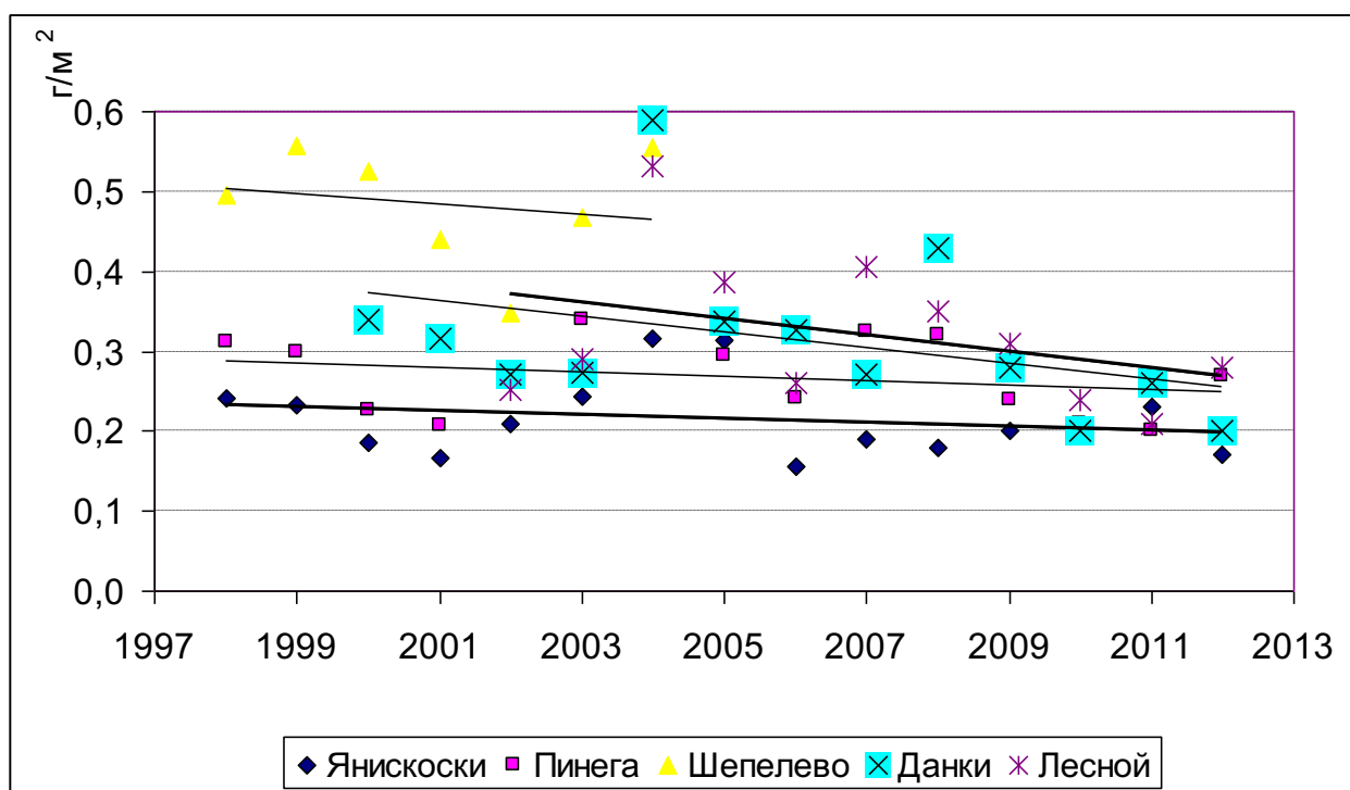
Рис. 2.34. Среднегодовые выпадения сульфатной серы из атмосферы с осадками, г S/m^2/год
