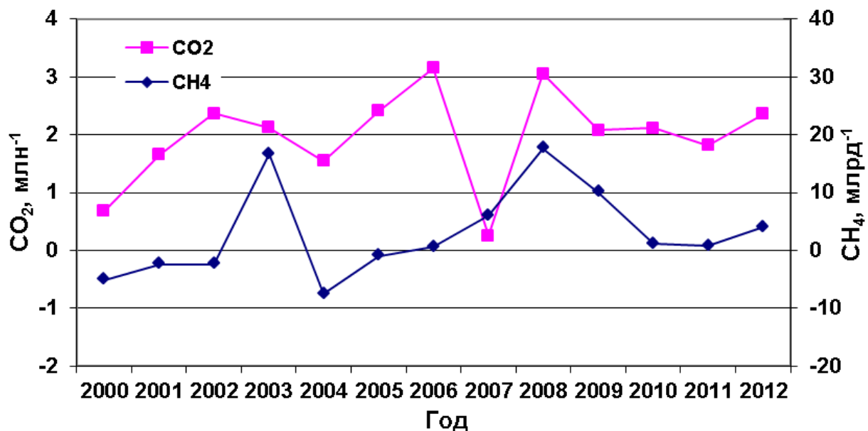
Рис. 2.6. Межгодовой рост концентрации \text{CO}_2 и \text{CH}_4 на станции Териберка
