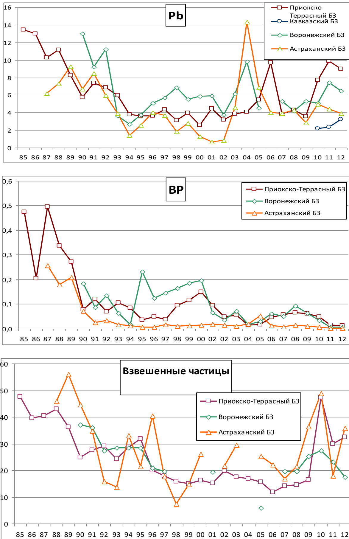
Рис. 2.21. Изменение фоновое содержания свинца ( \text{мкг/м}^3 ), 3,4-бензпирена ( \text{нг/м}^3 ) и взвешенных частиц ( \text{мкг/м}^3 ) в атмосферном воздухе фоновых районов
