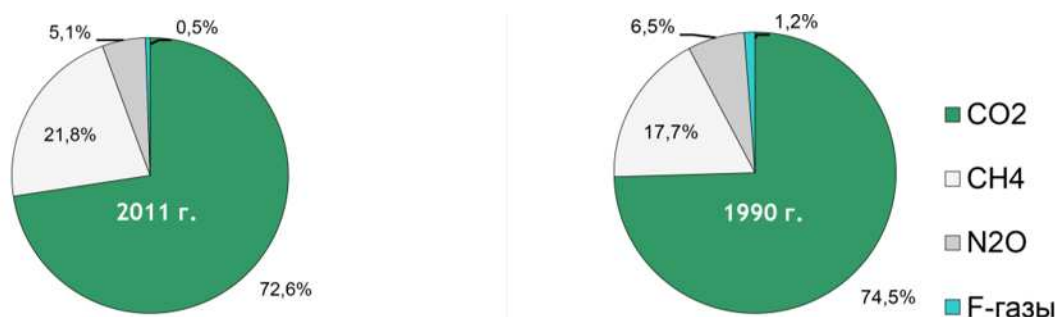
Рис. 2.4. Доля отдельных парниковых газов в их общем выбросе (CO 2 - экв.) в 1990 и 2011 гг. (без учета сектора «Землепользование, изменение землепользования и лесное хозяйство»)
