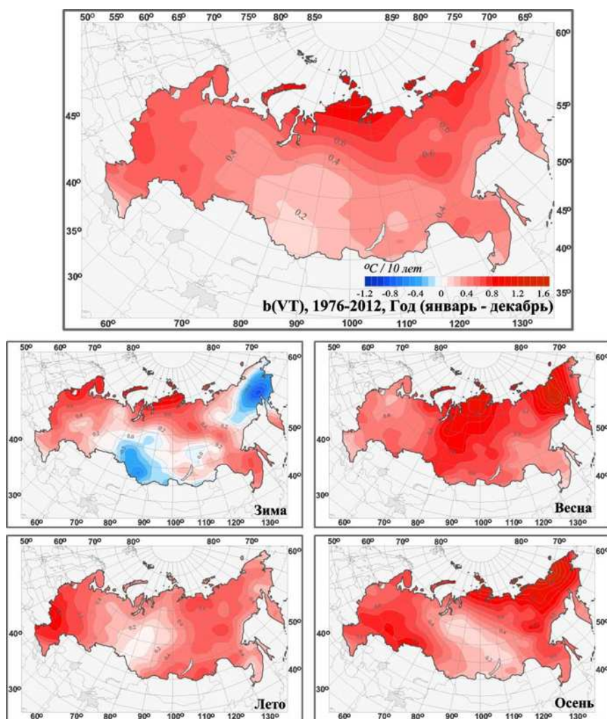
Рис. 1.8. Распределение коэффициентов линейного тренда среднегодовой и средних сезонных значений температуры приземного воздуха на территории России за период 1976-2012 гг. (в ^{\circ}\text{C}/10 лет)
