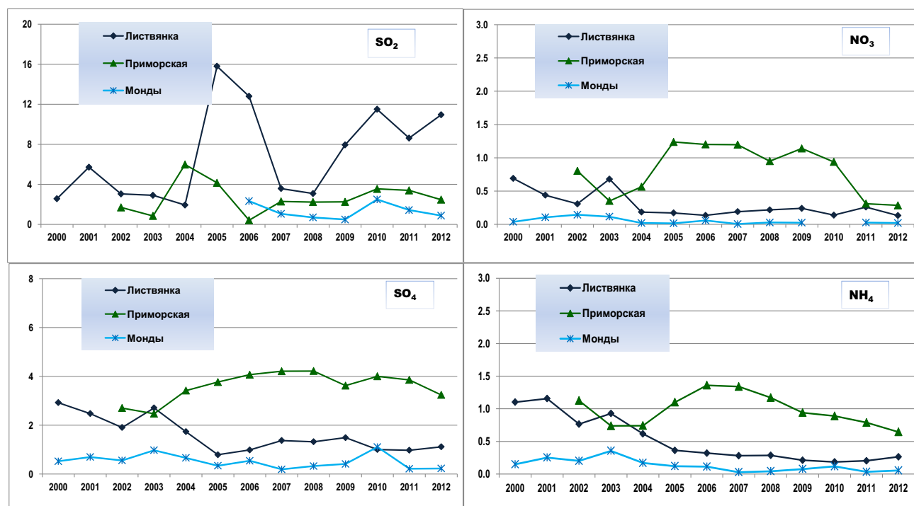
Рис. 2.38. Изменения средних годовых концентрации соединений серы (слева) и азота (справа) в воздухе на станциях ЕАНЕТ (мкг/м 3 )
