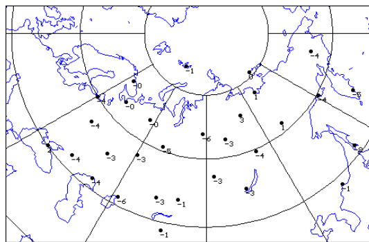
Рис. 2.16. Поле отклонений (%) общего содержания озона в 2012 г. от средних многолетних значений по данным озонометрической сети СНГ
