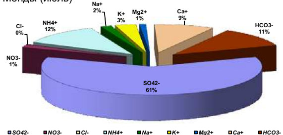
Приморская (июль)
