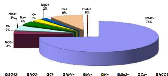
Монды (июль)
