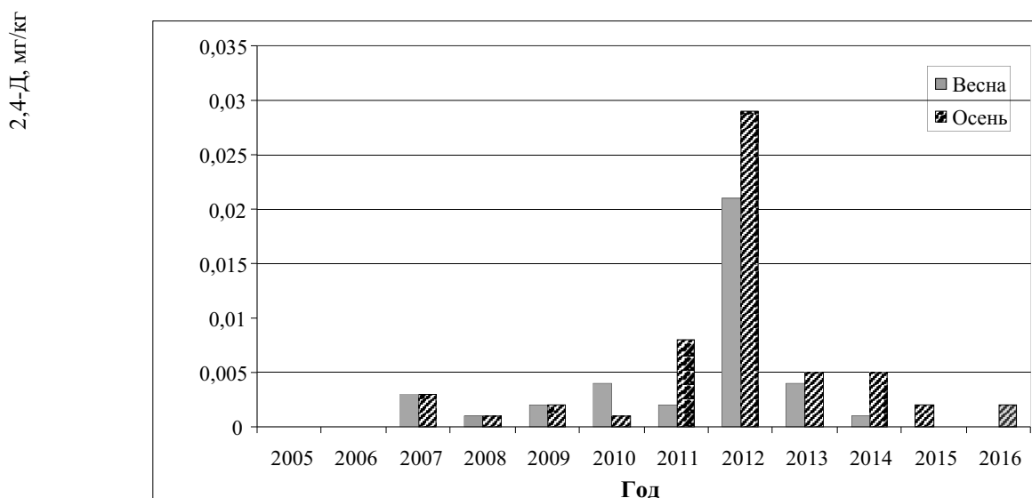
Рис.8. Среднее содержание ОК 2,4-Д в почве сельхозугодий вблизи захоронения ядохимикатов в Лебяжье-вском районе Курганской области
