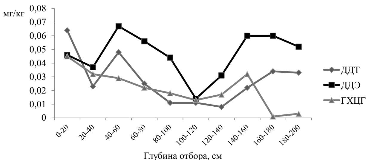
Рис. 4. Содержание хлорорганических пестицидов (мг/кг) в горизонтах почвенного разреза
