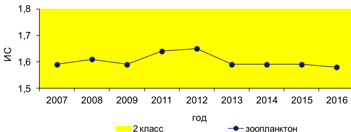
Рисунок 141. Динамика значений ИС в 2007-2016 гг., р.Амур, г.Амурск
