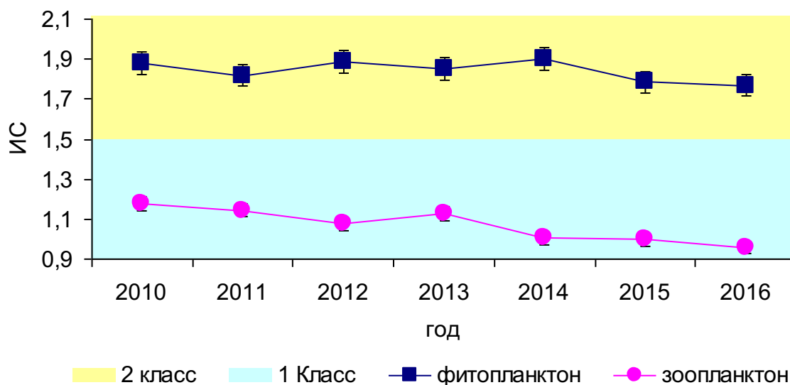
Рисунок 98. Динамика значений ИС в 2010-2016 гг., р. Ангара
