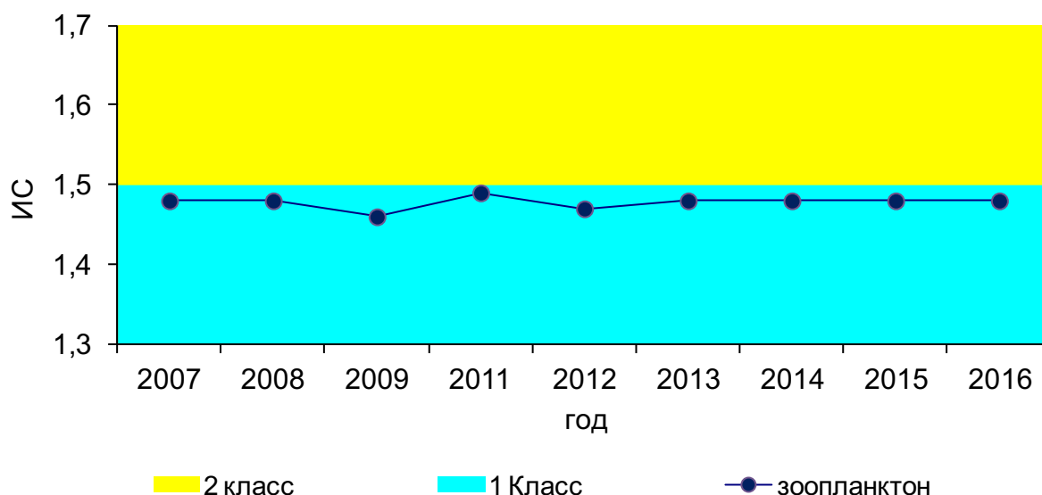
Рисунок 130. Динамика значений ИС в 2007-2016 гг., р.Зея, г. Зея
