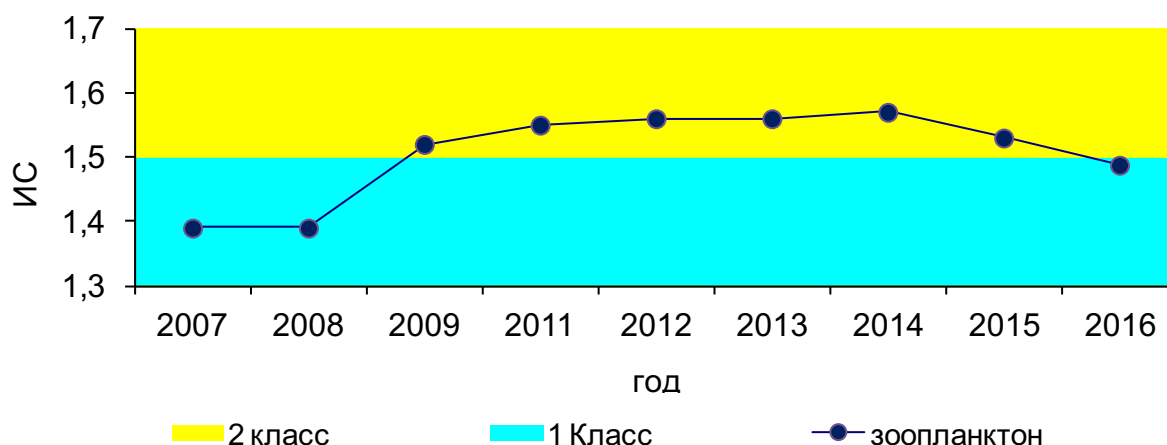
Рисунок 131. Динамика значений ИС в 2007-2016 гг., вдхр. Зейское
