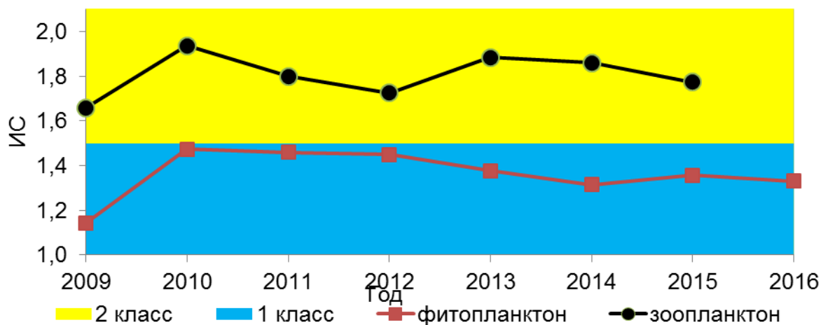
Рисунок 19. Динамика значений ИС в 2009-2016 гг., р. Териберка
