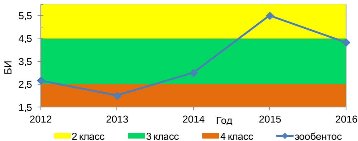
Рисунок 74. Динамика значений БИ в 2012-2016 гг., р. Маныч
