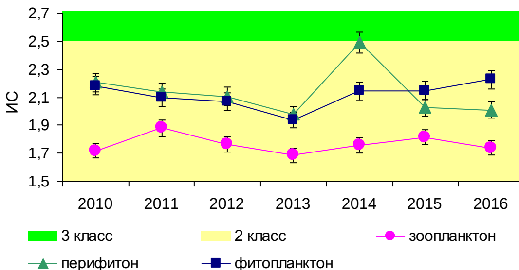
Рисунок 55. Динамика значений ИС в 2010-2016 гг. Куйбышевское вдхр. в р-не г. Тольятти
