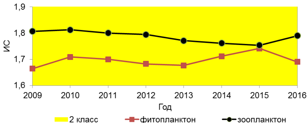
Рисунок 29. Динамика значений ИС в 2009-2016 гг., оз. Имандра
