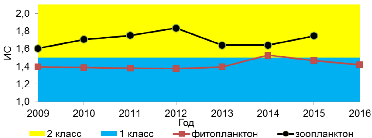
Рисунок 15. Динамика значений ИС в 2009-2016 гг., р. Акким
