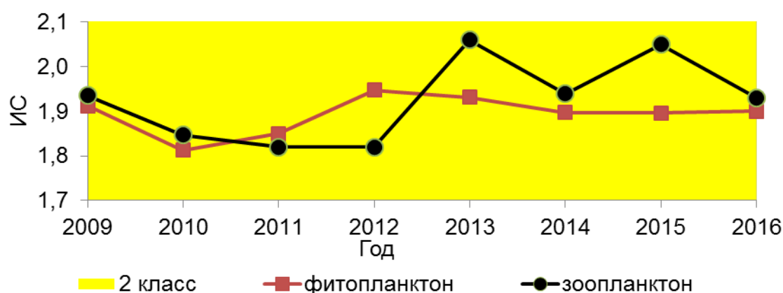
Рисунок 39. Динамика значений ИС в 2009-2016 гг., оз. Семеновское
