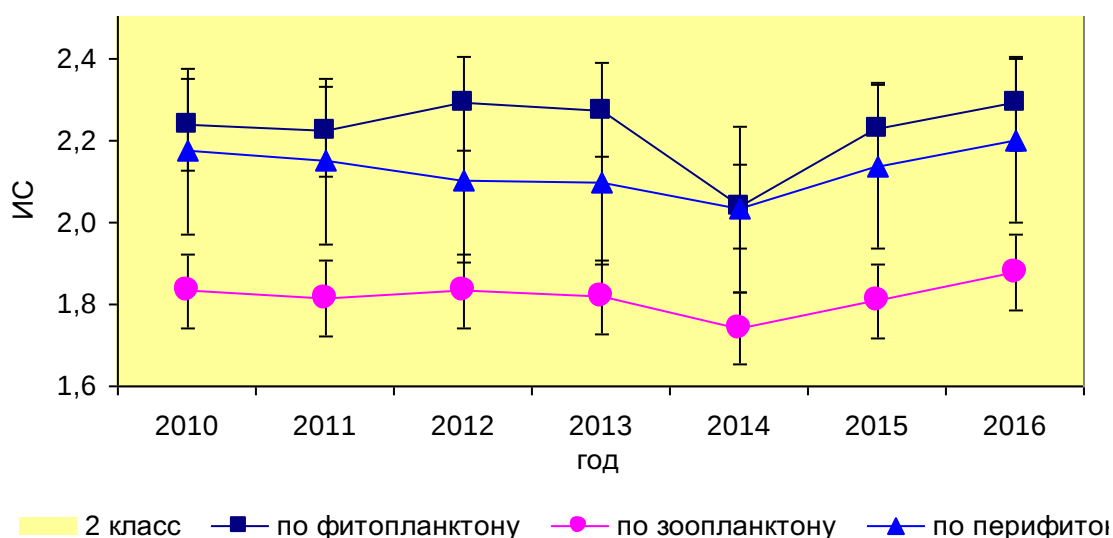
Рисунок 58. Динамика значений ИС в 2010-2016 гг. Саратовское вдхр., г. Сызрань
