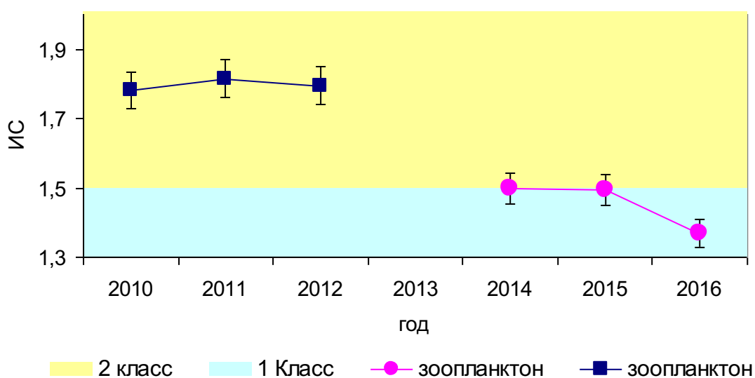
Рисунок 102. Динамика значений ИС в 2010-2016 гг., р. Белая
