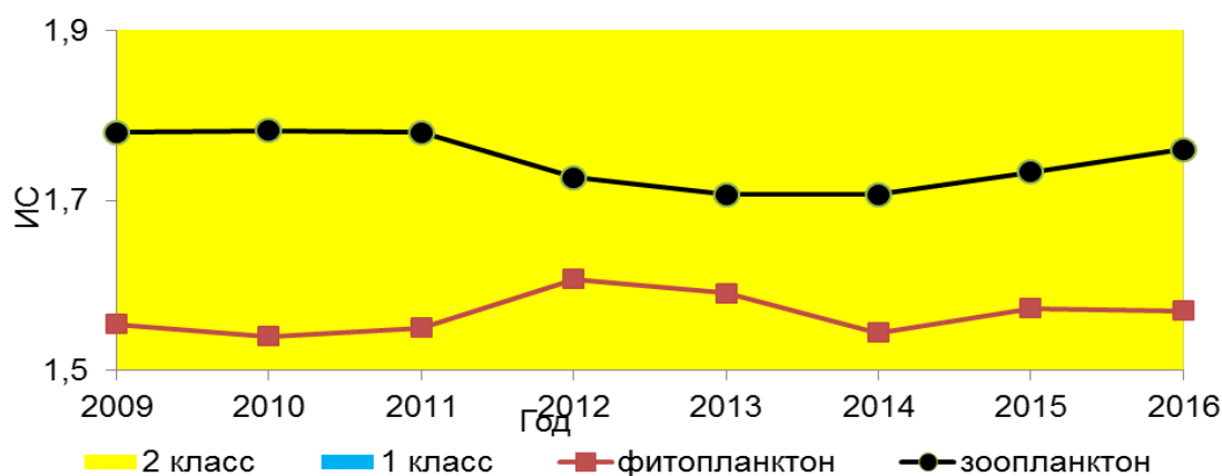
Рисунок 17. Динамика значений ИС в 2009-2016 гг., р. Кола
