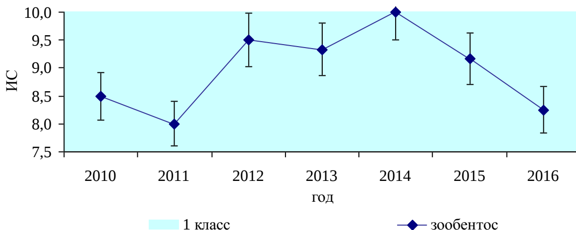
Рисунок 101. Динамика значений БИ в 2010-2016 гг., р. Куда
