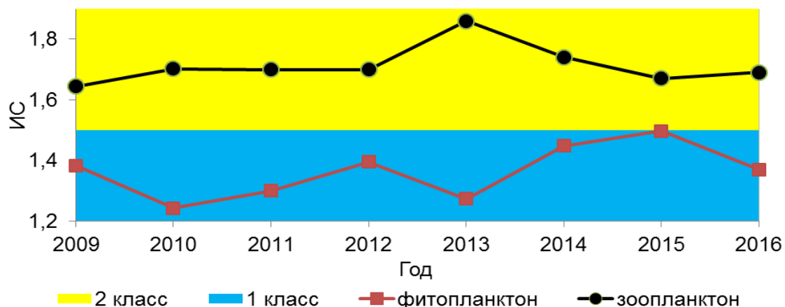
Рисунок 26. Динамика значений ИС в 2009-2016 гг., оз. Умбозеро
