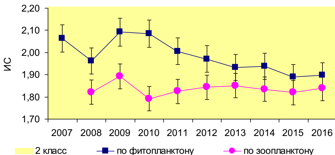
Рисунок 47. Динамика значений ИС за период 2007-2016 гг. Горьковское вдхр.
