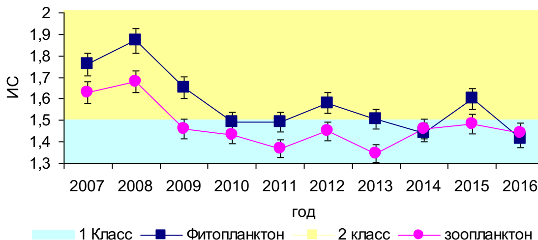
Рисунок 115. Динамика значений ИС в 2007-2016 гг. р. Джида
