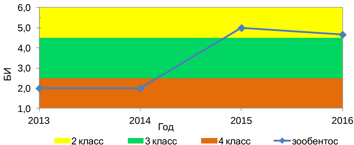
Рисунок 79. Динамика значений БИ в 2012-2016 гг., р. Калитва
