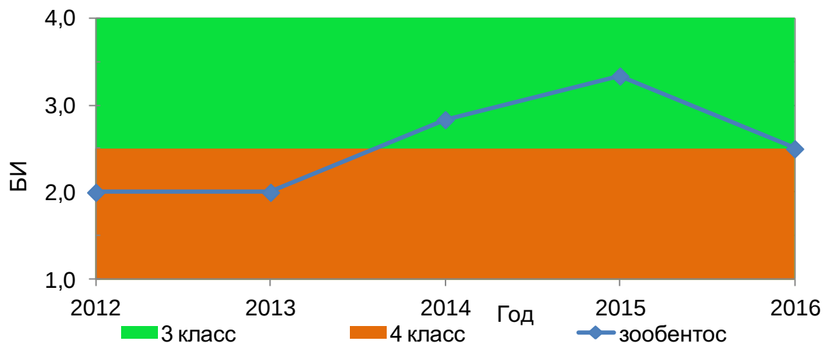
Рисунок 77. Динамика значений БИ в 2012-2016 гг., р. Дон, г. Ростов-на-Дону
