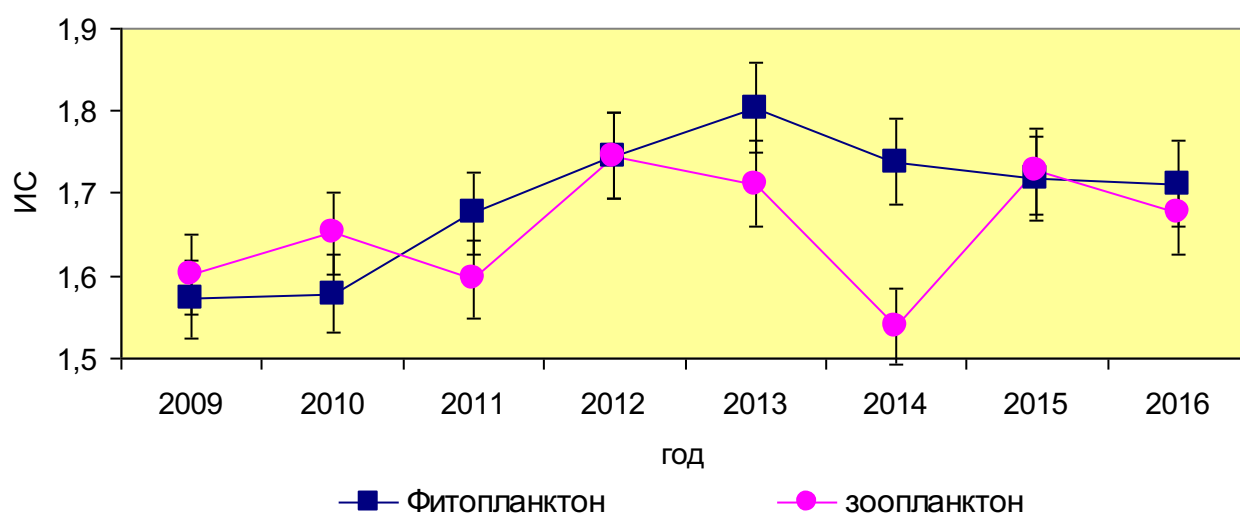
Рисунок 88. Динамика значений ИС в 2009-2016 р. Селенга
