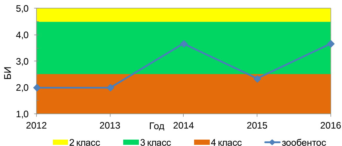
Рисунок 75. Динамика значений БИ в 2012-2016 гг., Пролетарское водохранилище
