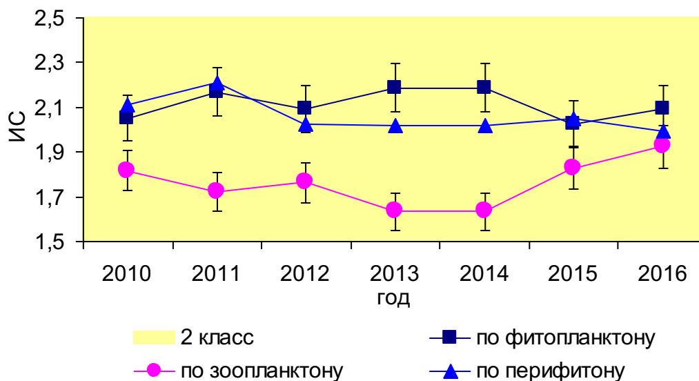
Рисунок 60. Динамика значений ИС в 2010-2016 гг. Саратовское вдхр., г. Балаково
