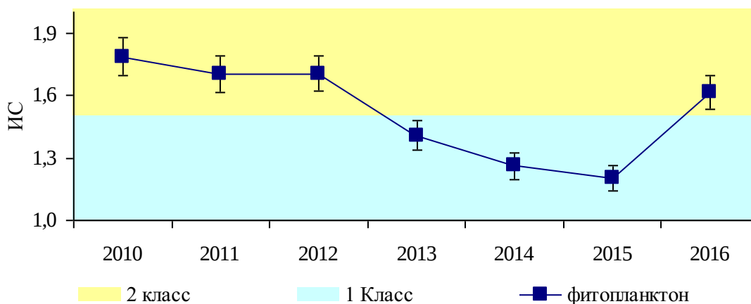
Рисунок 108. Динамика значений БИ в 2010-2016 гг., р.Ушаковка
