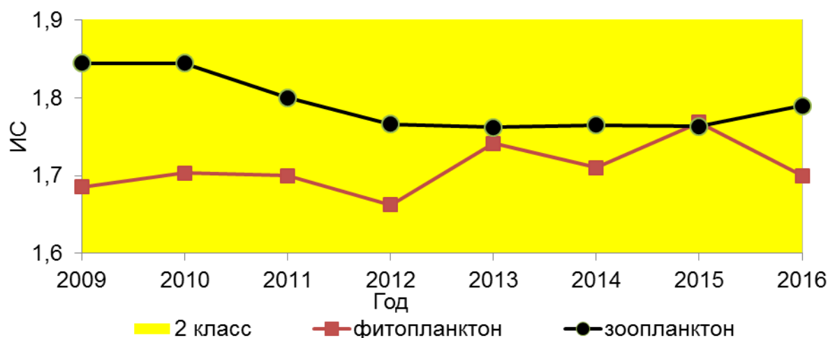
Рисунок 25. Динамика значений ИС в 2009-2016 гг., оз. Ловозеро
