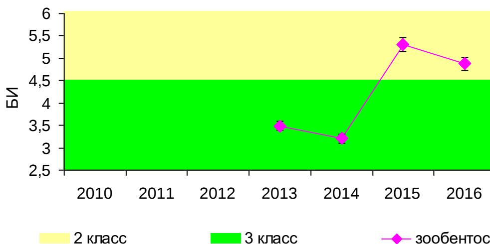
Рисунок 56. Динамика значений БИ в 2010-2016 гг. Куйбышевское вдхр. в р-не г. Тольятти
