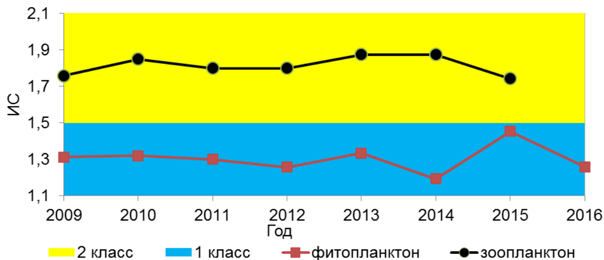
Рисунок 35. Динамика значений ИС в 2009-2016 гг., р. Лотта
