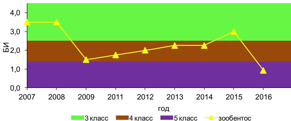
Рисунок 128. Динамика значений БИ в 2007-2016 гг., р.Сита
