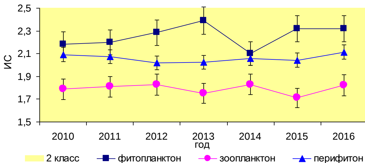
Рисунок 59. Динамика значений ИС в 2010-2015 гг. Саратовское вдхр., г. Хвалы́нск
