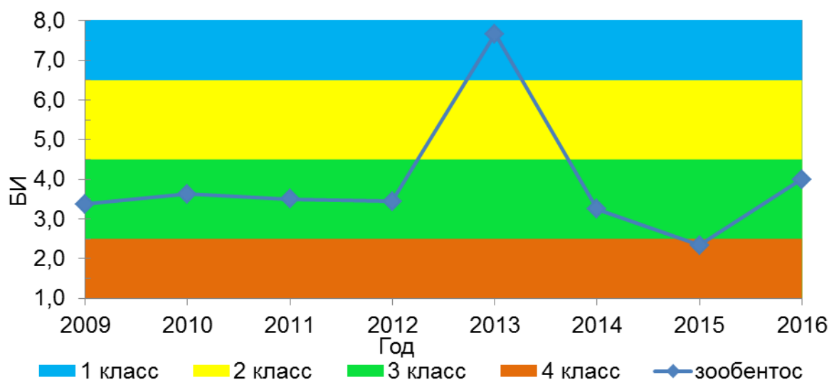
Рисунок 18. Динамика значений БИ в 2009-2016 гг., р. Кола
