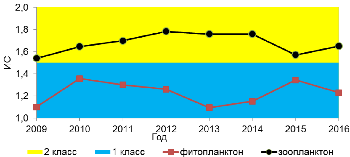
Рисунок 37. Динамика значений ИС в 2009-2016 гг., р. Кица
