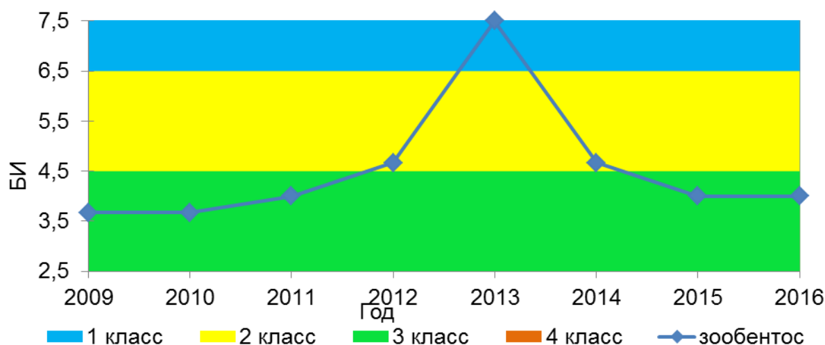
Рисунок 36. Динамика значений БИ в 2009-2016 гг., р. Лотта
