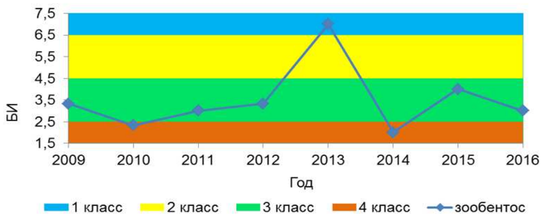
Рисунок 34. Динамика значений БИ в 2009-2016 гг., оз. Чунозеро
