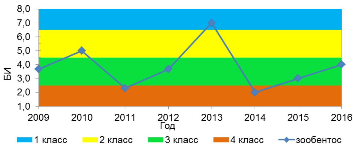
Рисунок 16. Динамика значений БИ в 2009-2016 гг., р. Акким
