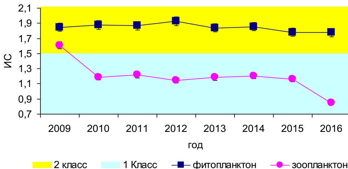
Рисунок 99. Динамика значений БИ в 2010-2016 гг., Братское вдхр.
