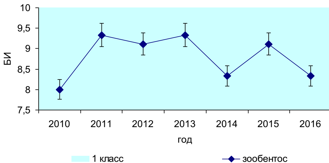
Рисунок 103. Динамика значений БИ в 2010-2016 гг., р. Беляя
