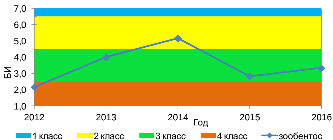
Рисунок 69. Динамика значений БИ в 2012-2016 гг., р. Дон, г. Семикаракорск
