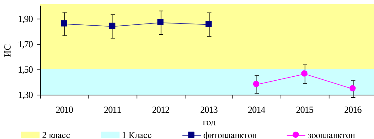
Рисунок 100. Динамика значений ИС в 2010-2016 гг., р. Куда
