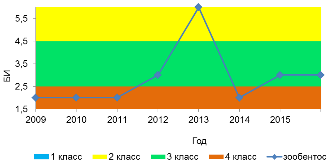
Рисунок 8. Динамика значений БИ в 2009-2016 гг., протока Сальми-ярви
