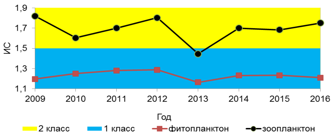
Рисунок 33. Динамика значений ИС в 2009-2016 гг., оз. Чунозеро
