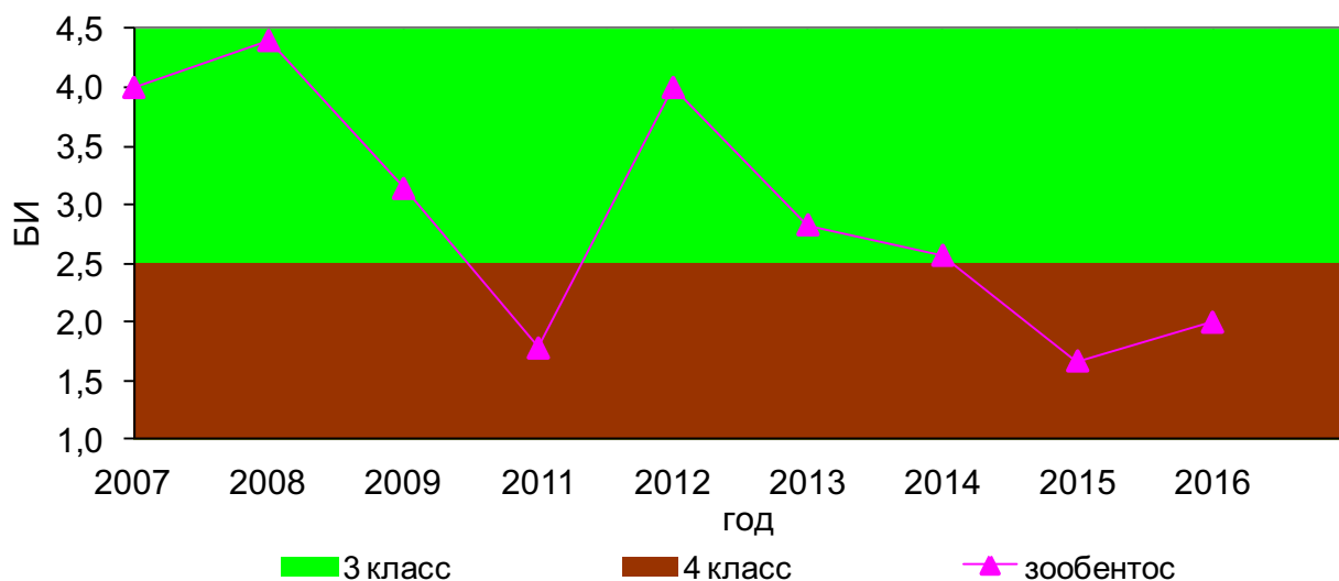
Рисунок 124. Динамика значений БИ в 2007-2016 гг., р. Хор
