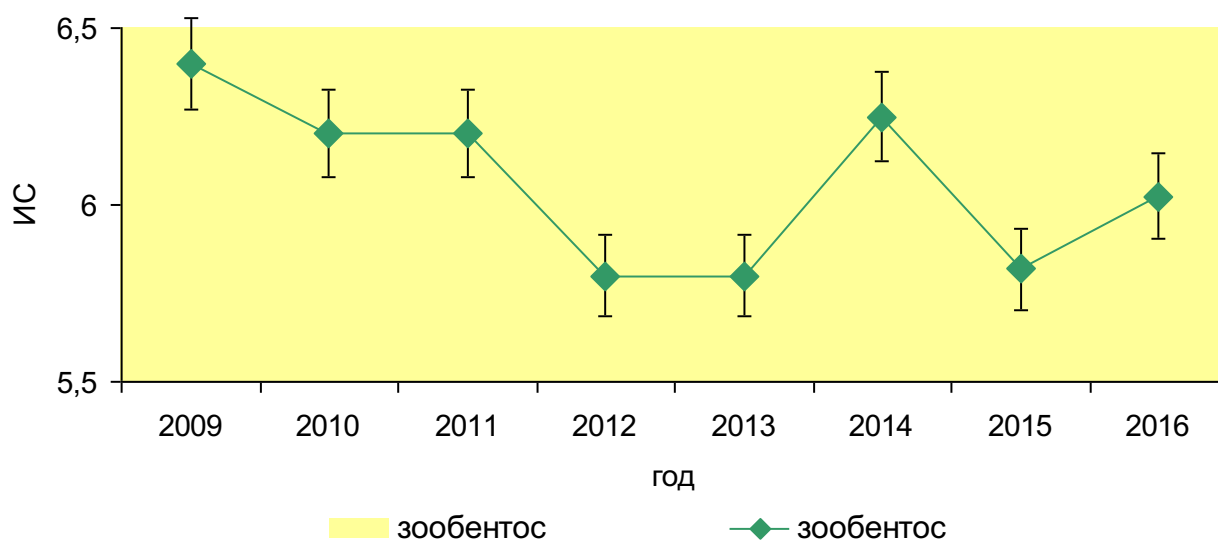
Рисунок 89. Динамика значений БИ в 2009-2016 р. Селенга
