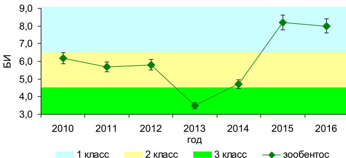
Рисунок 107. Динамика значений БИ в 2010-2016 гг., р. Мана
