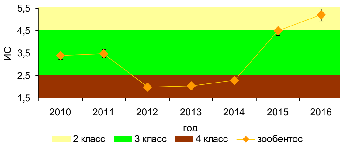
Рисунок 110. Динамика значений БИ в 2010-2016 гг., р. Березовка
