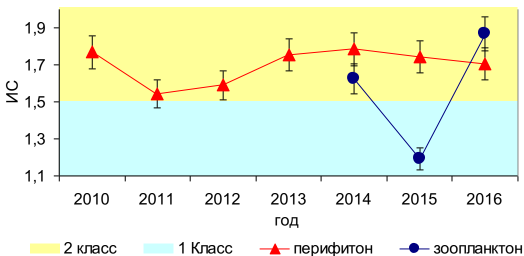
Рисунок 113. Динамика значений ИС в 2010-2016 гг., р. Базаиха
