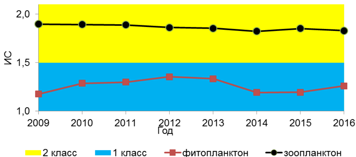
Рисунок 41. Динамика значений ИС в 2009-2016 гг., оз. Большое
