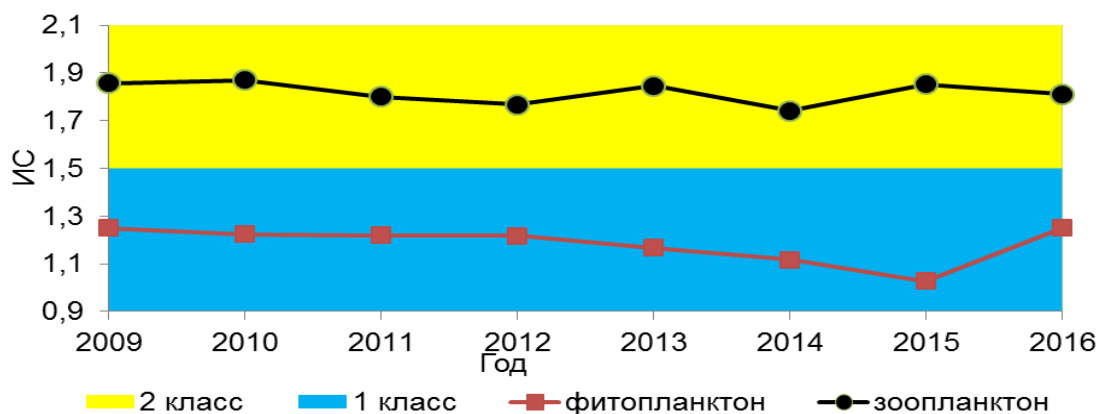
Рисунок 31. Динамика значений ИС в 2009-2016 гг., р. Вите
