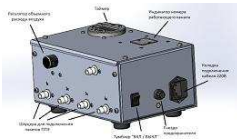
Рис. 3.1. Автоматический нагнетатель анализируемого воздуха в пробоотборные пакеты.
