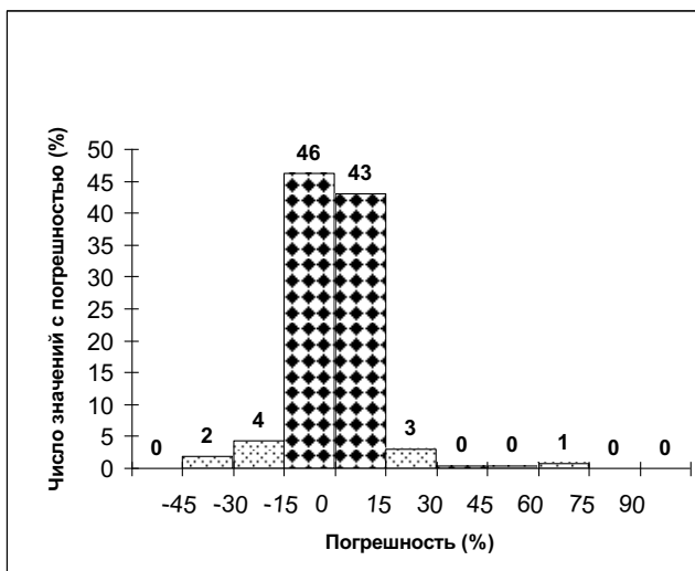
Рис.2.1 Гистограмма распределения погрешности измерения концентраций аммиака
