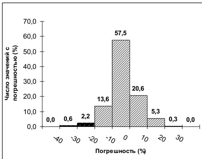
Рис.2.3 Гистограмма распределения погрешности измерения концентраций фенола
