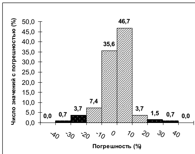
Рис.2.2 Гистограмма распределения погрешности измерения концентраций хлористого водорода
