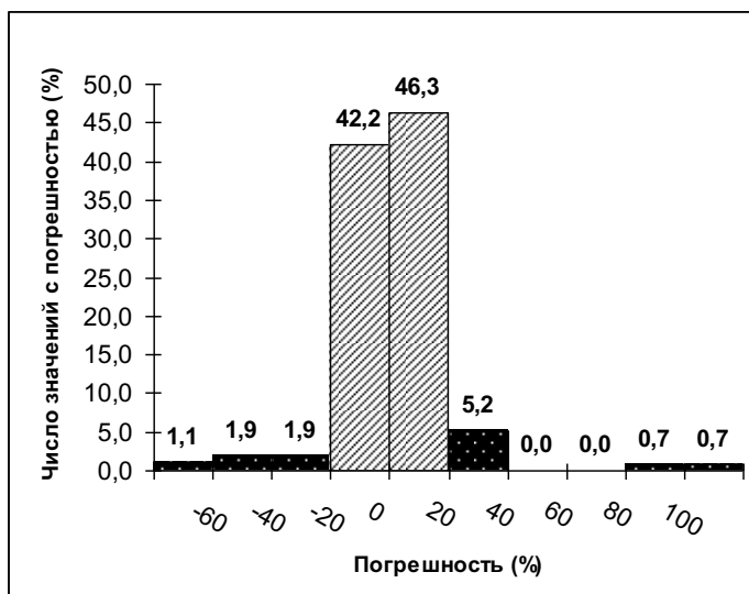
Рис.2.1 Гистограмма распределения погрешности измерения концентраций сероводорода
