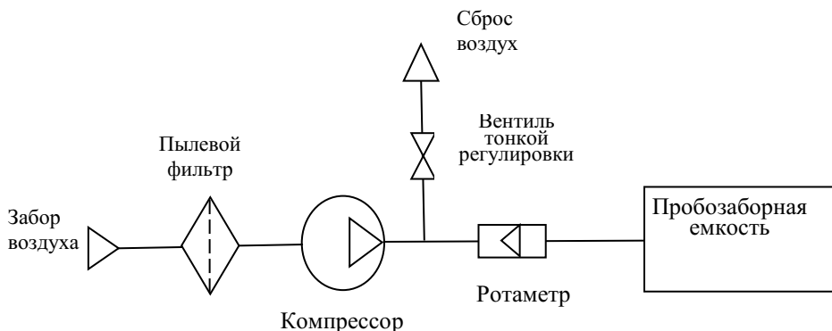
Рис. 4.1 Схема подключения пробозаборной емкости
