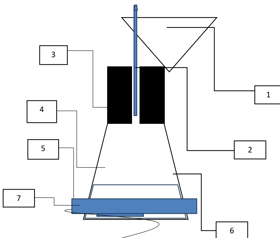
Рисунок-схема. 1 — воронка; 2 — стеклянная трубка; 3 — резиновая пробка с отверстием; 4 — стеклянная колба из термостойкого стекла вместимостью 500 см 3 ; 5 — кипелки (капиллярные трубочки); 6 — дистиллированная вода; 7 — электроплитка.
