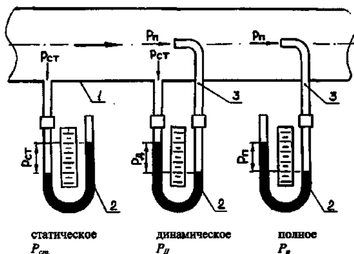
Рис. 1.4.1. Схемы измерения давлений в газоходе: 1 – газоход; 2 – U-образный манометр; 3 – напорная трубка.
