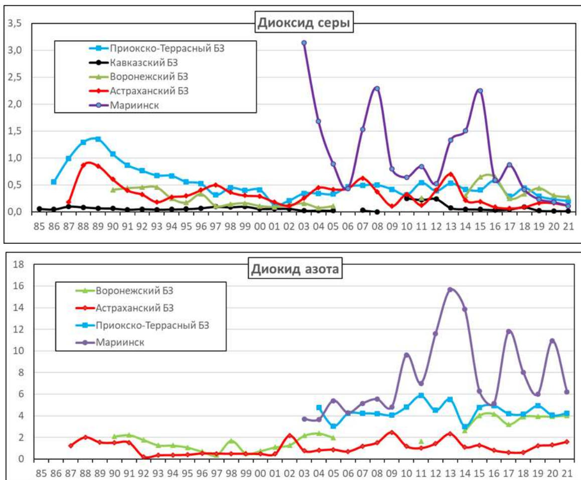
Рис. 1.1.2. Изменение фоновое содержания диоксида серы и диоксида азота в атмосферном воздухе фоновых районов (мкг/м 3 ) за многолетний период (геофизические года)
