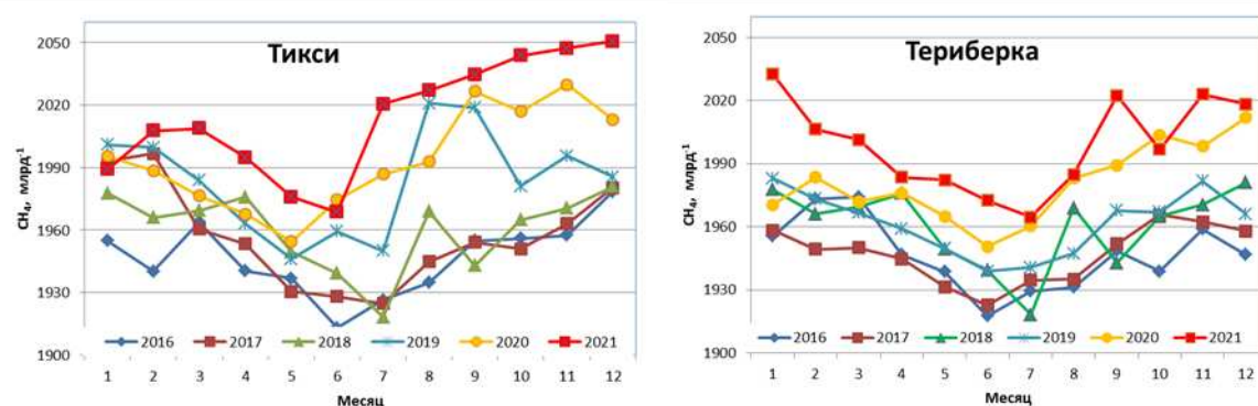
Рис. 1.2.1.2. Сезонный ход концентрации \text{CH}_4 на станциях Тикси и Териберка
