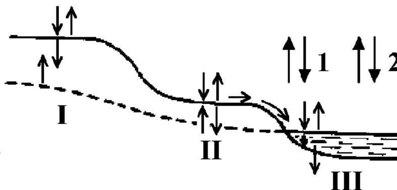
Рис.1. Схема основных типов элементарных ландшафтов по Б. Б. Побынову.
