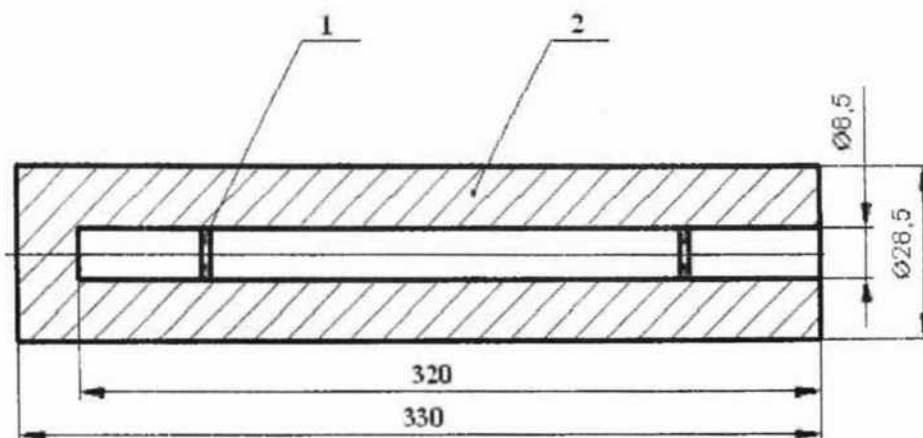
Рисунок Д.1 - Термостабилизирующий стакан для датчика HMP155
