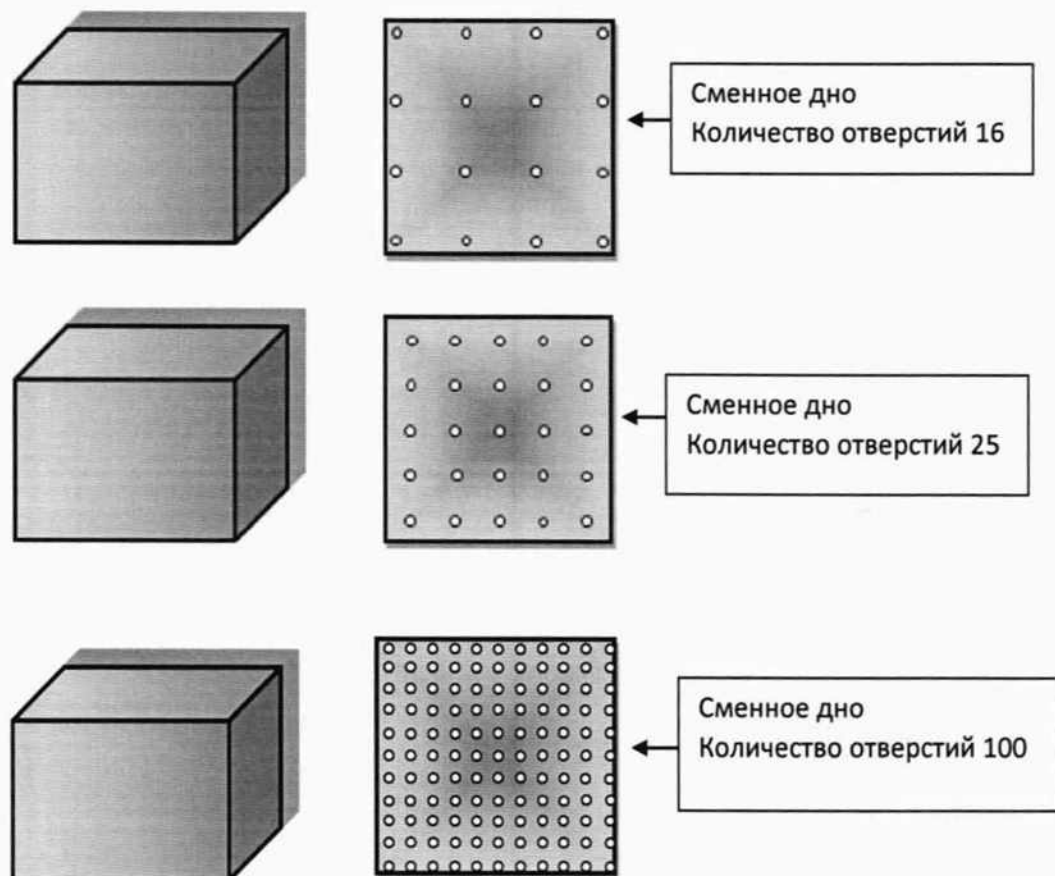
Рисунок 2 – Общий вид устройств каплеобразования
