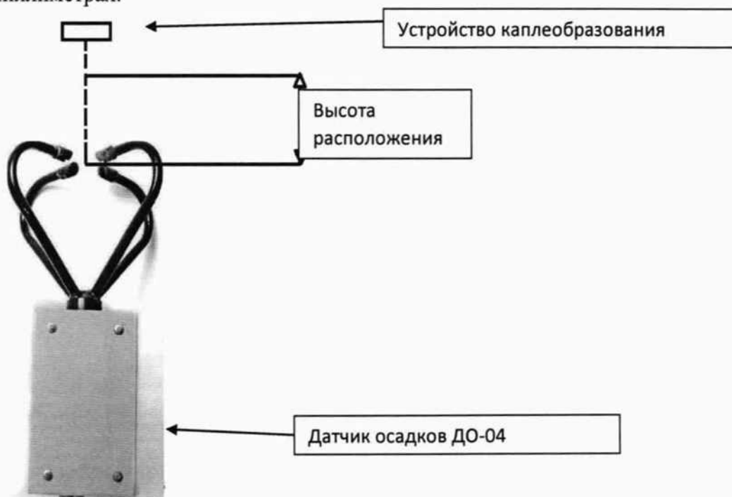
Рисунок 1 – Схема расположения устройства каплеобразования
