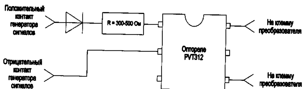
Рис. 1 Схема подключения генератора к преобразователю ИСО-1
