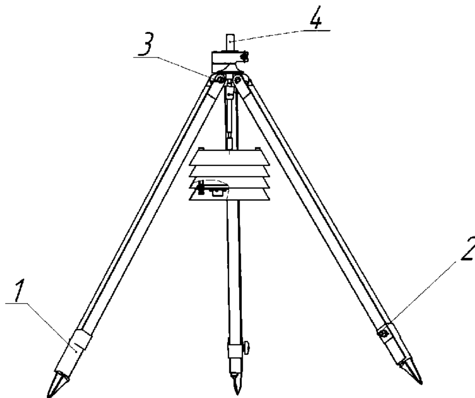
1 - тавр; 2 - зажим; 3 - барашек; 4 – опора.
