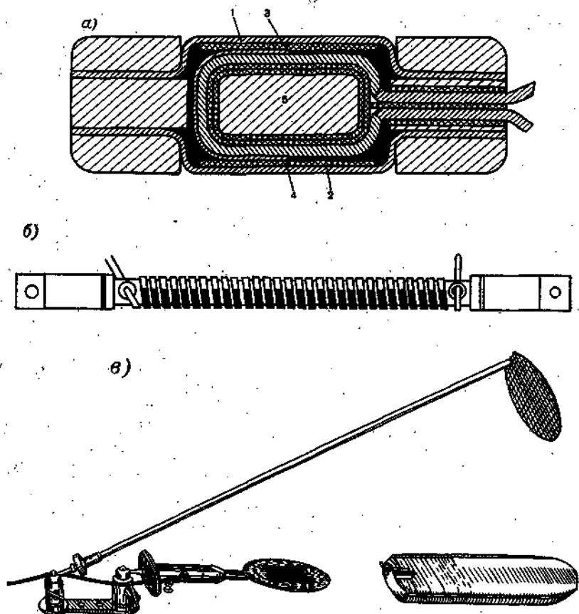
Рис. 7.11. Термoeлектрический балансомер М-10.
