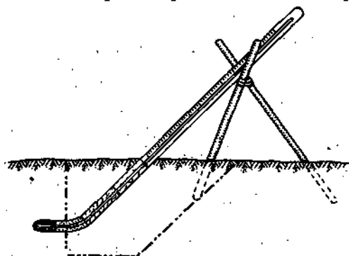
Рис. 2.39. Установка коленчатого термометра (Савинова).
