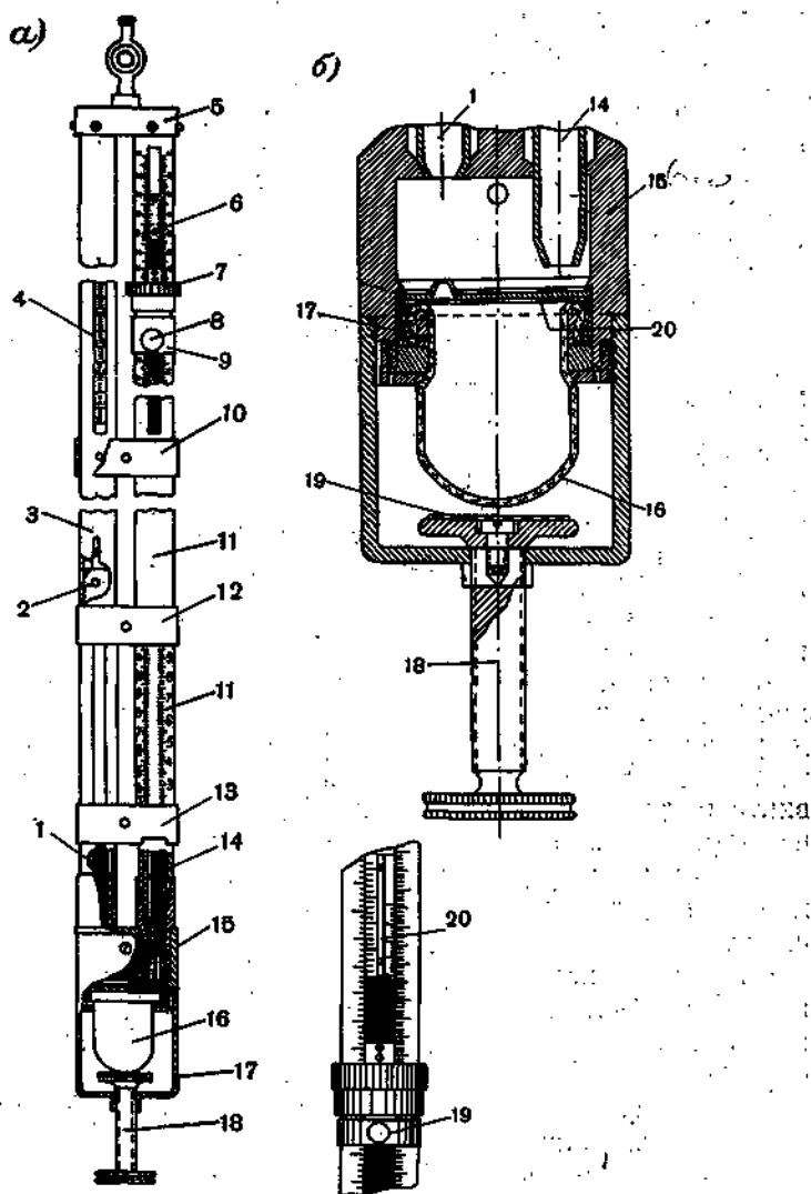
Рис. 3.9. Испекторский барометр.
