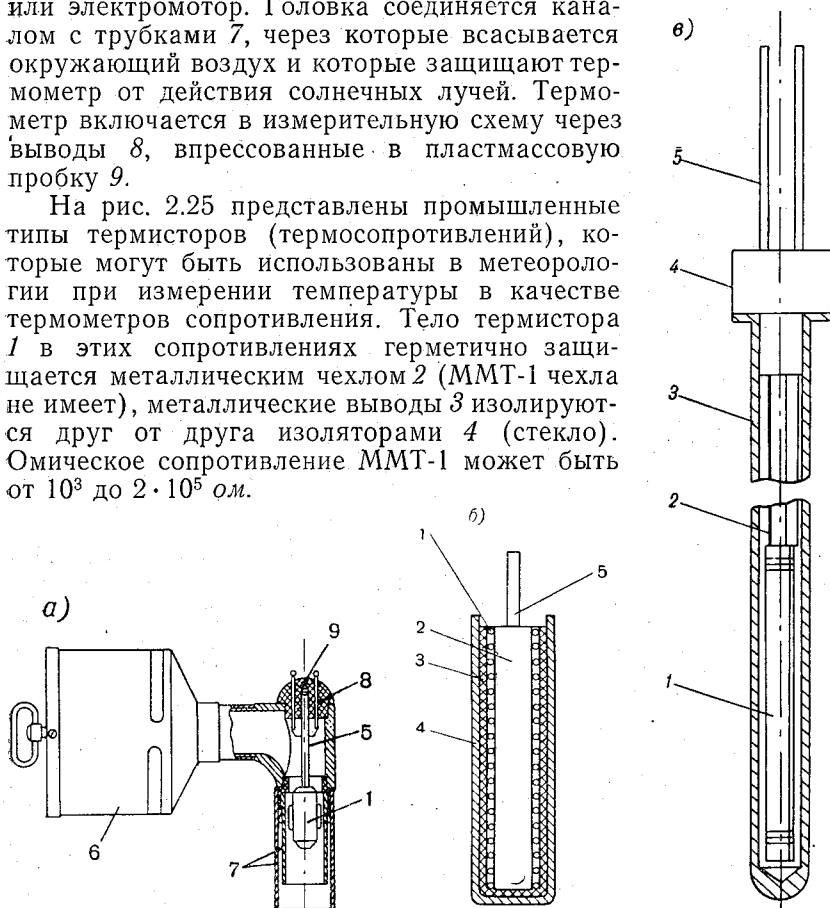
Рис. 2.24. Термометры сопротивления.
