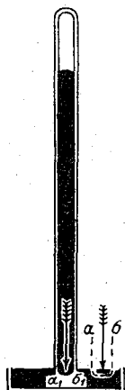
Рис. 3.1. Схема чашечного барометра.
