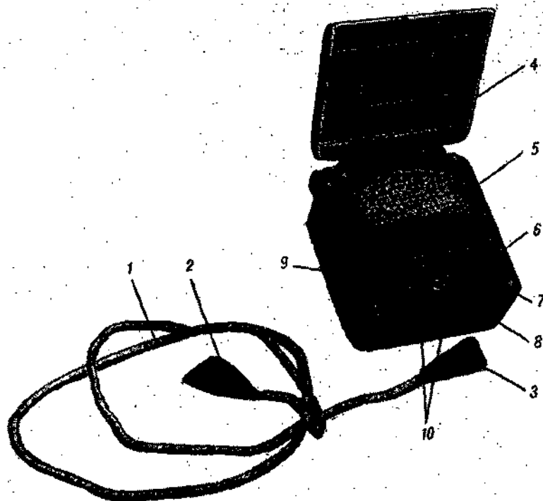
Рис. 2.27. Термометр АМ-2М.
