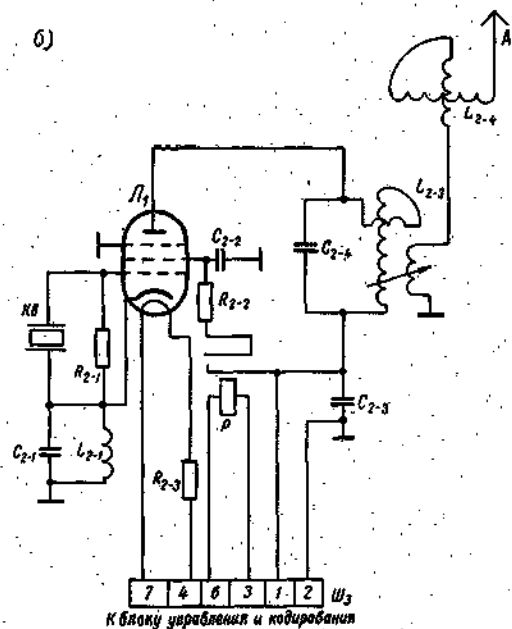
Рис. 12.39. Радиопередатчик АРИВ.
