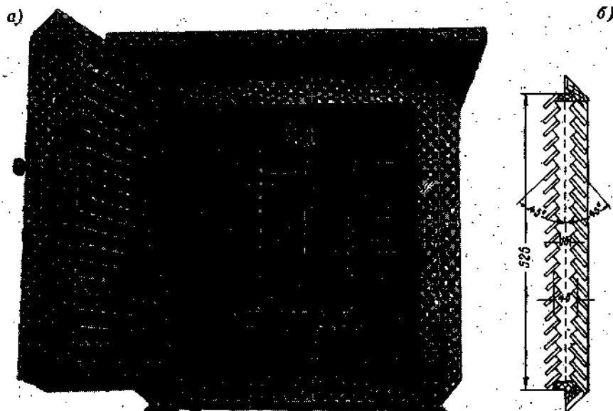
Рис. 2.34. Психрометрическая жалюзийная будка.
