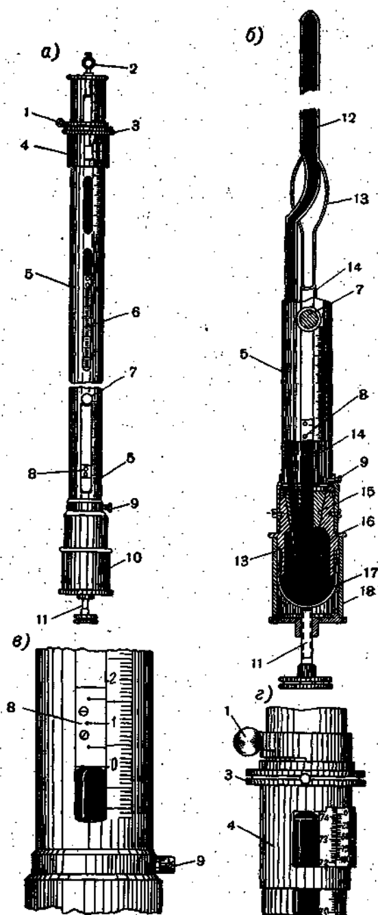
Рис. 3.7. Контрольный барометр.
