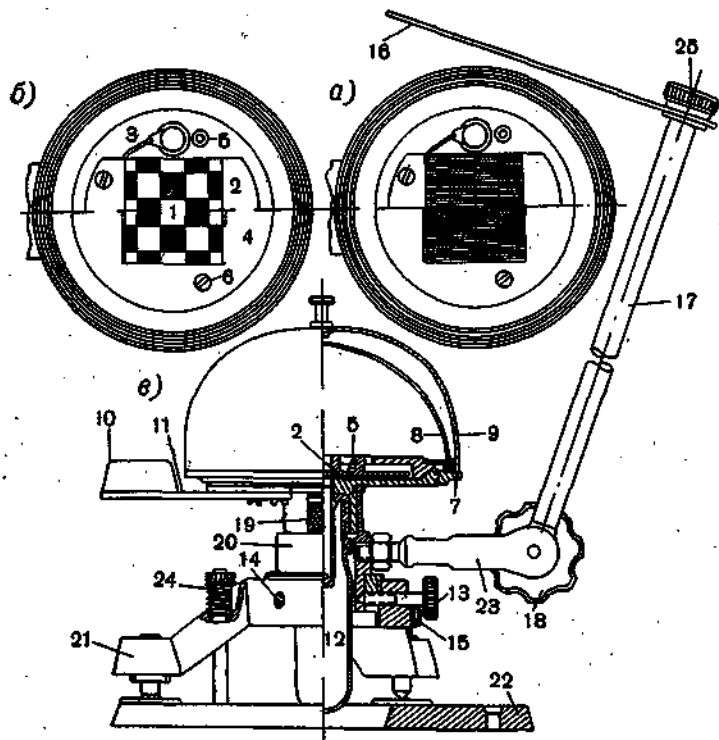
Рис. 7.7. Пиранометр ПЗ×3.
