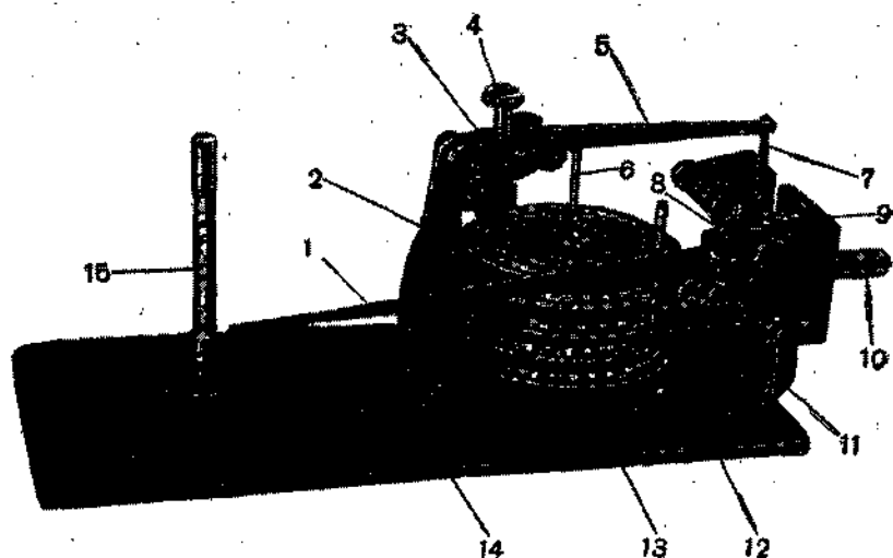
Рис. 3.18. Механизм барографа.
