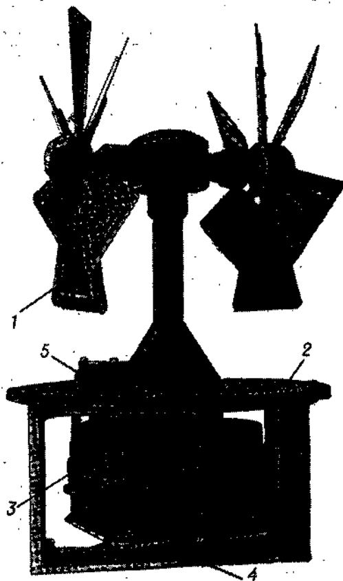
Рис. 12.35. Румбометр АРИВ.
