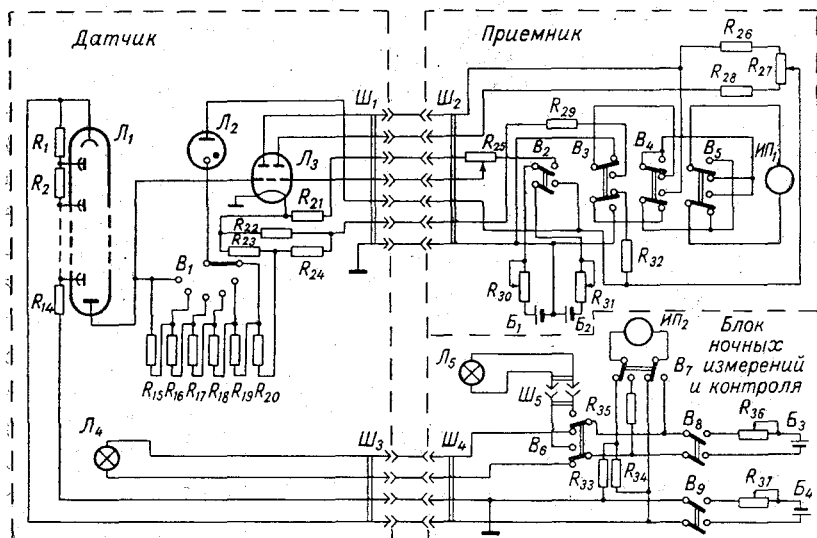
Рис. 7.17. Принципиальная электрическая схема озонометра.
