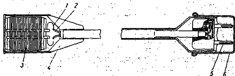
Рис. 2.28. Датчик термометра.
