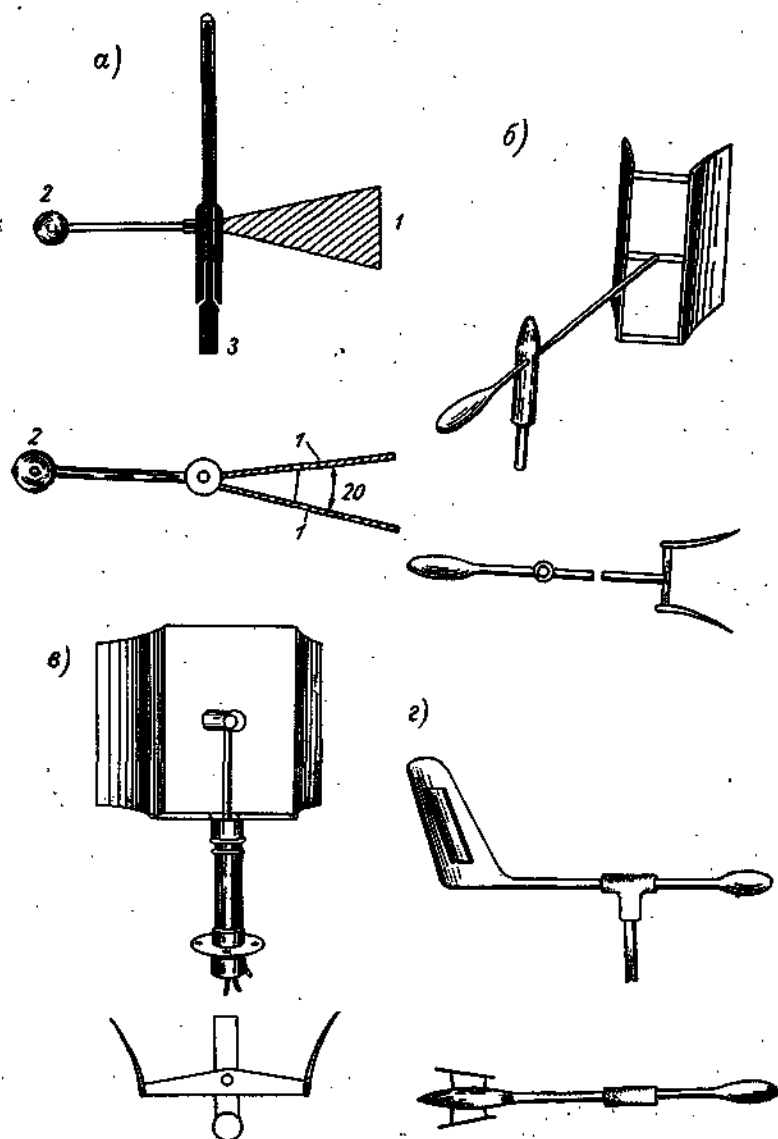
Рис. 8.2. Флогарки.
