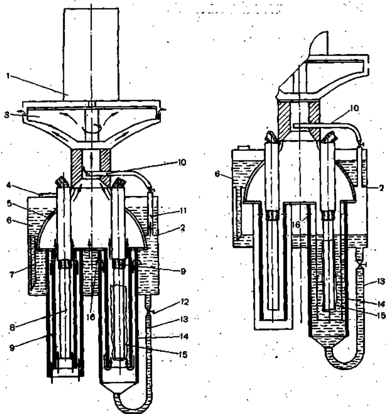
Рис. 12.14. Психрометр.
