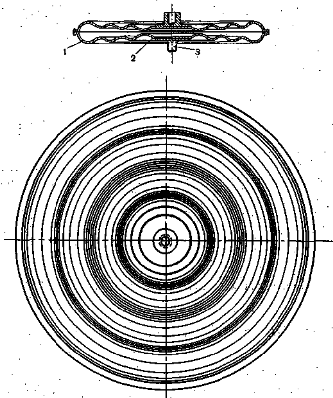
Рис. 3.11. Мембранная коробка.
