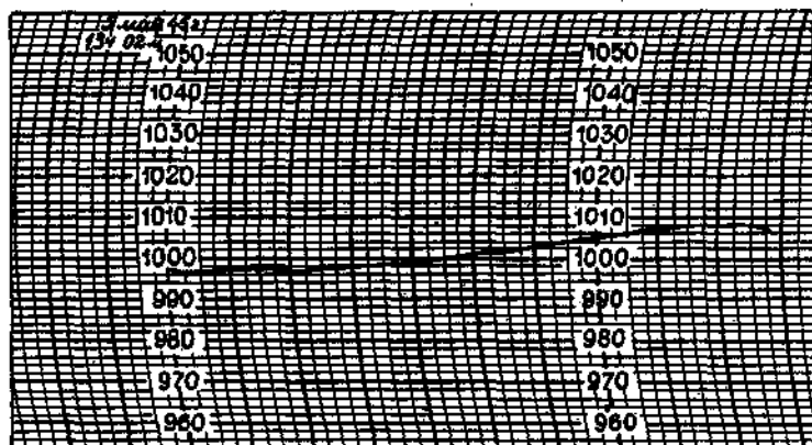
Рис. 3.20. Лента барографа.
