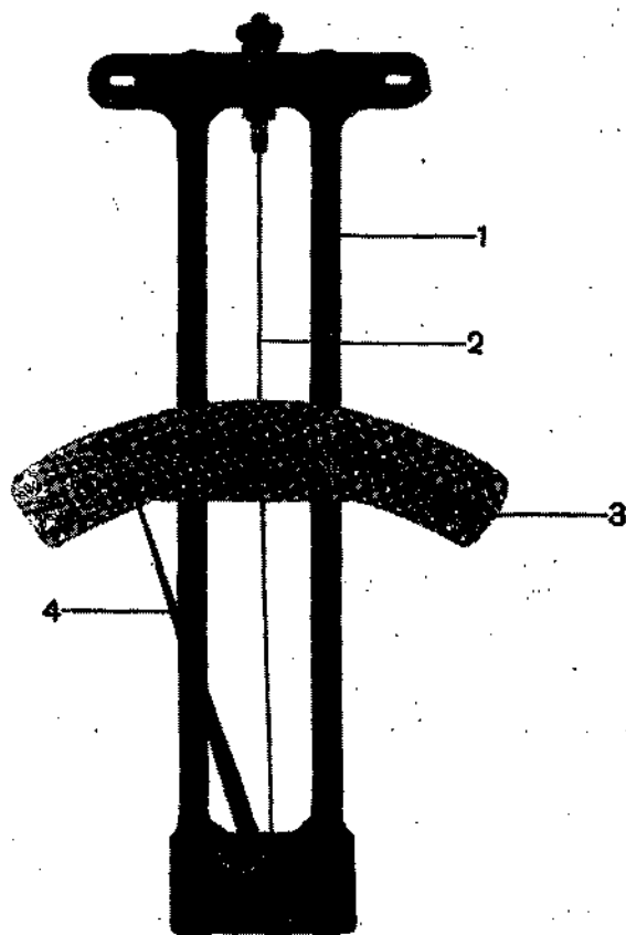
Рис. 4.5. Волосной гигрометр.
