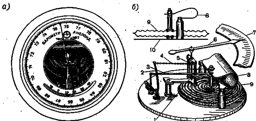
Рис. 3.12. Анероид.
