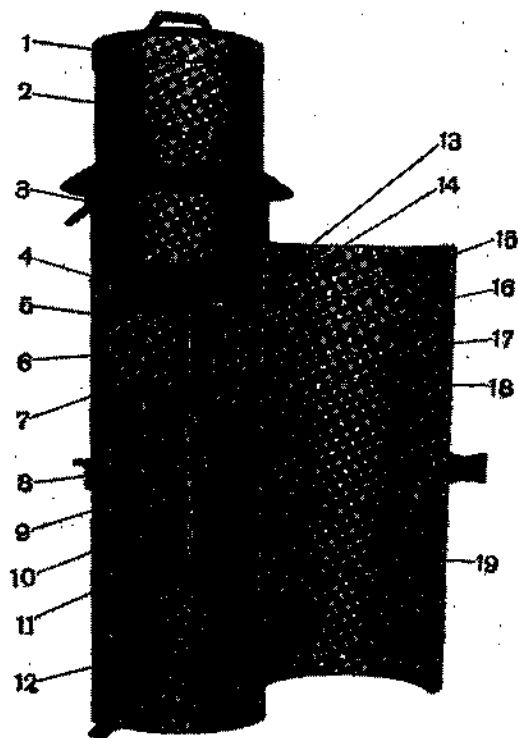
Рис. 5.9. Плювиограф.
