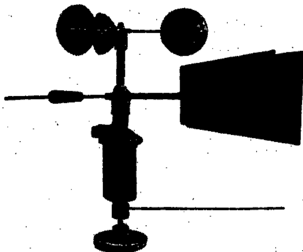
Рис. 8.25. Датчик М-12.
