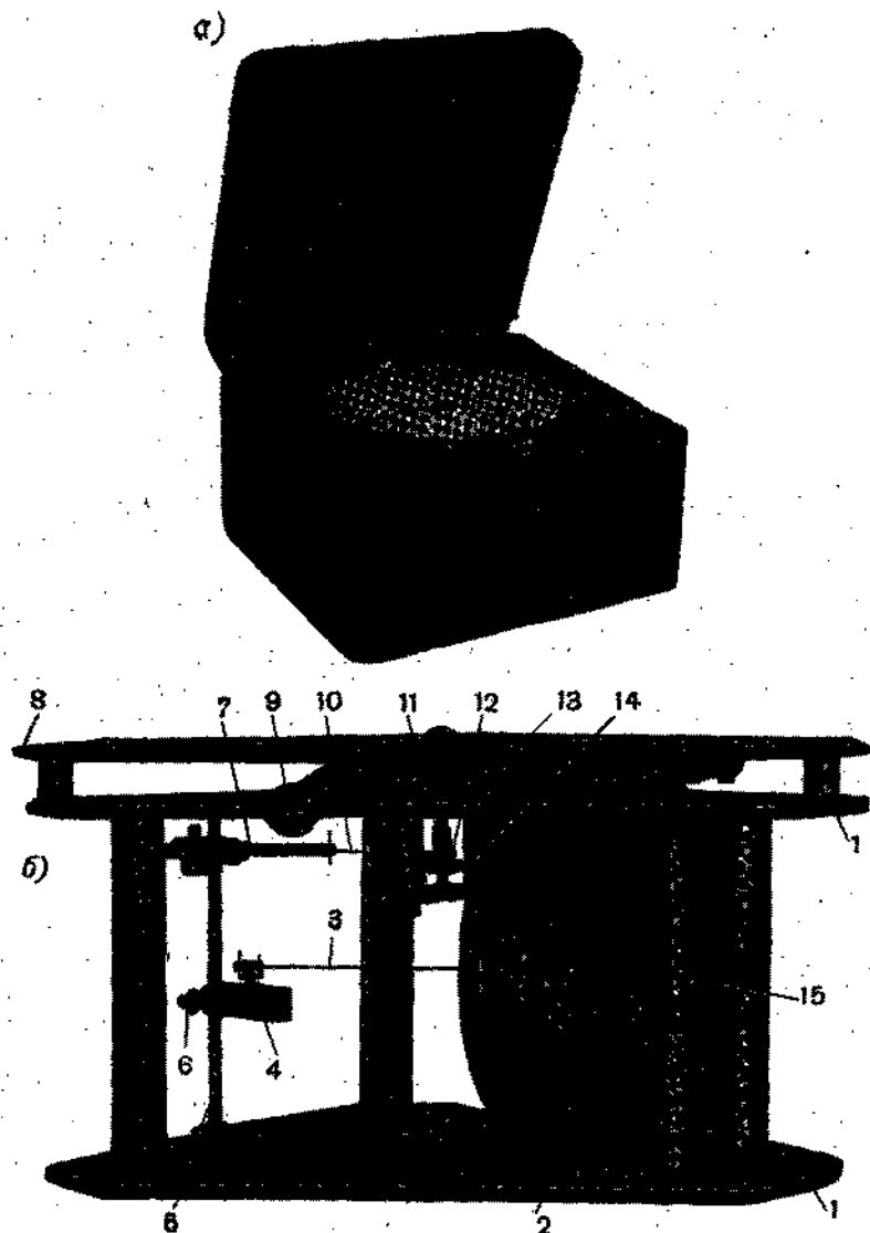
Рис. 3.13. Анероид БАМ.
