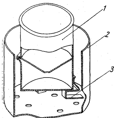
Рис. 6.7. Дождемер ГГИ-500.
