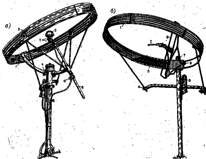
Рис. 7.13. Теневые кольца (поставлены по широте 60^\circ ).
