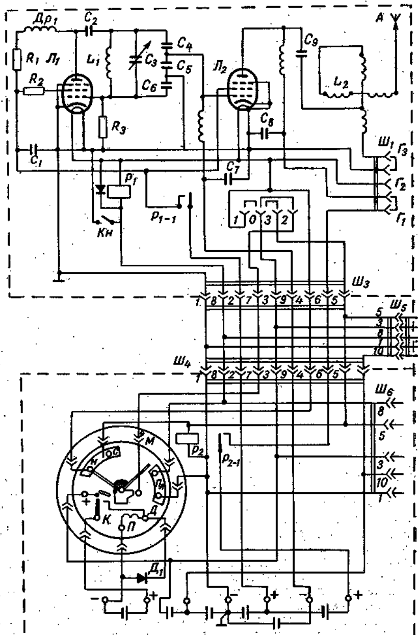
Рис. 1248. Схема радиопередатчика и блока управления ДАРМС.
