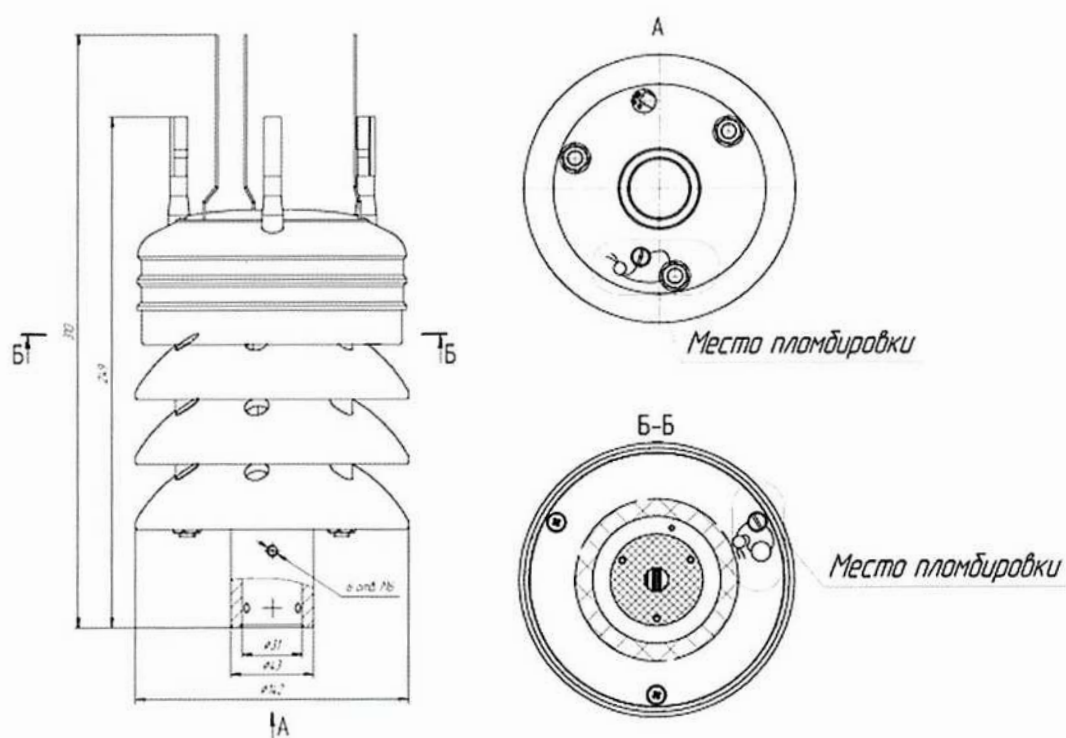
Рисунок 2 – Схема пломбировки метеостанции Перископ-М
