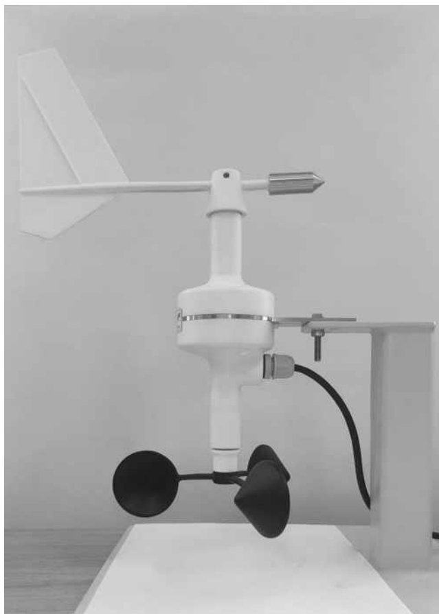
Рисунок 1 – Общий вид датчика
