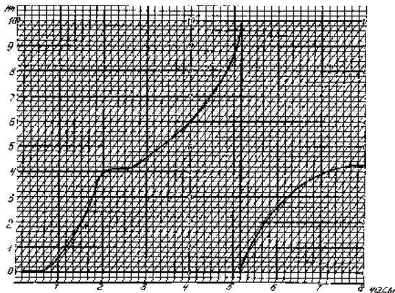
Рисунок 2 – Диаграммный бланк плувиографа П-2М с образцом записи
