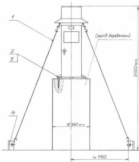
Рисунок 3 – Установка плювиографа П-2М на месте эксплуатации
