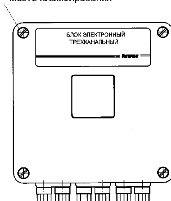
Рисунок 2 – Место пломбирования блока электронного трехканального
