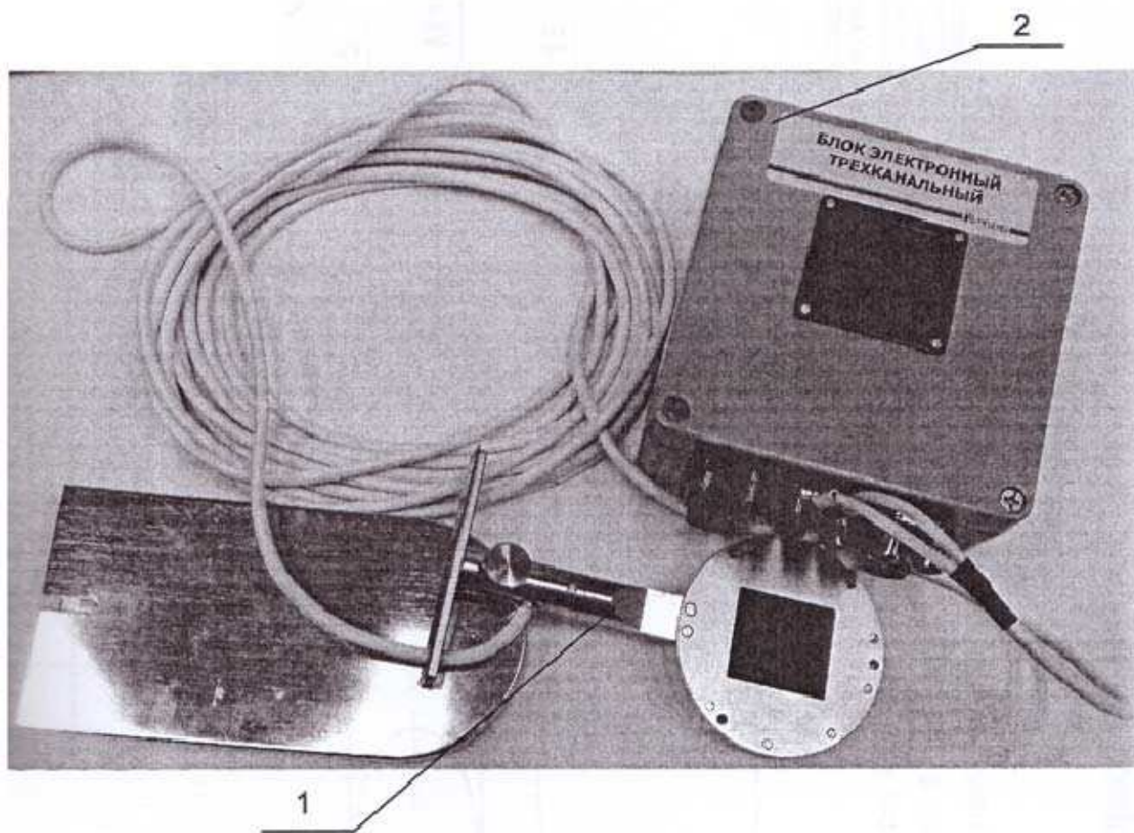
Рисунок 1 – Общий вид балансомеров ПЕЛЕНГ СФ-08
