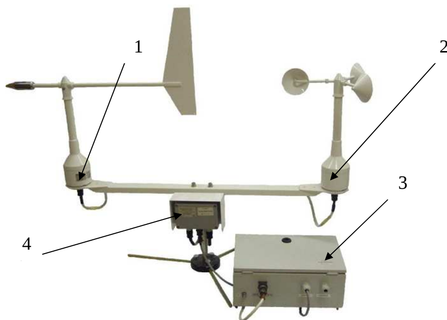
1 - румбометр, 2 - анемометр, 3 - блок питания, 4 - блок измерения
