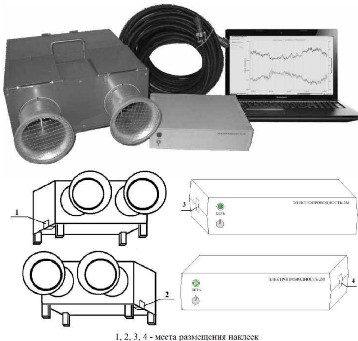
Рисунок 1 – Общий вид измерителя «Электропроводность-2М» и места размещения наклеек
