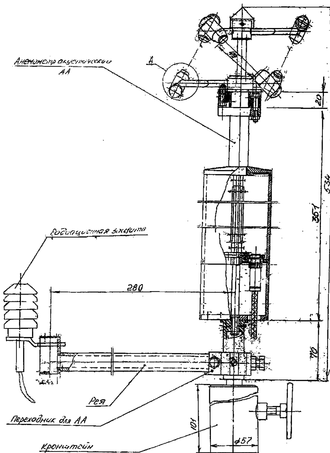
Рисунок 2 - Сборочный чертеж АА с переходником, реей и кронштейном
