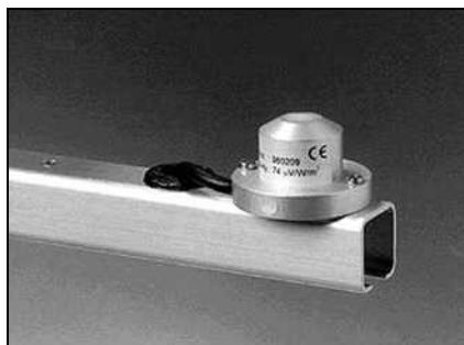
Рисунок 65 Пиранометр QMS101
