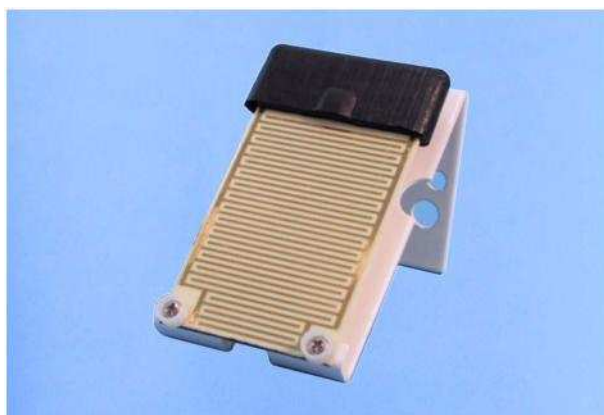
Рисунок 79 Пластинчатый датчик влажности QLW101
