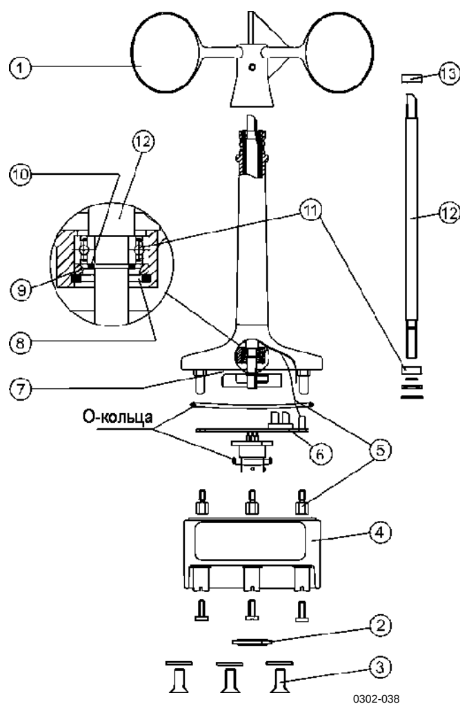
Рисунок 134 Блок WAA151
