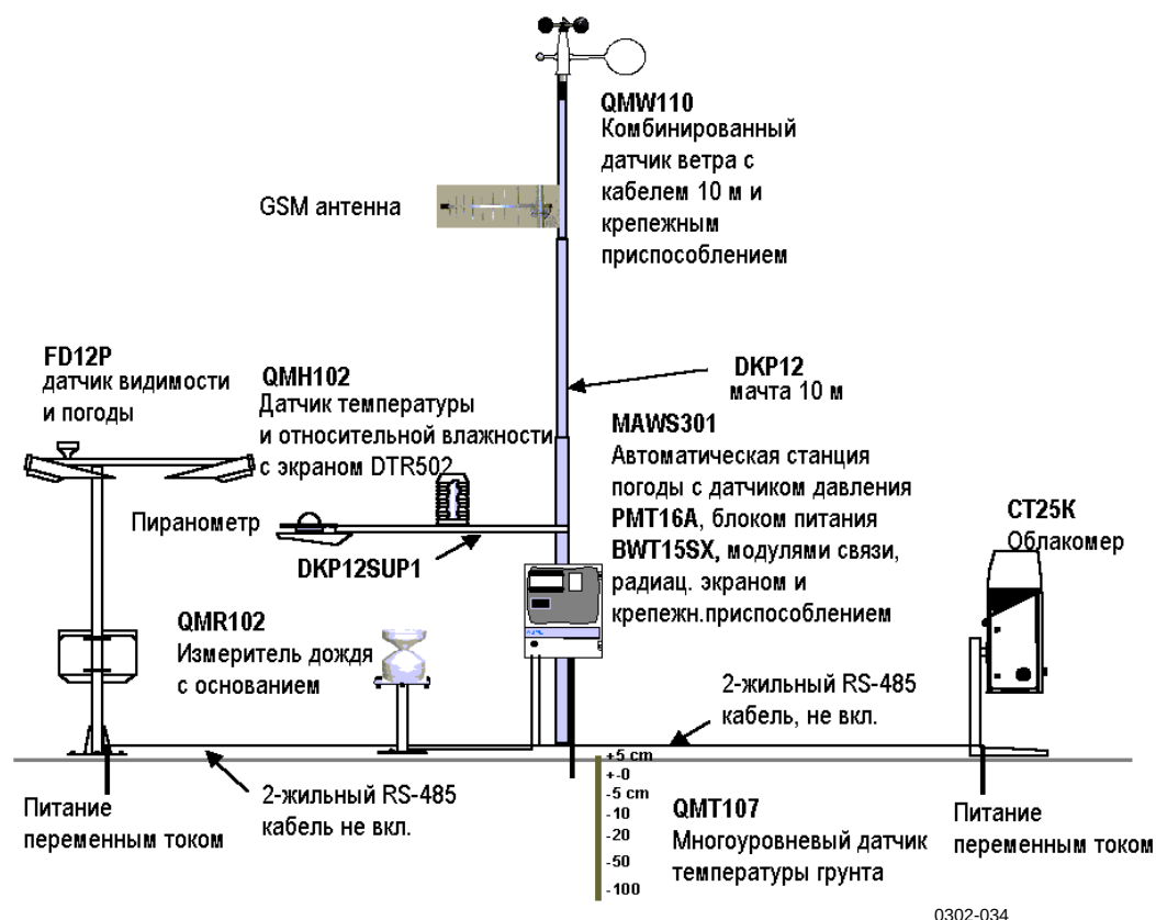
Рисунок 7 Объединенная система MAWS301
