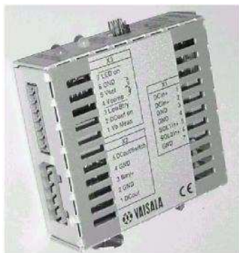
Рисунок 29 Регулятор батареи QBR101B
