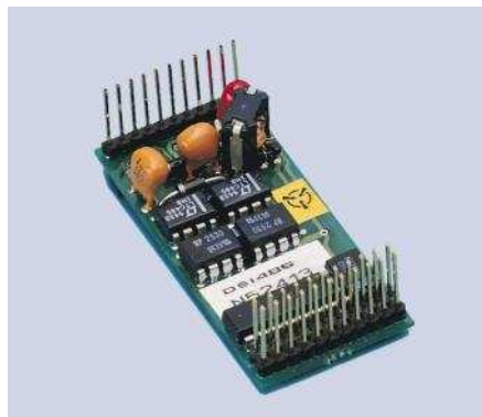
Рисунок 35 Двойной изолированный модуль DSI486
