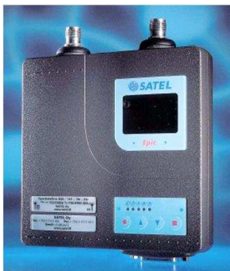
Рисунок 42 Радиомодем Sateline 3AS Epic с дополнительным дисплеем
