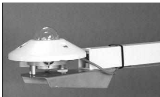
Рисунок 67 Пиранометр CM6B
