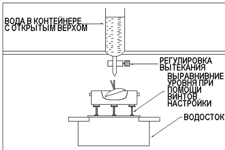
Рисунок 140 Динамическая калибровка
