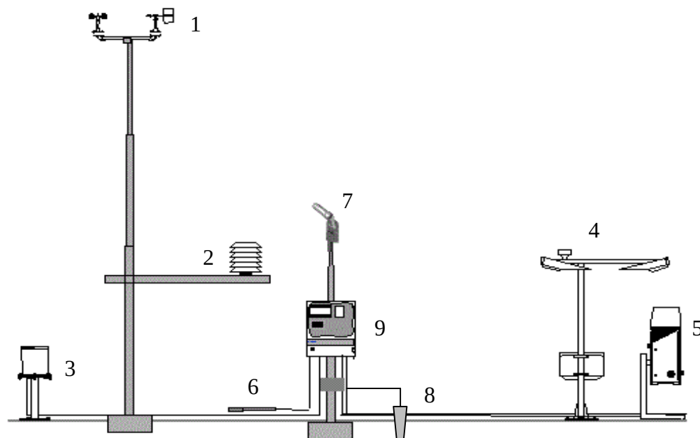
Рис.1 Общий вид станций погодных автоматических MAWS. 1 – измерительные преобразователи скорости и направления воздушного потока; 2 – измерительные преобразователи температуры и влажности воздуха; 3 - измерительные преобразователи количества осадков; 4 - измерительные преобразователи метеорологической оптической дальности; 5 - измерительные преобразователи высоты облачности; 6 - измерительные преобразователи температуры воды (почвы); 7 - измерительные преобразователи энергетической освещенности и продолжительности солнечного сияния; 8 - измерительные преобразователи уровня воды (гидростатического давления); 9 – центральная система и модуль электропитания в защитном корпусе.
