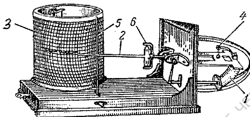
Рис. 2.3. Термограф.
