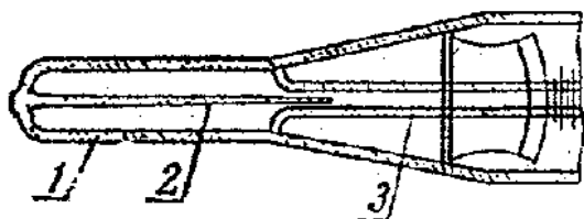
Рис. 2.1. Приспособление для сохранения максимальных показаний термометра. 1-резервуар, 2-штифт, 3-капилляр
