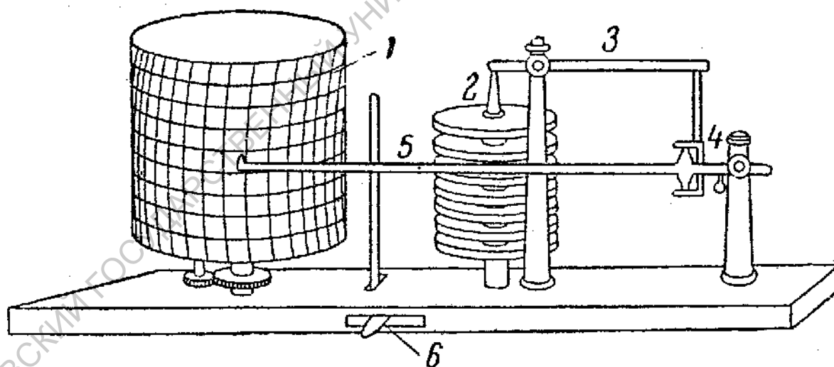
Рис. 2.10. Барограф метеорологический.
