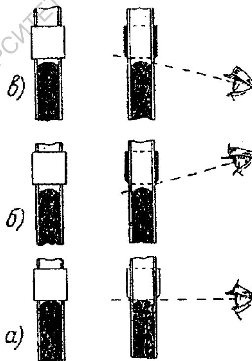
Рис. 2.9. Нониус станционного чашечного барометра. Различное положение глаза при отсчете по барометру: а)- правильное; б) и в)- неправильное
