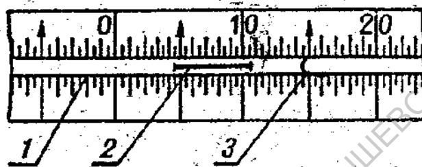
Рис.2.2. Приспособление для отсчета минимальных показаний термометра. 1-капилляр, 2-штифт, 3-мениск спирта
