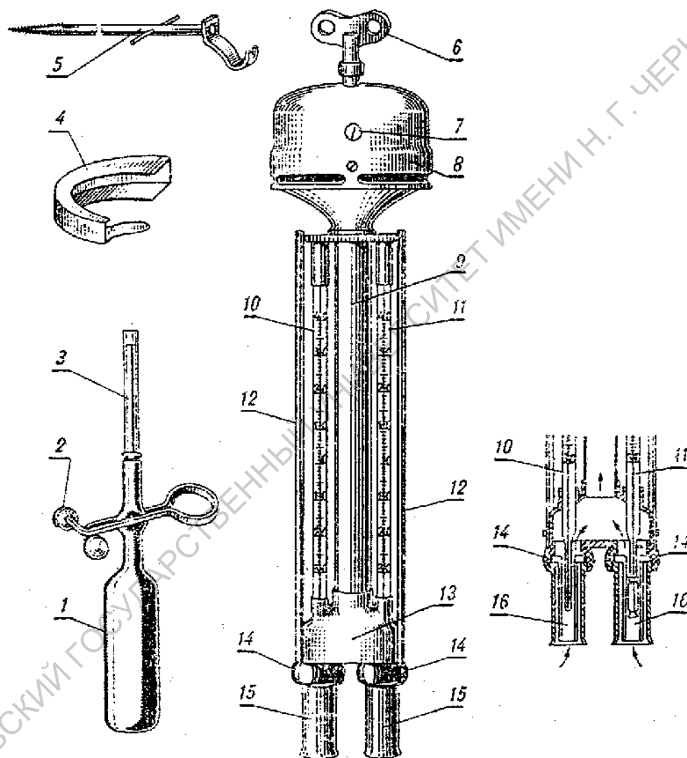
Рис. 2.6 Аспирационный психрометр МВ-4М.
